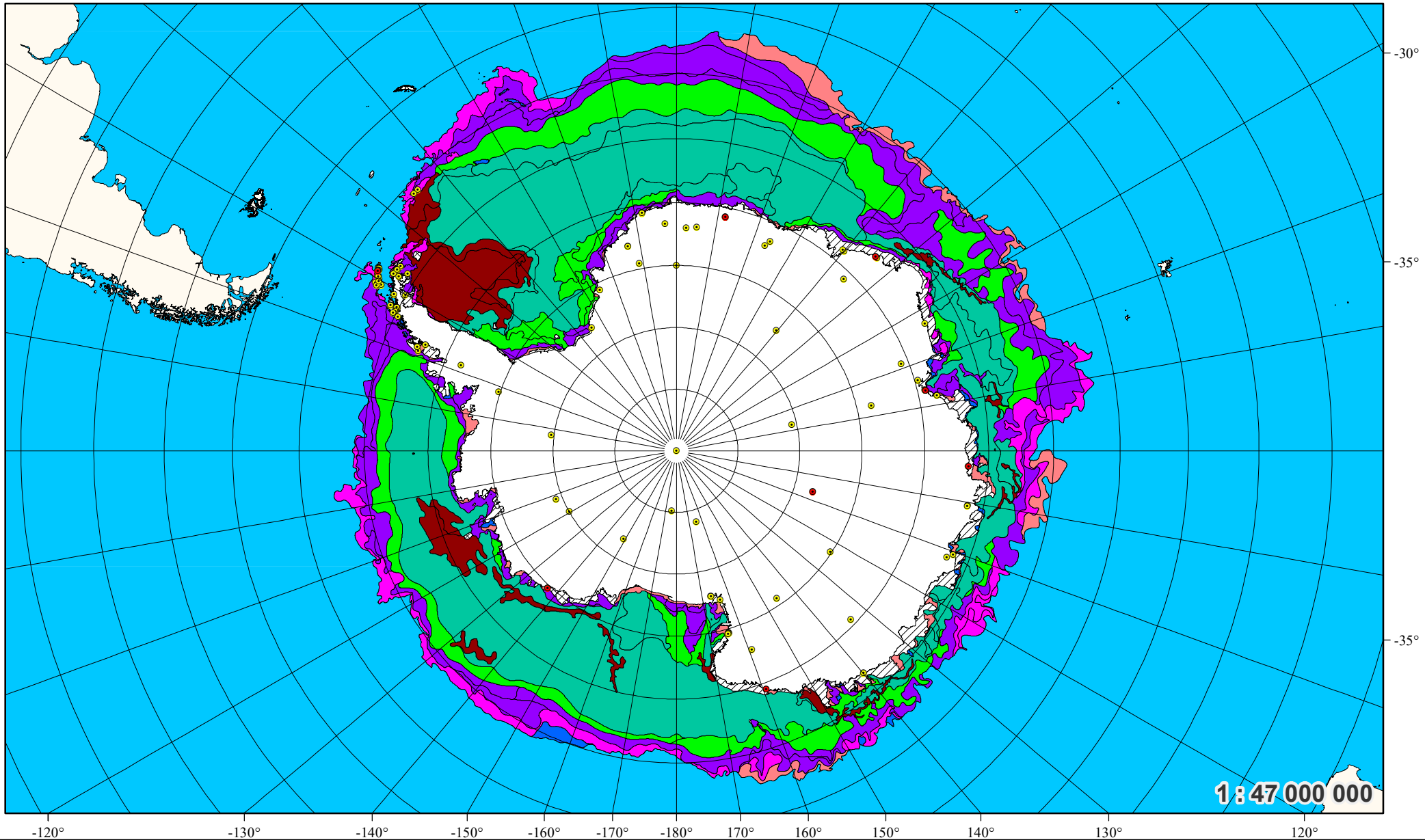
Южный океан / Southern Ocean Обзорная ледовая карта / Overview Ice Chart 01-05 октября 2023 г. / October 01-05, 2023
