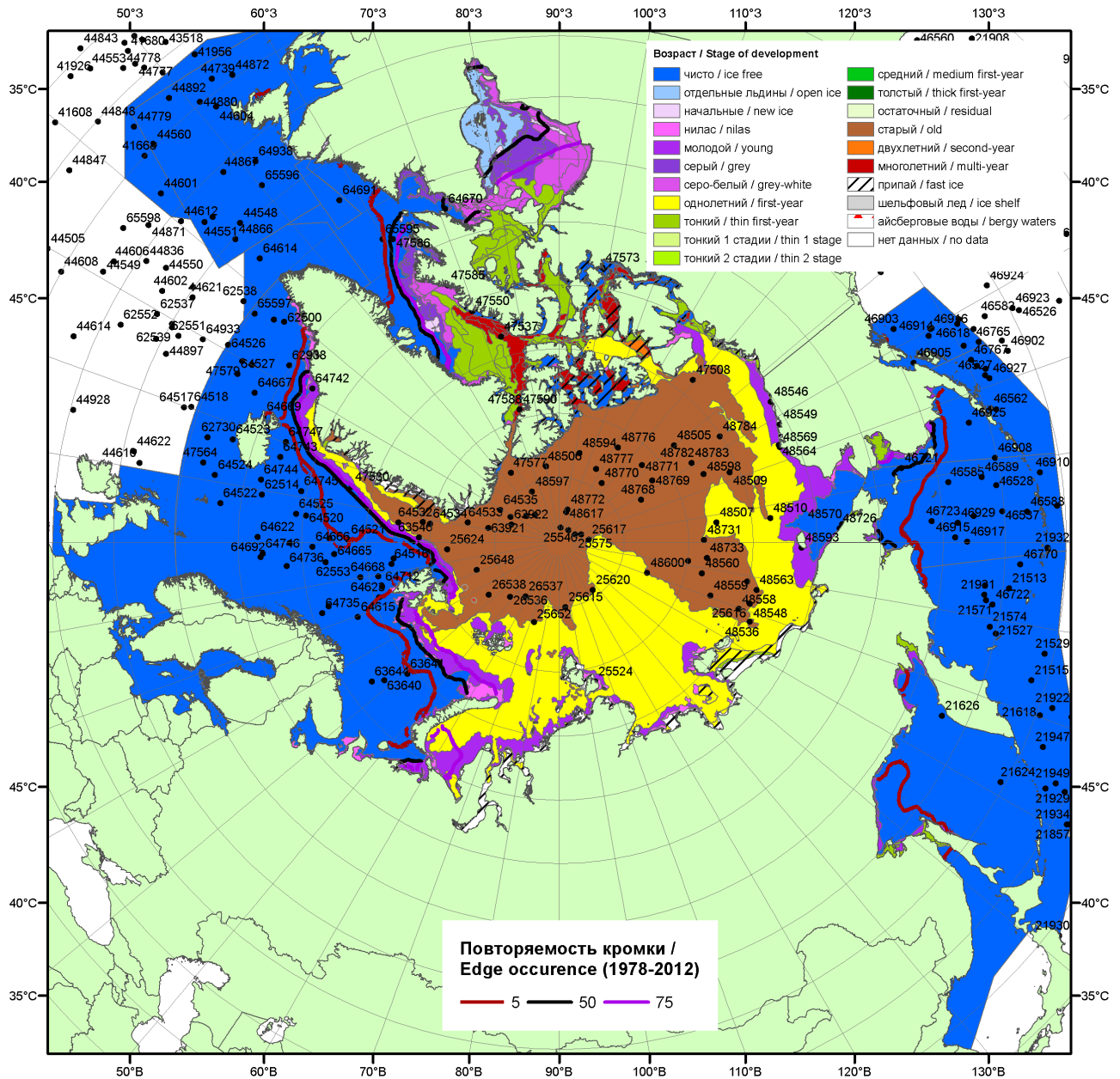
Рисунок 1а – Обзорная ледовая карта СЛО за 01.12.2014-09.12.2014 г. на основе ледового анализа ААНИИ (09.12), Национального ледового центра США (Берингово море, 04.12), Канадской ледовой службы (01.12), положение метеорологической дрейфующих буев IABP и Argos на 09.12.2014T1200+00 и повторяемость кромки за 01-05.12 за период 1978-2012 гг. по наблюдениям SSMR-SSM/I-SSMIS (алгоритм NASATEAM).
