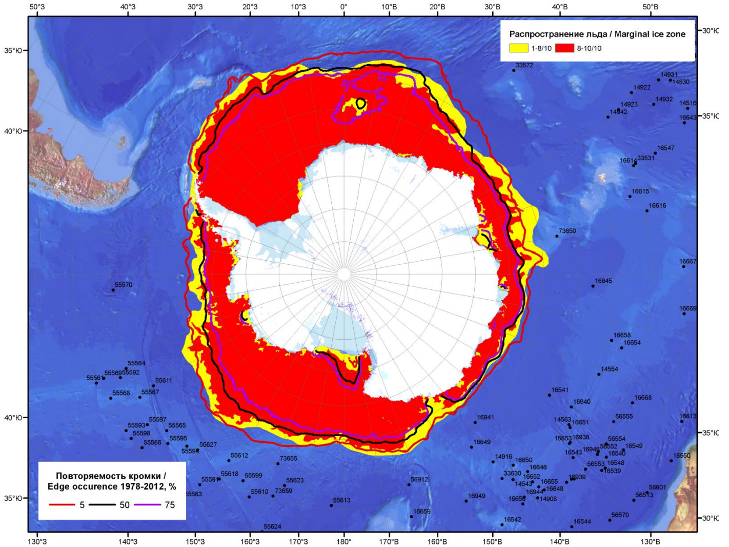
Рисунок 7а – Положение кромки льда и зон разреженных ( <8/10 ) и сплоченных ( \geq 8/10 ) льдов Южного океана за 08.12.2014 г. на основе ледового анализа Национального Ледового Центра США, положение метеорологический дрейфующих буев IABP и Argos на 09.12.2014T1200+00 и повторяемость кромки за 06-10.12 за период 1979-2012 гг. по наблюдениям SSMR-SSM/I-SSMIS (алгоритм NASATEAM)
