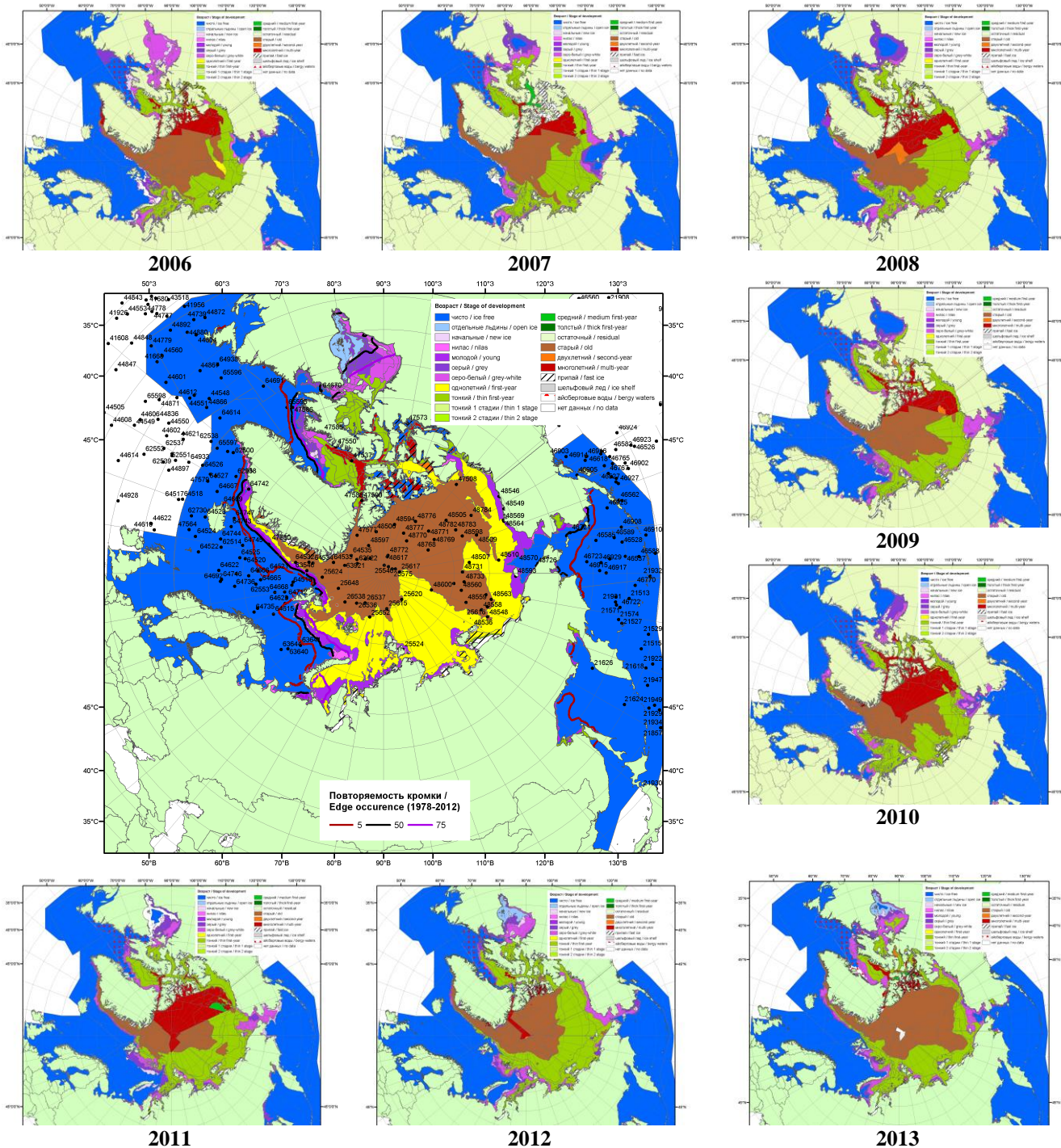
Рисунок 3 – Обзорная ледовая карта СЮ за 01.12.2014 - 09.12.2014 г. и аналогичные периоды 2006-2013 гг. на основе ледового анализа ААНИИ, Канадской ледовой службы и Национального ледового центра США.
