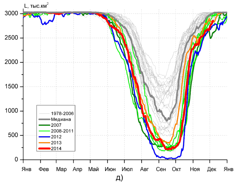
Рисунок 5 – Ежедневные оценки сезонного хода ледовитости для Северной Полярной Области и трех меридиональных секторов за период 26.10.1978 - 07.12.2014 по годам на основе расчетов по данным SSMR-SSM/I-SSMIS-AMSR2, алгоритмы NASATEAM/BOOTSTRAP: а) Северная полярная область, б) сектор 45°W-95°E (Гренландское – Карское моря), в) сектор 95°E-170°W (моря Лаптевых – Чукотское и Берингово, Охотское), г) сектор 170°W-45°W (море Бофорта и Канадская Арктика), д) Северный морской путь (Карское - Чукотское моря).
