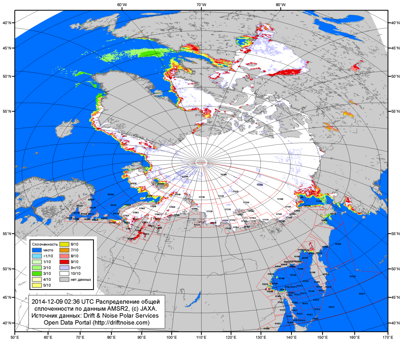
Рисунок 2а – Общая сплоченность морского льда СЛЮ и субарктических морей по данным AMSR2 на 09.12.2014 02:23UTC и границы районов ГМССБ МЕТЗОН XIII, XX и XXI.
