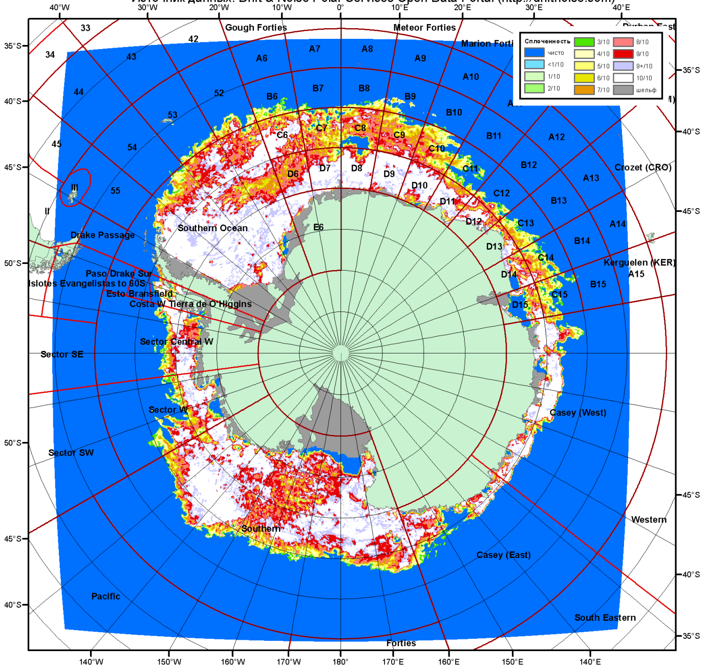
Рисунок 76 – Общая сплоченность морского льда Южного океана по данным AMSR2 на 09.12.2014 02:36UTC и границы районов ГМССБ МЕТЗОН VI, VII, X, XIV и XV.
