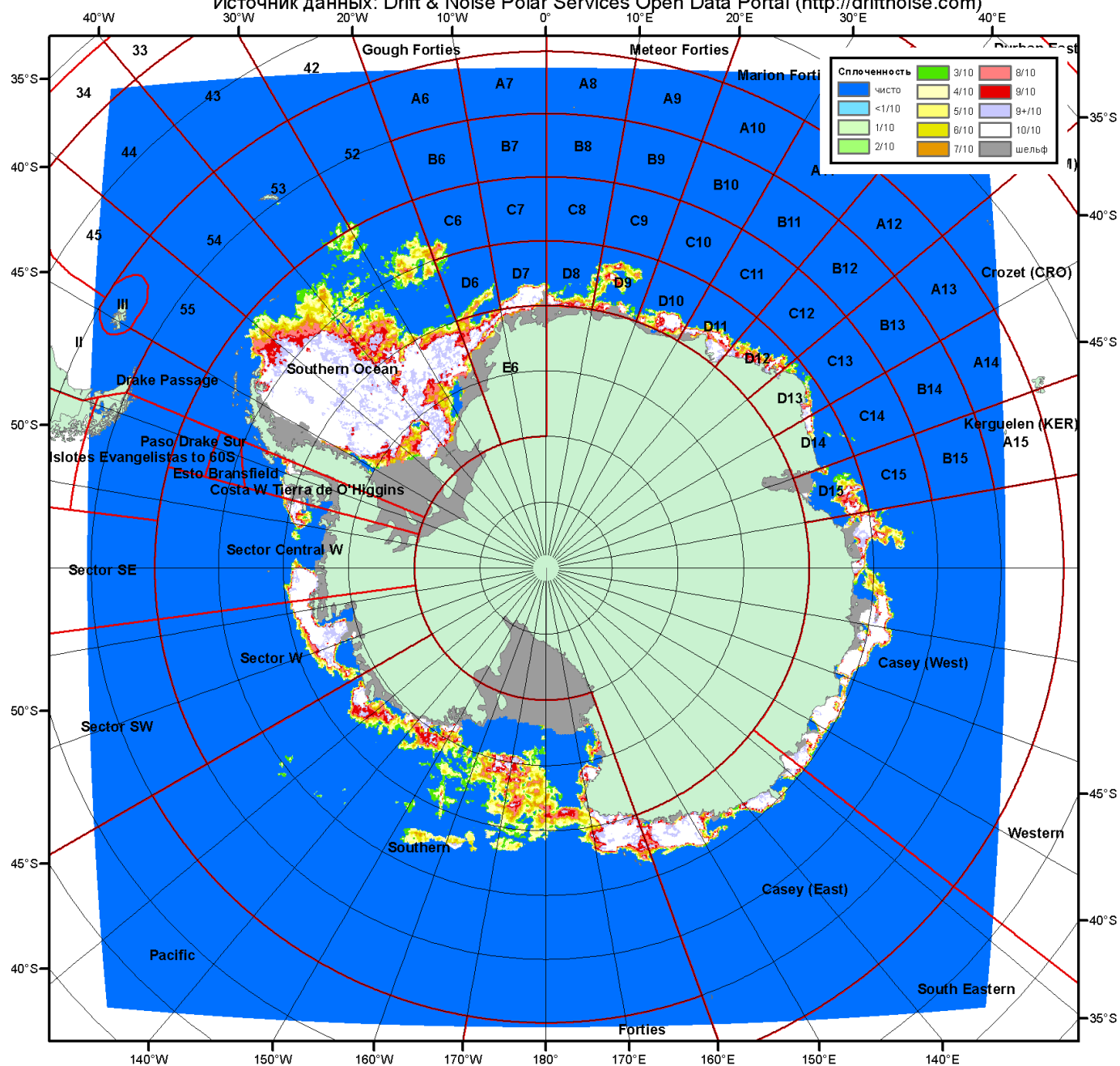
Рисунок 7в – Общая сплоченность морского льда Южного океана по данным AMSR2 на 27.01.2015 01:42UTC и границы районов ГМССБ МЕТЗОН VI, VII, X, XIV и XV.
