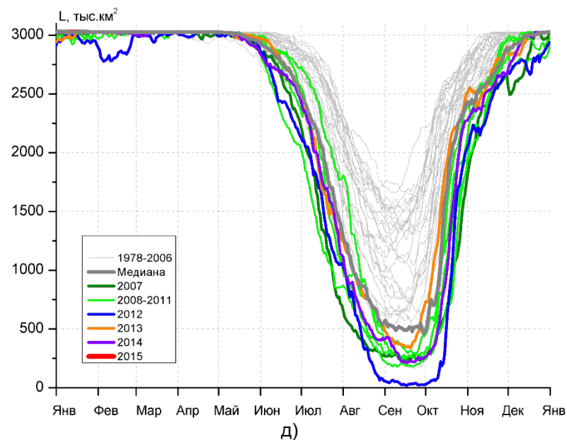
Рисунок 5 – Ежедневные оценки сезонного хода ледовитости для Северной Полярной Области и трех меридиональных секторов за период 26.10.1978 - 25.01.2015 по годам на основе расчетов по данным SSMR-SSM/I-SSMIS-AMSR2, алгоритмы NASATEAM/BOOTSTRAP: а) Северная полярная область, б) сектор 45°W-95°E (Гренландское – Карское моря), в) сектор 95°E-170°W (моря Лаптевых – Чукотское и Берингово, Охотское), г) сектор 170°W-45°W (море Бофорта и Канадская Арктика), д) Северный морской путь (Карское - Чукотское моря).
