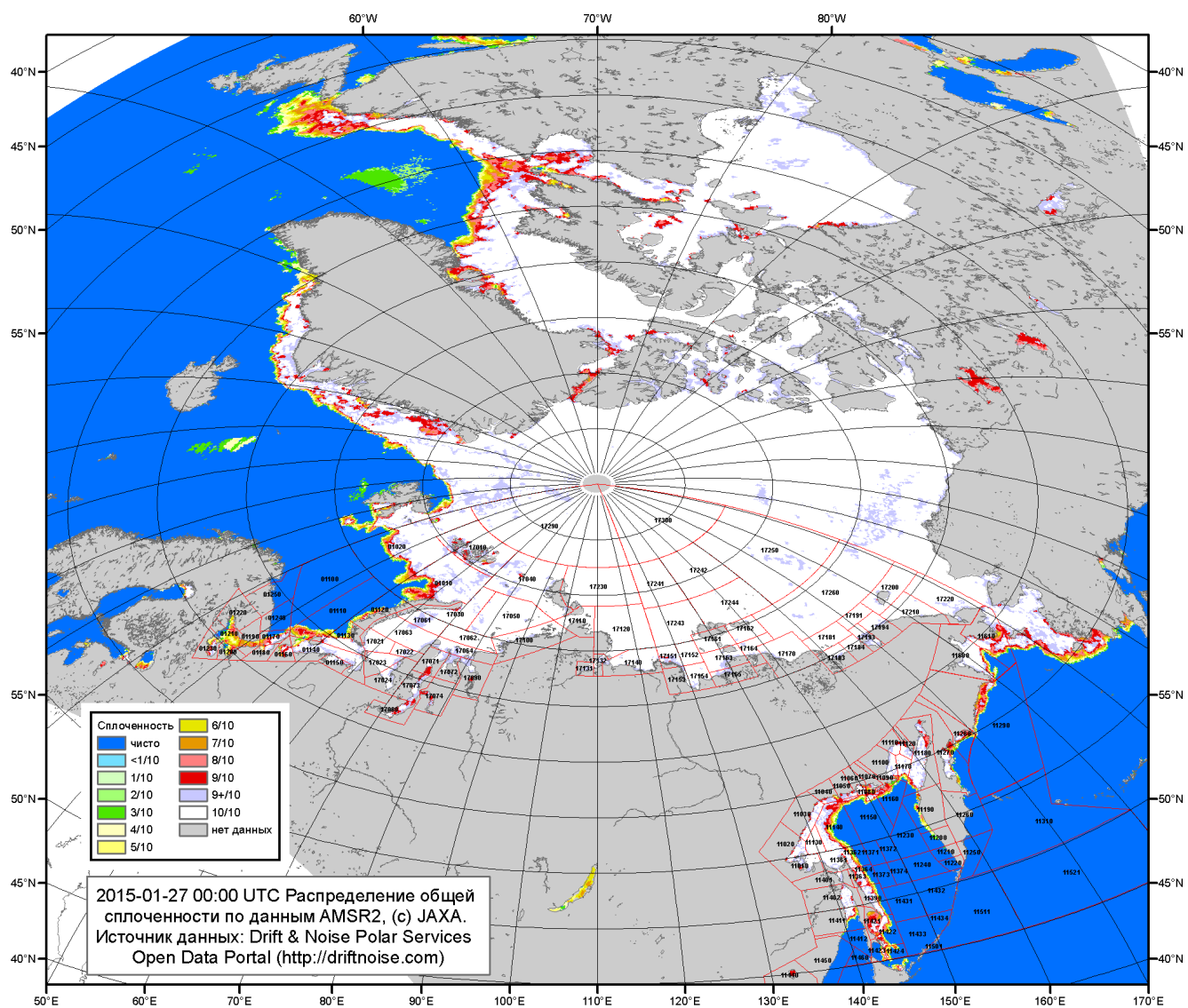
Рисунок 2а – Общая сплоченность морского льда СЛО и субарктических морей по данным AMSR2 на 27.01.2015 00:00UTC и границы районов ГМССБ МЕТЗОН XIII, XX и XXI.
