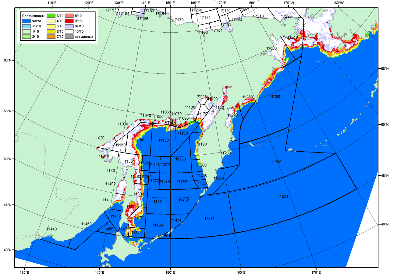
Рисунок 2в – Общая сплоченность морского льда дальневосточных морей по данным AMSR2 на 27.01.2015 00:00UTC и границы районов ГМССБ МЕТЗОНЫ XIII.
