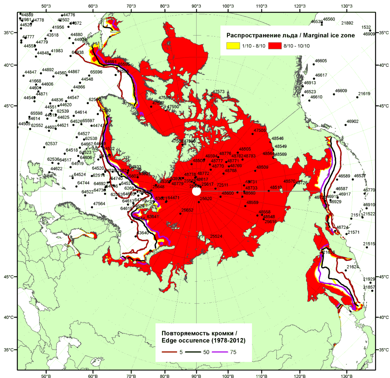
Рисунок 16 – Положение кромки льда и зон разреженных ( <8/10 ) и сплоченных ( \geq 8/10 ) льдов СЛЮ за 26.01.2015 г. на основе ледового анализа Национального Ледового Центра США, положение метеорологический дрейфующих буев IABP и Argos на 27.01.2015T1200+00 и повторяемость кромки за 26-31.01 за период 1979-2012 гг. по наблюдениям SSMR-SSM/I-SSMIS (алгоритм NASATEAM)
