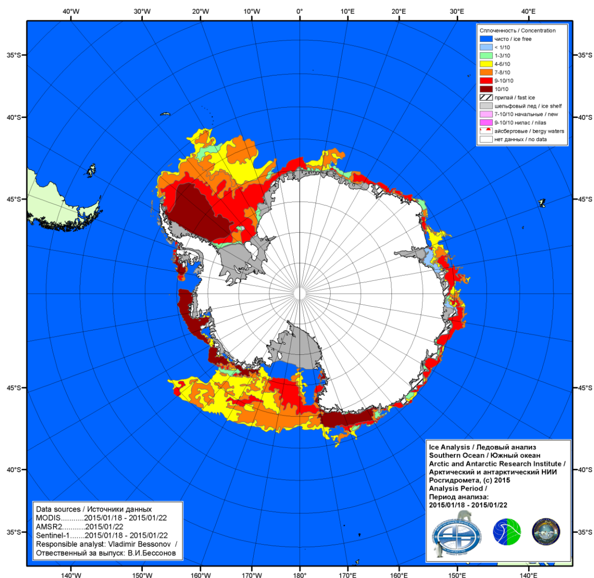
Рисунок 7а – Ледовая карта ААНИИ Южного океана за 22.01.2015.
