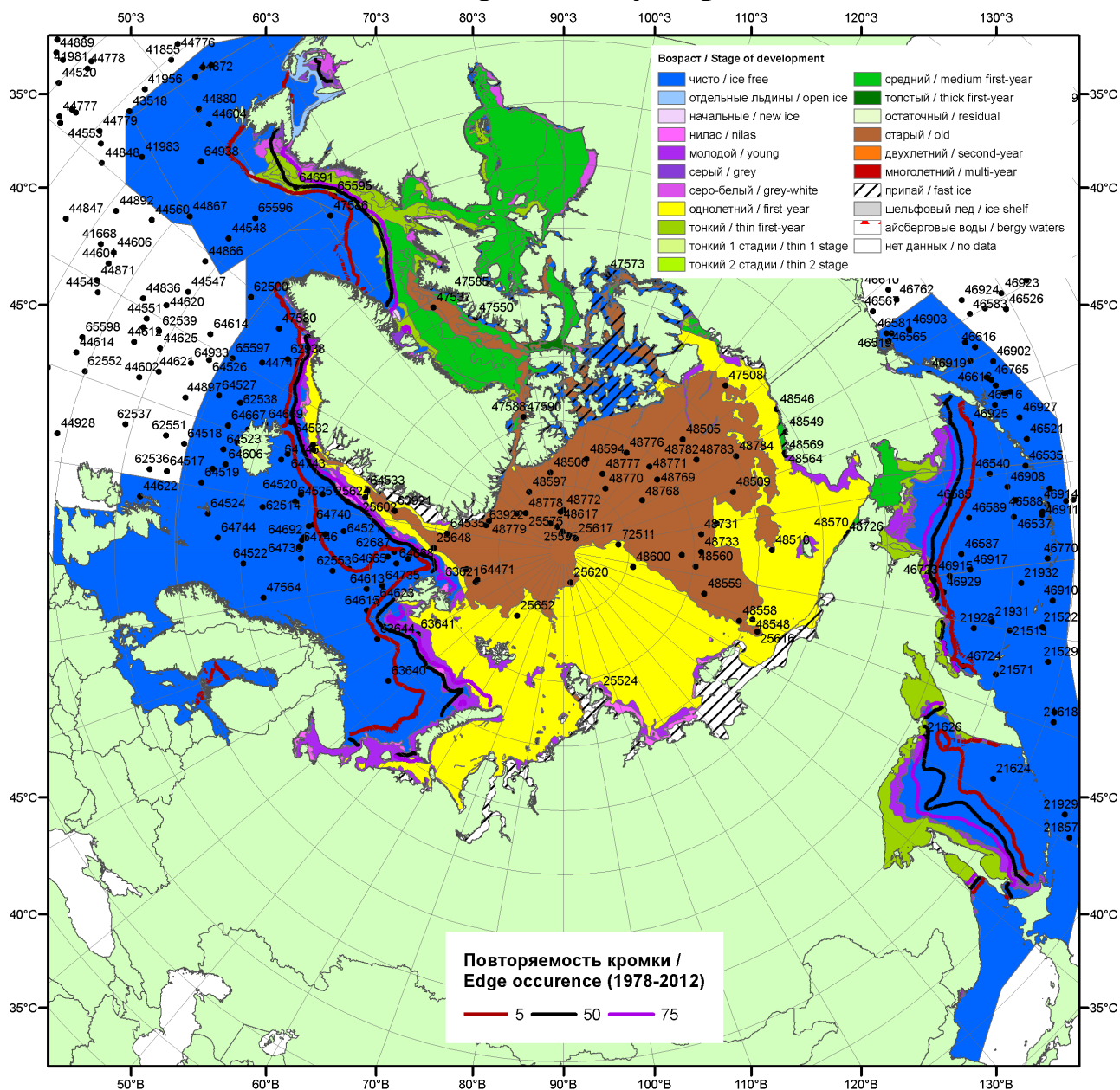
Рисунок 1а – Обзорная ледовая карта СЛО за 19.01.2015-27.01.2015 г. на основе ледового анализа ААНИИ (27.01), Национального ледового центра США (Берингово море, 22.01), Канадской ледовой службы (19.01), положение метеорологический дрейфующих буев IABP и Argos на 27.01.2015T1200+00 и повторяемость кромки за 21-25.01 за период 1978-2012 гг. по наблюдениям SSMR-SSM/I-SSMIS (алгоритм NASATEAM).
