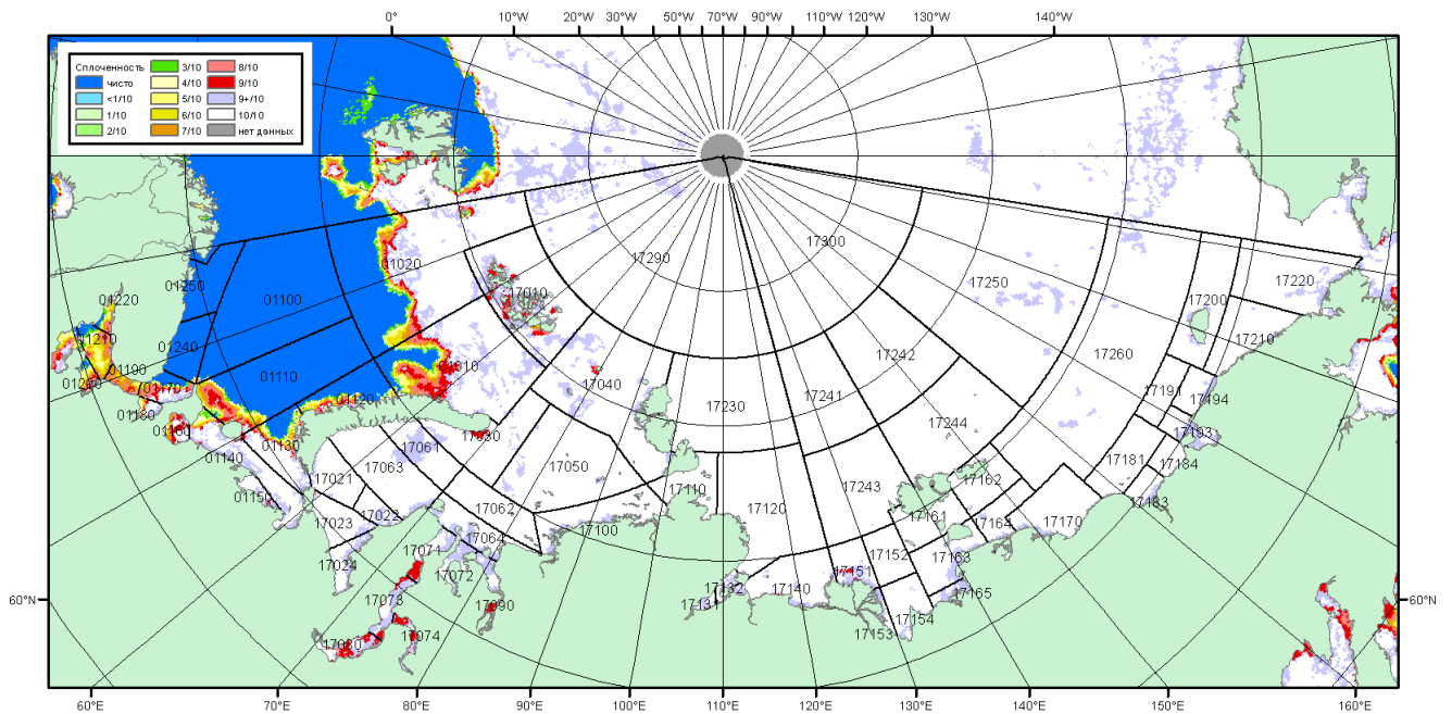
2015-01-27 00:00 UTC Распределение общей сплоченности по данным AMSR2, (с) JAXA Источник данных: Drift & Noise Polar Services Open Data Portal ( http://driftnoise.com )
