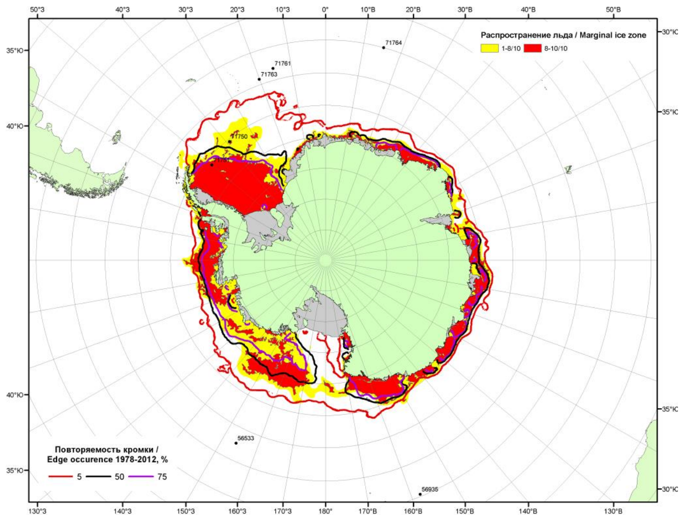
Рисунок 6в – Положение кромки льда и зон разреженных ( <8/10 ) и сплошных ( \geq 8/10 ) льдов Южного океана за 16.01.2017 г. на основе ледового анализа Национального Ледового Центра США, положение метеорологический дрейфующих буев IABP и Argos на 17.01.2017T1200+00 и повторяемость кромки за 16-20.01 за период 1979-2014 гг. по наблюдениям SSMR-SSM/I-SSMIS (алгоритм NASATEAM)
