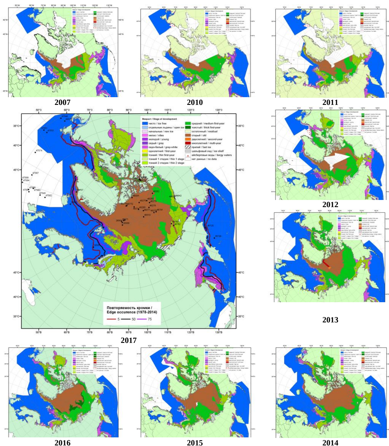
Рисунок 2 – Обзорная ледовая карта СЛО за 09 - 17.01.2017 г. и аналогичные периоды 2007-2016 гг. на основе ледового анализа ААНИИ, Канадской ледовой службы и Национального ледового центра США.
