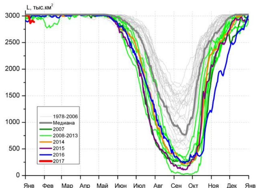
Рисунок 4 – Ежедневные оценки сезонного хода ледовитости для Северной Полярной Области и трех меридиональных секторов за период 26.10.1978 - 15.01.2017 по годам на основе расчетов по данным SSMR-SSM/I-SSMIS, алгоритмы NASATEAM: а) Северная полярная область, б) сектор 45°W-95°E (Гренландское – Карское моря), в) сектор 95°E-170°W (моря Лаптевых – Чукотское и Берингово, Охотское), г) сектор 170°W-45°W (море Бофорта и Канадская Арктика), д) Северный Ледовитый океан, е) Северный морской путь (Карское - Чукотское моря).
