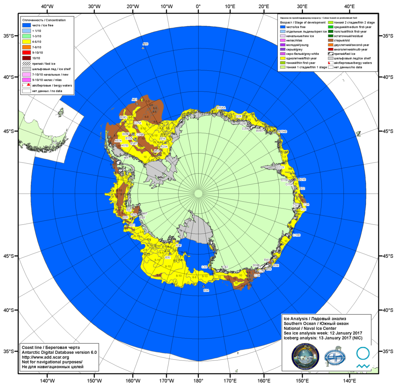
Рисунок 6б – Ледовая карта Южного океана (цветовая окраска по возрасту) и расположение крупных айсбергов на основе информации совместного ледового анализа НЛЦ США, ААНИИ и НМИ (Норвегия) за 12.01.2017.
