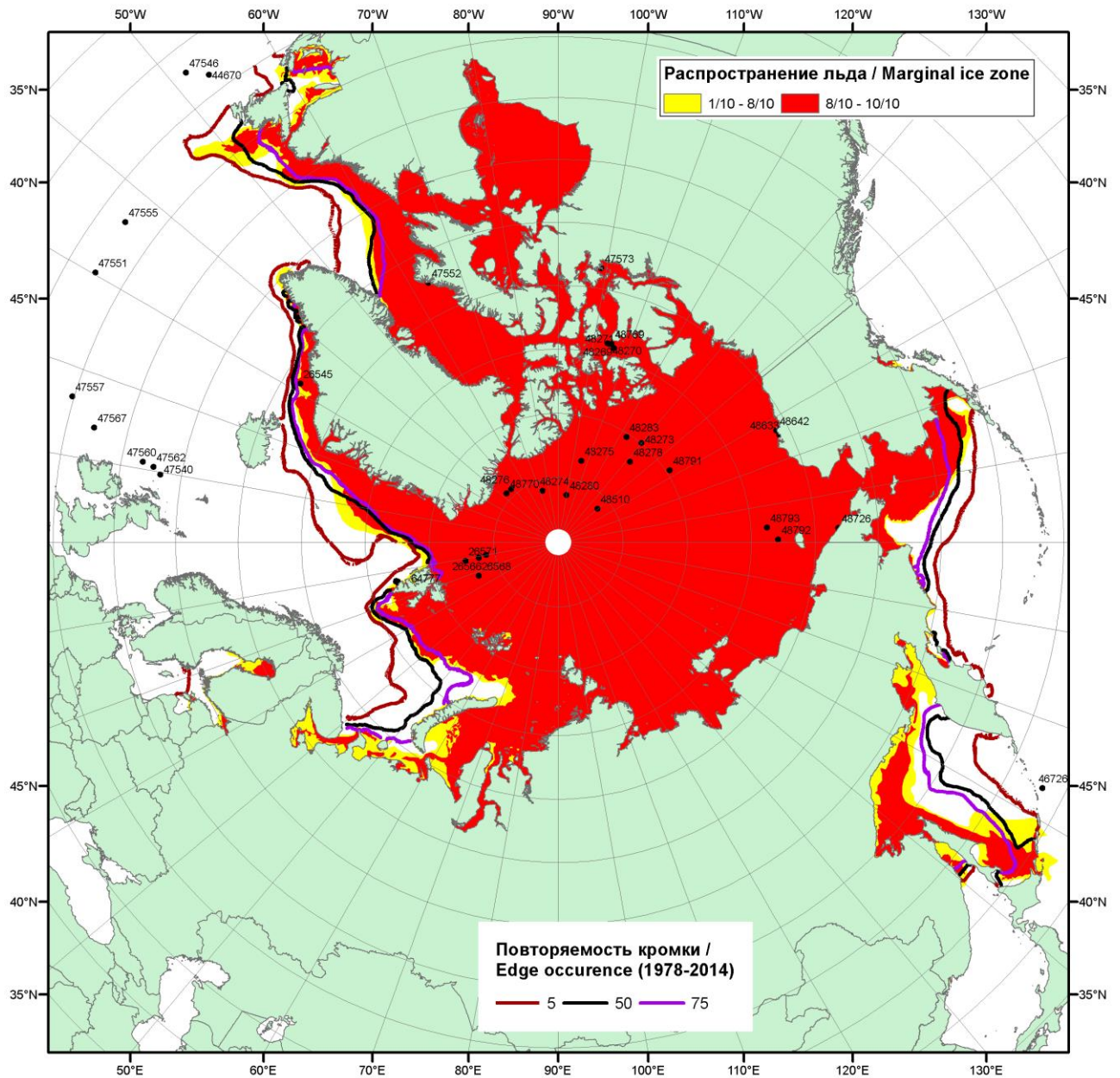
Рисунок 16 – Положение кромки льда и зон разреженных (<8/10) и сплошных (≥8/10) льдов СЛО за 20.03.2017 г. на основе ледового анализа Национального Ледового Центра США, положение метеорологический дрейфующих буев IABP и Argos на 21.03.2017T1200+00 и повторяемость кромки за 16-20.03 за период 1979-2012 гг. по наблюдениям SSMR-SSM/I-SSMIS (алгоритм NASATEAM)
