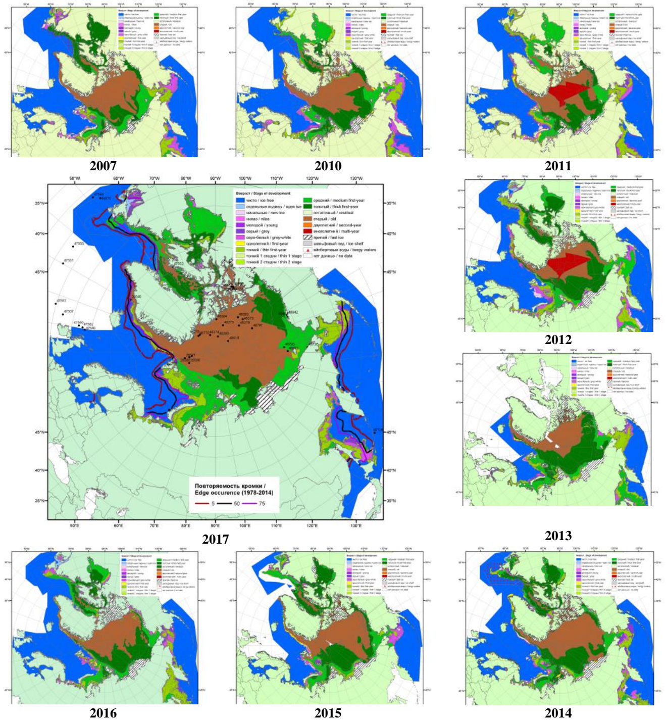
Рисунок 2 – Обзорная ледовая карта СЛО за 13.03 - 16.03.2017 г. и аналогичные периоды 2007-2016 гг. на основе ледового анализа ААНИИ, Канадской ледовой службы и Национального ледового центра США.
