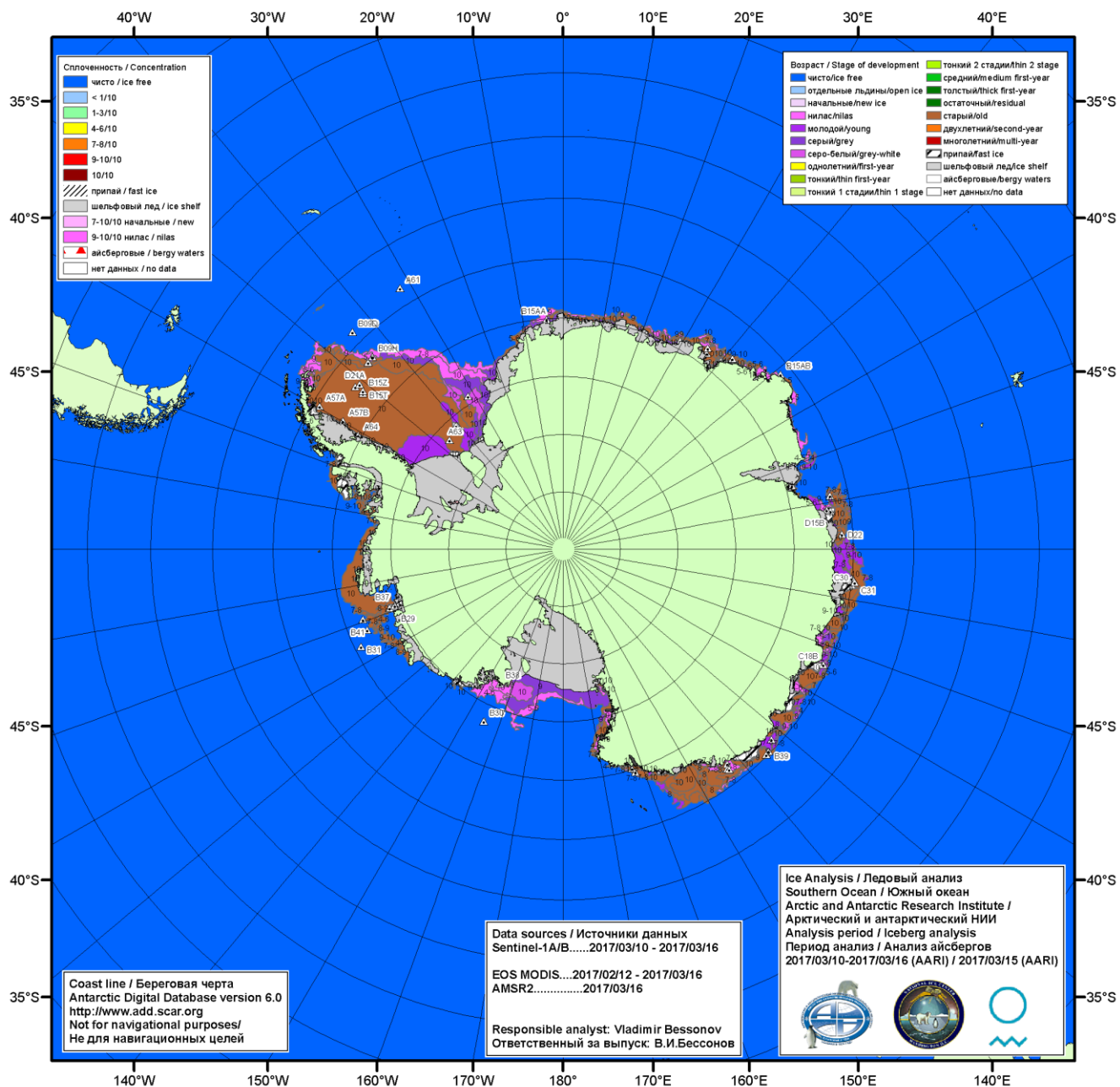
Рисунок бб – Ледовая карта Южного океана (цветовая окраска по возрасту) и расположение крупных айсбергов на основе информации совместного ледового анализа НЛЦ США, ААНИИ и НМИ (Норвегия) за 16.03.2017.
