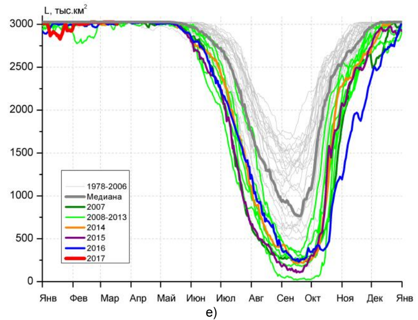
Рисунок 4 – Ежедневные оценки сезонного хода ледовитости для Северной Полярной Области и трех меридиональных секторов за период 26.10.1978 - 18.03.2017 по годам на основе расчетов по данным SSMR-SSM/I-SSMIS, алгоритмы NASATEAM: а) Северная полярная область, б) сектор 45°W-95°E (Гренландское – Карское моря), в) сектор 95°E-170°W (моря Лаптевых – Чукотское и Берингово, Охотское), г) сектор 170°W-45°W (море Бофорта и Канадская Арктика), д) Северный Ледовитый океан, е) Северный морской путь (Карское - Чукотское моря).
