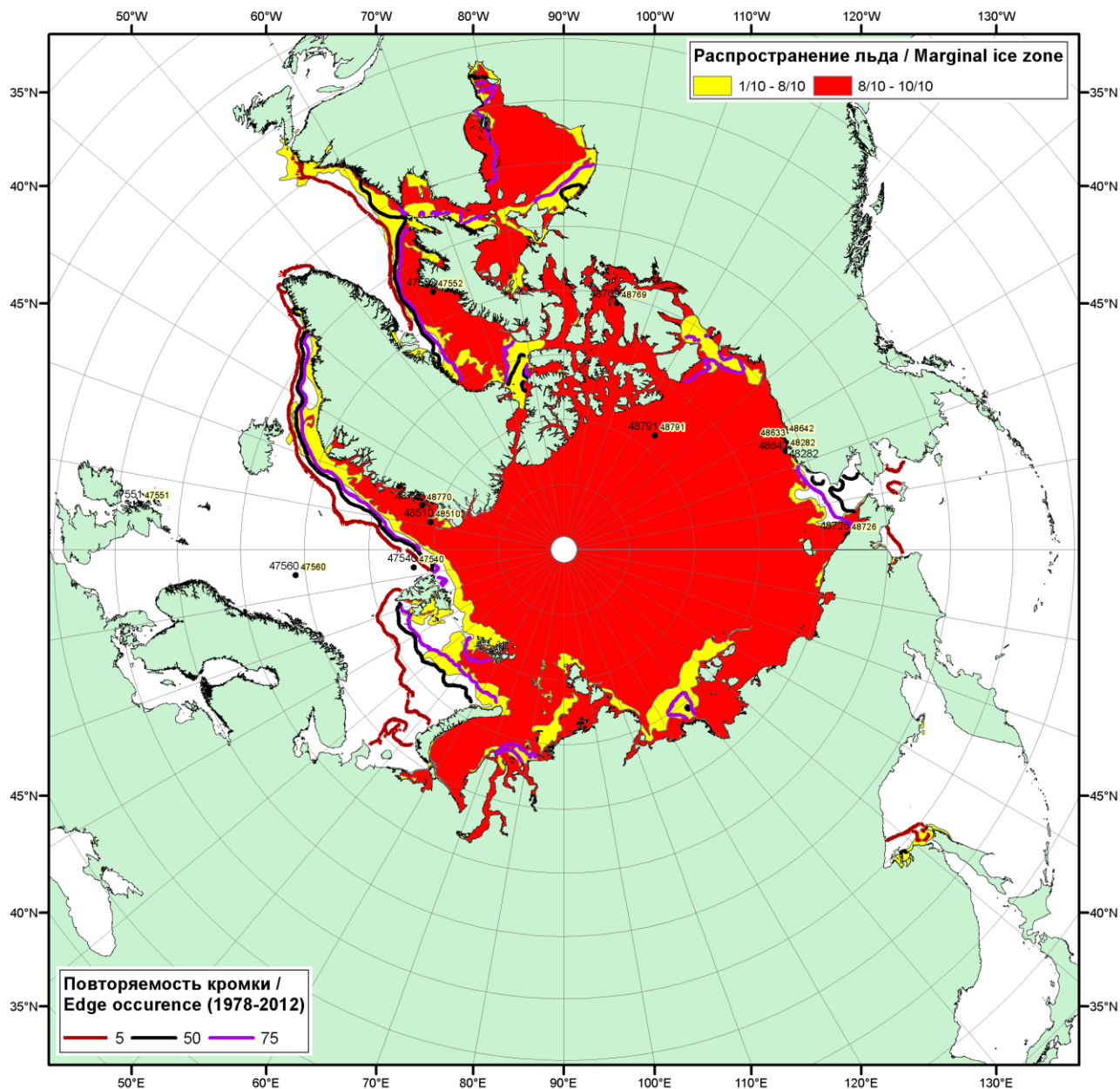
Рисунок 1в – Положение кромки льда и зон разреженных (<8/10) и сплошных ( \geq 8/10 ) льдов СЛО за 12.06.2018 г. на основе ледового анализа Национального Ледового Центра США и повторяемость кромки за 11-15.06 за период 1979-2012 гг. по наблюдениям SSMR-SSM/I-SSMIS (алгоритм NASATEAM)
