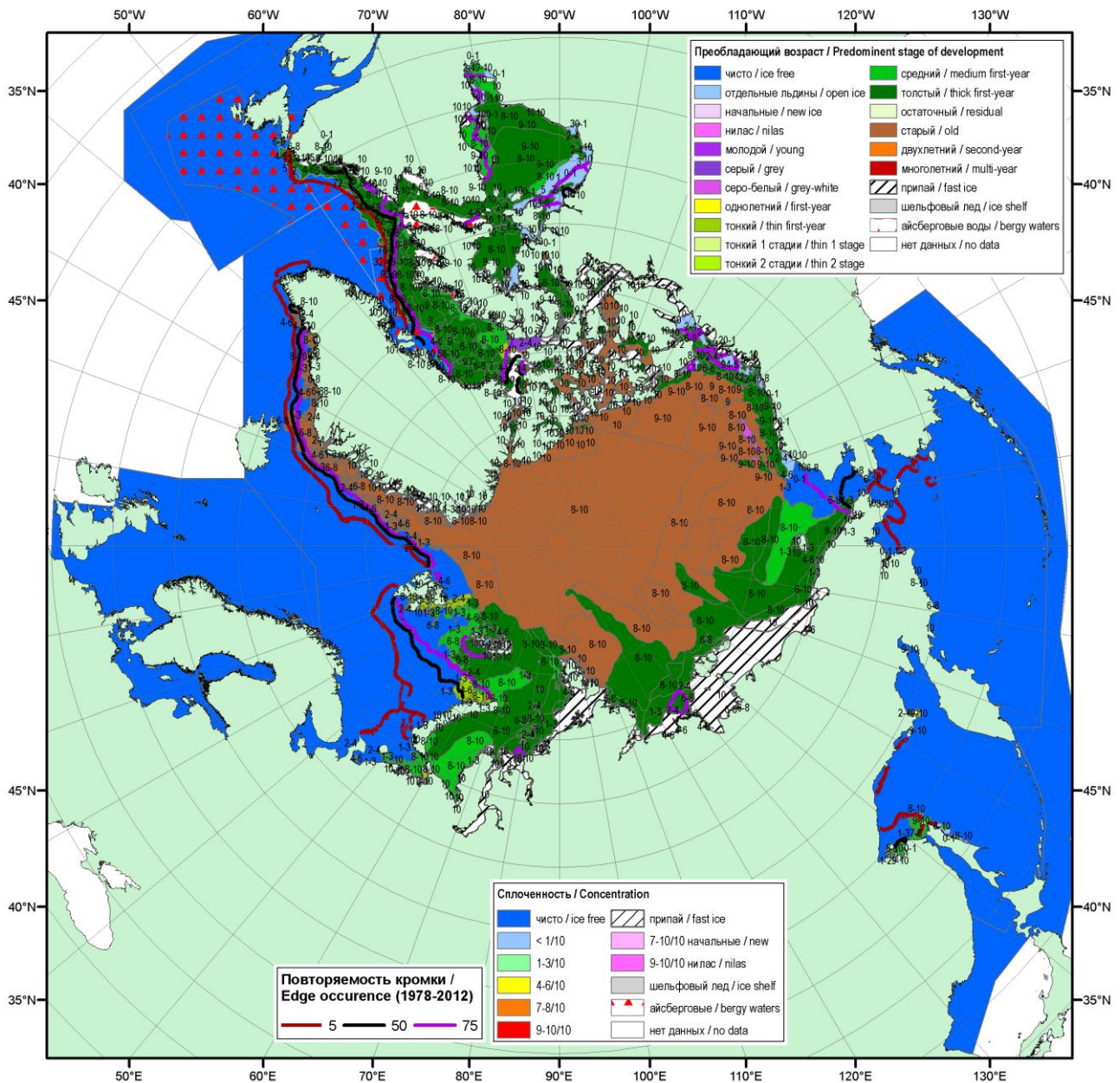
Рисунок 1а – Обзорная ледовая карта СЛО за 04.06.2018-07.06.2018 г. (цветовая раскраска по преобладающему возрасту) на основе ледового анализа НИЦ Планета (Берингово, Охотское моря, 04.06), Канадской ледовой службы (04.06), Национального ледового центра США (07.06), и повторяемость кромки за 06-10.06 за период 1979-2012 гг. по наблюдениям SSMR-SSM/I-SSMIS (алгоритм NASATEAM).
