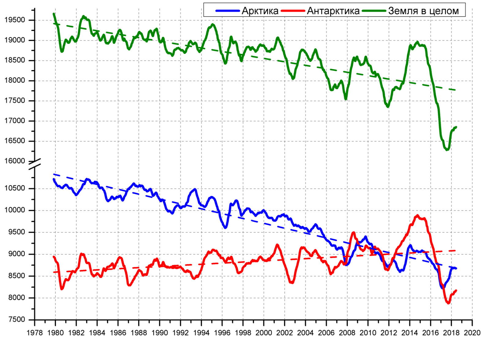
Рисунок 10 – Ежедневные сглаженные окном 365 суток значения приведенной ледовитости (площади морского льда) Арктики, Антарктики и Земли в целом с 26.10.1978 по 10.06.2018 на основе SSMR-SSM/I-SSMIS
