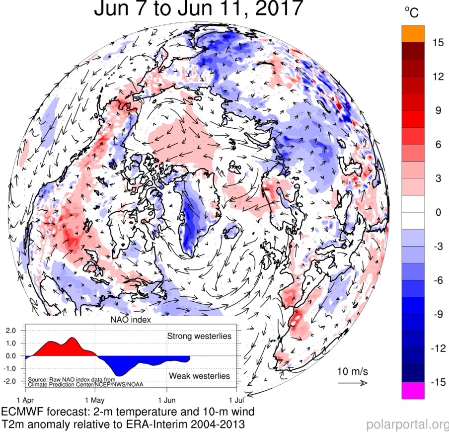
Рисунок 2е – Аномалии приземной температуры воздуха (2м) и осредненные вектора скорости ветра (10 м) за 07.06-11.06 2017-2018 гг. относительно периода 2004-2013 гг. ( http://polarportal.dk )
