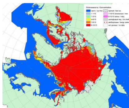
Рисунок 2а – Обзорная ледовая карта СЛО за 04.06 - 07.06.2018 г. и аналогичные периоды 2007-2017 гг. на основе ледового анализа ААНИИ, НИЦ Планета, Канадской ледовой службы и Национального ледового центра США.
