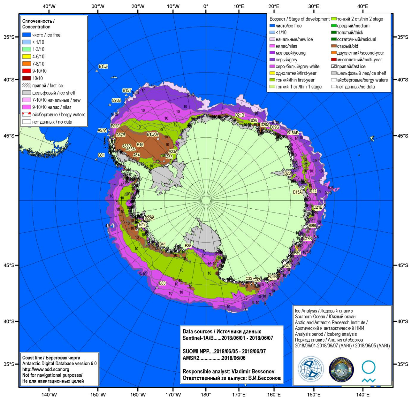
Рисунок 5б – Ледовая карта Южного океана (цветовая окраска по возрасту) и расположение крупных айсбергов на основе информации совместного ледового анализа НЛЦ США, ААНИИ и НМИ (Норвегия) за 07.06.2018.
