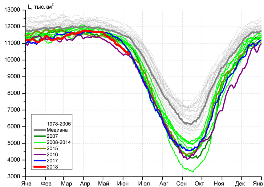
Рисунок 3 – Ежедневные оценки сезонного хода ледовитости для Северной Полярной Области и трех меридиональных секторов за период 26.10.1978 - 10.06.2018 по годам на основе расчетов по данным SSMR-SSM/I-SSMIS, алгоритмы NASATEAM: а) Северная полярная область, б) сектор 45°W-95°E (Гренландское – Карское моря), в) сектор 95°E-170°W (моря Лаптевых – Чукотское и Берингово, Охотское), г) сектор 170°W-45°W (море Бофорта и Канадская Арктика), д) Северный Ледовитый океан, е) Северный морской путь (Карское - Чукотское моря).
