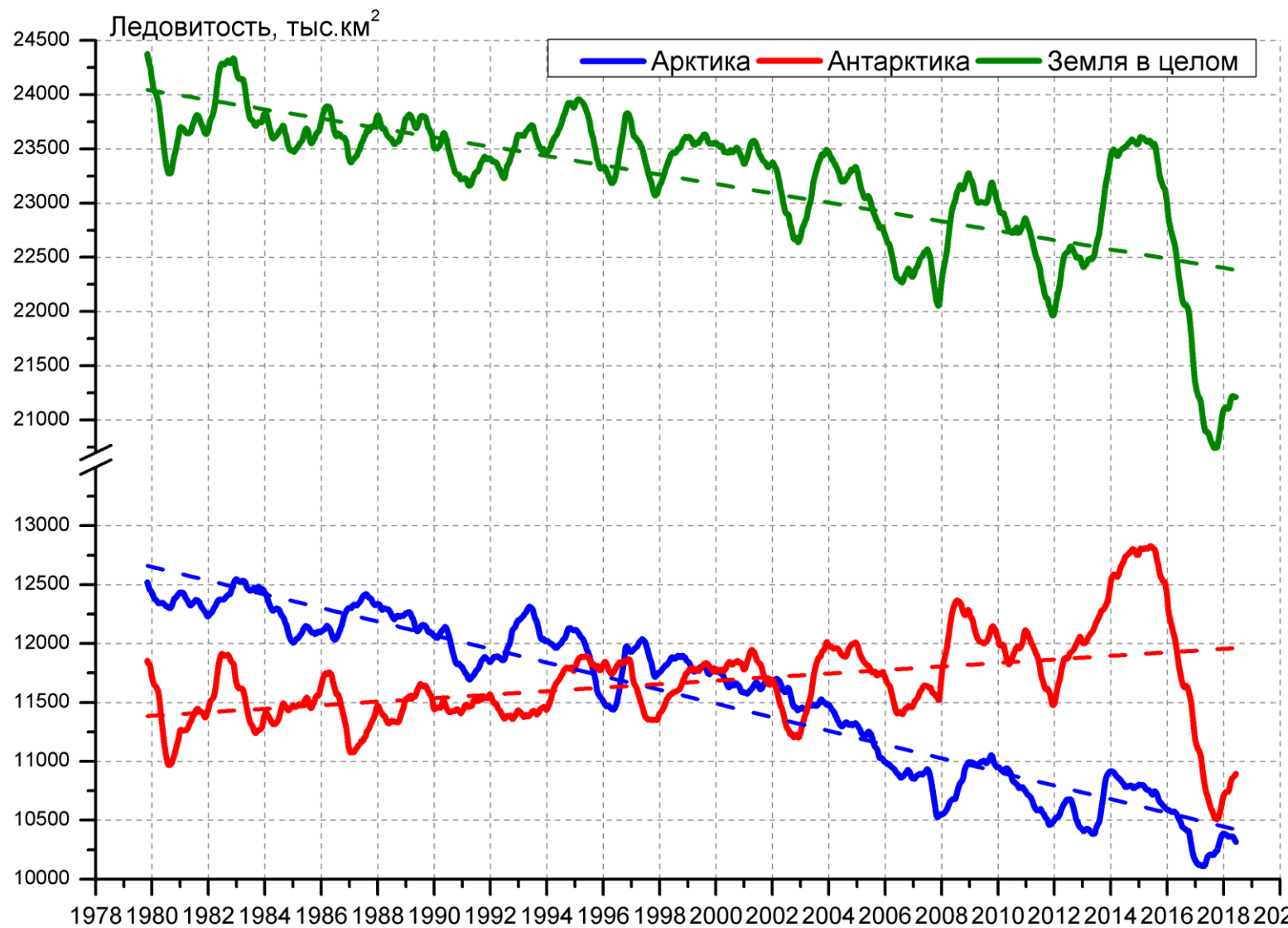
Рисунок 9 – Ежедневные сглаженные окном 365 суток значения ледовитости Арктики, Антарктики и Земли в целом с 26.10.1978 по 10.06.2018 на основе SSMR-SSM/I-SSMIS
