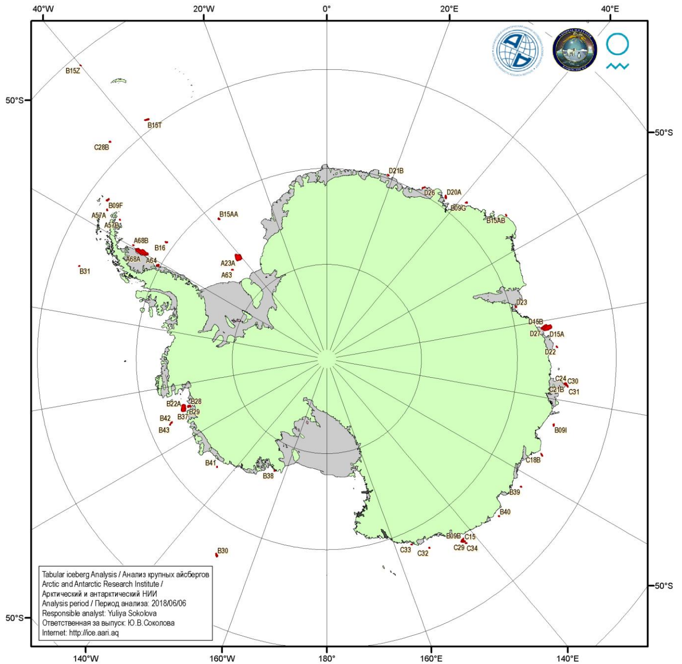
Рисунок 5д – Анализ ААНИИ крупных айсбергов Южного океана за 06.06.2018.
