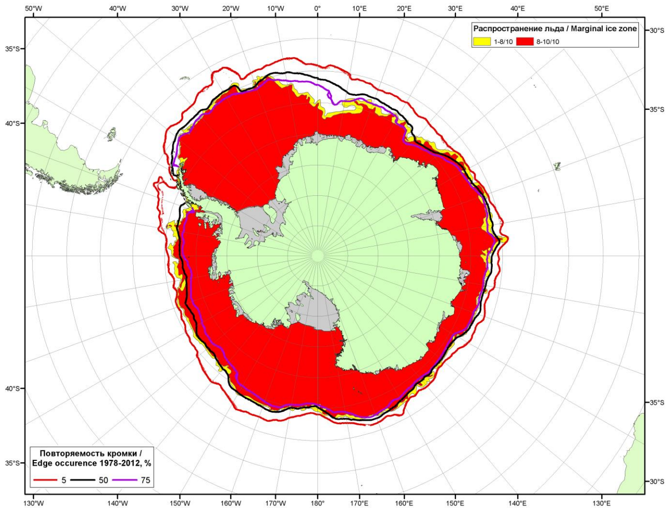
Рисунок 5в – Положение кромки льда и зон разреженных ( <8/10 ) и сплоченных ( \geq 8/10 ) льдов Южного океана за 12.06.2018 г. на основе ледового анализа Национального Ледового Центра США и повторяемость кромки за 11-15.06 за период 1979-2012 гг. по наблюдениям SSMR-SSM/I-SSMIS (алгоритм NASATEAM).
