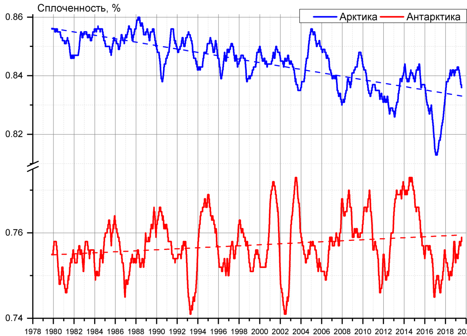
Рисунок 10 – Ежедневные сглаженные окном 365 суток значения средней общей сплоченности Арктики и Антарктики с 26.10.1978 по 28.07.2019 на основе SSMR-SSM/I-SSMIS
