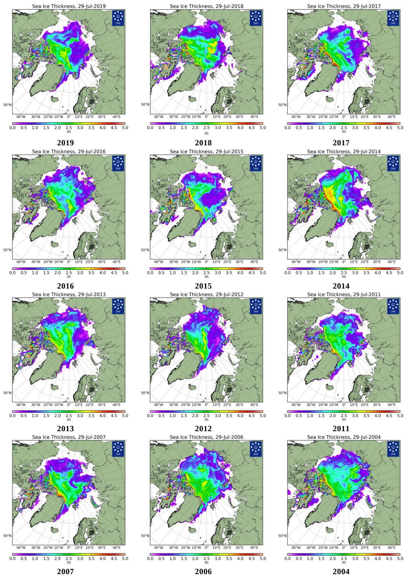
Рисунок 26 – Поля распределения средневзвешенной толщины льда совместной модели морского льда – океана НУСOM/CICE Датского метеорологического института 29.07 2004...2019 гг.
