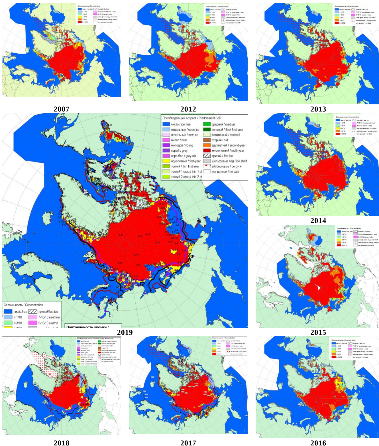
Рисунок 2а – Обзорная ледовая карта СЛО за 25.07 - 30.07.2019 г. и аналогичные периоды 2007-2018 гг. на основе ледового анализа ААНИИ, НИЦ Планета, Канадской ледовой службы и Национального ледового центра США.
