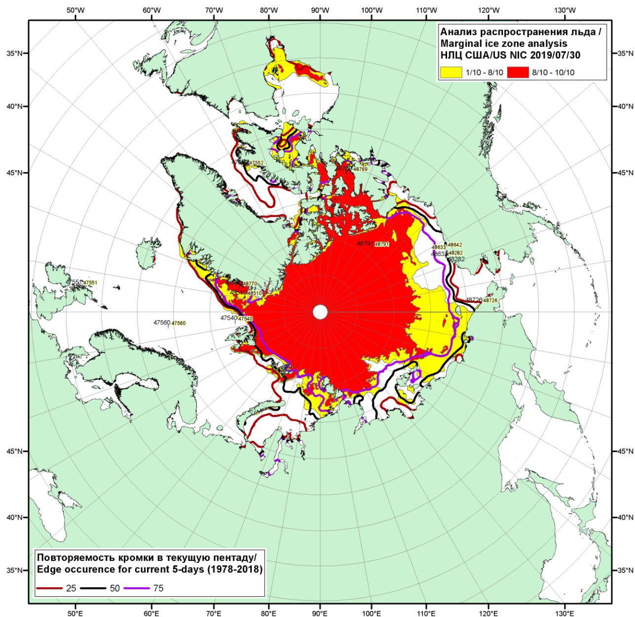
Рисунок 1в – Положение кромки льда и зон разреженных ( <8/10 ) и сплошных ( \geq 8/10 ) льдов СЛО за 30.07.2019 г. на основе ледового анализа Национального Ледового Центра США и повторяемость кромки за 26-31.07 за период 1979-2018 гг. по наблюдениям SSMR-SSM/I-SSMIS (алгоритм NASATEAM)
