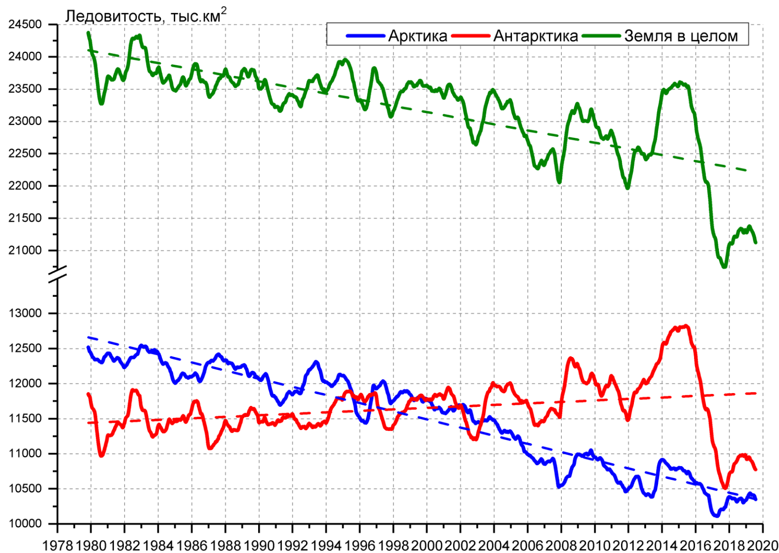
Рисунок 9 – Ежедневные сглаженные окном 365 суток значения приведенной ледовитости (площади морского льда) Арктики, Антарктики и Земли в целом с 26.10.1978 по 28.07.2019 на основе SSMR-SSM/I-SSMIS
