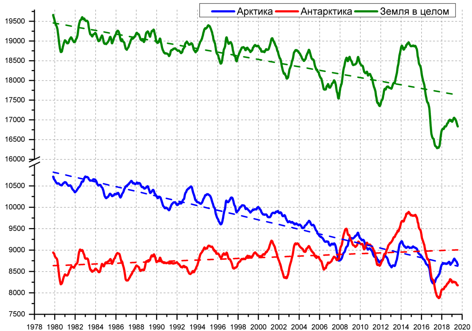
Рисунок 10 – Ежедневные сглаженные окном 365 суток значения ледовитости (площади распространения морского льда) Арктики, Антарктики и Земли в целом с 26.10.1978 по 28.07.2019 на основе SSMR-SSM/I-SSMIS
