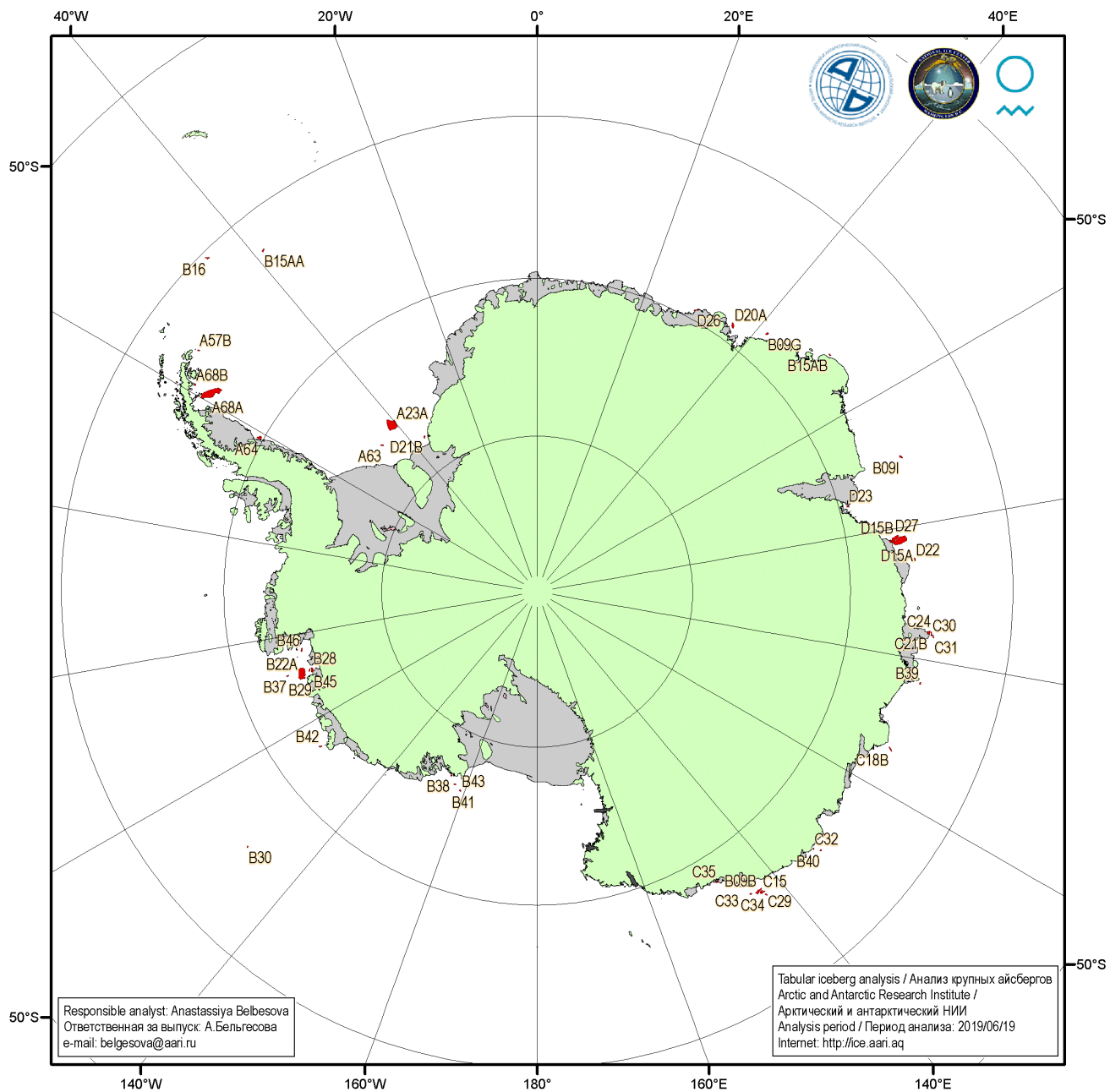
Рисунок 5д – Анализ ААНИИ крупных айсбергов Южного океана за 19.06.2019.
