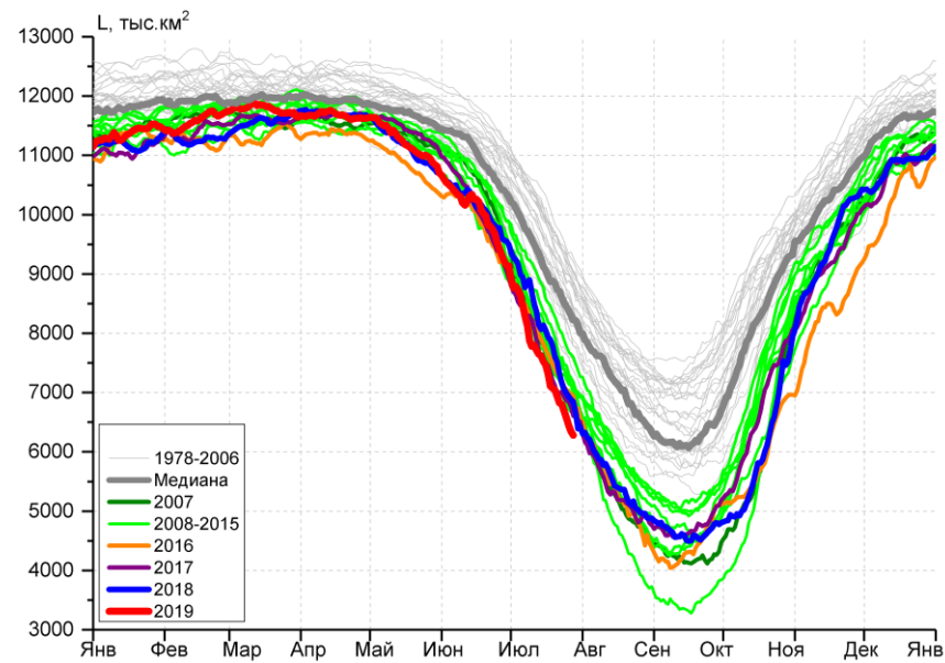
Рисунок 3а – Ежедневные оценки сезонного хода ледовитости для Северной Полярной Области и трех меридиональных секторов за период 26.10.1978 - 28.07.2019 по годам на основе расчетов по данным SSMR-SSM/I-SSMIS, алгоритмы NASATEAM: а) Северная полярная область, б) сектор 45°W-95°E (Гренландское – Карское моря), в) сектор 95°E-170°W (моря Лаптевых – Чукотское и Берингово, Охотское), г) сектор 170°W-45°W (море Бофорта и Канадская Арктика), д) Северный Ледовитый океан, е) Северный морской путь (Карское - Чукотское моря).
