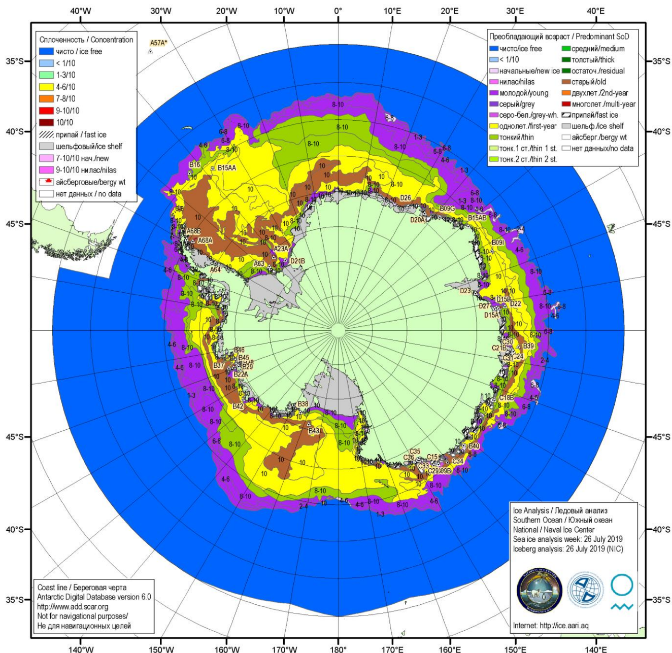
Рисунок 56 – Ледовая карта Южного океана (цветовая окраска по возрасту) и расположение крупных айсбергов на основе информации совместного ледового анализа НЛЦ США, ААНИИ и НМИ (Норвегия) за 26.07.2019.
