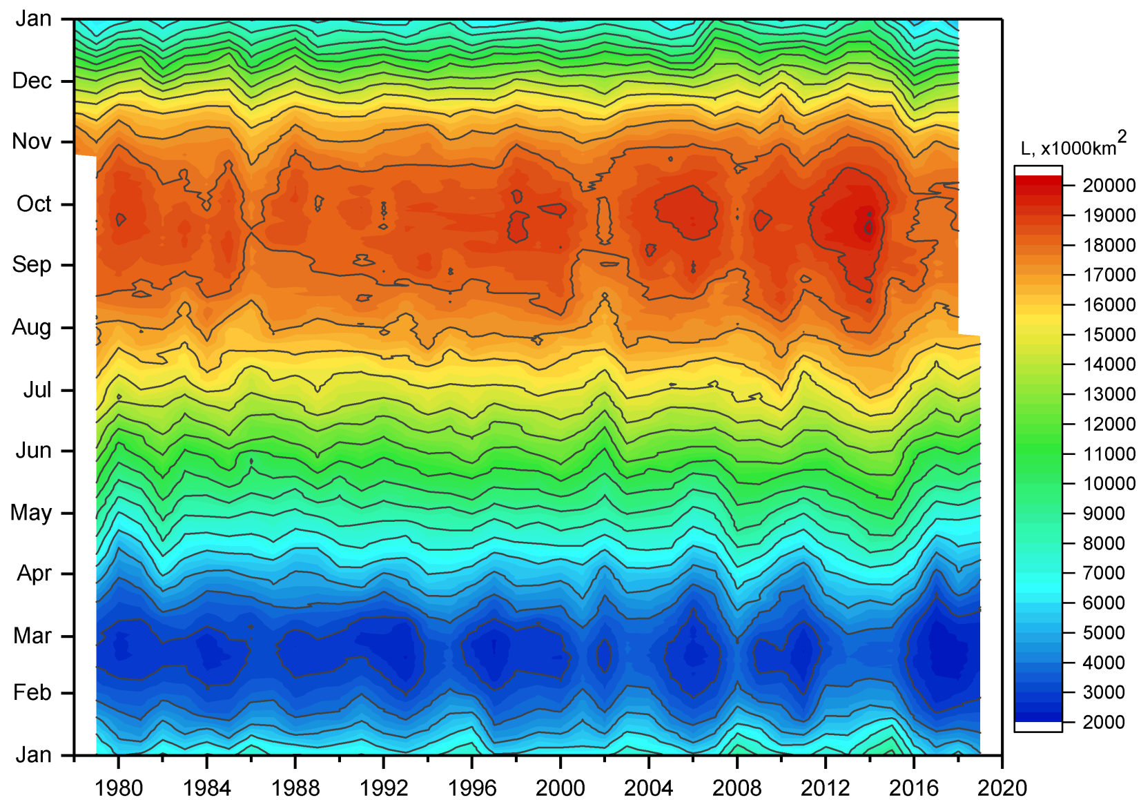
Рисунок 76 – Ежедневные оценки сезонных изменений ледовитости для Южного океана за период 26.10.1978 -28.07.2019 на основе расчетов по данным SSMR-SSM/I-SSMIS, алгоритм NASATEAM.
