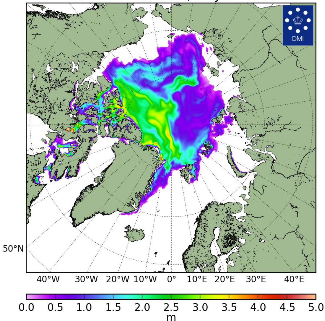
Рисунок 2д – Ежедневные оценки сезонного хода объема морского льда СЛО на основе расчетов средневзвешенной толщины льда совместной модели морского льда – океана HYCOM/CICE Датского метеорологического института с 01.01.2004 по 29.07.2019 гг.
