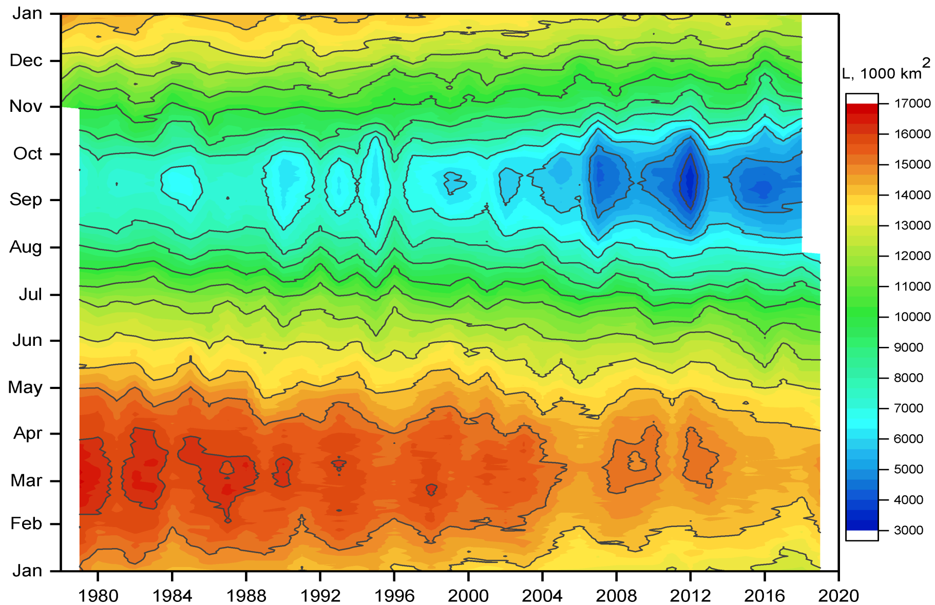
Рисунок 36 – Ежедневные оценки сезонных изменений ледовитости для Северной Полярной Области за период 26.10.1978 -28.07.2019 на основе расчетов по данным SSMR-SSM/I-SSMIS, алгоритм NASATEAM.
