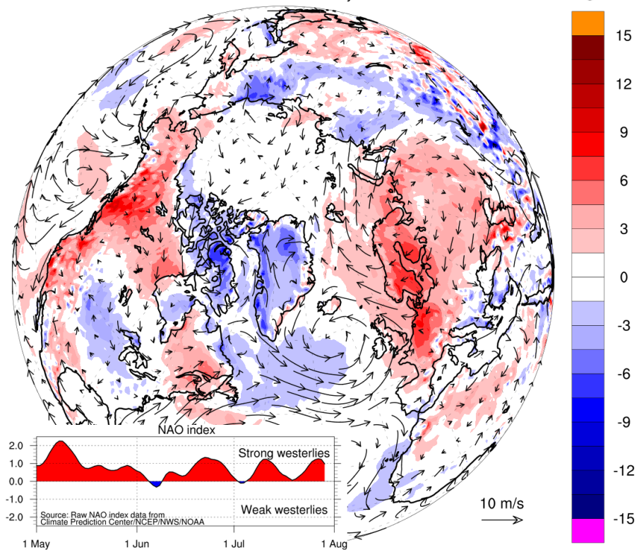
Рисунок 2е – Аномалии приземной температуры воздуха (2м) и осредненные вектора скорости ветра (10 м) за 25.07-29.07 2018-2019 гг. относительно периода 2004-2013 гг. ( http://polarportal.dk )
