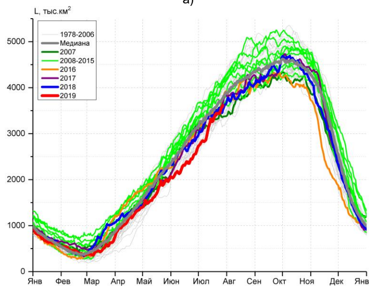
Рисунок 7а – Ежедневные оценки сезонного хода ледовитости Южного Океана и меридиональных секторов за период 26.10.1978 – 28.07.2019 по годам на основе расчетов по данным SSMR-SSM/I-SSMIS, алгоритм NASATEAM: а) Южный Океан, б) Атлантический сектор (60°W-30°E, море Уэдделла), в) Индоокеанский сектор (30°E-150°E, моря Космонавтов, Содружества, Моусона), г) Тихоокеанский сектор (150°E-60°W, моря Росса, Беллинсгаузена)
