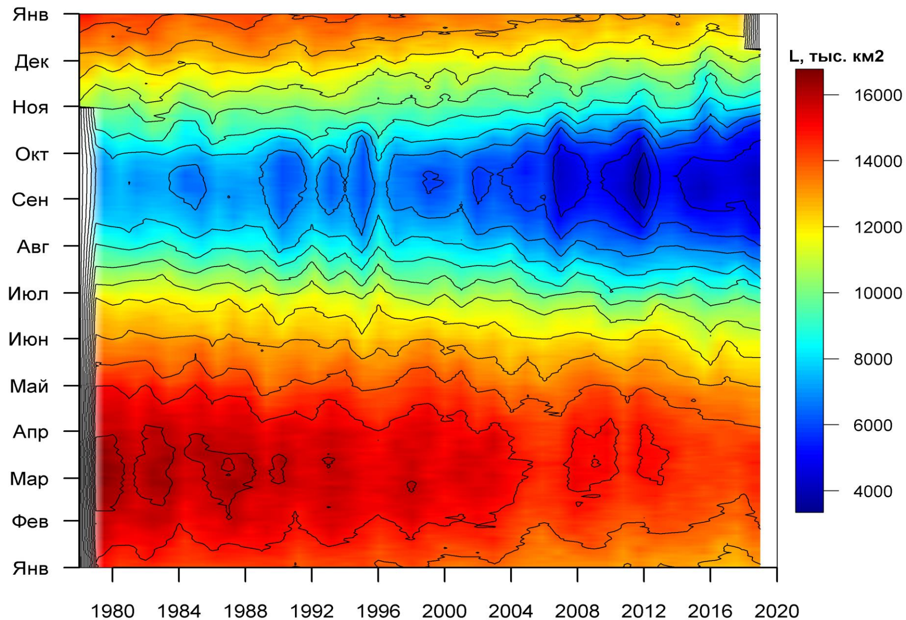
Рисунок 3б – Ежедневные оценки сезонных изменений ледовитости для Северной Полярной Области за период 26.10.1978 -08.12.2019 на основе расчетов по данным SSMR-SSM/I-SSMIS, алгоритм NASATEAM.
