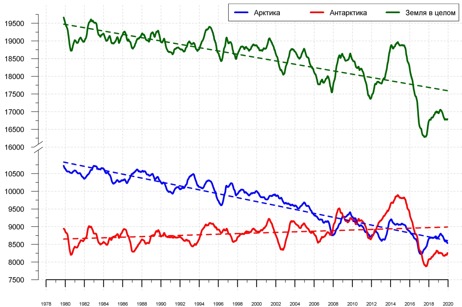
Рисунок 10 – Ежедневные сглаженные окном 365 суток значения ледовитости (площади распространения морского льда) Арктики, Антарктики и Земли в целом с 26.10.1978 по 08.12.2019 на основе SSMR-SSM/I-SSMIS
