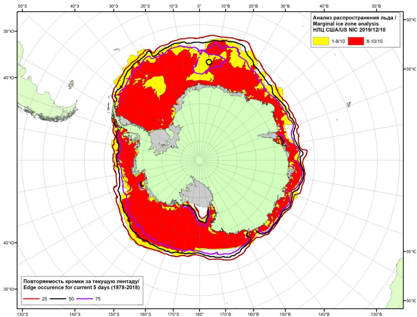
Рисунок 5в – Положение кромки льда и зон разреженных ( <8/10 ) и сплоченных ( \geq 8/10 ) льдов Южного океана за 10.12.2019 г. на основе ледового анализа Национального Ледового Центра США и повторяемость кромки за 06-10.12 за период 1979-2018 гг. по наблюдениям SSMR-SSM/I-SSMIS (алгоритм NASATEAM).
