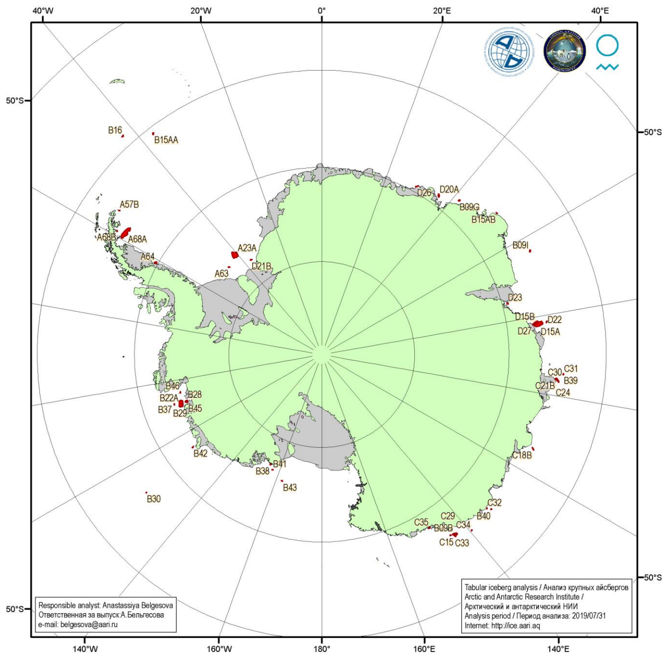
Рисунок 5д – Анализ ААНИИ крупных айсбергов Южного океана за 31.07.2019.
