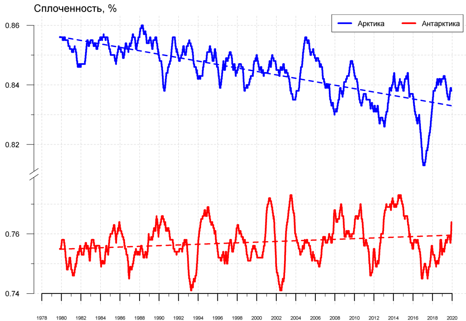
Рисунок 11 – Ежедневные сглаженные окном 365 суток значения средней общей сплоченности Арктики и Антарктики с 26.10.1978 по 08.12.2019 на основе SSMR-SSM/I-SSMIS
