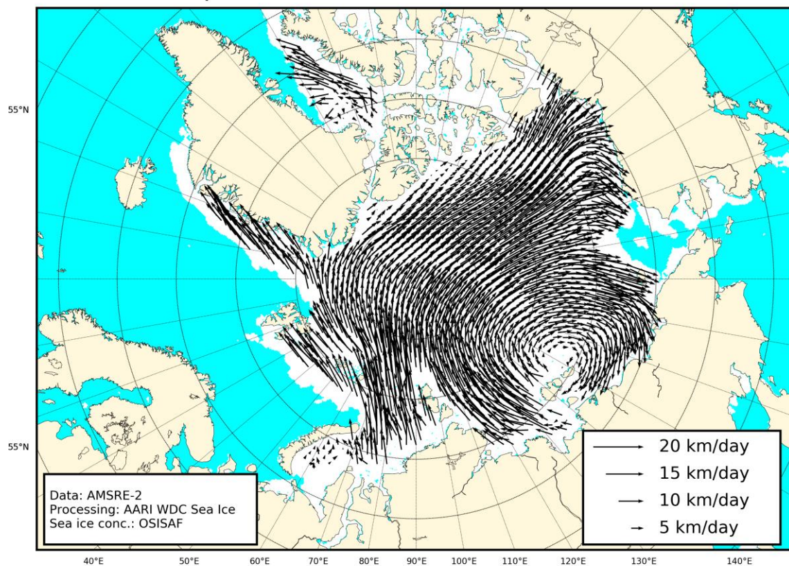
Рисунок 2г – Поле дрейфа морского льда Арктики за 02.12-09.12.2019 г. по расчетам МЦД МЛ ААНИИ, источник данных EUMETSAT OSISAF, AMSR-2.
