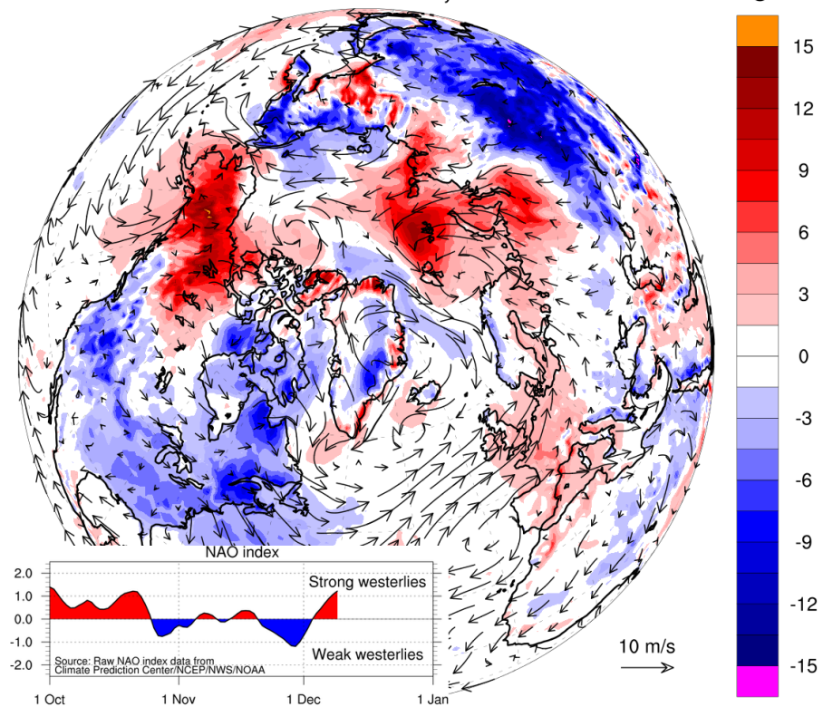
Рисунок 2е – Аномалии приземной температуры воздуха (2м) и осредненные вектора скорости ветра (10 м) за 05.12-09.12 2018-2019 гг. относительно периода 2004-2013 гг. ( http://polarportal.dk )
