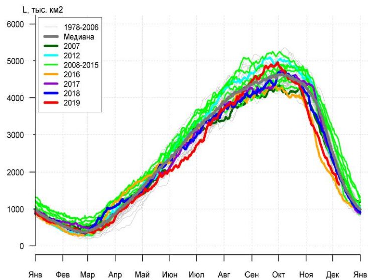
Рисунок 7а – Ежедневные оценки сезонного хода ледовитости Южного Океана и меридиональных секторов за период 26.10.1978 – 08.12.2019 по годам на основе расчетов по данным SSMR-SSM/I-SSMIS, алгоритм NASATEAM: а) Южный Океан, б) Атлантический сектор (60°W-30°E, море Уэдделла), в) Индоокеанский сектор (30°E-150°E, моря Космонавтов, Содружества, Моусона), г) Тихоокеанский сектор (150°E-60°W, моря Росса, Беллингаузена)
