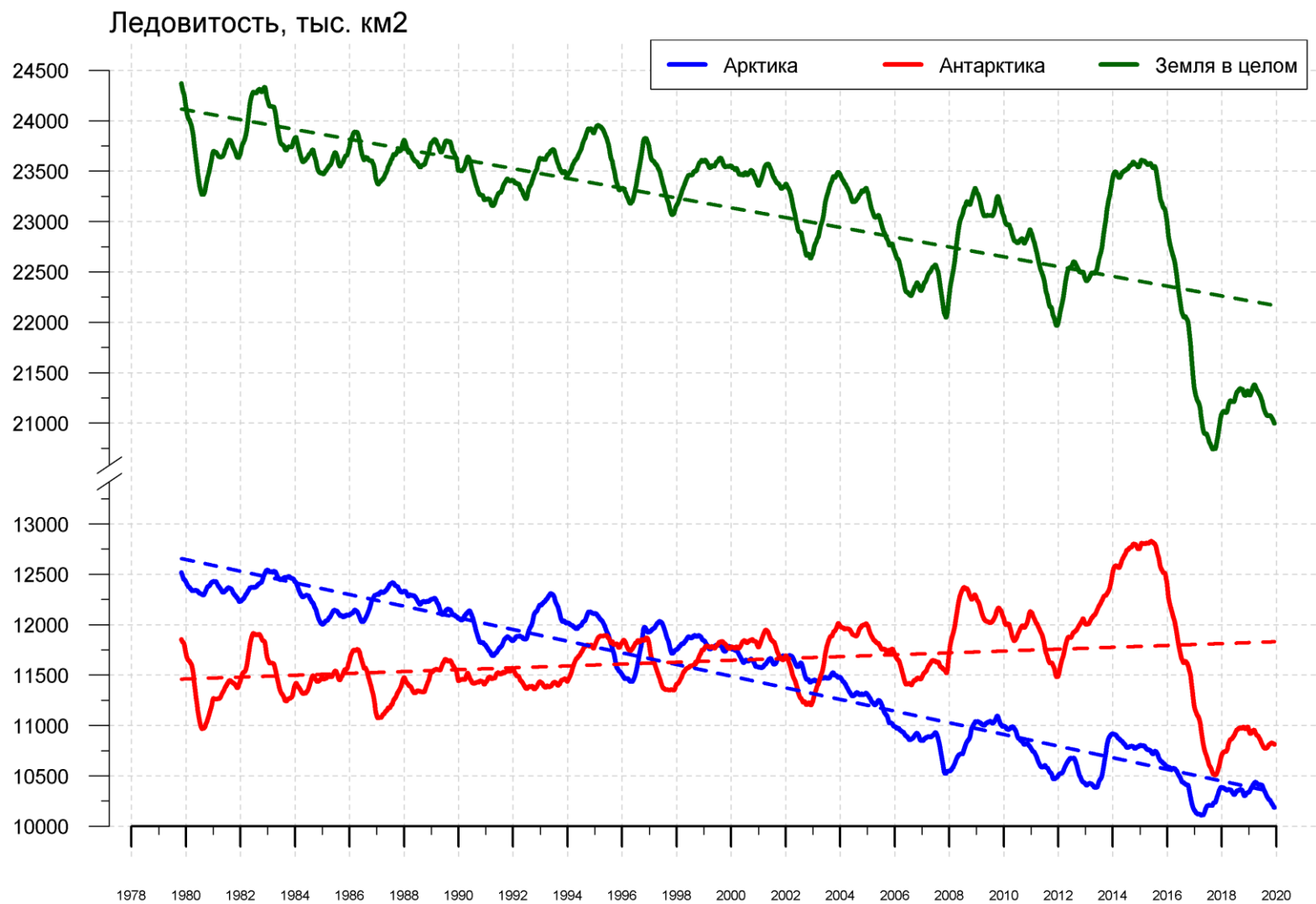
Рисунок 9 – Ежедневные сглаженные окном 365 суток значения приведенной ледовитости (площади морского льда) Арктики, Антарктики и Земли в целом с 26.10.1978 по 08.12.2019 на основе SSMR-SSM/I-SSMIS
