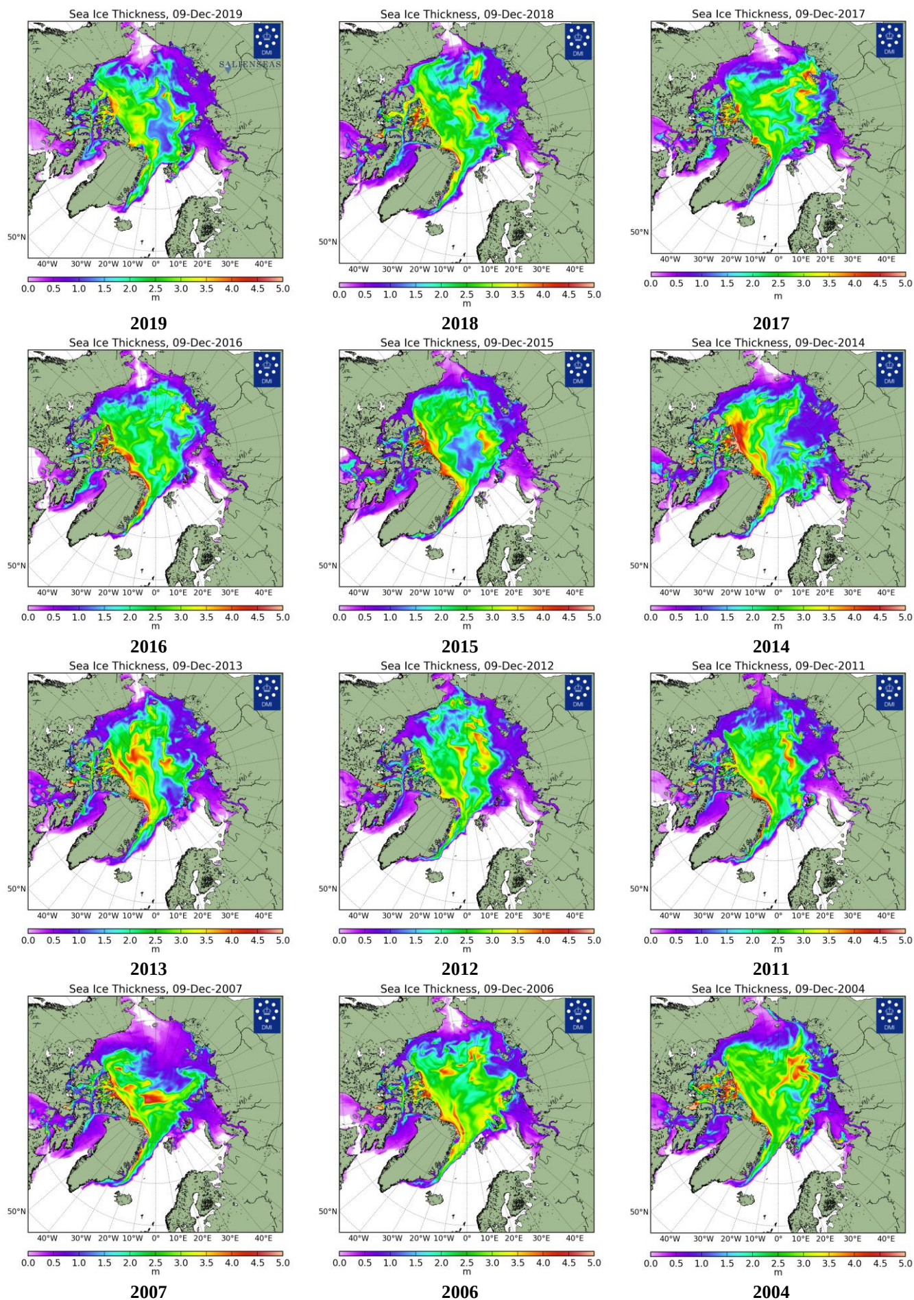
Рисунок 26 – Поля распределения средневзвешенной толщины льда совместной модели морского льда – океана NUCOM/CICE Датского метеорологического института 09.12 2004...2019 гг.
