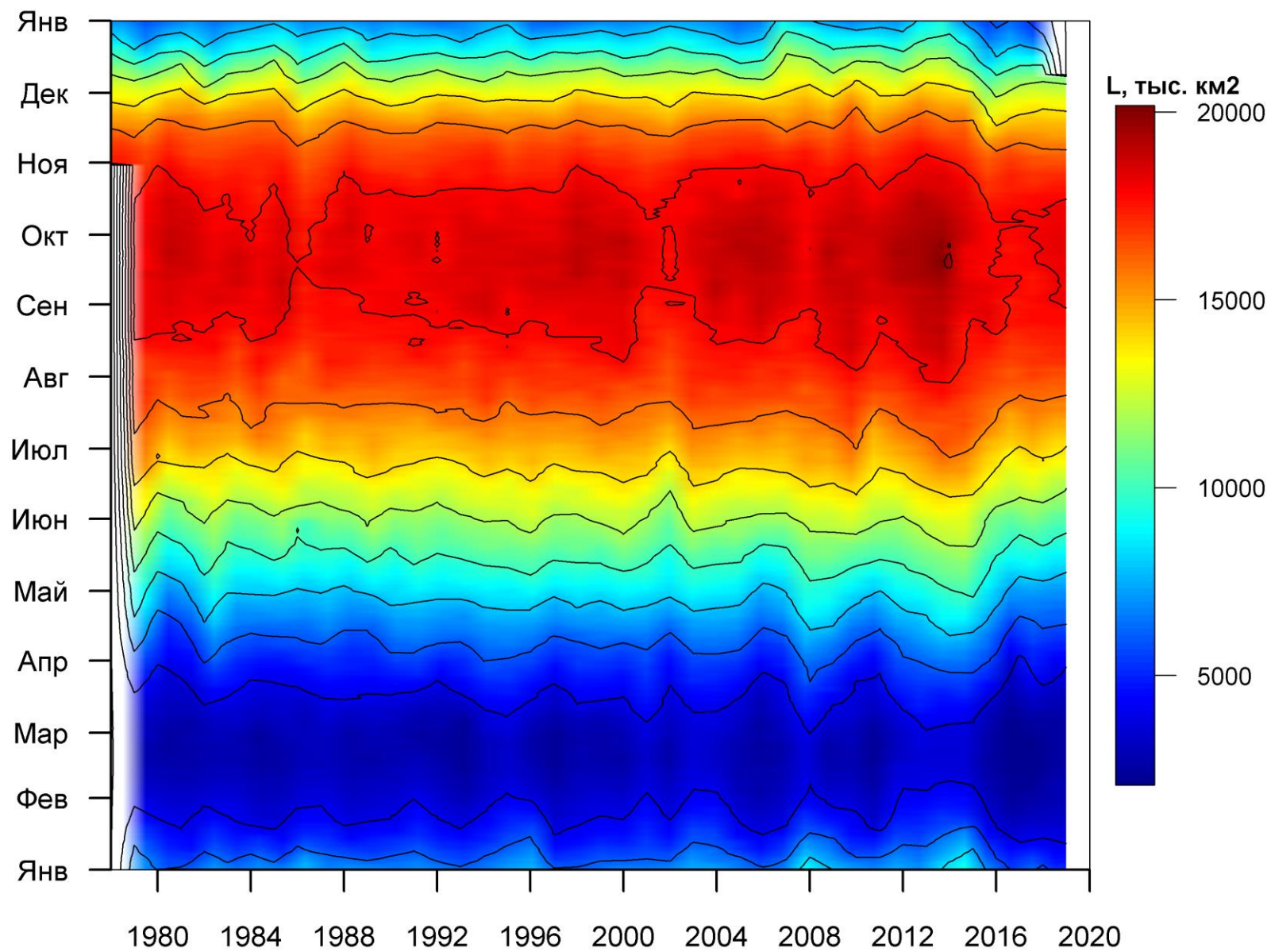
Рисунок 76 – Ежедневные оценки сезонных изменений ледовитости для Южного океана за период 26.10.1978 -08.12.2019 на основе расчетов по данным SSMR-SSM/I-SSMIS, алгоритм NASATEAM.
