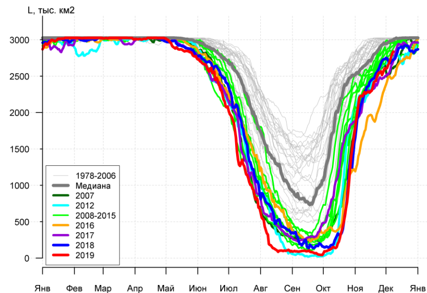
Рисунок 3а – Ежедневные оценки сезонного хода ледовитости для Северной Полярной Области и трех меридиональных секторов за период 26.10.1978 - 08.12.2019 по годам на основе расчетов по данным SSMR-SSM/I-SSMIS, алгоритмы NASATEAM: а) Северная полярная область, б) сектор 45°W-95°E (Гренландское – Карское моря), в) сектор 95°E-170°W (моря Лаптевых – Чукотское и Берингово, Охотское), г) сектор 170°W-45°W (море Бофорта и Канадская Арктика), д) Северный Ледовитый океан, е) Северный морской путь (Карское - Чукотское моря).
