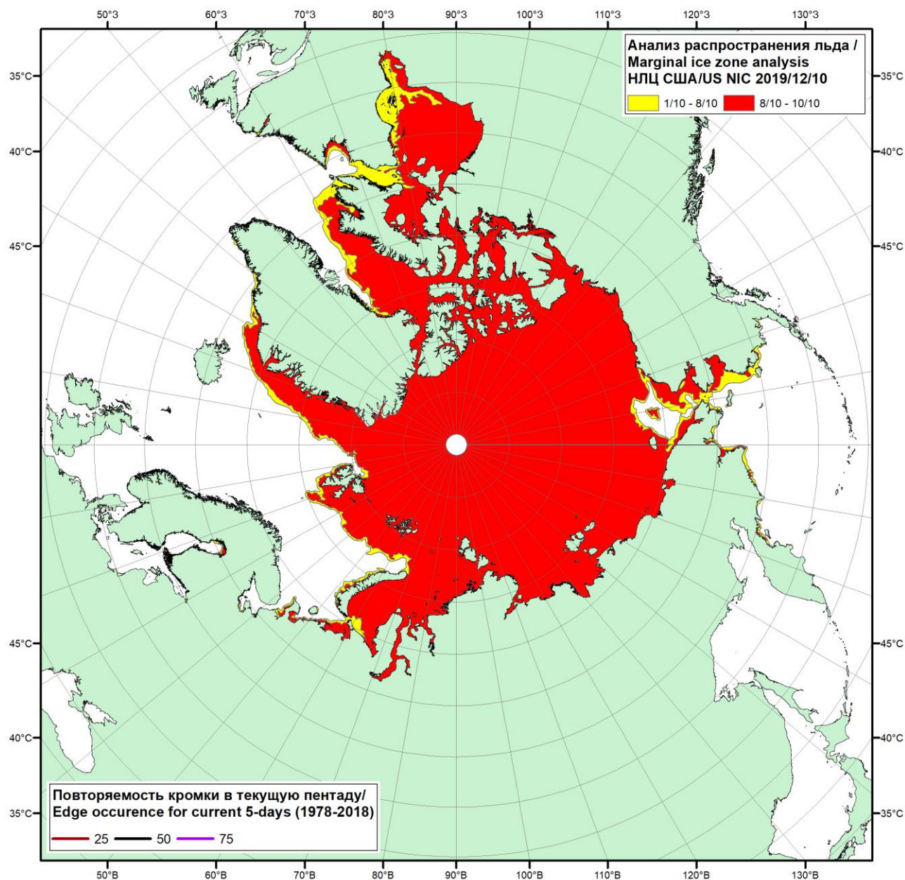
Рисунок 1в – Положение кромки льда и зон разреженных ( <8/10 ) и сплошных ( \geq 8/10 ) льдов СЛО за 10.12.2019 г. на основе ледового анализа Национального Ледового Центра США и повторяемость кромки за 06-10.12 за период 1979-2018 гг. по наблюдениям SSMR-SSM/I-SSMIS (алгоритм NASATEAM)
