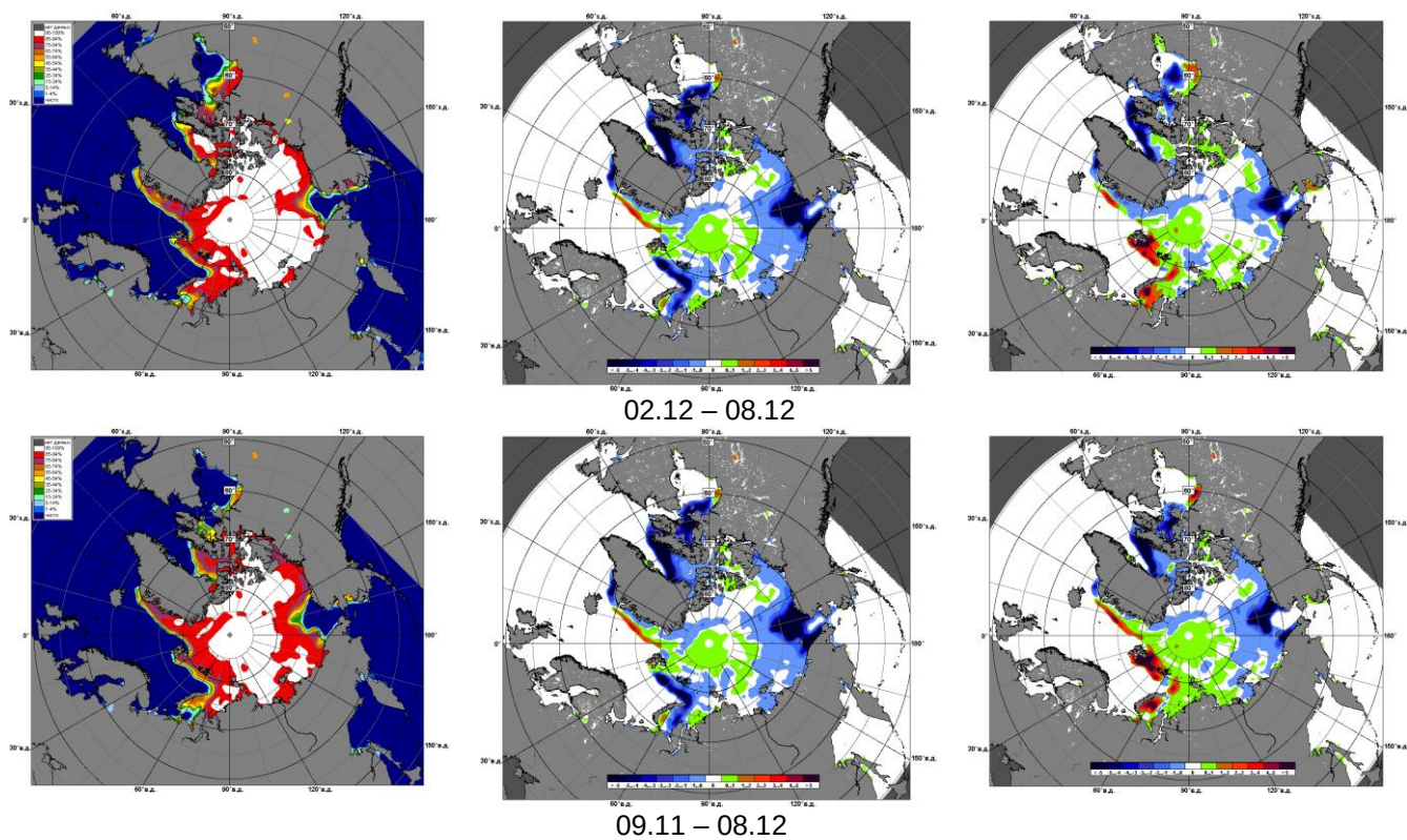
Рисунок 4 – Медианные распределения сплоченности льда за текущие 7 дневные промежутки и её разности относительно медианного распределения за те же промежутки за периоды 1979-2019 (центр) и 2009-2019 гг. (справа) на основе расчетов по данным SSMR-SSM/I-SSMIS, алгоритмы NASATEAM.
