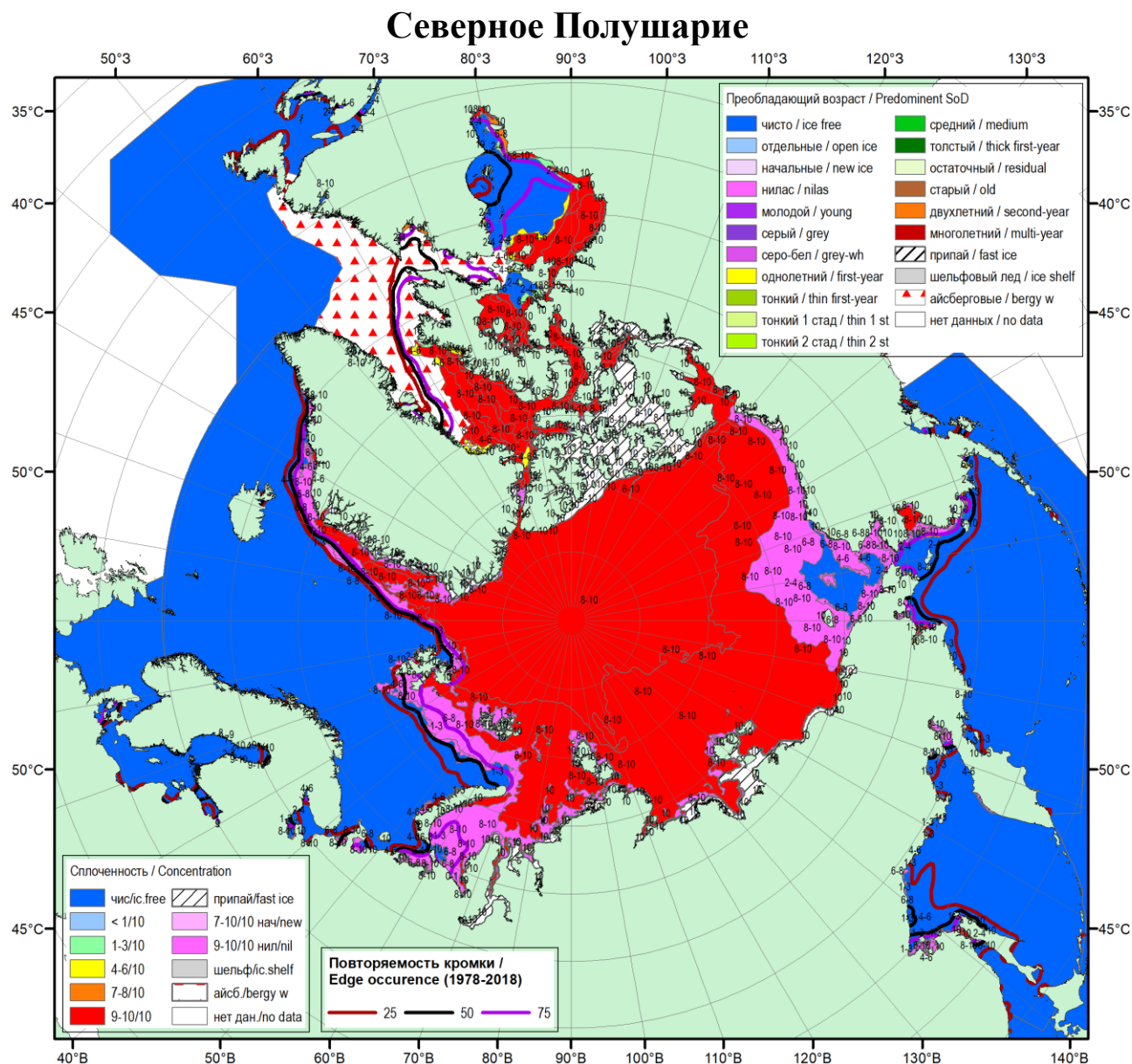
Рисунок 1а – Обзорная ледовая карта СЛЮ за 06.12.2019-10.12.2019 г. (цветовая раскраска по общей сплоченности) на основе ледового анализа ААНИИ (10.12), Национального ледового центра США (06.12) и повторяемость кромки за 06-10.12 за период 1979-2018 гг. по наблюдениям SSMR-SSM/I-SSMIS (алгоритм NASATEAM).
