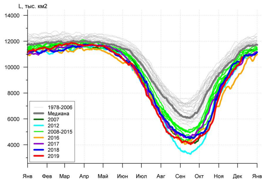
Рисунок 3а – Ежедневные оценки сезонного хода ледовитости для Северной Полярной Области и трех меридиональных секторов за период 26.10.1978 - 08.12.2019 по годам на основе расчетов по данным SSMR-SSM/I-SSMIS, алгоритмы NASATEAM: а) Северная полярная область, б) сектор 45°W-95°E (Гренландское – Карское моря), в) сектор 95°E-170°W (моря Лаптевых – Чукотское и Берингово, Охотское), г) сектор 170°W-45°W (море Бофорта и Канадская Арктика), д) Северный Ледовитый океан, е) Северный морской путь (Карское - Чукотское моря).
