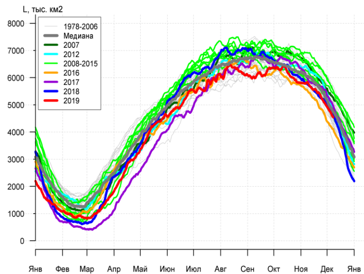
Рисунок 7а – Ежедневные оценки сезонного хода ледовитости Южного Океана и меридиональных секторов за период 26.10.1978 – 08.12.2019 по годам на основе расчетов по данным SSMR-SSM/I-SSMIS, алгоритм NASATEAM: а) Южный Океан, б) Атлантический сектор (60°W-30°E, море Уэдделла), в) Индоокеанский сектор (30°E-150°E, моря Космонавтов, Содружества, Моусона), г) Тихоокеанский сектор (150°E-60°W, моря Росса, Беллингаузена)
