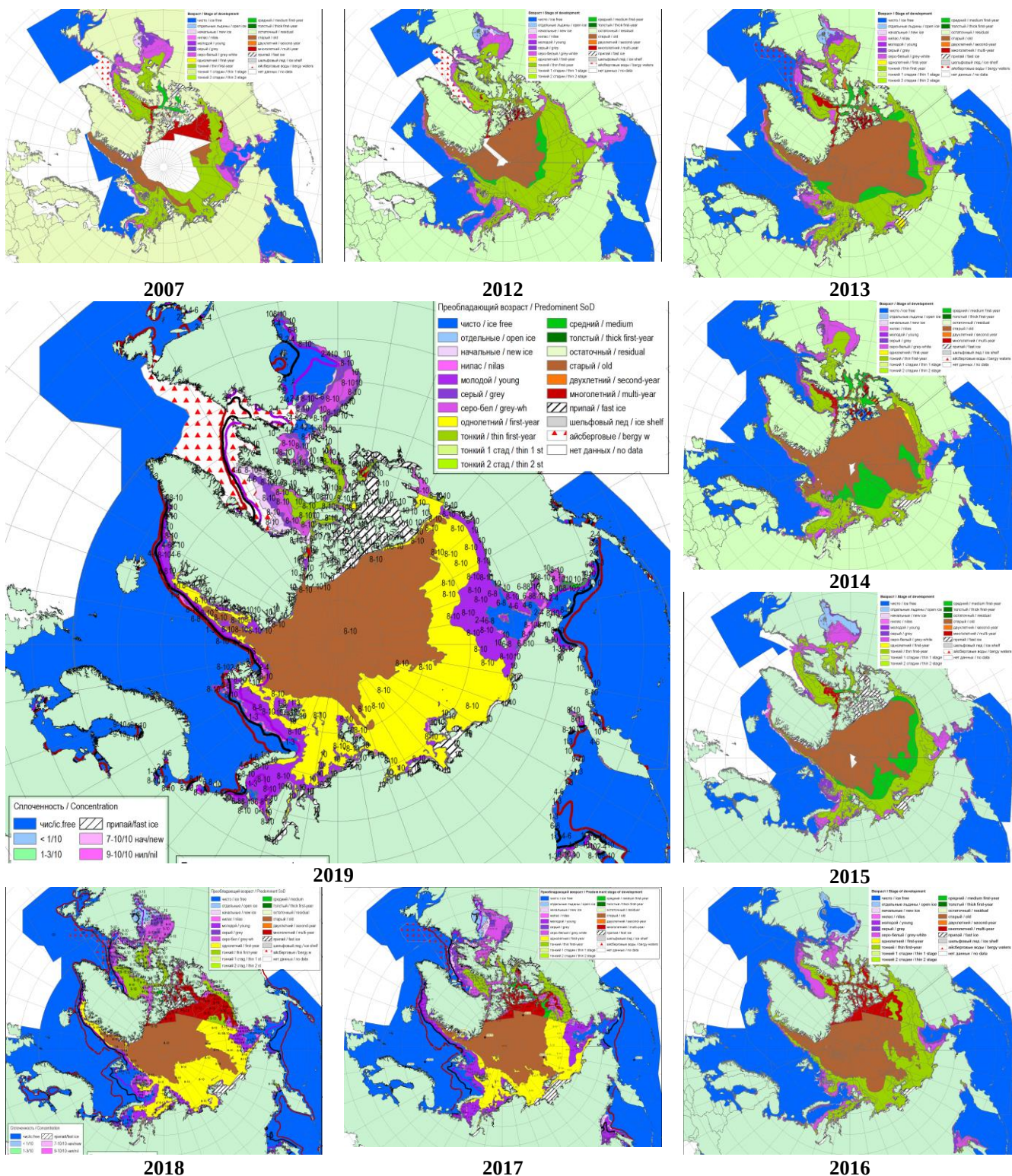
Рисунок 2а – Обзорная ледовая карта СЛО за 06.12 – 10.12.2019 г. и аналогичные периоды 2007-2018 гг. на основе ледового анализа ААНИИ, НИЦ Планета, Канадской ледовой службы и Национального ледового центра США.
