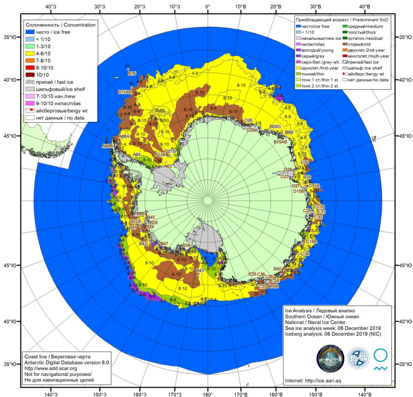
Рисунок 5б – Ледовая карта Южного океана (цветовая окраска по возрасту) и расположение крупных айсбергов на основе информации совместного ледового анализа НЛЦ США, ААНИИ и НМИ (Норвегия) за 06.12.2019.
