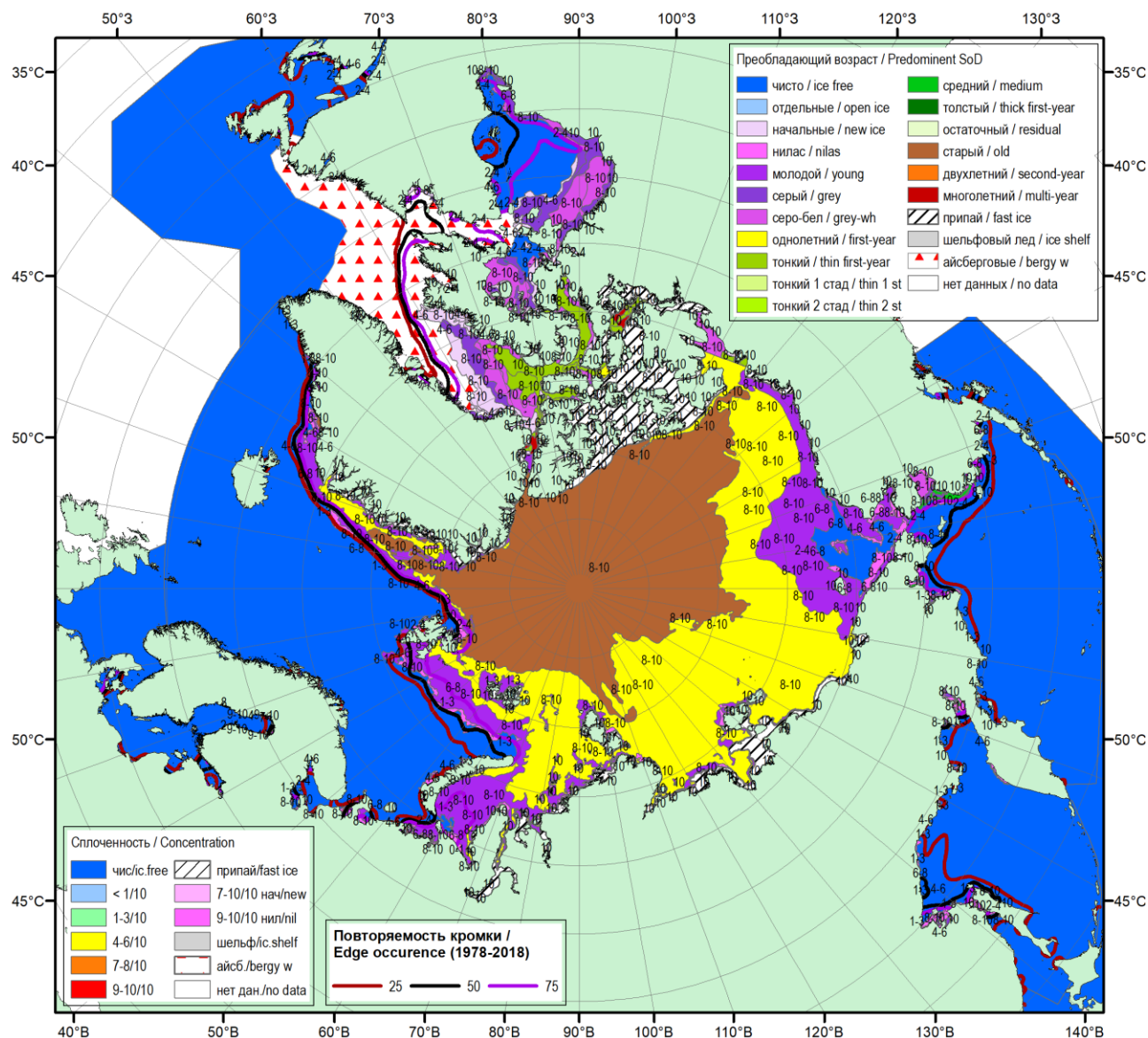
Рисунок 16 – Обзорная ледовая карта СЛО за 06.12.2019-10.12.2019 г. (цветовая раскраска по преобладающему возрасту) на основе ледового анализа ААНИИ (10.12), Национального ледового центра США (06.12) и повторяемость кромки за 06-10.12 за период 1979-2018 гг. по наблюдениям SSMR-SSM/I-SSMIS (алгоритм NASATEAM).
