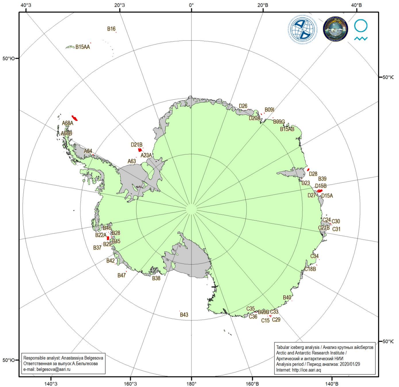
Рисунок 5д – Анализ ААНИИ крупных айсбергов Южного океана за 29.01.2020.
