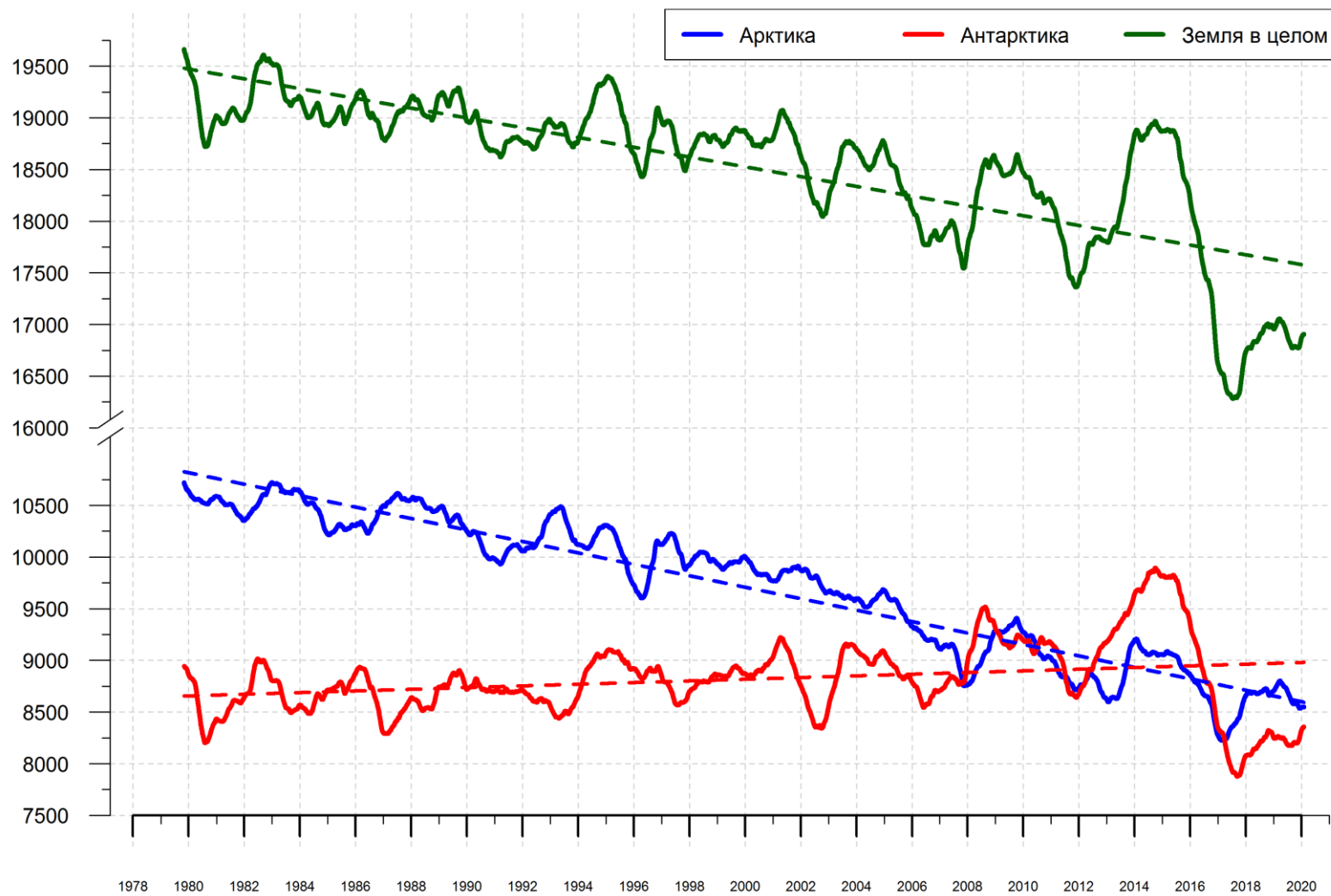
Рисунок 10 – Ежедневные сглаженные окном 365 суток значения ледовитости (площади распространения морского льда) Арктики, Антарктики и Земли в целом с 26.10.1978 по 02.02.2020 на основе SSMR-SSM/I-SSMIS
