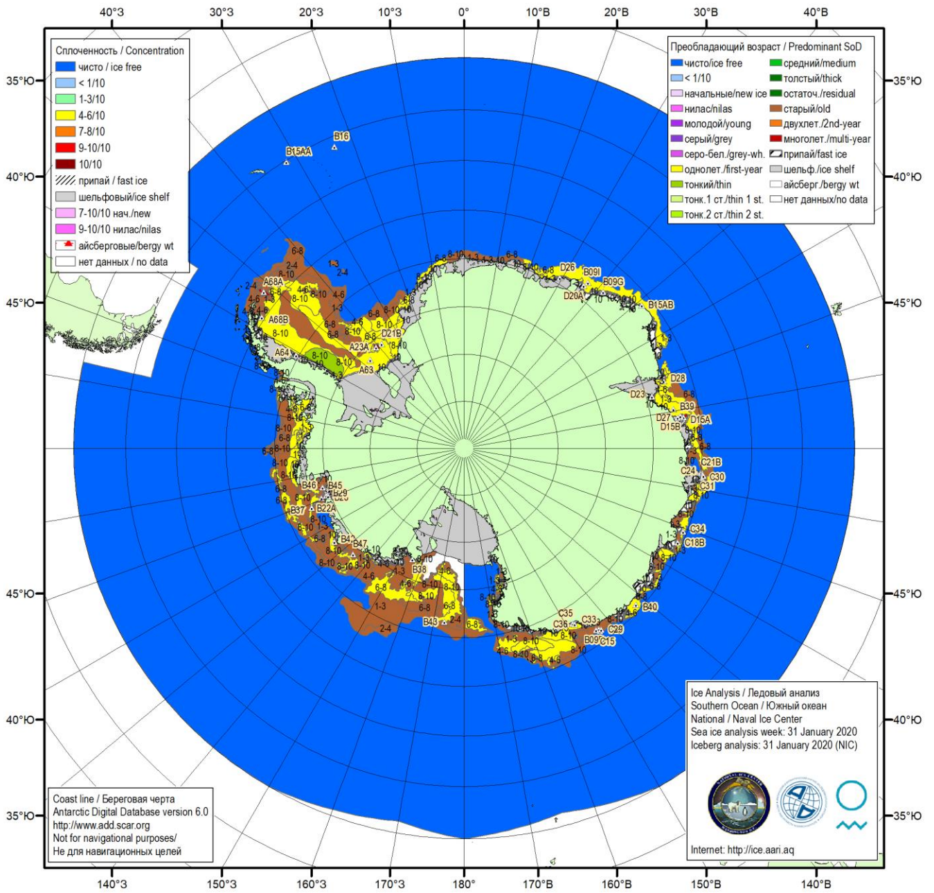
Рисунок 5б – Ледовая карта Южного океана (цветовая окраска по возрасту) и расположение крупных айсбергов на основе информации совместного ледового анализа НЛЦ США, ААНИИ и НМИ (Норвегия) за 31.01.2020.
