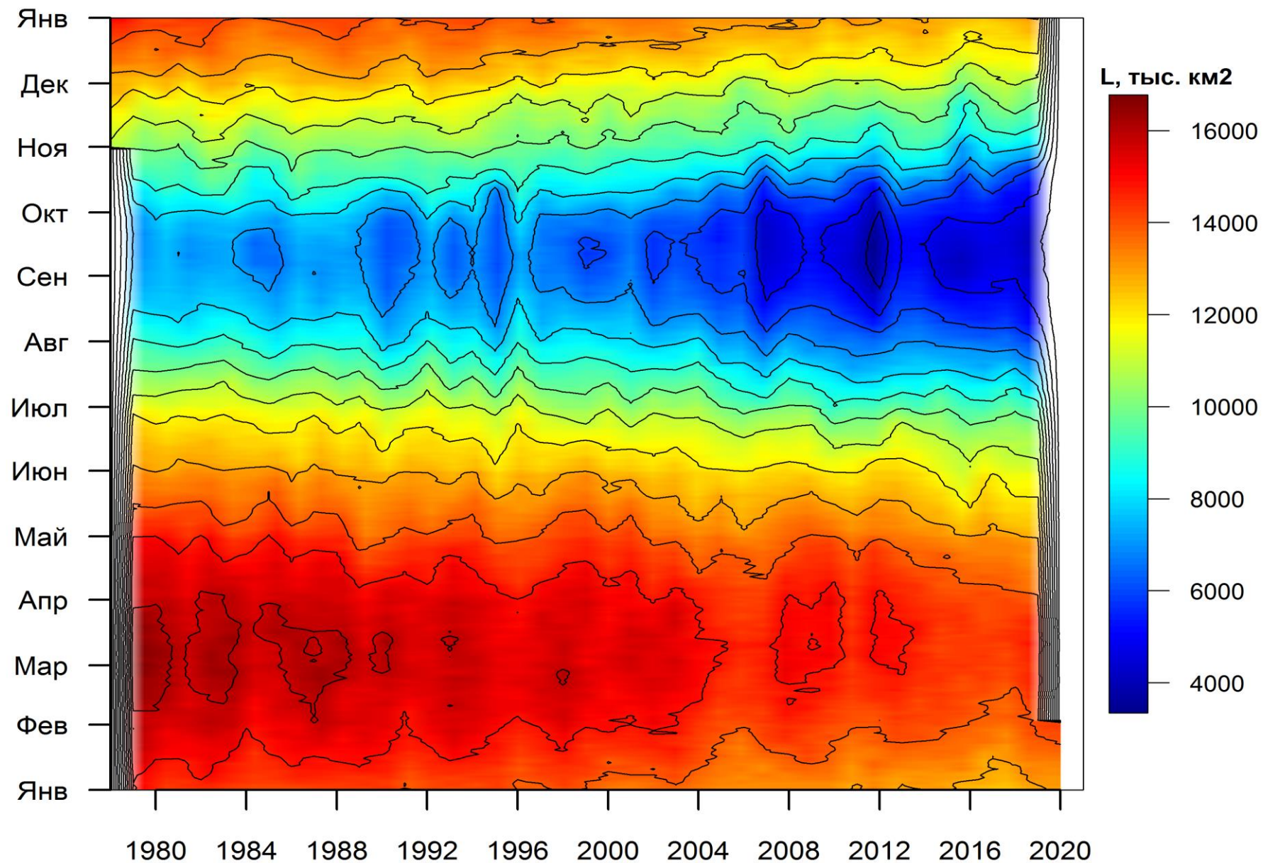
Рисунок 3б – Ежедневные оценки сезонных изменений ледовитости для Северной Полярной Области за период 26.10.1978 -02.02.2020 на основе расчетов по данным SSMR-SSM/I-SSMIS, алгоритм NASATEAM.
