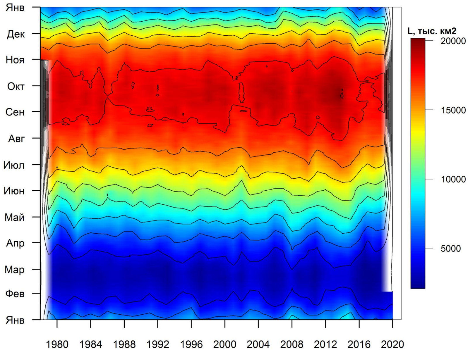
Рисунок 76 – Ежедневные оценки сезонных изменений ледовитости для Южного океана за период 26.10.1978 -02.02.2020 на основе расчетов по данным SSMR-SSM/I-SSMIS, алгоритм NASATEAM.
