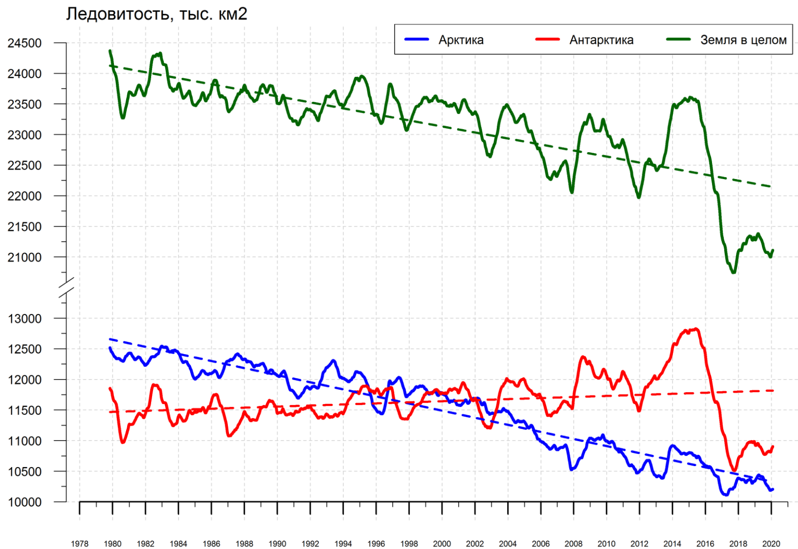
Рисунок 9 – Ежедневные сглаженные окном 365 суток значения приведенной ледовитости (площади морского льда) Арктики, Антарктики и Земли в целом с 26.10.1978 по 02.02.2020 на основе SSMR-SSM/I-SSMIS
