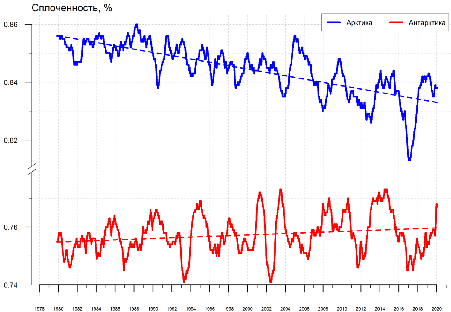
Рисунок 11 – Ежедневные сглаженные окном 365 суток значения средней общей сплоченности Арктики и Антарктики с 26.10.1978 по 02.02.2020 на основе SSMR-SSM/I-SSMIS
