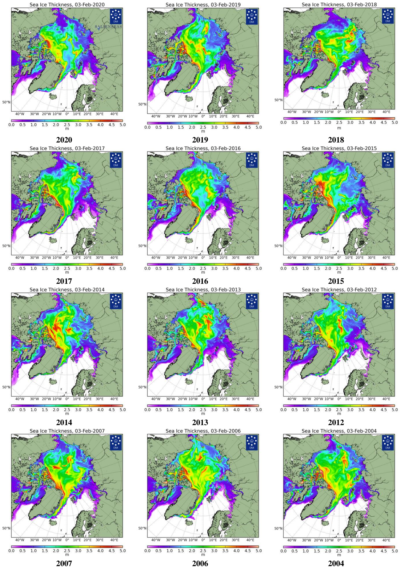
Рисунок 26 – Поля распределения средневзвешенной толщины льда совместной модели морского льда – океана NUCOM/CICE Датского метеорологического института 03.02 2004...2020 гг.
