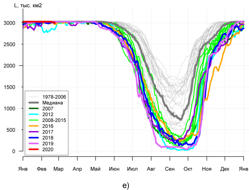
Рисунок 3а – Ежедневные оценки сезонного хода ледовитости для Северной Полярной Области и трех меридиональных секторов за период 26.10.1978 -23.02.2020 по годам на основе расчетов по данным SSMR-SSM/I-SSMIS, алгоритмы NASATEAM: а) Северная полярная область, б) сектор 45°W-95°E (Гренландское – Карское моря), в) сектор 95°E-170°W (моря Лаптевых – Чукотское и Берингово, Охотское), г) сектор 170°W-45°W (море Бофорта и Канадская Арктика), д) Северный Ледовитый океан, е) Северный морской путь (Карское - Чукотское моря).
