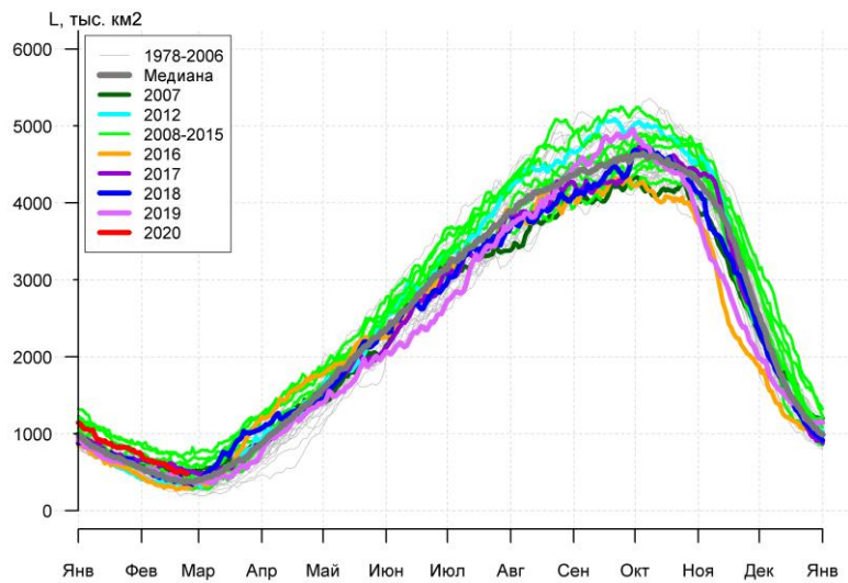
Рисунок 7а – Ежедневные оценки сезонного хода ледовитости Южного Океана и меридиональных секторов за период 26.10.1978 – 23.02.2020 по годам на основе расчетов по данным SSMR-SSM/I-SSMIS, алгоритм NASATEAM: а) Южный Океан, б) Атлантический сектор (60°W-30°E, море Уэдделла), в) Индоокеанский сектор (30°E-150°E, моря Космонавтов, Содружества, Моусона), г) Тихоокеанский сектор (150°E-60°W, моря Росса, Беллинсгаузена)
