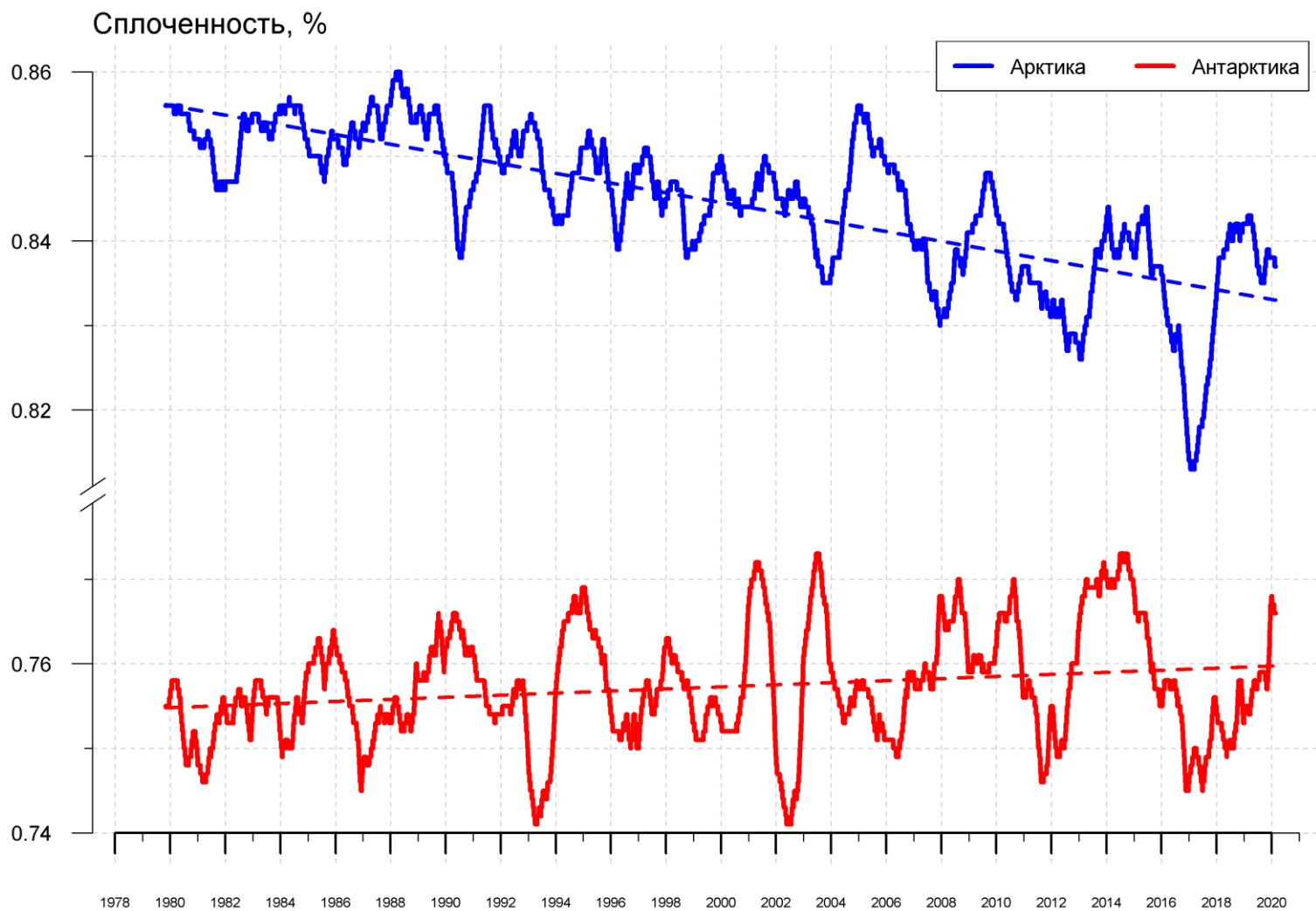
Рисунок 11 – Ежедневные сглаженные окном 365 суток значения средней общей сплоченности Арктики и Антарктики с 26.10.1978 по 23.02.2020 на основе SSMR-SSM/I-SSMIS
