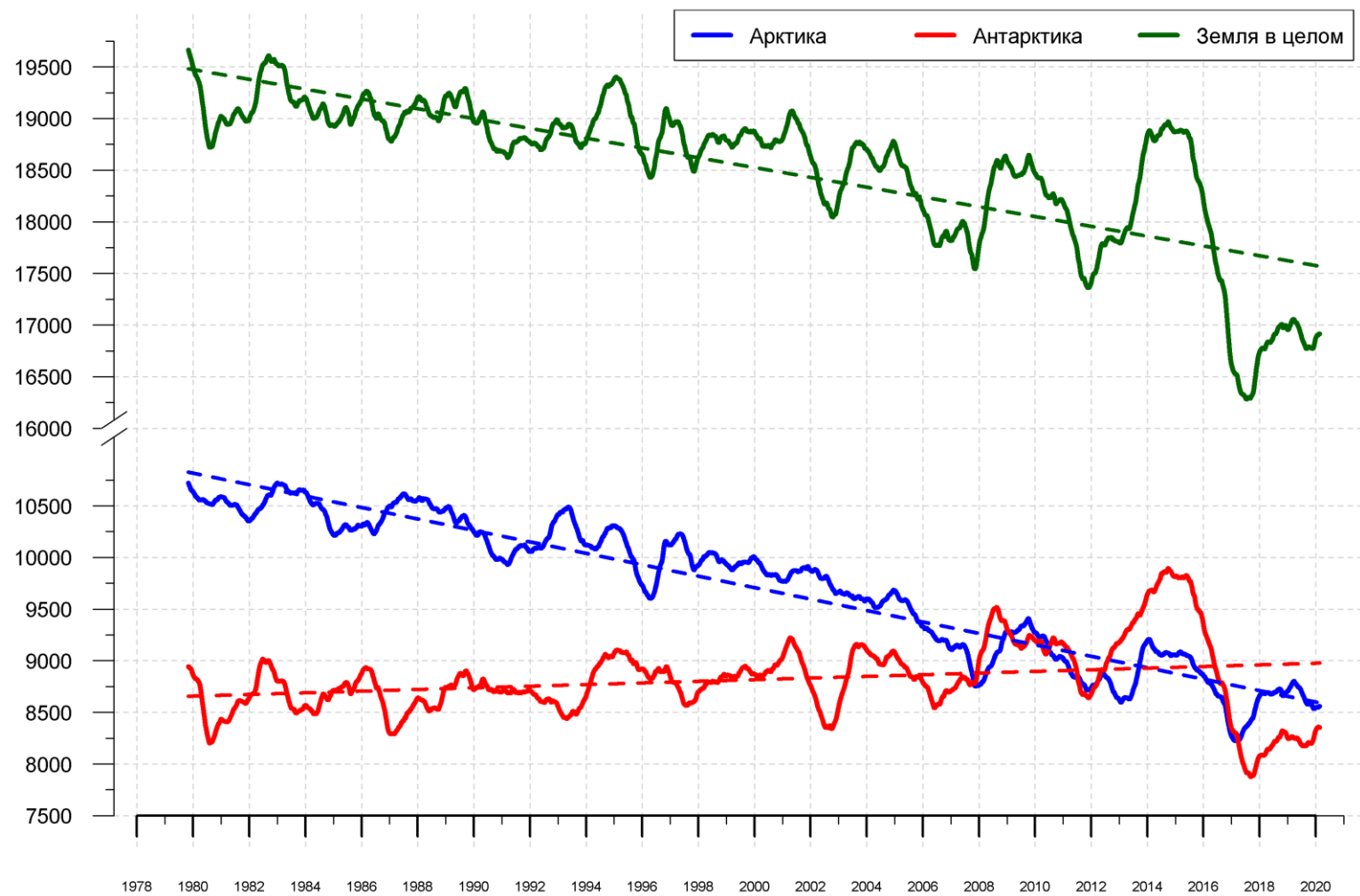
Рисунок 10 – Ежедневные сглаженные окном 365 суток значения ледовитости (площади распространения морского льда) Арктики, Антарктики и Земли в целом с 26.10.1978 по 23.02.2020 на основе SSMR-SSM/I-SSMIS
