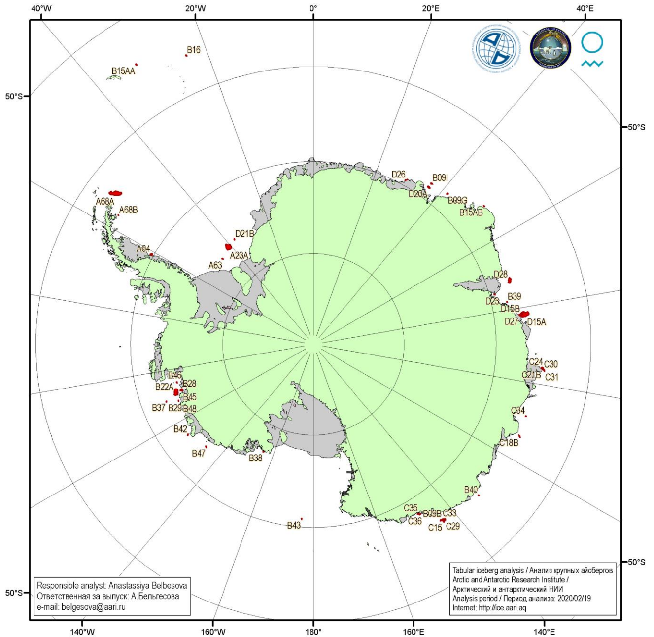
Рисунок 5д – Анализ ААНИИ крупных айсбергов Южного океана за 19.02.2020.
