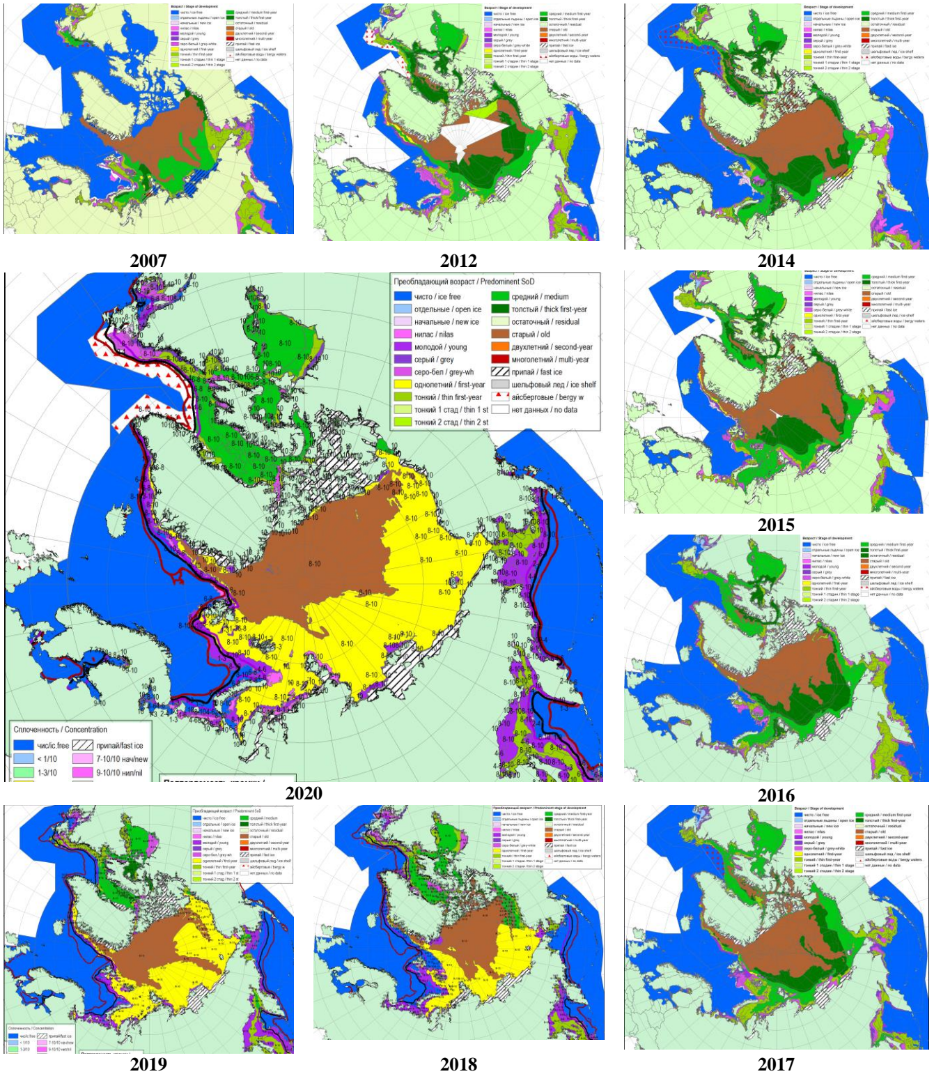
Рисунок 2а – Обзорная ледовая карта СЛО за 21.02 –25.02.2020 г. и аналогичные периоды 2007-2019 гг. на основе ледового анализа ААНИИ, НИЦ Планета, Канадской ледовой службы и Национального ледового центра США.
