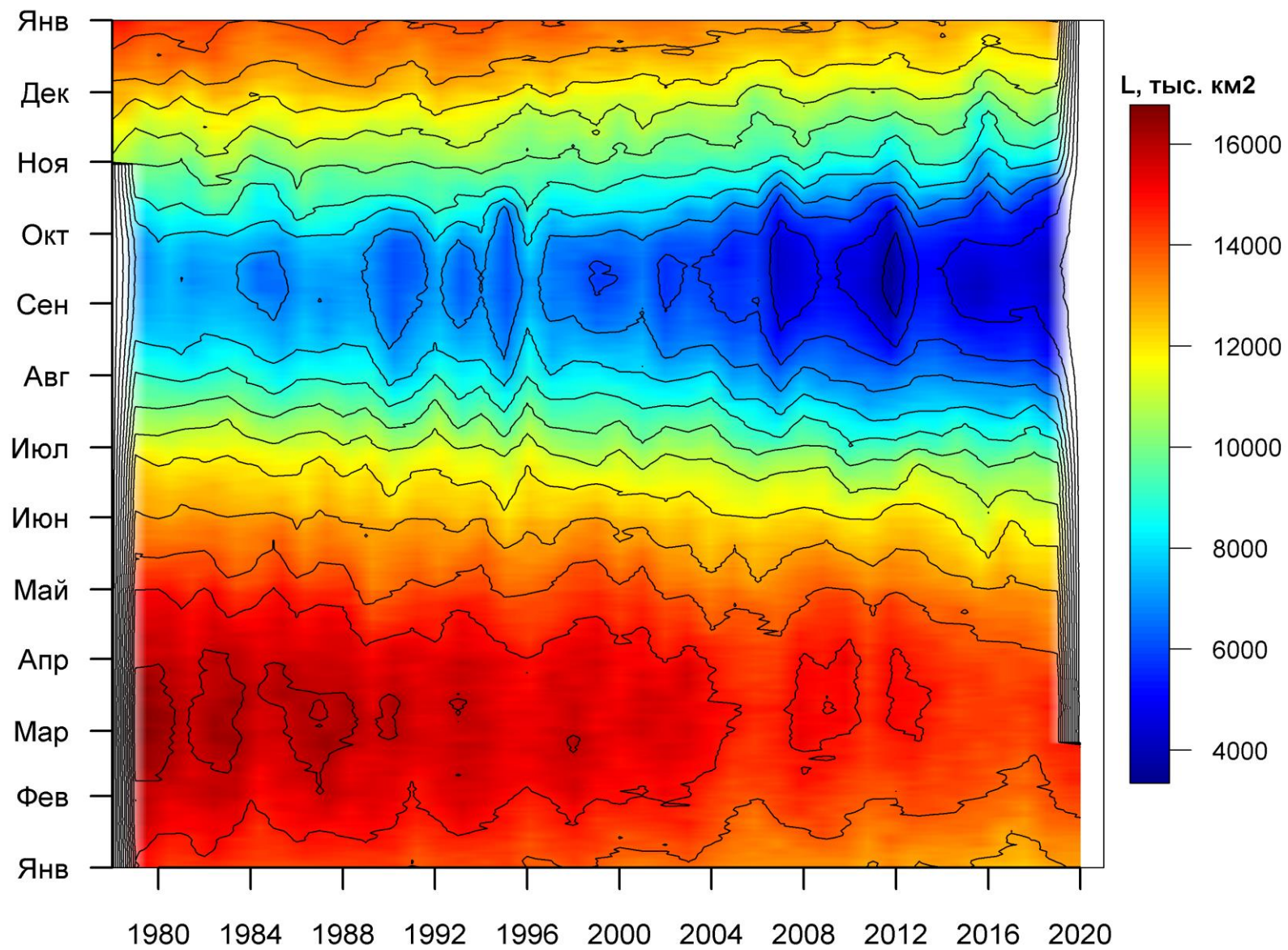
Рисунок 3б – Ежедневные оценки сезонных изменений ледовитости для Северной Полярной Области за период 26.10.1978 -23.02.2020 на основе расчетов по данным SSMR-SSM/I-SSMIS, алгоритм NASATEAM.
