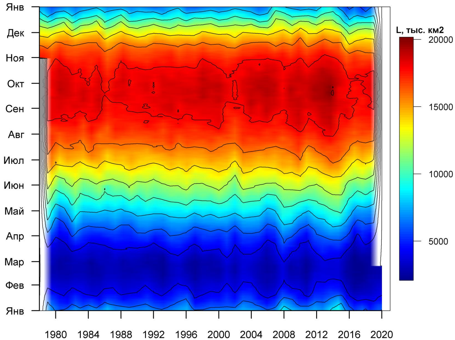
Рисунок 76 – Ежедневные оценки сезонных изменений ледовитости для Южного океана за период 26.10.1978 -23.02.2020 на основе расчетов по данным SSMR-SSM/I-SSMIS, алгоритм NASATEAM.
