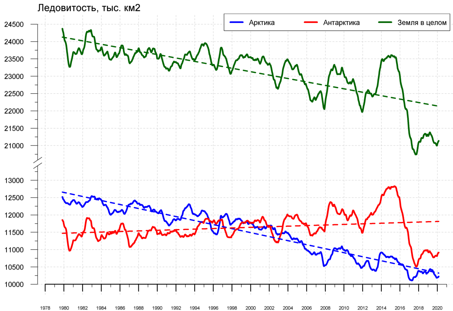
Рисунок 9 – Ежедневные сглаженные окном 365 суток значения приведенной ледовитости (площади морского льда) Арктики, Антарктики и Земли в целом с 26.10.1978 по 23.02.2020 на основе SSMR-SSM/I-SSMIS
