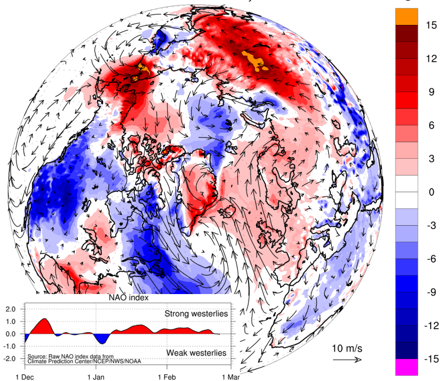
Рисунок 2е – Аномалии приземной температуры воздуха (2м) и осредненные вектора скорости ветра (10 м) за 20.02-24.02.2020 гг. относительно периода 2004-2013 гг. ( http://polarportal.dk )
