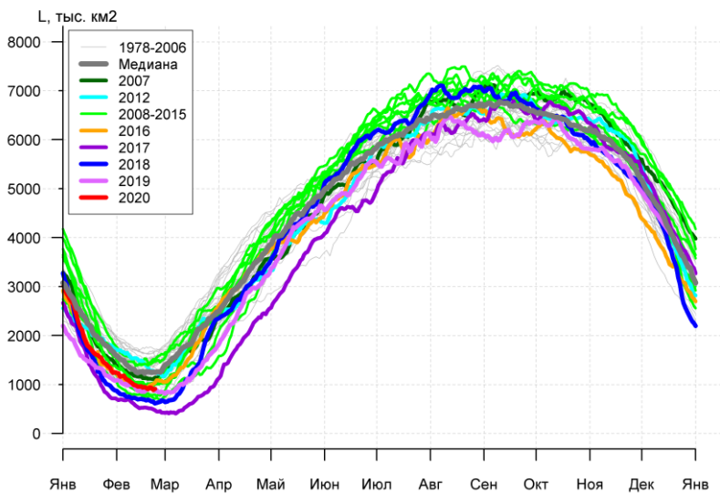
Рисунок 7а – Ежедневные оценки сезонного хода ледовитости Южного Океана и меридиональных секторов за период 26.10.1978 – 23.02.2020 по годам на основе расчетов по данным SSMR-SSM/I-SSMIS, алгоритм NASATEAM: а) Южный Океан, б) Атлантический сектор (60°W-30°E, море Уэдделла), в) Индоокеанский сектор (30°E-150°E, моря Космонавтов, Содружества, Моусона), г) Тихоокеанский сектор (150°E-60°W, моря Росса, Беллинсгаузена)
