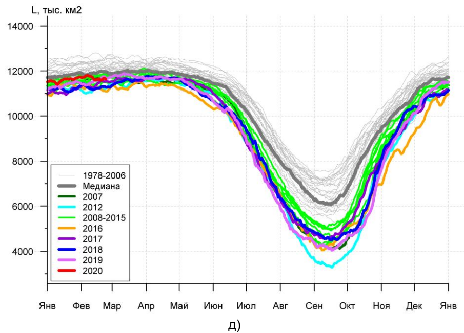
Рисунок 3а – Ежедневные оценки сезонного хода ледовитости для Северной Полярной Области и трех меридиональных секторов за период 26.10.1978 -23.02.2020 по годам на основе расчетов по данным SSMR-SSM/I-SSMIS, алгоритмы NASATEAM: а) Северная полярная область, б) сектор 45°W-95°E (Гренландское – Карское моря), в) сектор 95°E-170°W (моря Лаптевых – Чукотское и Берингово, Охотское), г) сектор 170°W-45°W (море Бофорта и Канадская Арктика), д) Северный Ледовитый океан, е) Северный морской путь (Карское - Чукотское моря).
