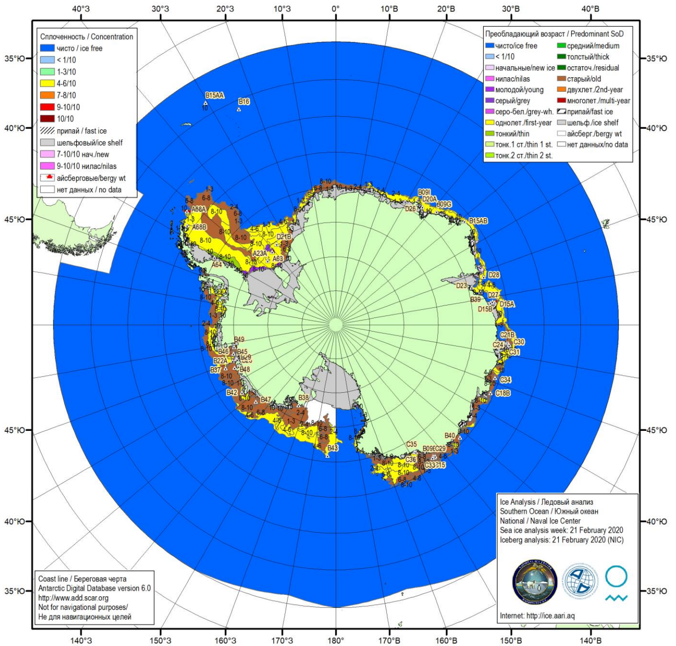
Рисунок 5б – Ледовая карта Южного океана (цветовая окраска по возрасту) и расположение крупных айсбергов на основе информации совместного ледового анализа НЛЦ США, ААНИИ и НМИ (Норвегия) за 21.02.2020.
