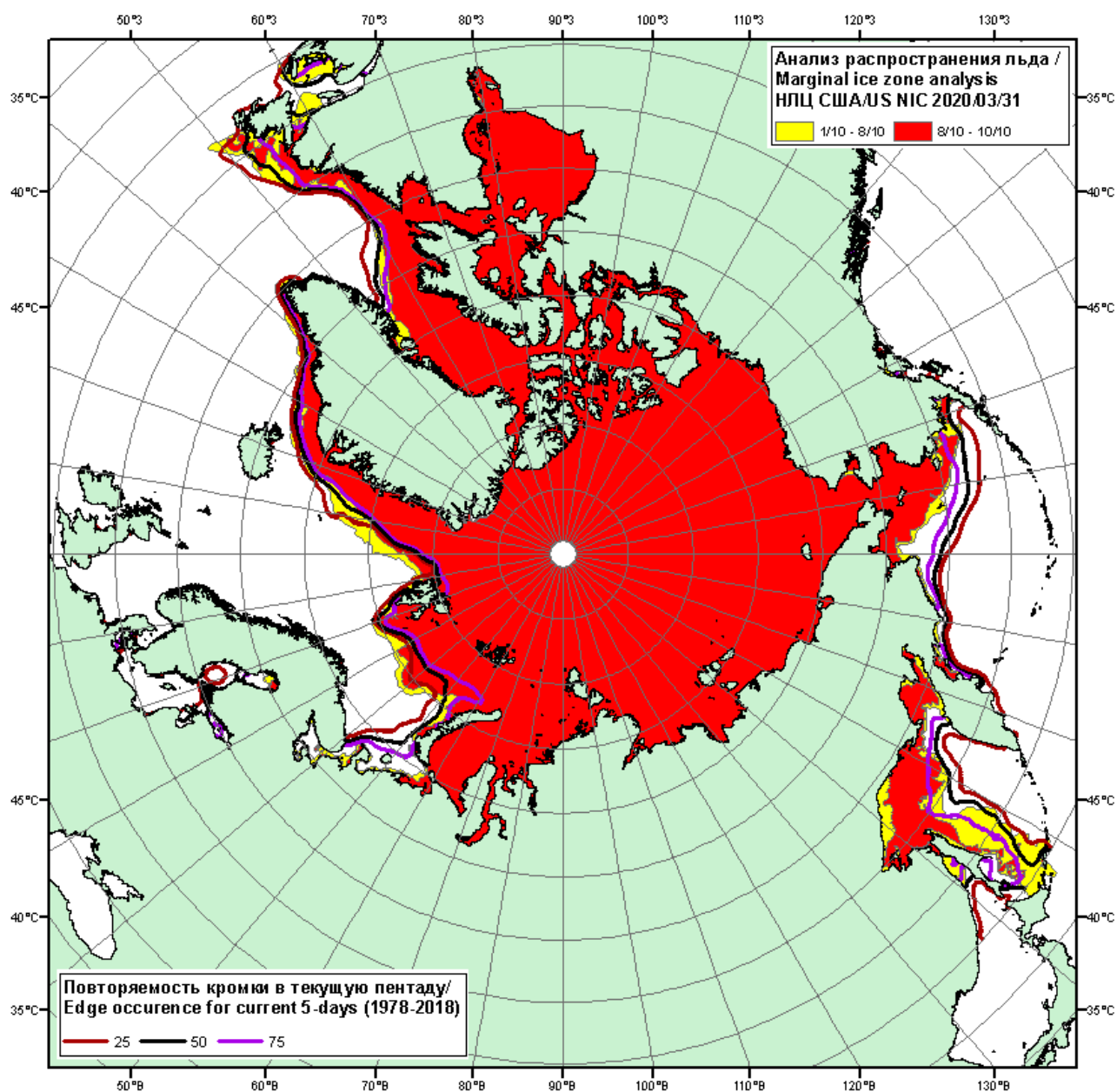
Рисунок 1в – Положение кромки льда и зон разреженных ( <8/10 ) и сплоченных ( \geq 8/10 ) льдов СЛО за 31.03.2020 г. на основе ледового анализа Национального Ледового Центра США и повторяемость кромки за 26-31.03 за период 1979-2018 гг. по наблюдениям SSMR-SSM/I-SSMIS (алгоритм NASATEAM)
