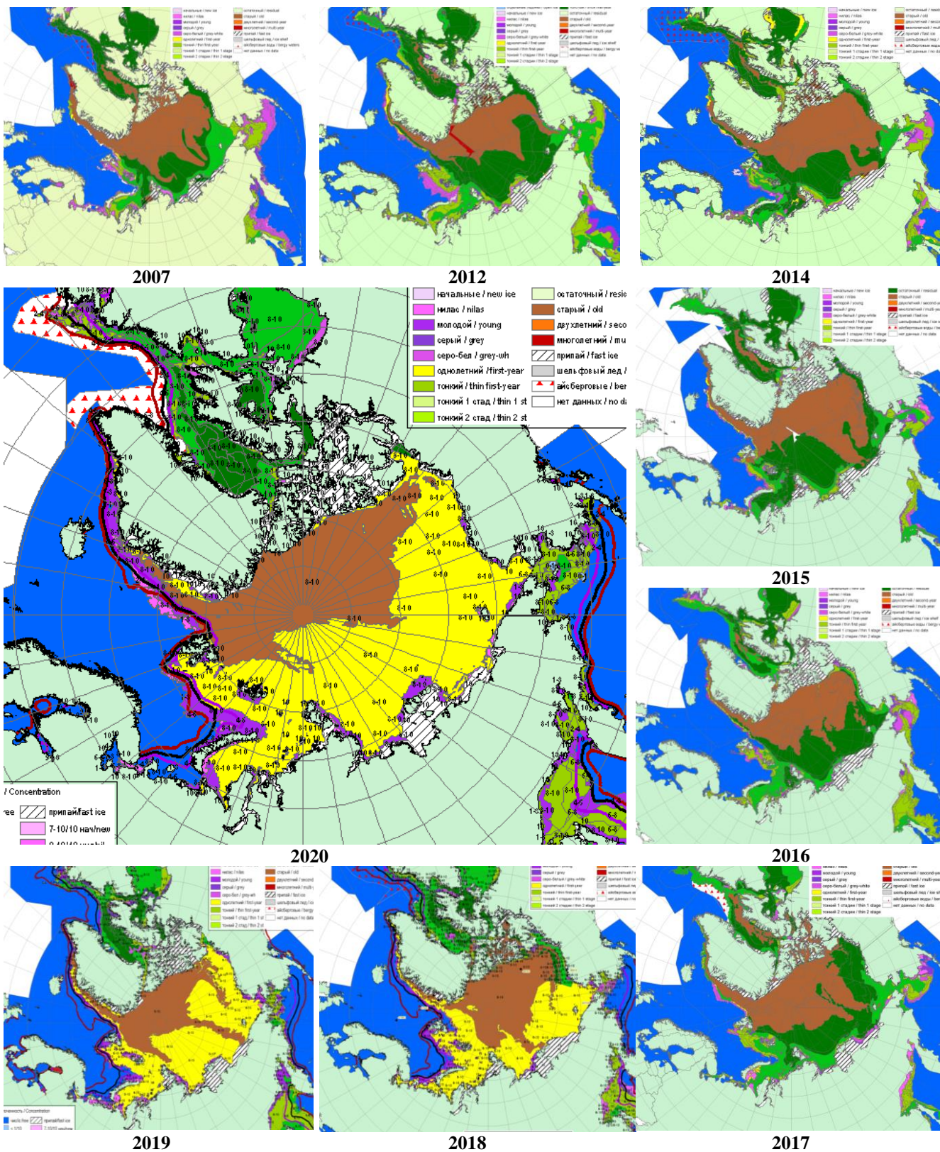
Рисунок 2а – Обзорная ледовая карта СЛО за 26.03 – 31.03.2020 г. и аналогичные периоды 2007-2019гг. на основе ледового анализа ААНИИ, НИЦ Планета, Канадской ледовой службы и Национального ледового центра США.
