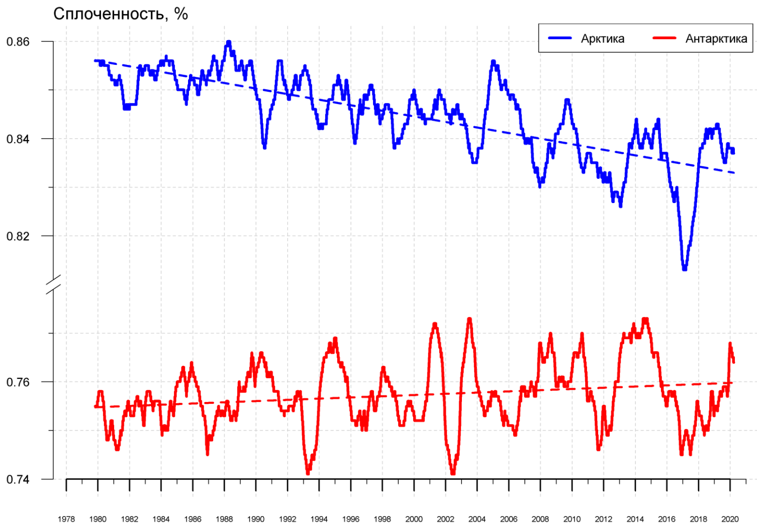
Рисунок 11 – Ежедневные сглаженные окном 365 суток значения средней общей сплоченности Арктики и Антарктики с 26.10.1978 по 25.03.2020 на основе SSMR-SSM/I-SSMIS
