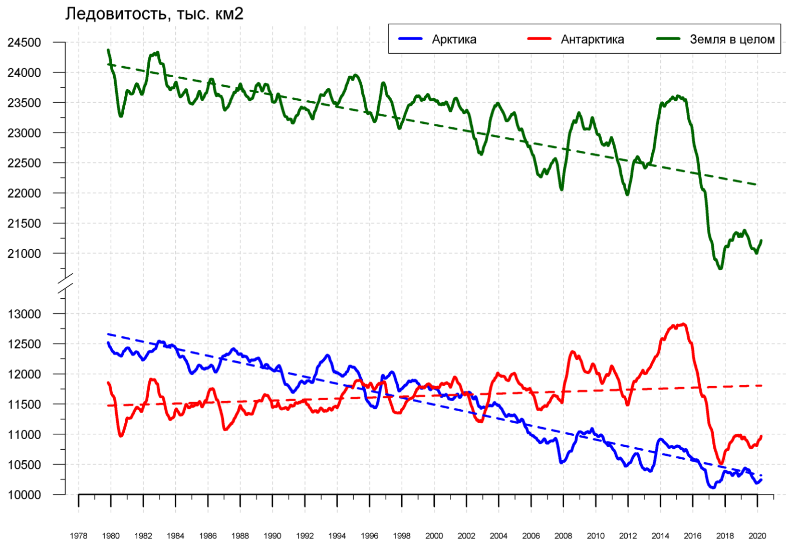
Рисунок 9 – Ежедневные сглаженные окном 365 суток значения приведенной ледовитости (площади морского льда) Арктики, Антарктики и Земли в целом с 26.10.1978 по 25.03.2020 на основе SSMR-SSM/I-SSMIS
