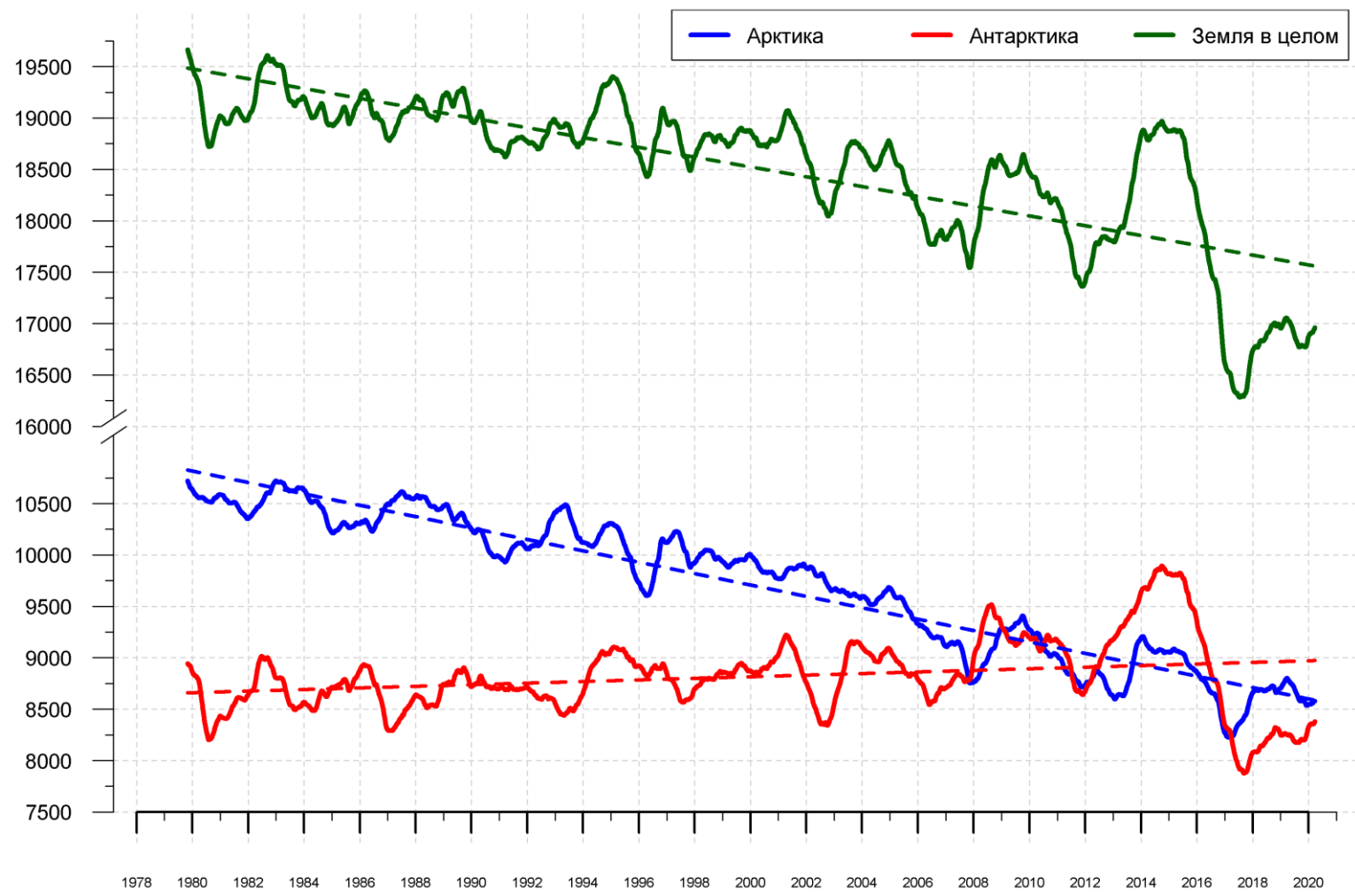
Рисунок 10 – Ежедневные сглаженные окном 365 суток значения ледовитости (площади распространения морского льда) Арктики, Антарктики и Земли в целом с 26.10.1978 по 25.03.2020 на основе SSMR-SSM/I-SSMIS
