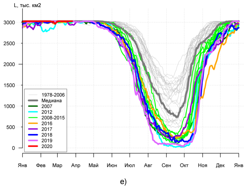
Рисунок 3а – Ежедневные оценки сезонного хода ледовитости для Северной Полярной Области и трех меридиональных секторов за период 26.10.1978 -25.03.2020 по годам на основе расчетов по данным SSMR-SSM/I-SSMIS, алгоритмы NASATEAM: а) Северная полярная область, б) сектор 45°W-95°E (Гренландское – Карское моря), в) сектор 95°E-170°W (моря Лаптевых – Чукотское и Берингово, Охотское), г) сектор 170°W-45°W (море Бофорта и Канадская Арктика), д) Северный Ледовитый океан, е) Северный морской путь (Карское - Чукотское моря).
