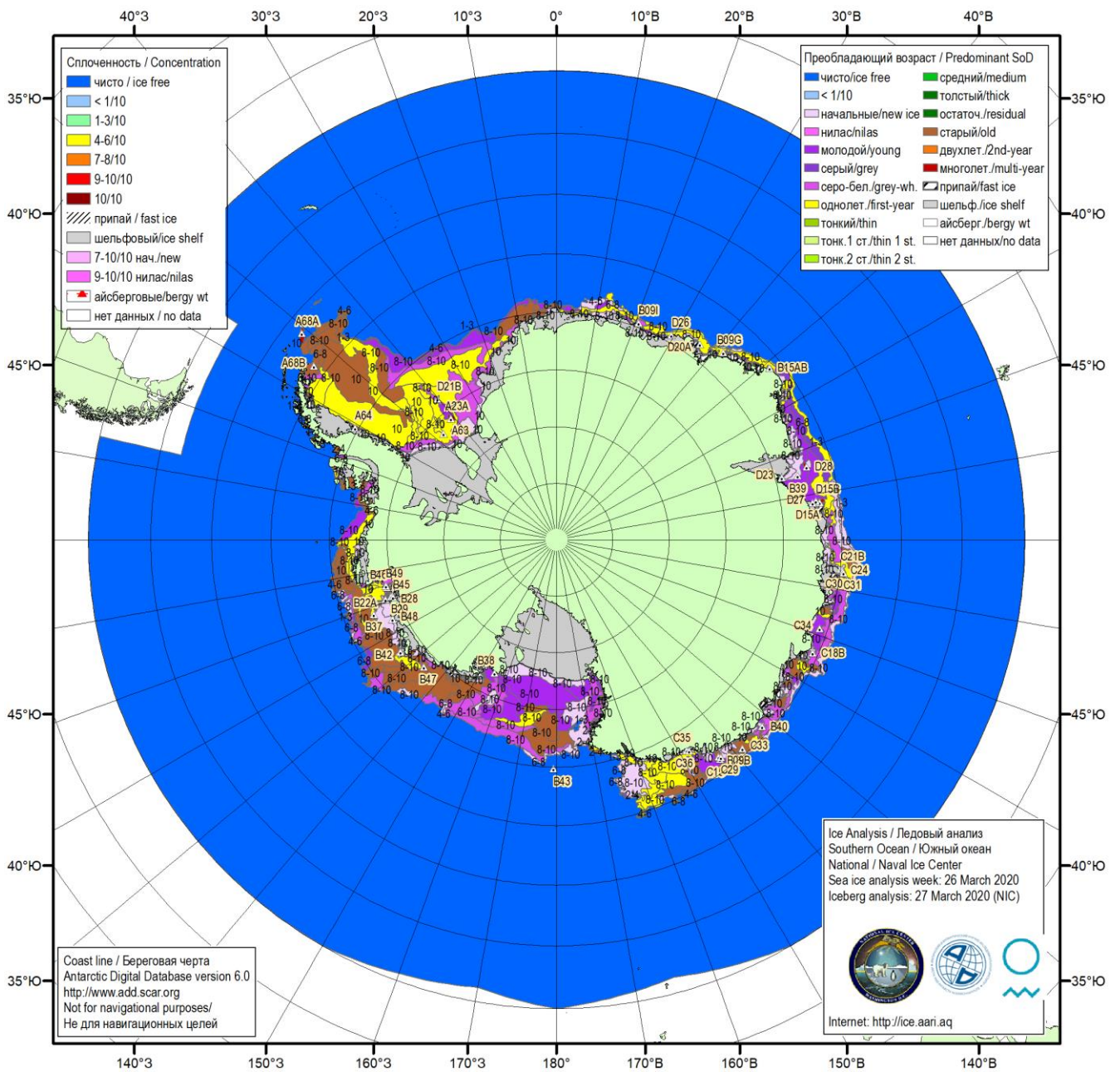
Рисунок 5б – Ледовая карта Южного океана (цветовая окраска по возрасту) и расположение крупных айсбергов на основе информации совместного ледового анализа НЛЦ США, ААНИИ и НМИ (Норвегия) за 26.03.2020.
