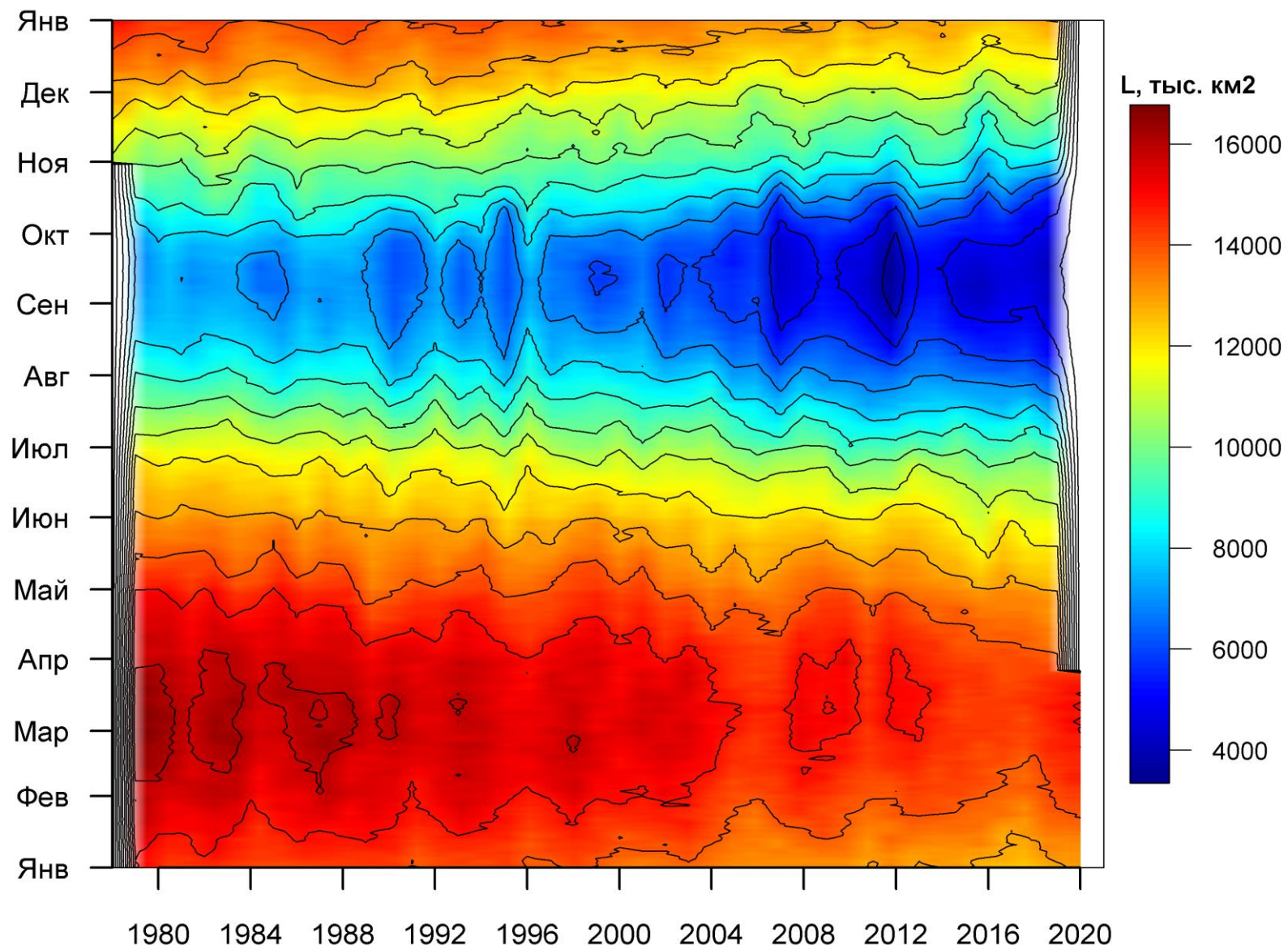
Рисунок 3б – Ежедневные оценки сезонных изменений ледовитости для Северной Полярной Области за период 26.10.1978 - 25.03.2020 на основе расчетов по данным SSMR-SSM/I-SSMIS, алгоритм NASATEAM.
