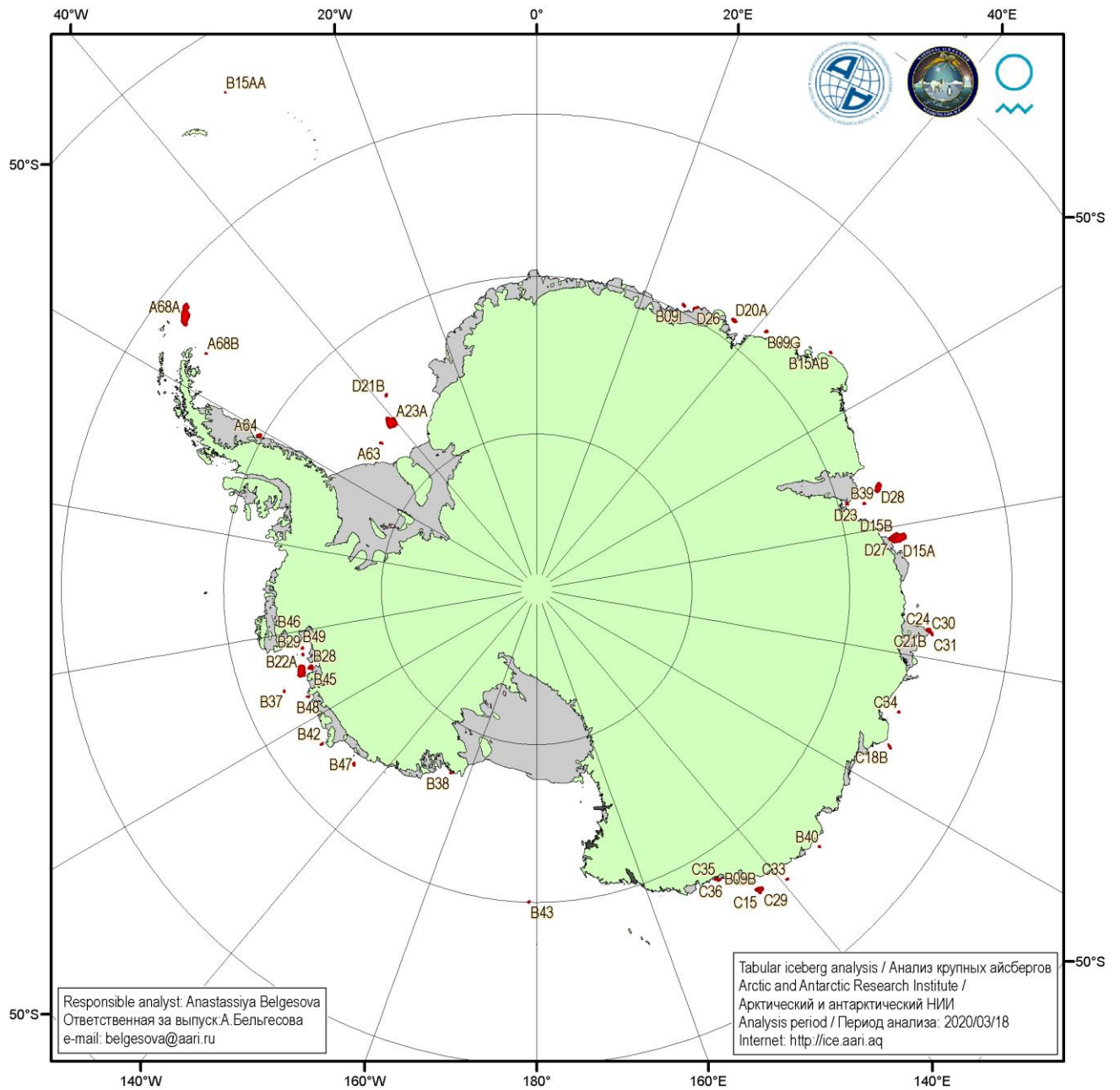
Рисунок 5д – Анализ ААНИИ крупных айсбергов Южного океана за 18.03.2020.
