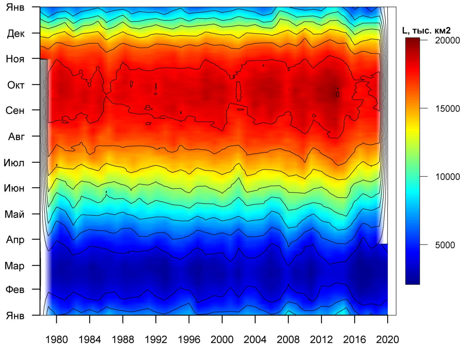
Рисунок 76 – Ежедневные оценки сезонных изменений ледовитости для Южного океана за период 26.10.1978 -25.03.2020 на основе расчетов по данным SSMR-SSM/I-SSMIS, алгоритм NASATEAM.
