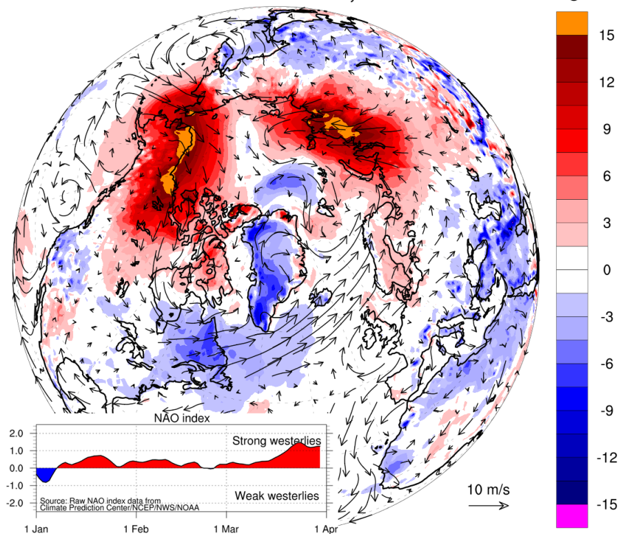
Рисунок 2е – Аномалии приземной температуры воздуха (2м) и осредненные вектора скорости ветра (10 м) за 26.03-30.03.2020 гг. относительно периода 2004-2013 гг. ( http://polarportal.dk )
