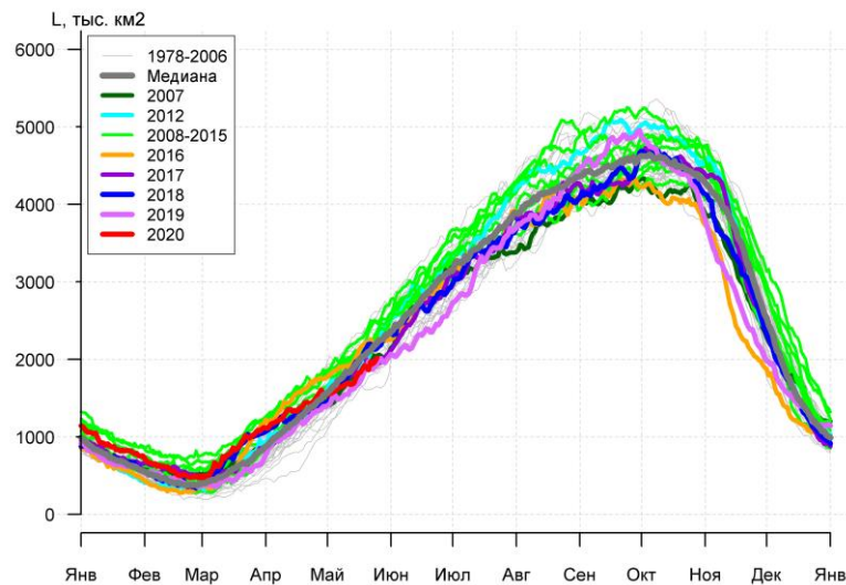
Рисунок 7а – Ежедневные оценки сезонного хода ледовитости Южного Океана и меридиональных секторов за период 26.10.1978 – 24.05.2020 по годам на основе расчетов по данным SSMR-SSM/I-SSMIS, алгоритм NASATEAM: а) Южный Океан, б) Атлантический сектор (60°W-30°E, море Уэдделла), в) Индоокеанский сектор (30°E-150°E, моря Космонавтов, Содружества, Моусона), г) Тихоокеанский сектор (150°E-60°W, моря Росса, Беллингаузена)
