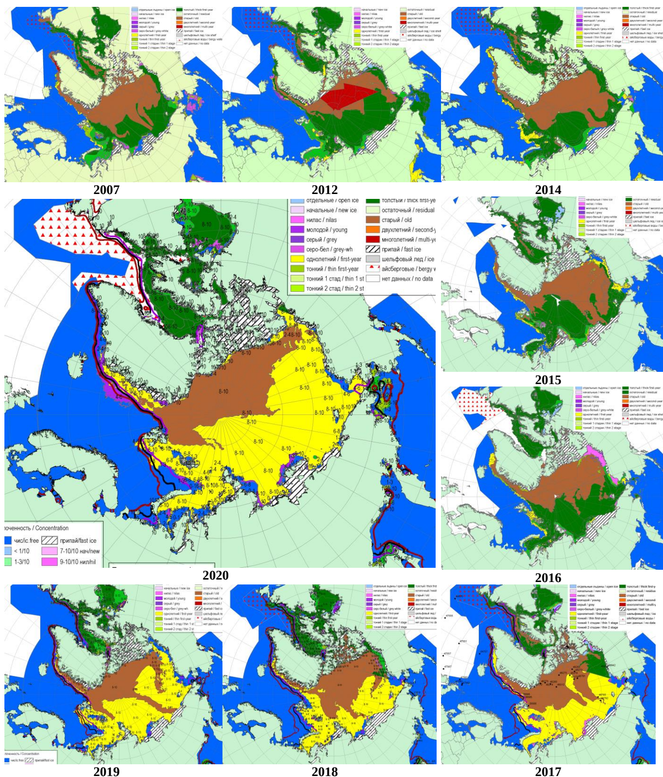
Рисунок 2а – Обзорная ледовая карта СЛО за 21.05 – 26.05.2020 г. и аналогичные периоды 2007-2019гг. на основе ледового анализа ААНИИ, НИЦ Планета, Канадской ледовой службы и Национального ледового центра США.
