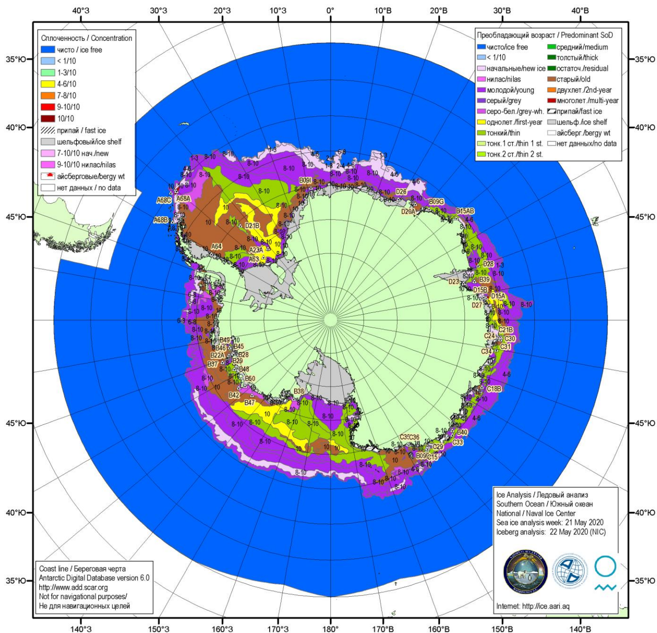
Рисунок 5б – Ледовая карта Южного океана (цветовая окраска по возрасту) и расположение крупных айсбергов на основе информации совместного ледового анализа НЛЦ США, ААНИИ и НМИ (Норвегия) за 21.05.2020.
