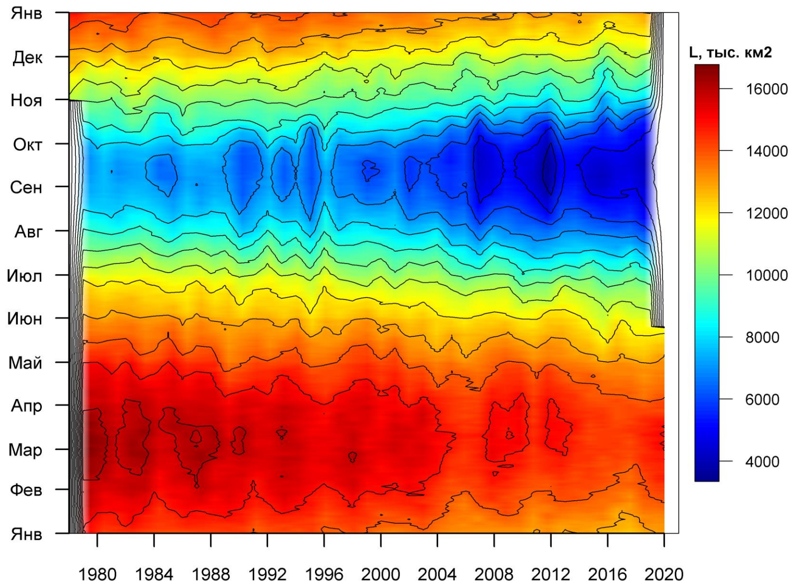
Рисунок 3б – Ежедневные оценки сезонных изменений ледовитости для Северной Полярной Области за период 26.10.1978 – 24.05.2020 на основе расчетов по данным SSMR-SSM/I-SSMIS, алгоритм NASATEAM.
