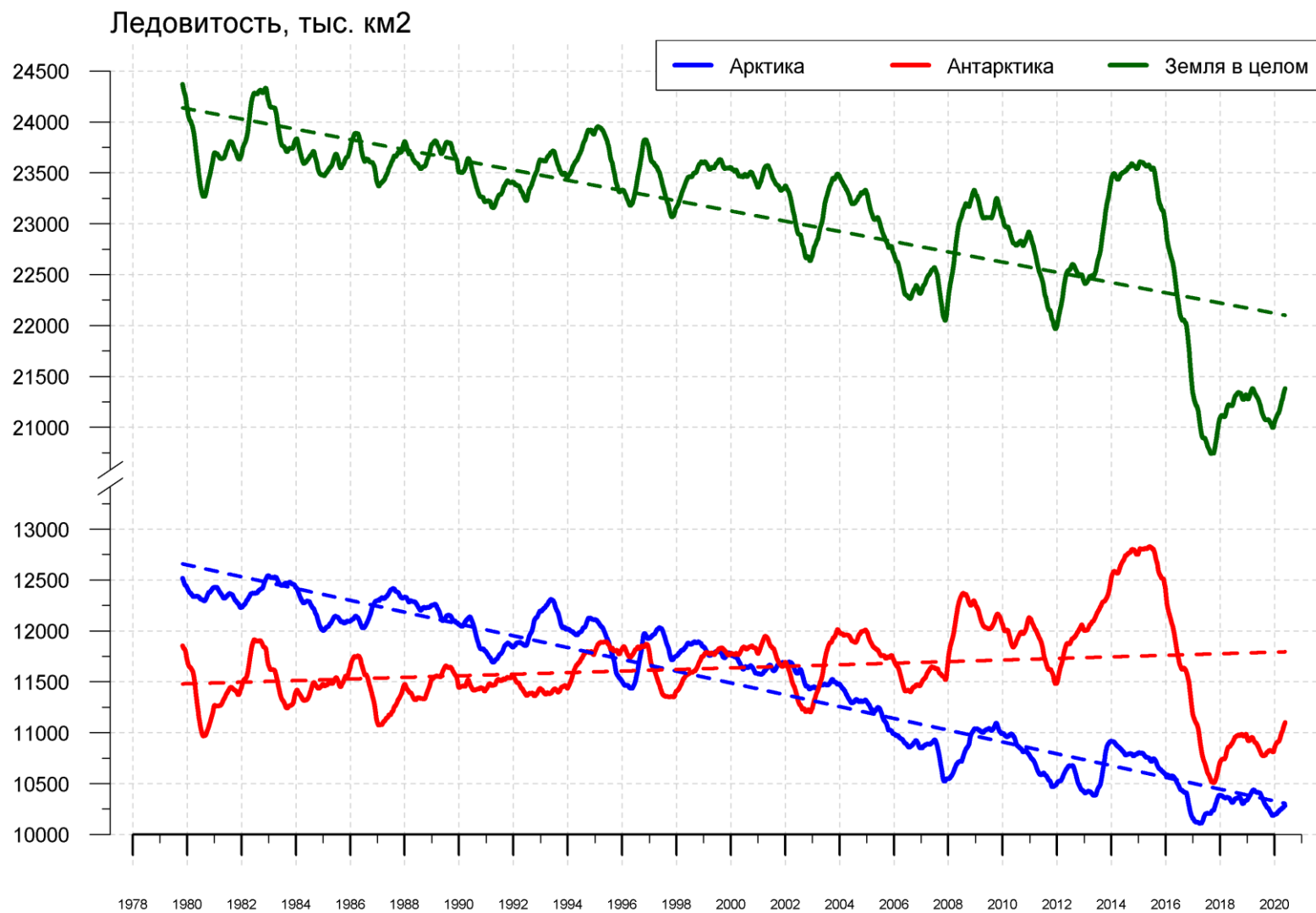
Рисунок 9 – Ежедневные сглаженные окном 365 суток значения приведенной ледовитости (площади морского льда) Арктики, Антарктики и Земли в целом с 26.10.1978 по 24.05.2020 на основе SSMR-SSM/I-SSMIS
