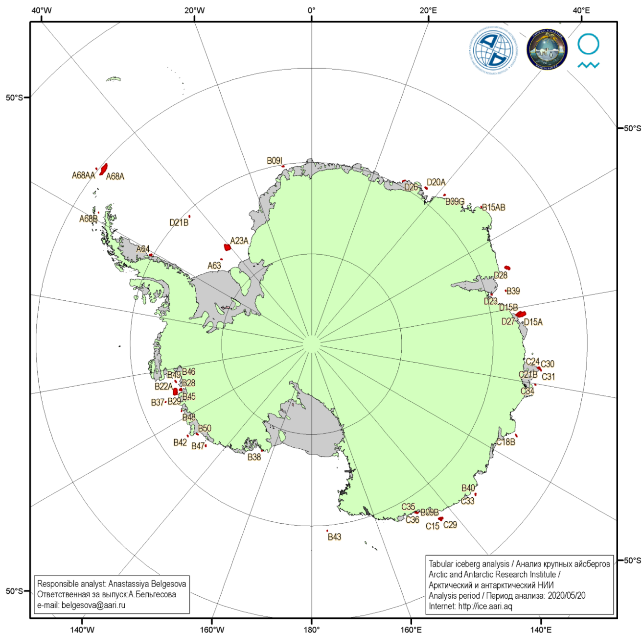
Рисунок 5д – Анализ ААНИИ крупных айсбергов Южного океана за 20.05.2020.
