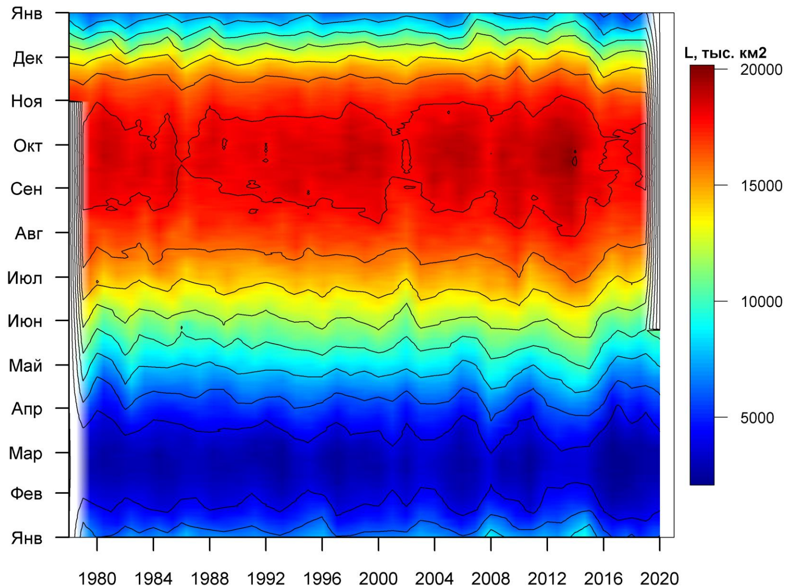
Рисунок 76 – Ежедневные оценки сезонных изменений ледовитости для Южного океана за период 26.10.1978 - 24.05.2020 на основе расчетов по данным SSMR-SSM/I-SSMIS, алгоритм NASATEAM.
