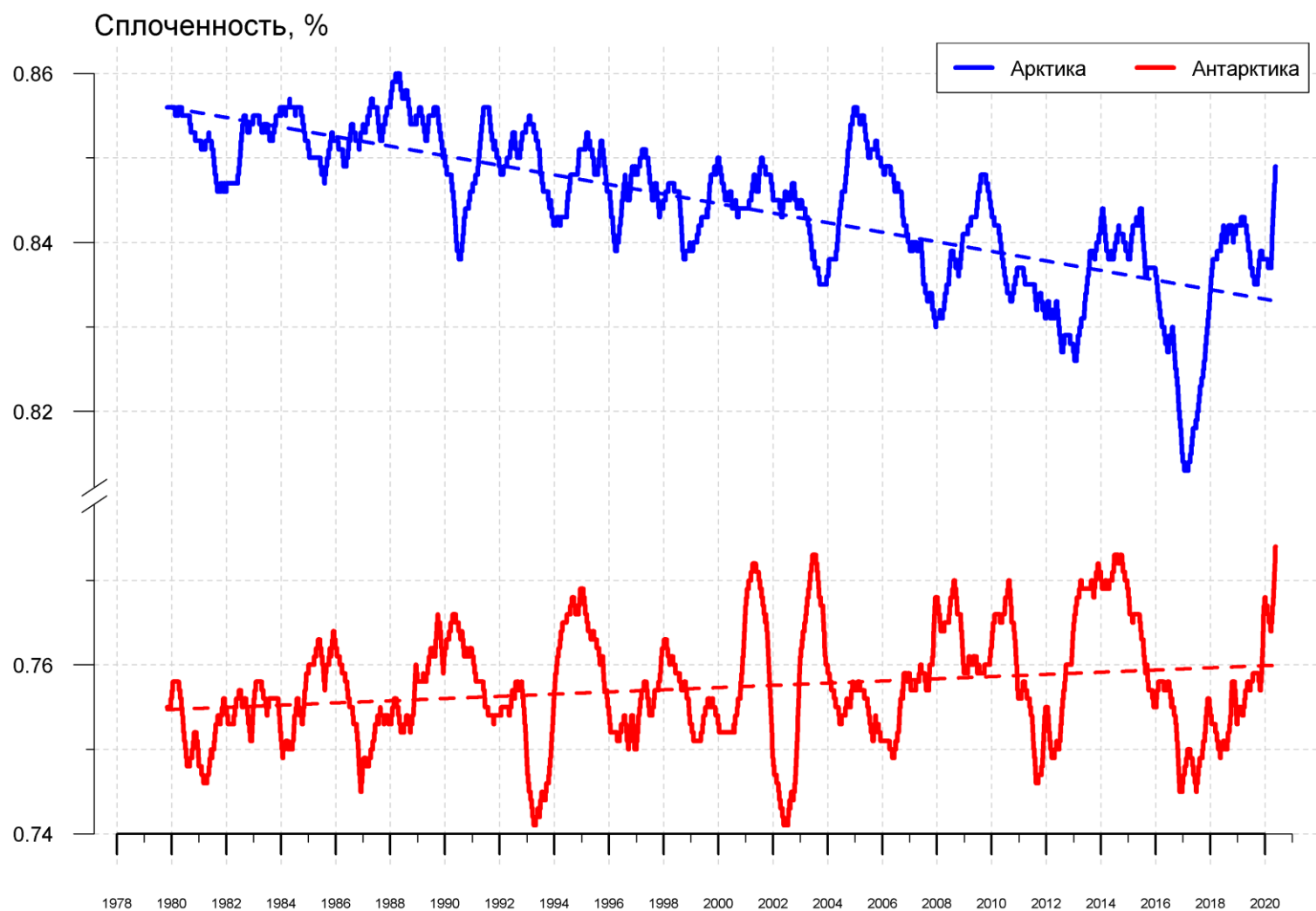
Рисунок 11 – Ежедневные сглаженные окном 365 суток значения средней общей сплоченности Арктики и Антарктики с 26.10.1978 по 24.05.2020 на основе SSMR-SSM/I-SSMIS
