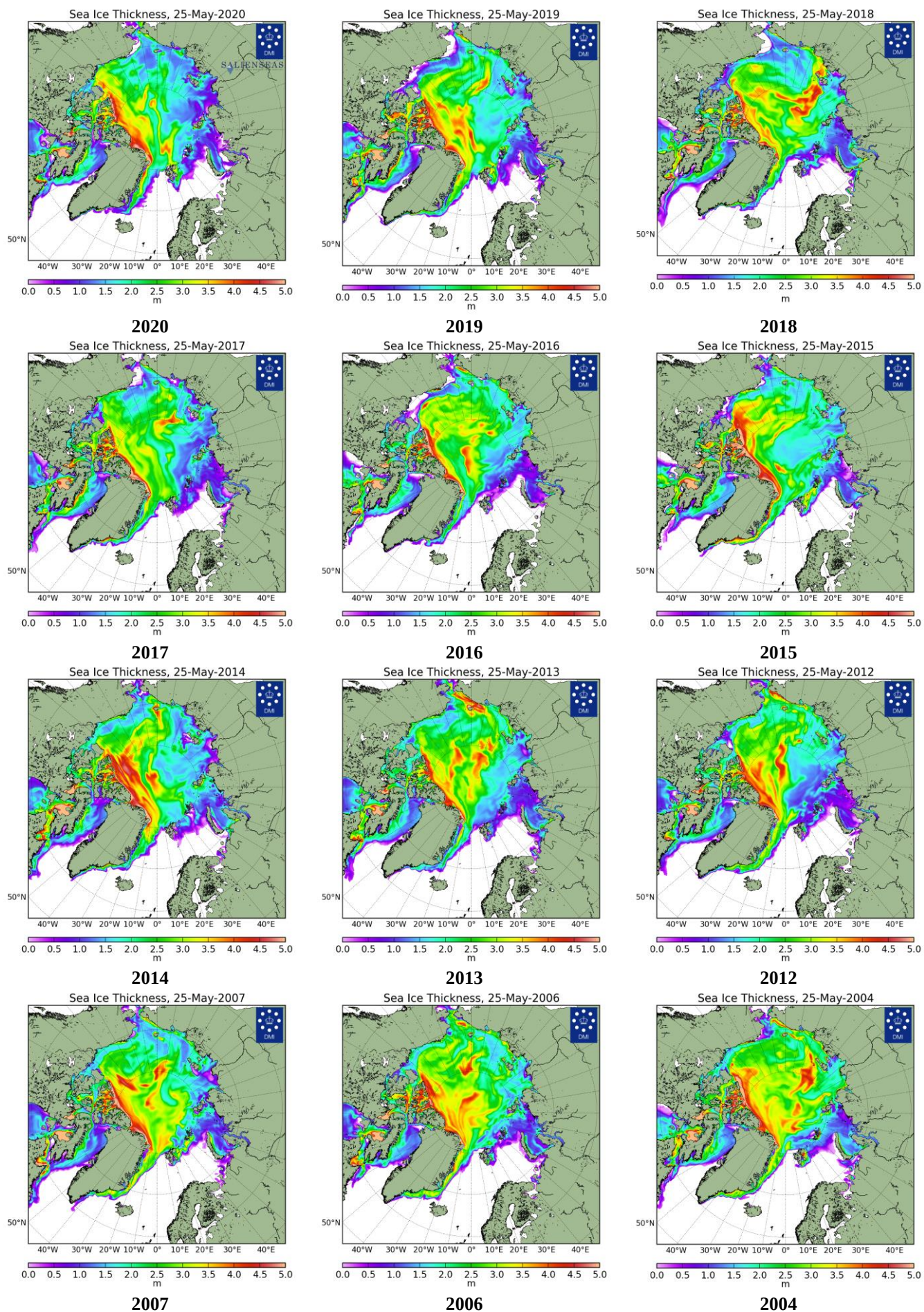
Рисунок 26 – Поля распределения средневзвешенной толщины льда совместной модели морского льда – океана NUCOM/CICE Датского метеорологического института 17.02.2004-25.05.2020 гг.
