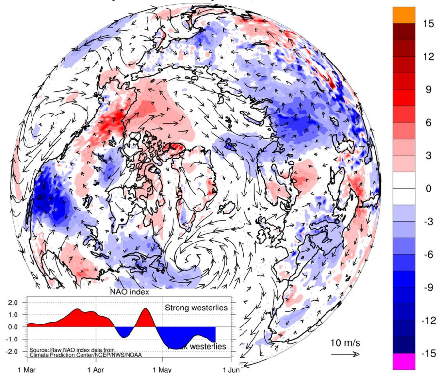
Рисунок 2е – Аномалии приземной температуры воздуха (2м) и осредненные вектора скорости ветра (10 м) за 21.05.-25.05.2020 гг. относительно периода 2004-2013 гг. ( http://polarportal.dk )
