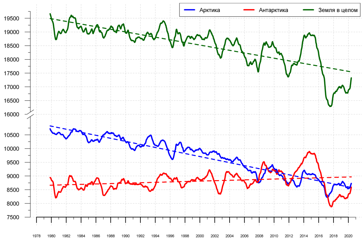
Рисунок 10 – Ежедневные сглаженные окном 365 суток значения ледовитости (площади распространения морского льда) Арктики, Антарктики и Земли в целом с 26.10.1978 по 24.05.2020 на основе SSMR-SSM/I-SSMIS
