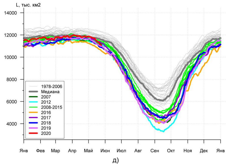
Рисунок 3а – Ежедневные оценки сезонного хода ледовитости для Северной Полярной Области и трех меридиональных секторов за период 26.10.1978 – 24.05.2020 по годам на основе расчетов по данным SSMR-SSM/I-SSMIS, алгоритмы NASATEAM: а) Северная полярная область, б) сектор 45°W-95°E (Гренландское – Карское моря), в) сектор 95°E-170°W (моря Лаптевых – Чукотское и Берингово, Охотское), г) сектор 170°W-45°W (море Бофорта и Канадская Арктика), д) Северный Ледовитый океан, е) Северный морской путь (Карское - Чукотское моря).
