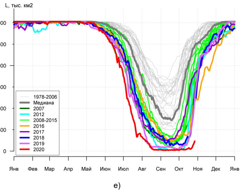
Рисунок 3а – Ежедневные оценки сезонного хода ледовитости для Северной Полярной Области и трех меридиональных секторов за период 26.10.1978 –25.10.2020 по годам на основе расчетов по данным SSMR-SSM/I-SSMIS, алгоритмы NASATEAM: а) Северная полярная область, б) сектор 45°W-95°E (Гренландское – Карское моря), в) сектор 95°E-170°W (моря Лаптевых – Чукотское и Берингово, Охотское), г) сектор 170°W-45°W (море Бофорта и Канадская Арктика), д) Северный Ледовитый океан, е) Северный морской путь (Карское - Чукотское моря).
