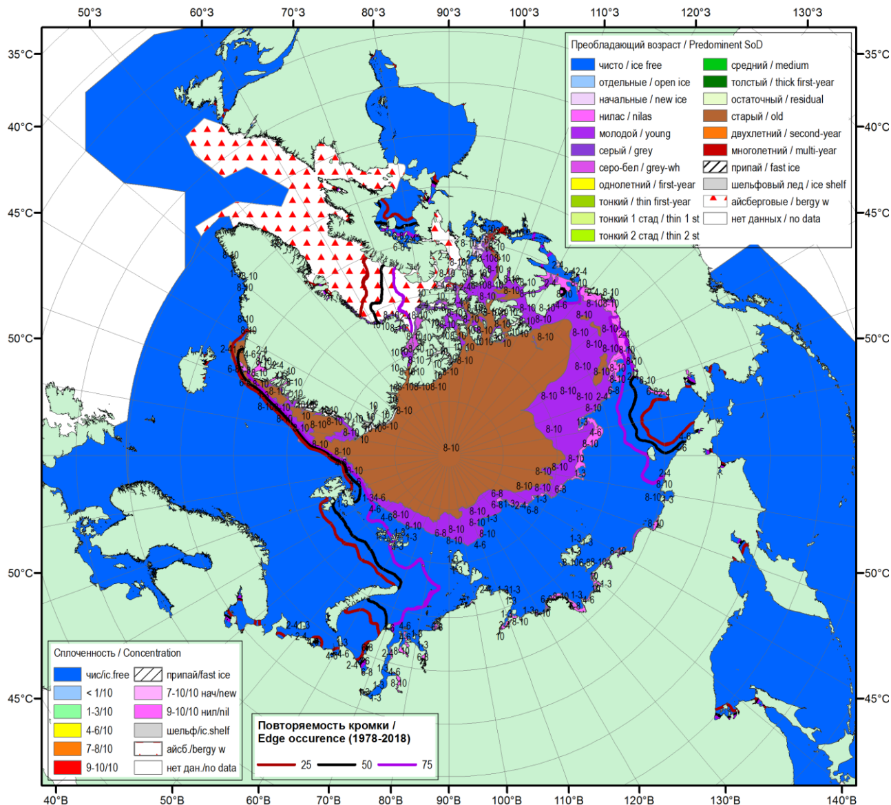
Рисунок 16 – Обзорная ледовая карта СЛО за 22.10.2020-27.10.2020 г. (цветовая раскраска по преобладающему возрасту) на основе ледового анализа ААНИИ (27.10), Национального ледового центра США (22.10) и повторяемость кромки за 26-31.10 за период 1979-2018 гг. по наблюдениям SSMR-SSM/I-SSMIS (алгоритм NASATEAM).
