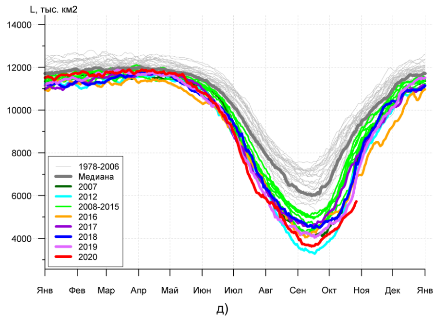
Рисунок 3а – Ежедневные оценки сезонного хода ледовитости для Северной Полярной Области и трех меридиональных секторов за период 26.10.1978 –25.10.2020 по годам на основе расчетов по данным SSMR-SSM/I-SSMIS, алгоритмы NASATEAM: а) Северная полярная область, б) сектор 45°W-95°E (Гренландское – Карское моря), в) сектор 95°E-170°W (моря Лаптевых – Чукотское и Берингово, Охотское), г) сектор 170°W-45°W (море Бофорта и Канадская Арктика), д) Северный Ледовитый океан, е) Северный морской путь (Карское - Чукотское моря).
