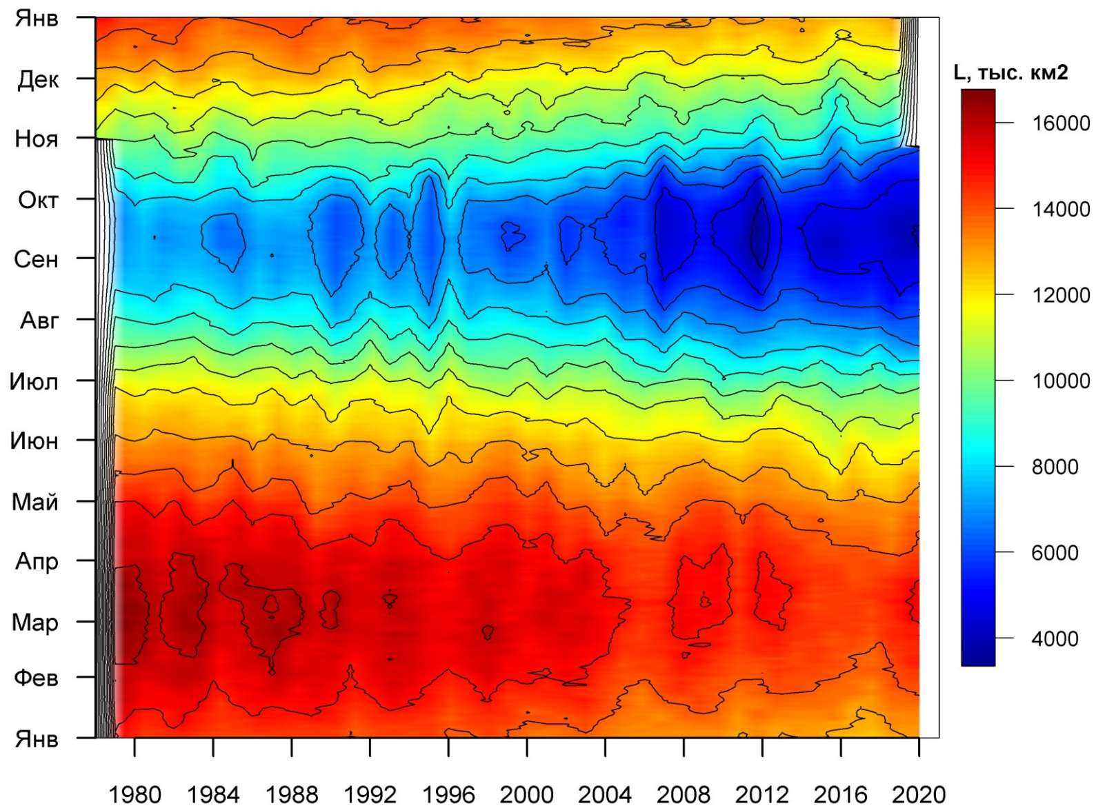
Рисунок 3б – Ежедневные оценки сезонных изменений ледовитости для Северной Полярной Области за период 26.10.1978 – 25.10.2020 на основе расчетов по данным SSMR-SSM/I-SSMIS, алгоритм NASATEAM.
