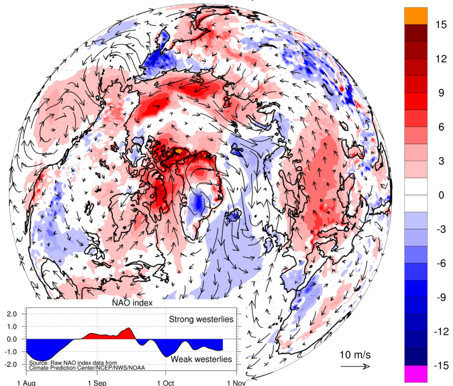
Рисунок 2е – Аномалии приземной температуры воздуха (2м) и осредненные вектора скорости ветра (10 м) за 22.10-26.10.2020 гг. относительно периода 2004-2013 гг. ( http://polarportal.dk )
