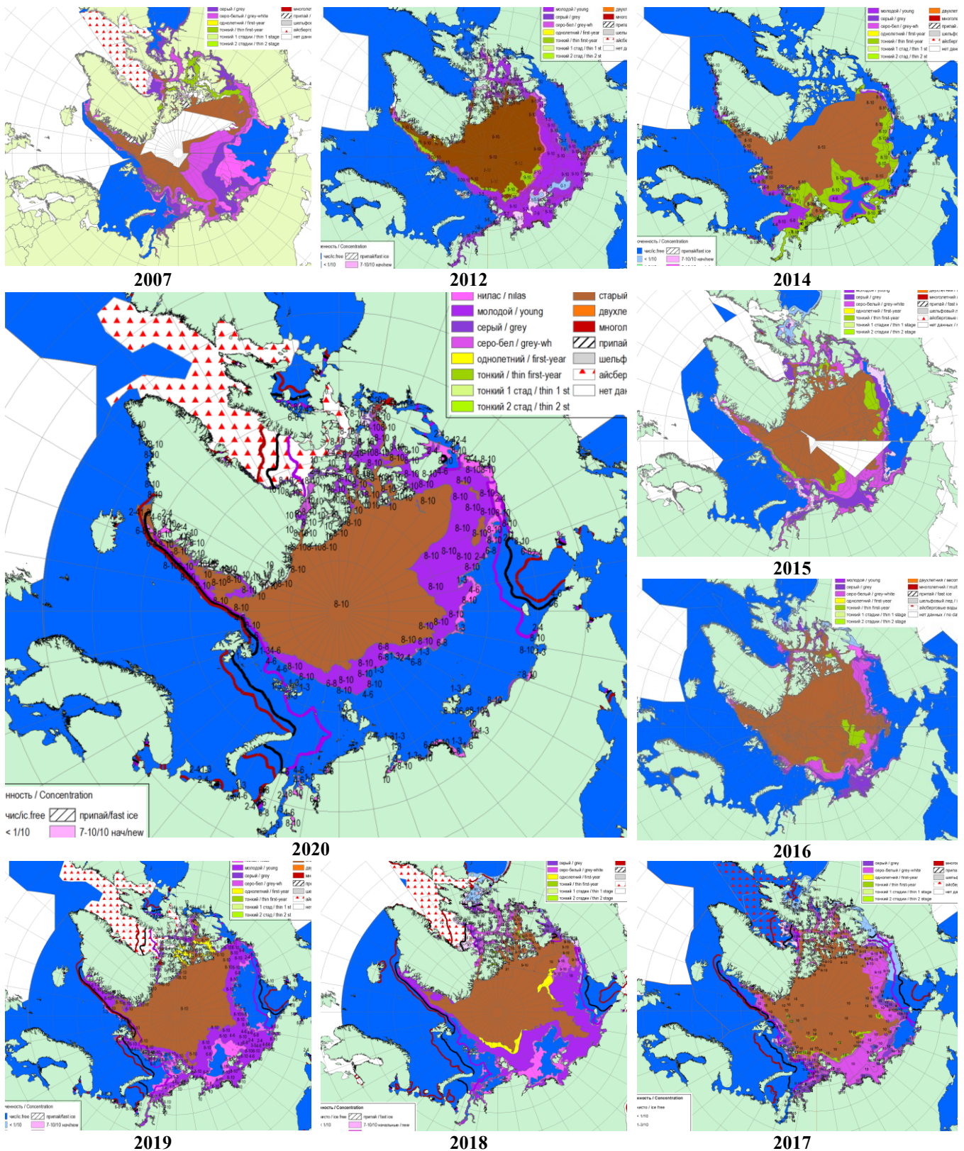
Рисунок 2а – Обзорная ледовая карта СЮ за 22.10 – 27.10.2020 г. и аналогичные периоды 2007–2019 гг. на основе ледового анализа ААНИИ, НИЦ Планета, Канадской ледовой службы и Национального ледового центра США.
