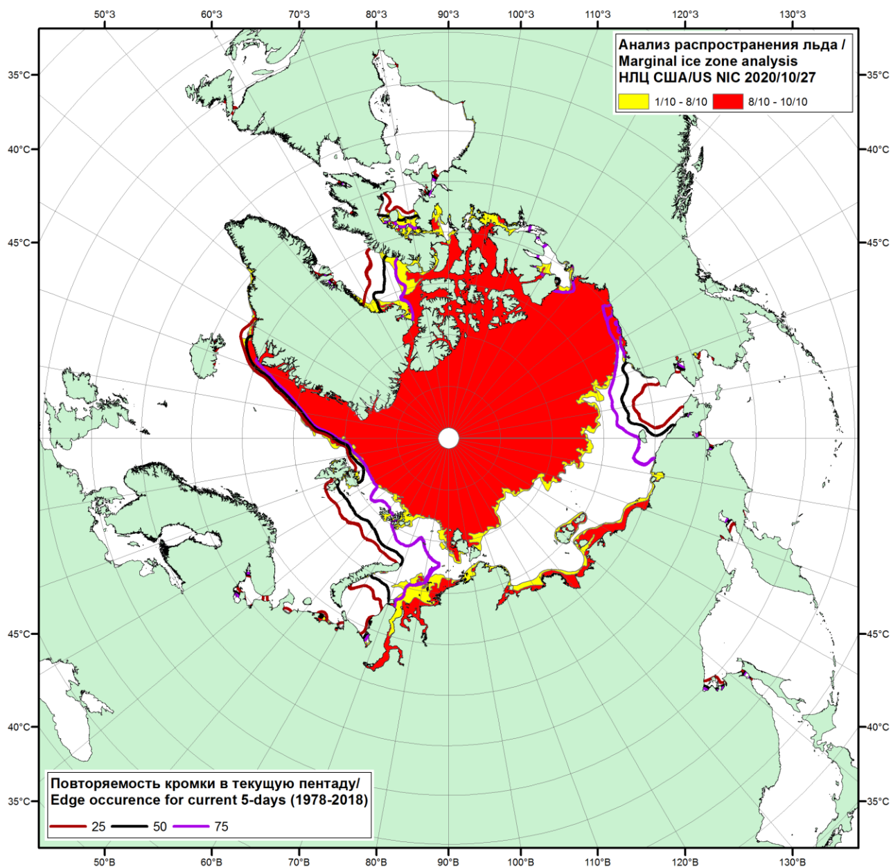
Рисунок 1в – Положение кромки льда и зон разреженных ( <8/10 ) и сплоченных ( \geq 8/10 ) льдов СЛО за 27.10.2020 г. на основе ледового анализа Национального Ледового Центра США и повторяемость кромки за 26-31.10 за период 1979-2018 гг. по наблюдениям SSMR-SSM/I-SSMIS (алгоритм NASATEAM)
