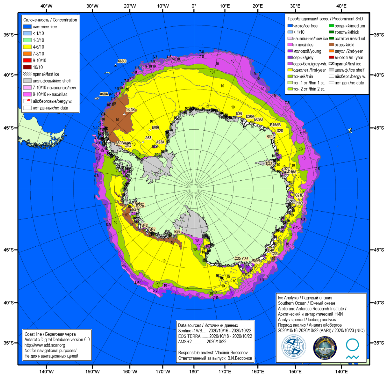
Рисунок 5б – Ледовая карта Южного океана (цветовая окраска по возрасту) и расположение крупных айсбергов на основе информации совместного ледового анализа НЛЦ США, ААНИИ и НМИ (Норвегия) за 22.10.2020.
