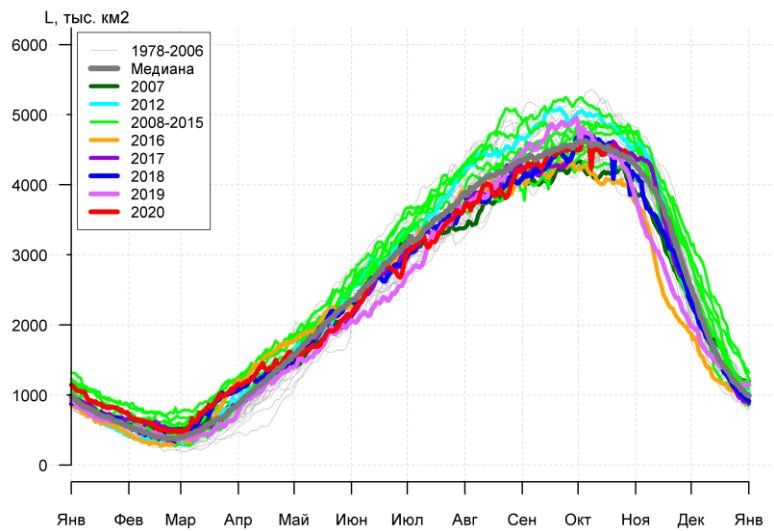
Рисунок 7а – Ежедневные оценки сезонного хода ледовитости Южного Океана и меридиональных секторов за период 26.10.1978 – 25.10.2020 по годам на основе расчетов по данным SSMR-SSM/I-SSMIS, алгоритм NASATEAM: а) Южный Океан, б) Атлантический сектор (60°W-30°E, море Уэдделла), в) Индоокеанский сектор (30°E-150°E, моря Космонавтов, Содружества, Моусона), г) Тихоокеанский сектор (150°E-60°W, моря Росса, Беллинсгаузена)
