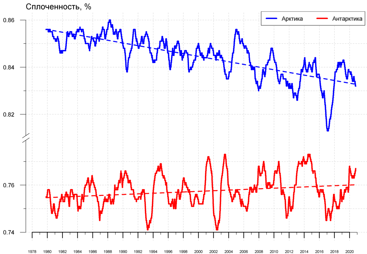
Рисунок 11 – Ежедневные сглаженные окном 365 суток значения средней общей сплоченности Арктики и Антарктики с 26.10.1978 по 25.10.2020 на основе SSMR-SSM/I-SSMIS
