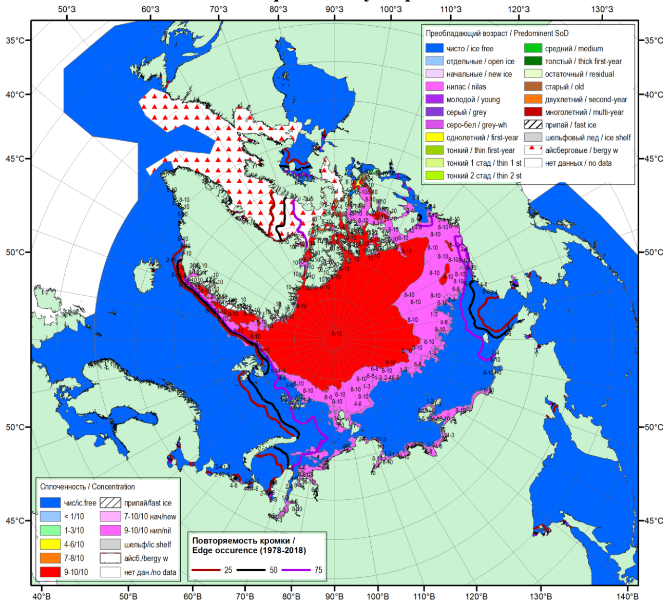
Рисунок 1а – Обзорная ледовая карта СЛО за 22.10.2020-27.10.2020 г. (цветовая раскраска по общей сплоченности) на основе ледового анализа ААНИИ (27.10), Национального ледового центра США (22.10) и повторяемость кромки за 26-31.10 за период 1979-2018 гг. по наблюдениям SSMR-SSM/I-SSMIS (алгоритм NASATEAM).
