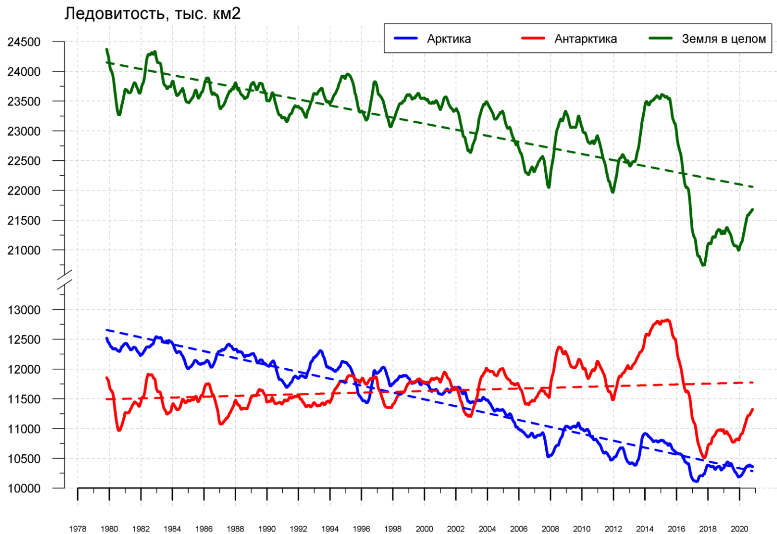
Рисунок 9 – Ежедневные сглаженные окном 365 суток значения приведенной ледовитости (площади морского льда) Арктики, Антарктики и Земли в целом с 26.10.1978 по 25.10.2020 на основе SSMR-SSM/I-SSMIS
