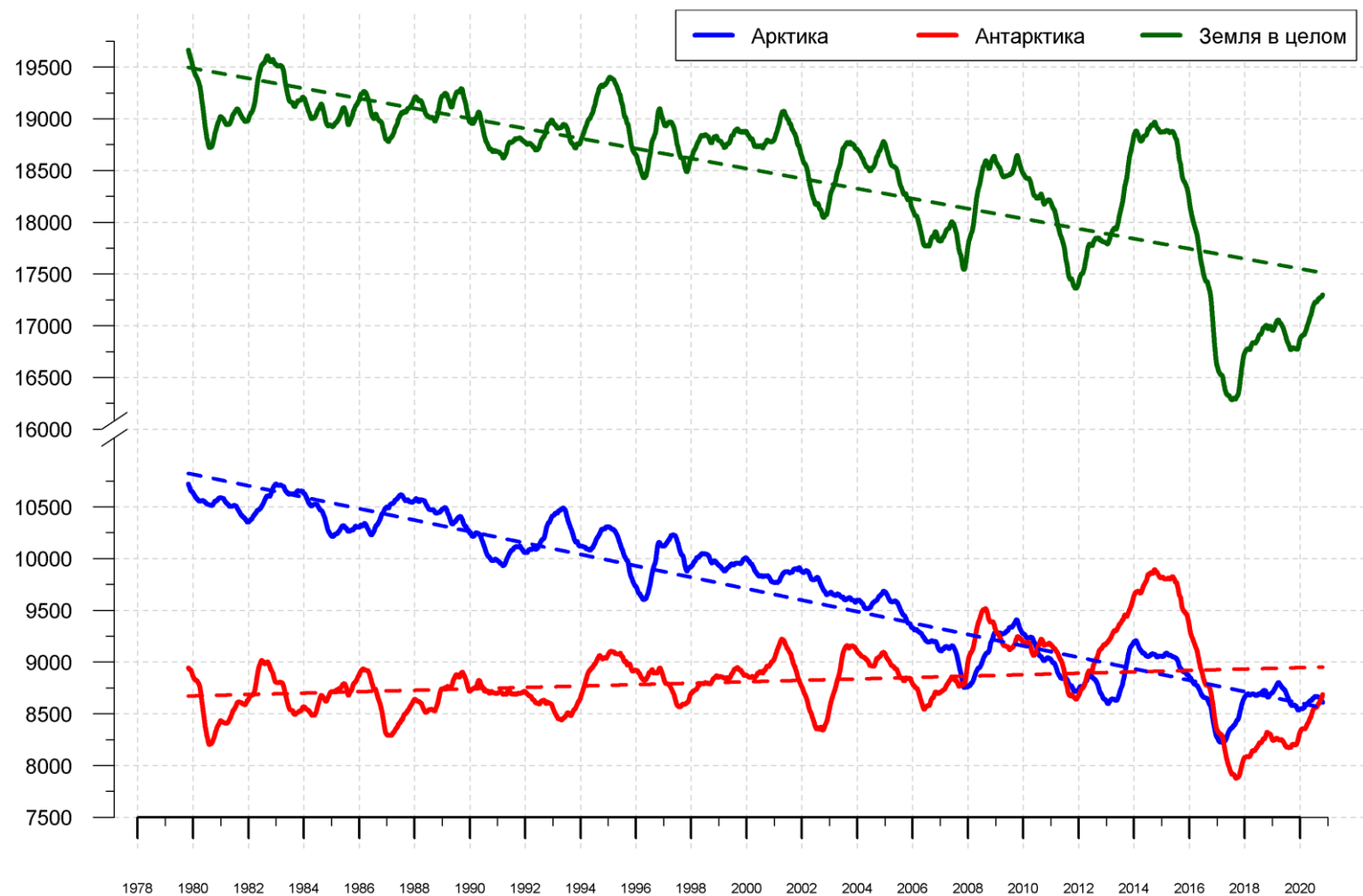
Рисунок 10 – Ежедневные сглаженные окном 365 суток значения ледовитости (площади распространения морского льда) Арктики, Антарктики и Земли в целом с 26.10.1978 по 25.10.2020 на основе SSMR-SSM/I-SSMIS
