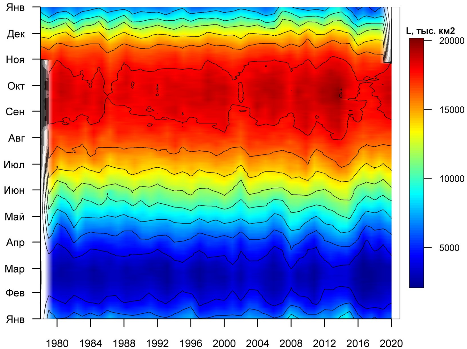
Рисунок 76 – Ежедневные оценки сезонных изменений ледовитости для Южного океана за период 26.10.1978 – 25.10.2020 на основе расчетов по данным SSMR-SSM/I-SSMIS, алгоритм NASATEAM.
