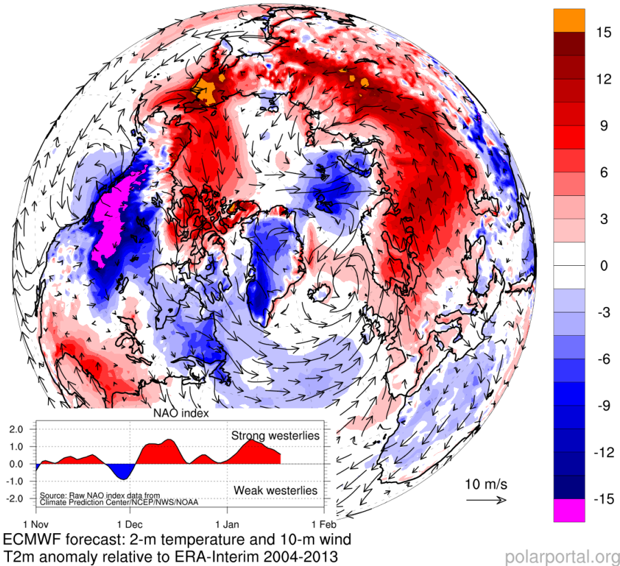
Рисунок 2е – Аномалии приземной температуры воздуха (2м) и осредненные вектора скорости ветра (10 м) за 14.01 -18.01.2021 гг. относительно периода 2004-2013 гг. ( http://polarportal.dk )
