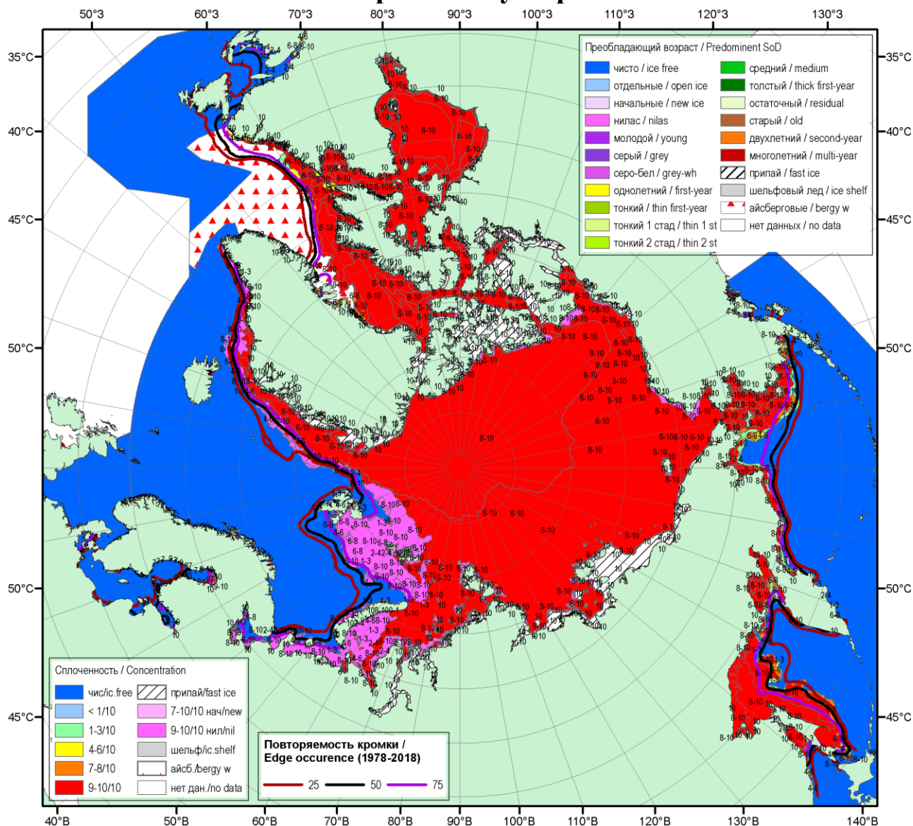
Рисунок 1а – Обзорная ледовая карта СЛЮ за 14.01-19.01.2021 г. (цветовая раскраска по общей сплоченности) на основе ледового анализа ААНИИ (19.01), Национального ледового центра США (14.01) и повторяемость кромки за 16-20.01 за период 1979-2018 гг. по наблюдениям SSMR-SSM/I-SSMIS (алгоритм NASATEAM).
