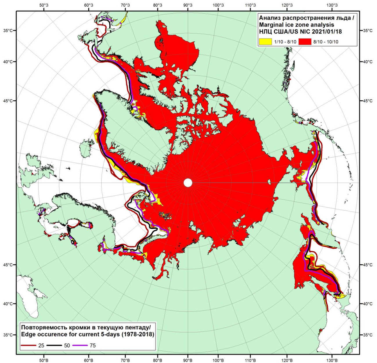
Рисунок 1в – Положение кромки льда и зон разреженных ( <8/10 ) и сплоченных ( \geq 8/10 ) льдов СЛО за 18.01.2021 г. на основе ледового анализа Национального Ледового Центра США и повторяемость кромки за 16-20.01 за период 1979-2018 гг. по наблюдениям SSMR-SSM/I-SSMIS (алгоритм NASATEAM)
