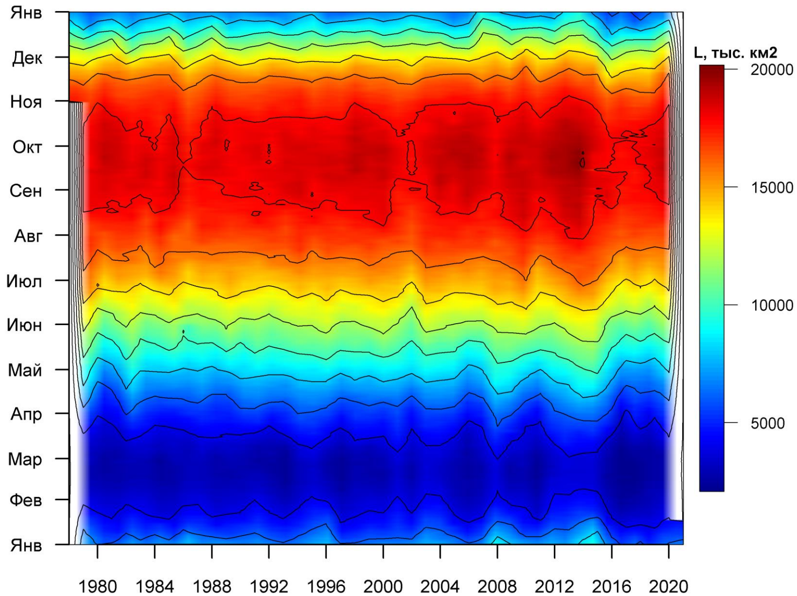
Рисунок 76 – Ежедневные оценки сезонных изменений ледовитости для Южного океана за период 26.10.1978 – 17.01.2021 на основе расчетов по данным SSMR-SSM/I-SSMIS, алгоритм NASATEAM.
