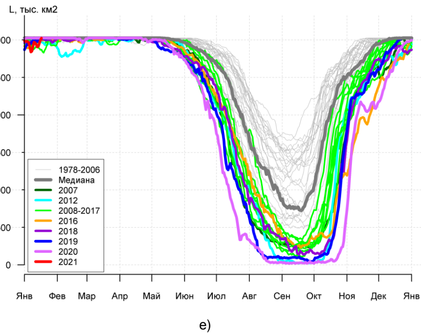
Рисунок 3а – Ежедневные оценки сезонного хода ледовитости для Северной Полярной Области и трех меридиональных секторов за период 26.10.1978 - 17.01.2021 по годам на основе расчетов по данным SSMR-SSM/I-SSMIS, алгоритмы NASATEAM: а) Северная полярная область, б) сектор 45°W-95°E (Гренландское – Карское моря), в) сектор 95°E-170°W (моря Лаптевых – Чукотское и Берингово, Охотское), г) сектор 170°W-45°W (море Бофорта и Канадская Арктика), д) Северный Ледовитый океан, е) Северный морской путь (Карское - Чукотское моря).
