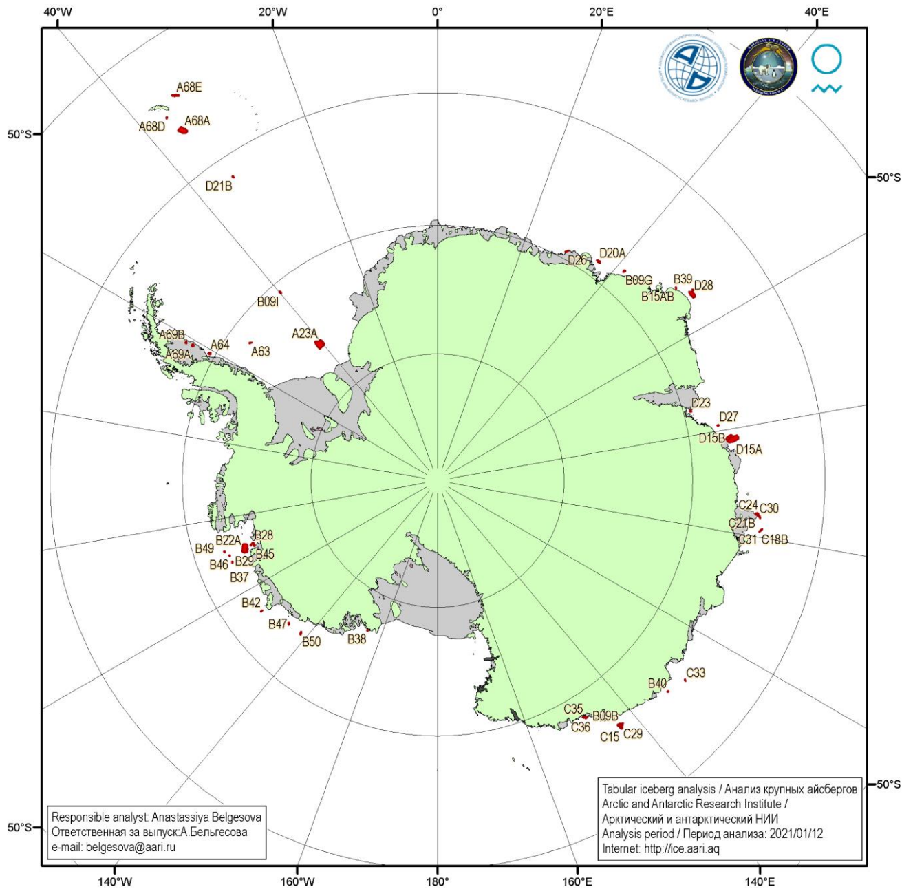
Рисунок 5д – Анализ ААНИИ крупных айсбергов Южного океана за 12.01.2021.
