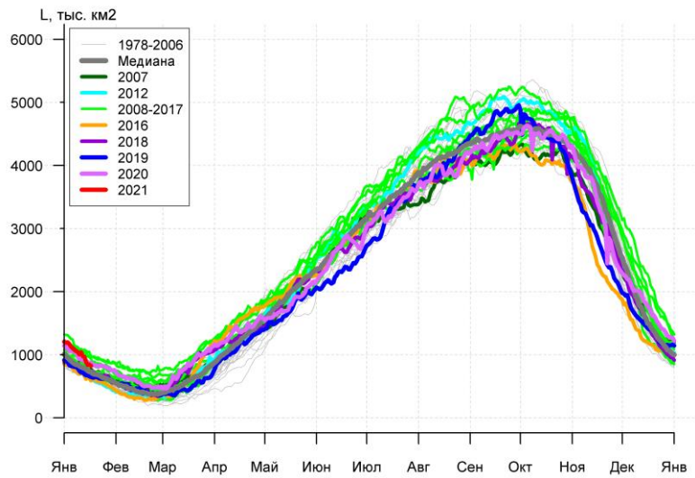
Рисунок 7а – Ежедневные оценки сезонного хода ледовитости Южного Океана и меридиональных секторов за период 26.10.1978 – 17.01.2021 по годам на основе расчетов по данным SSMR-SSM/I-SSMIS, алгоритм NASATEAM: а) Южный Океан, б) Атлантический сектор (60°W-30°E, море Уэдделла), в) Индоокеанский сектор (30°E-150°E, моря Космонавтов, Содружества, Моусона), г) Тихоокеанский сектор (150°E-60°W, моря Росса, Беллингаузена)
