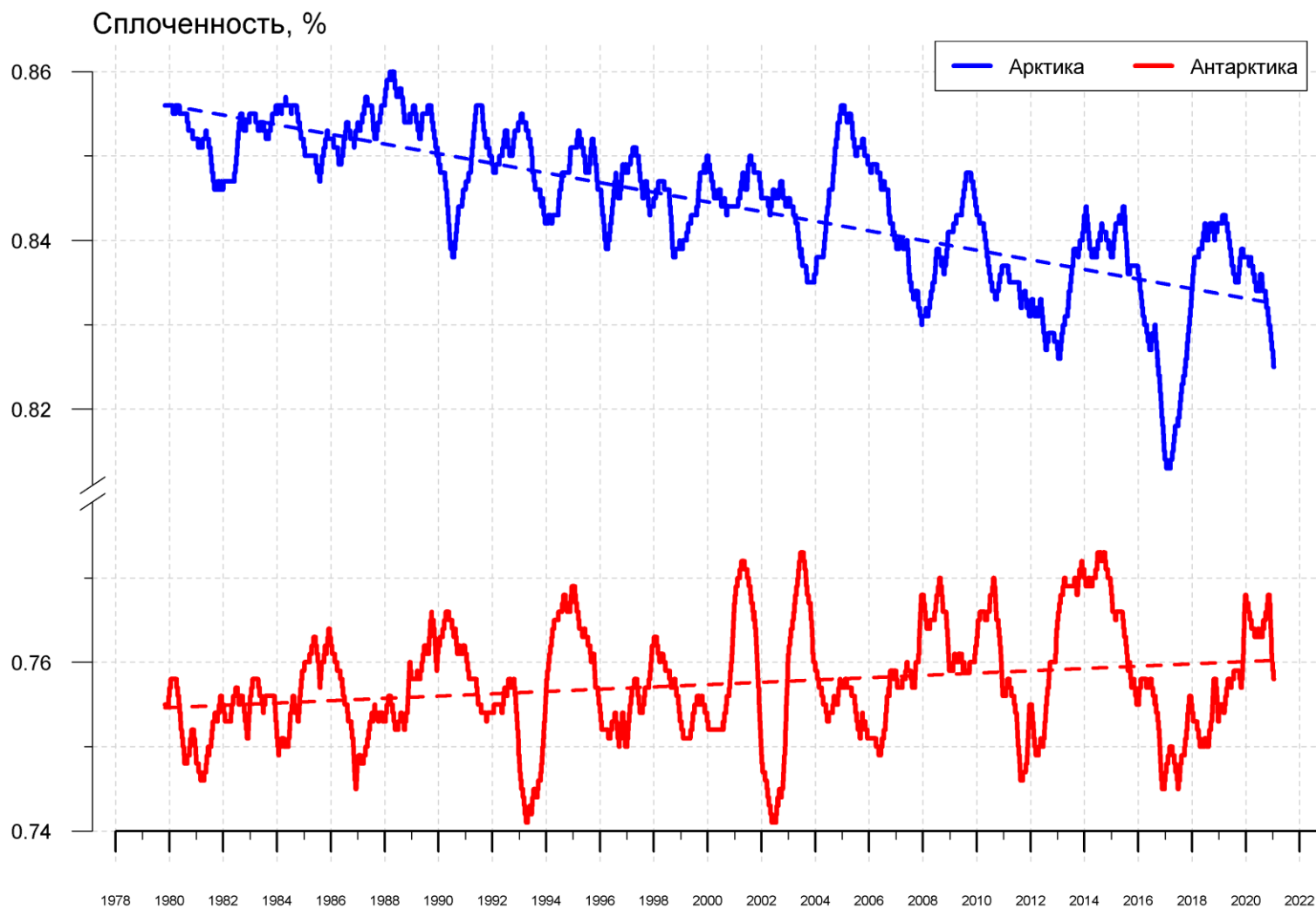
Рисунок 11 – Ежедневные сглаженные окном 365 суток значения средней общей сплоченности Арктики и Антарктики с 26.10.1978 по 17.01.2021 на основе SSMR-SSM/I-SSMIS
