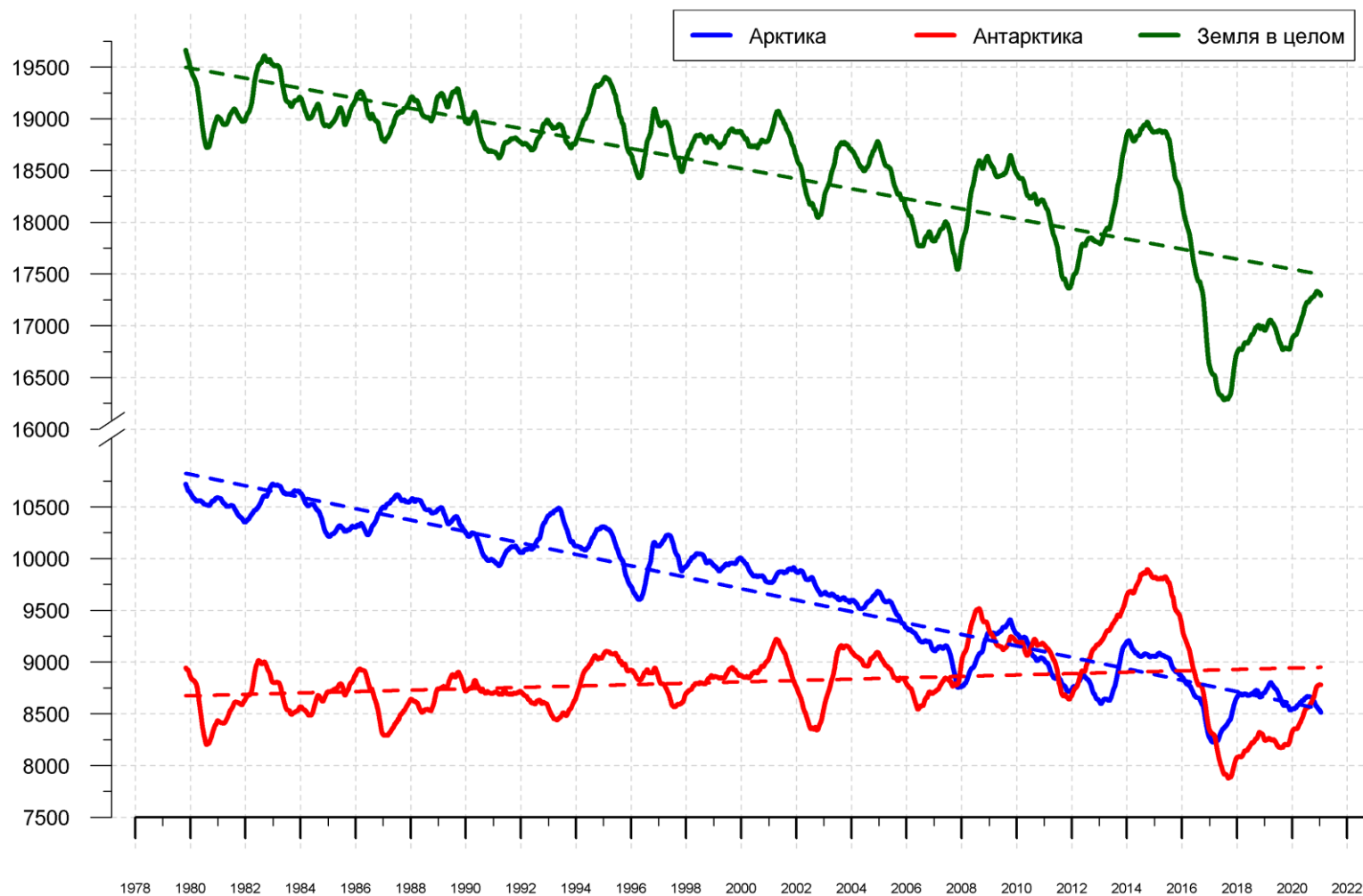
Рисунок 10 – Ежедневные сглаженные окном 365 суток значения ледовитости (площади распространения морского льда) Арктики, Антарктики и Земли в целом с 26.10.1978 по 17.01.2021 на основе SSMR-SSM/I-SSMIS
