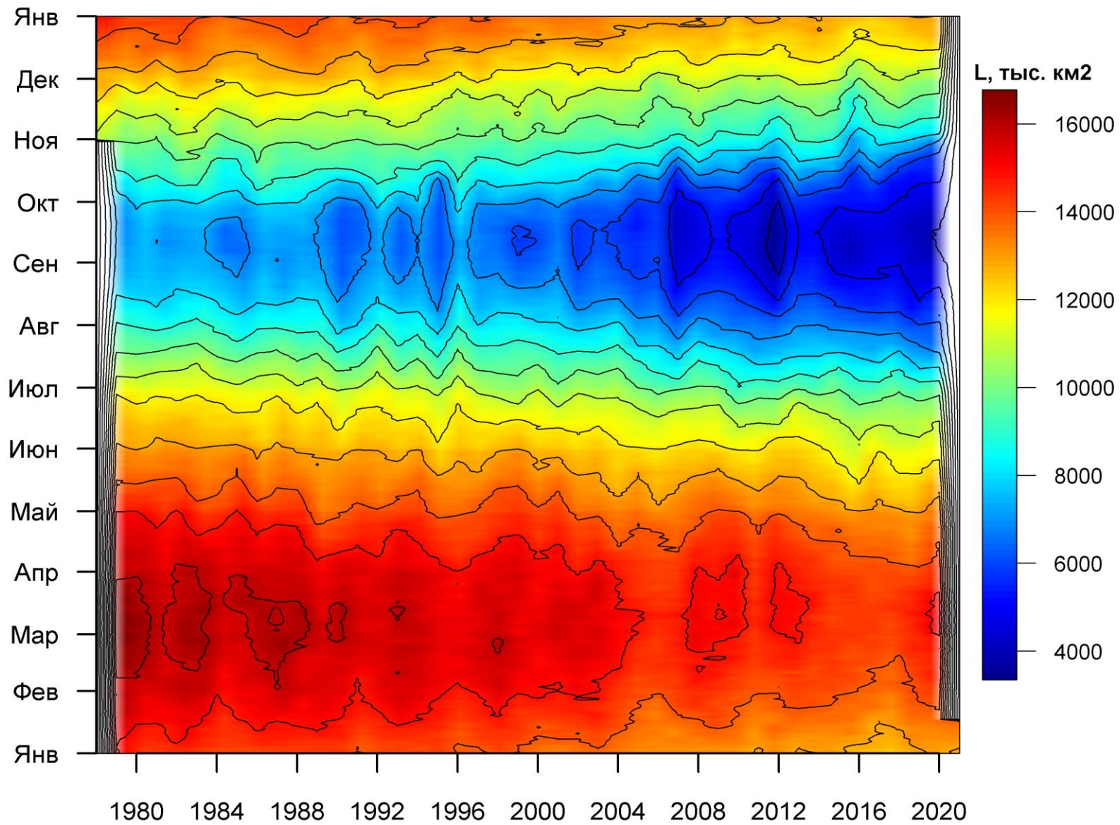
Рисунок 3б – Ежедневные оценки сезонных изменений ледовитости для Северной Полярной Области за период 26.10.1978 – 17.01.2021 на основе расчетов по данным SSMR-SSM/I-SSMIS, алгоритм NASATEAM.
