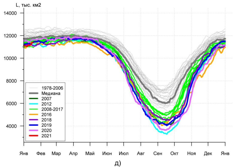
Рисунок 3а – Ежедневные оценки сезонного хода ледовитости для Северной Полярной Области и трех меридиональных секторов за период 26.10.1978 - 17.01.2021 по годам на основе расчетов по данным SSMR-SSM/I-SSMIS, алгоритмы NASATEAM: а) Северная полярная область, б) сектор 45°W-95°E (Гренландское – Карское моря), в) сектор 95°E-170°W (моря Лаптевых – Чукотское и Берингово, Охотское), г) сектор 170°W-45°W (море Бофорта и Канадская Арктика), д) Северный Ледовитый океан, е) Северный морской путь (Карское - Чукотское моря).
