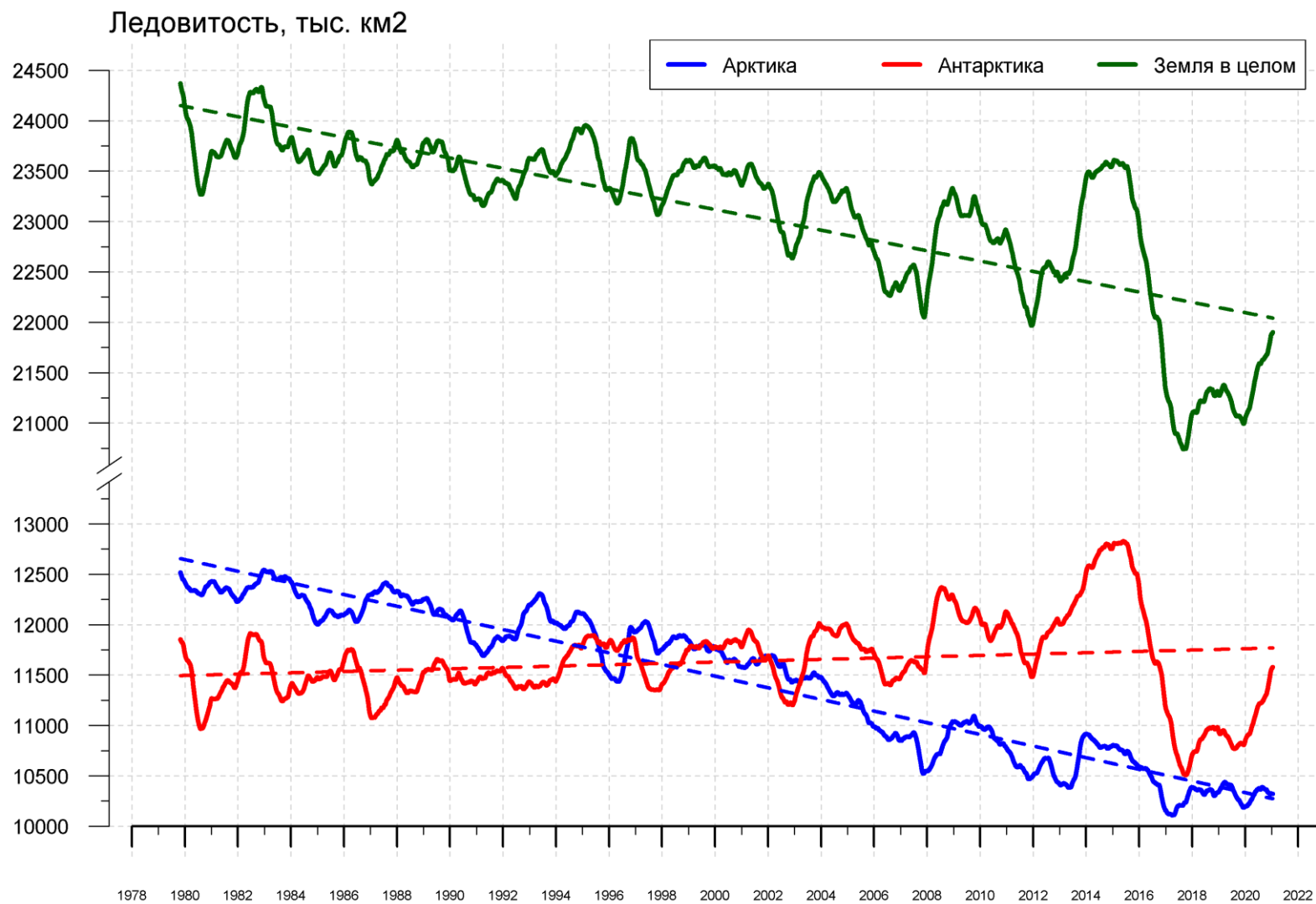
Рисунок 9 – Ежедневные сглаженные окном 365 суток значения приведенной ледовитости (площади морского льда) Арктики, Антарктики и Земли в целом с 26.10.1978 по 17.01.2021 на основе SSMR-SSM/I-SSMIS
