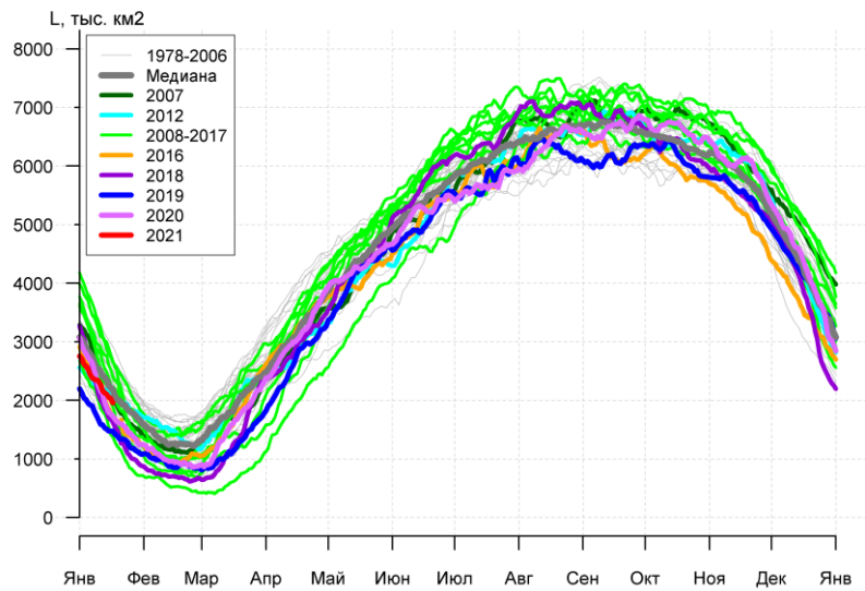
Рисунок 7а – Ежедневные оценки сезонного хода ледовитости Южного Океана и меридиональных секторов за период 26.10.1978 – 17.01.2021 по годам на основе расчетов по данным SSMR-SSM/I-SSMIS, алгоритм NASATEAM: а) Южный Океан, б) Атлантический сектор (60°W-30°E, море Уэдделла), в) Индоокеанский сектор (30°E-150°E, моря Космонавтов, Содружества, Моусона), г) Тихоокеанский сектор (150°E-60°W, моря Росса, Беллингаузена)
