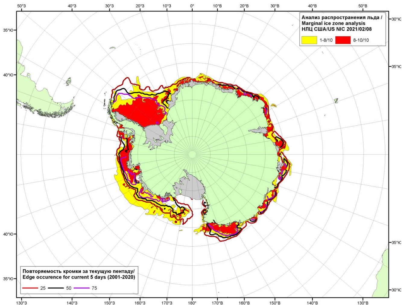
Рисунок 5в – Положение кромки льда и зон разреженных ( <8/10 ) и сплоченных ( \geq 8/10 ) льдов Южного океана за 08.02.2021 г. на основе ледового анализа Национального Ледового Центра США и повторяемость кромки за 06-10.02 за период 2001-2020 гг. по наблюдениям SSMR-SSM/I-SSMIS (алгоритм NASATEAM).
