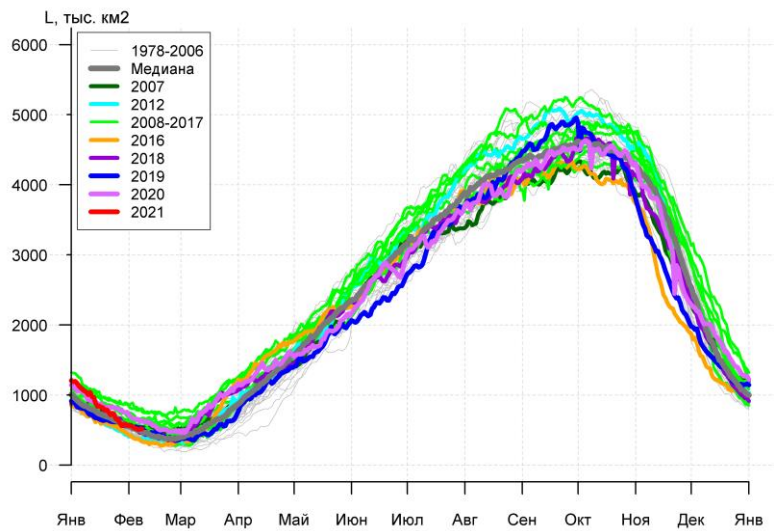
Рисунок 7а – Ежедневные оценки сезонного хода ледовитости Южного Океана и меридиональных секторов за период 26.10.1978 – 07.02.2021 по годам на основе расчетов по данным SSMR-SSM/I-SSMIS, алгоритм NASATEAM: а) Южный Океан, б) Атлантический сектор (60°W-30°E, море Уэдделла), в) Индоокеанский сектор (30°E-150°E, моря Космонавтов, Содружества, Моусона), г) Тихоокеанский сектор (150°E-60°W, моря Росса, Беллинсгаузена)
