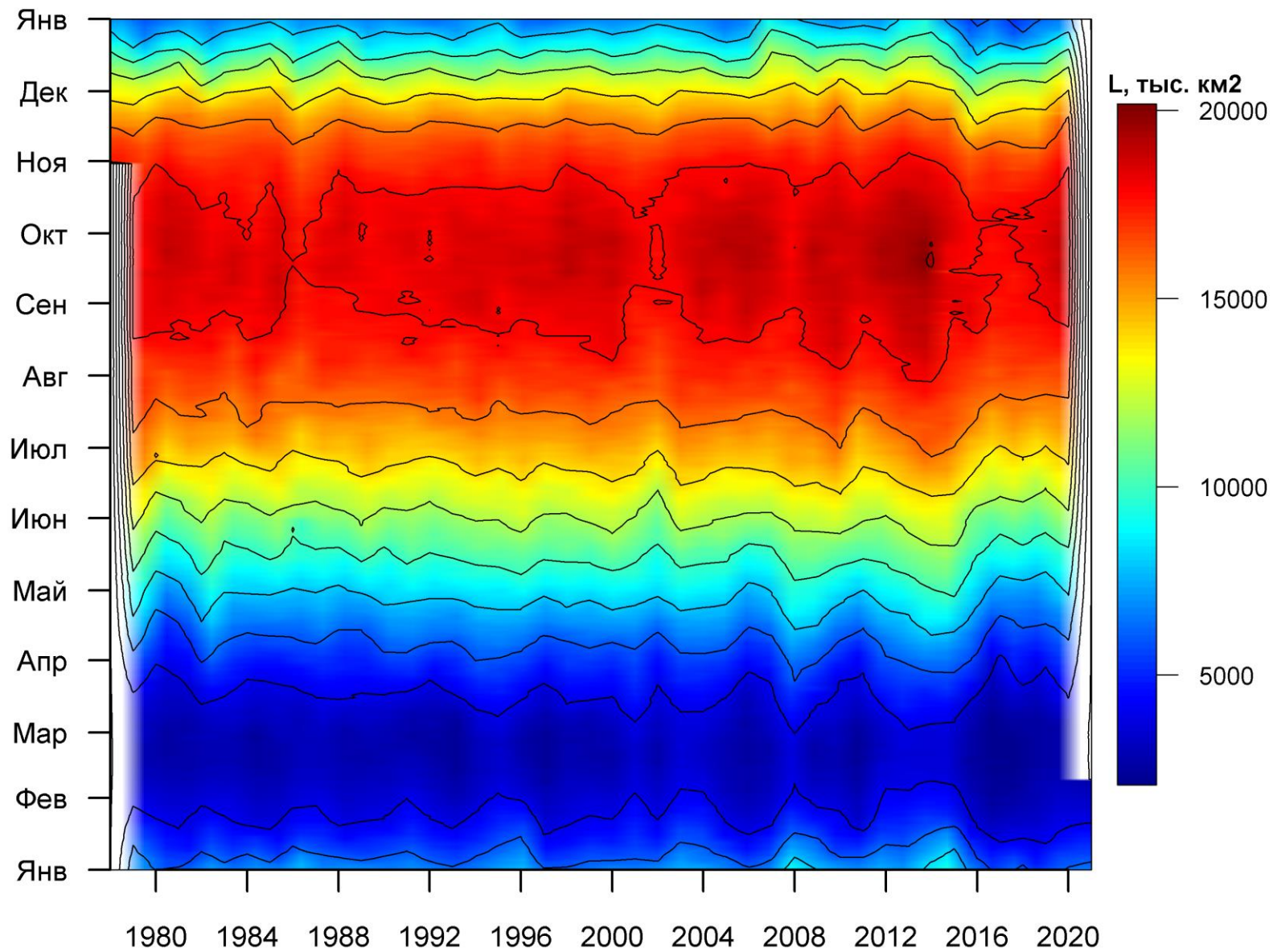
Рисунок 76 – Ежедневные оценки сезонных изменений ледовитости для Южного океана за период 26.10.1978 – 07.02.2021 на основе расчетов по данным SSMR-SSM/I-SSMIS, алгоритм NASATEAM.
