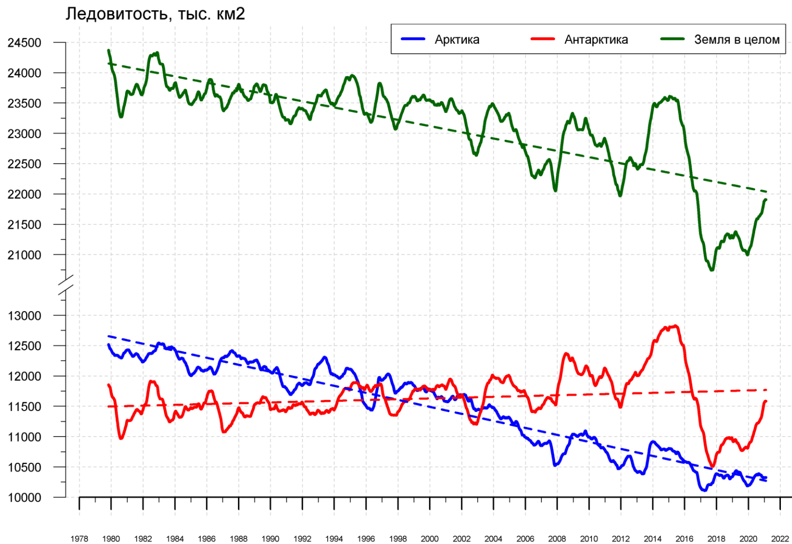
Рисунок 9 – Ежедневные сглаженные окном 365 суток значения ледовитости (площади распространения морского льда) Арктики, Антарктики и Земли в целом с 26.10.1978 по 07.02.2021 на основе SSMR-SSM/I-SSMIS
