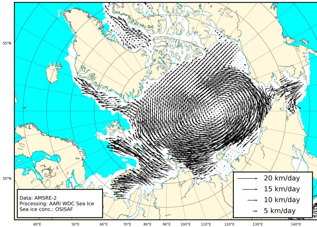
Рисунок 2г – Поле дрейфа морского льда Арктики за 01.02-08.02.2021 г., источник данных EUMETSAT OSISAF.
