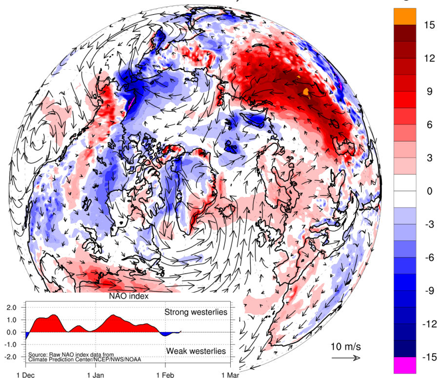
Рисунок 2е – Аномалии приземной температуры воздуха (2м) и осредненные вектора скорости ветра (10 м) за 04.02 -08.02.2021 гг. относительно периода 2004-2013 гг. ( http://polarportal.dk )
