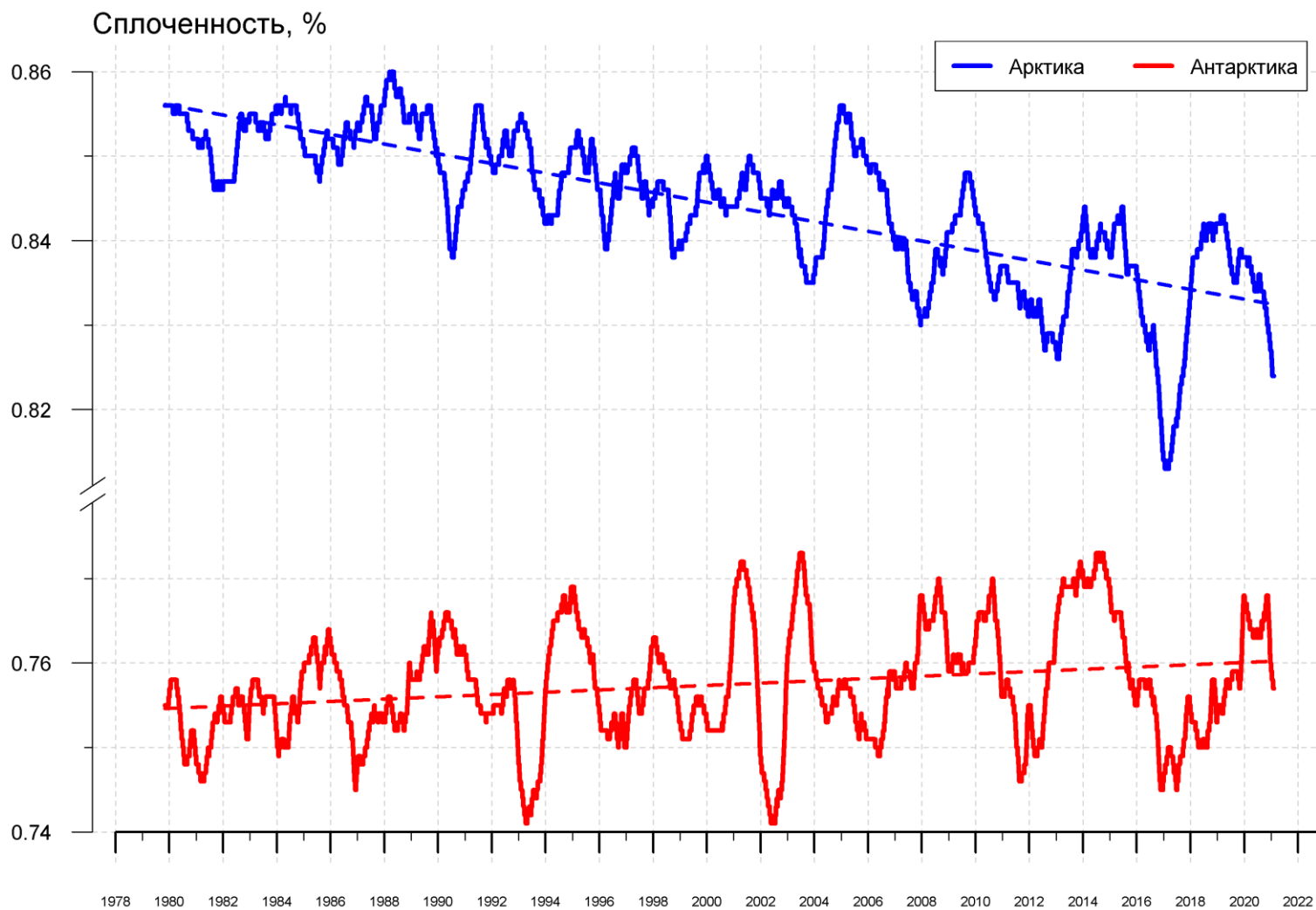
Рисунок 11 – Ежедневные сглаженные окном 365 суток значения средней общей сплоченности Арктики и Антарктики с 26.10.1978 по 07.02.2021 на основе SSMR-SSM/I-SSMIS
