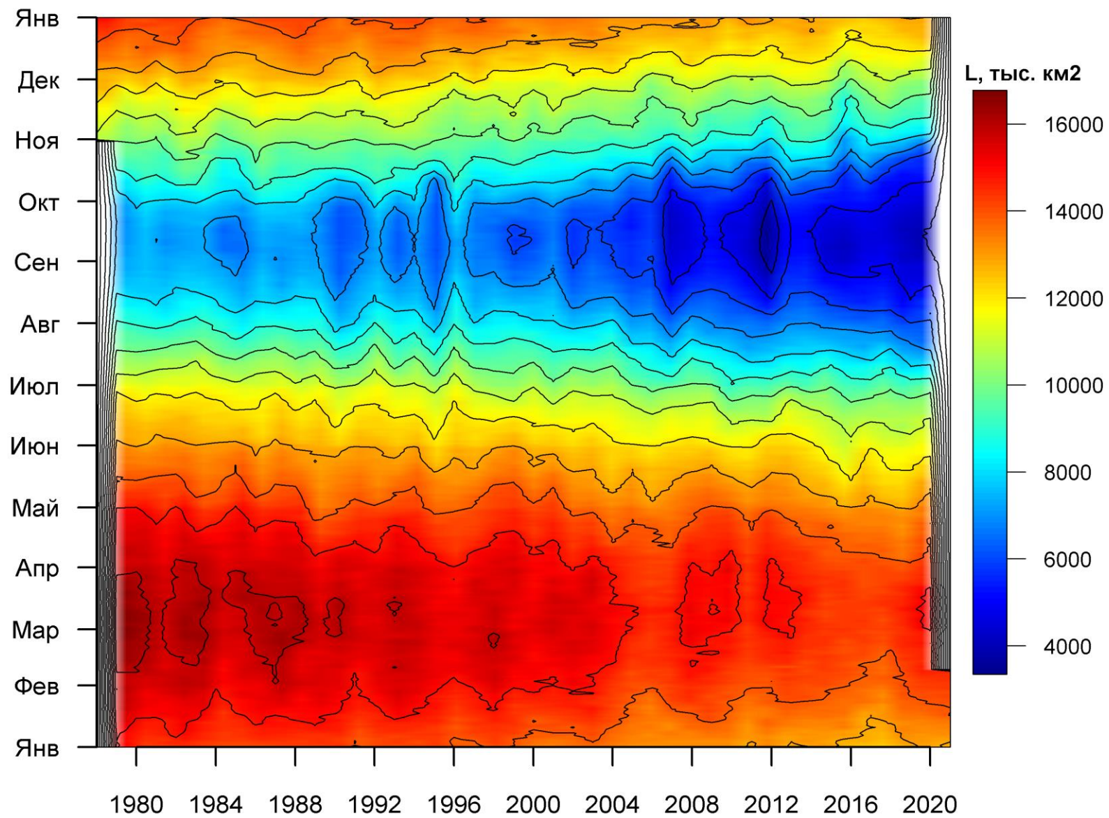
Рисунок 3б – Ежедневные оценки сезонных изменений ледовитости для Северной Полярной Области за период 26.10.1978 – 07.02.2021 на основе расчетов по данным SSMR-SSM/I-SSMIS, алгоритм NASATEAM.
