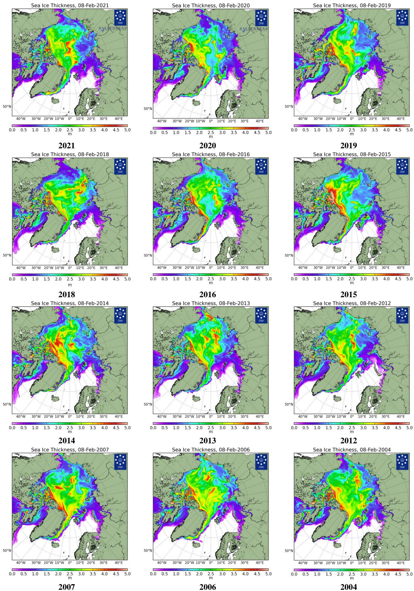
Рисунок 26 – Поля распределения средневзвешенной толщины льда совместной модели морского льда – океана НУСОМ/СИЕ Датского метеорологического института 17.02.2004-08.02.2021 гг.
