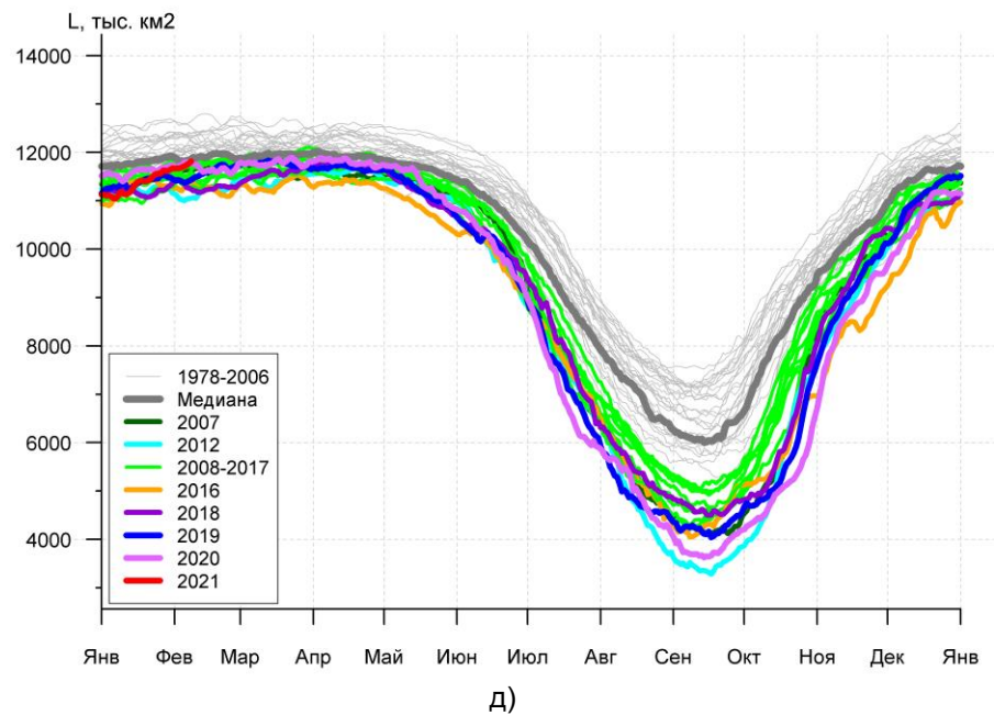
Рисунок 3а – Ежедневные оценки сезонного хода ледовитости для Северной Полярной Области и трех меридиональных секторов за период 26.10.1978 - 07.02.2021 по годам на основе расчетов по данным SSMR-SSM/I-SSMIS, алгоритмы NASATEAM: а) Северная полярная область, б) сектор 45°W-95°E (Гренландское – Карское моря), в) сектор 95°E-170°W (моря Лаптевых – Чукотское и Берингово, Охотское), г) сектор 170°W-45°W (море Бофорта и Канадская Арктика), д) Северный Ледовитый океан, е) Северный морской путь (Карское - Чукотское моря).
