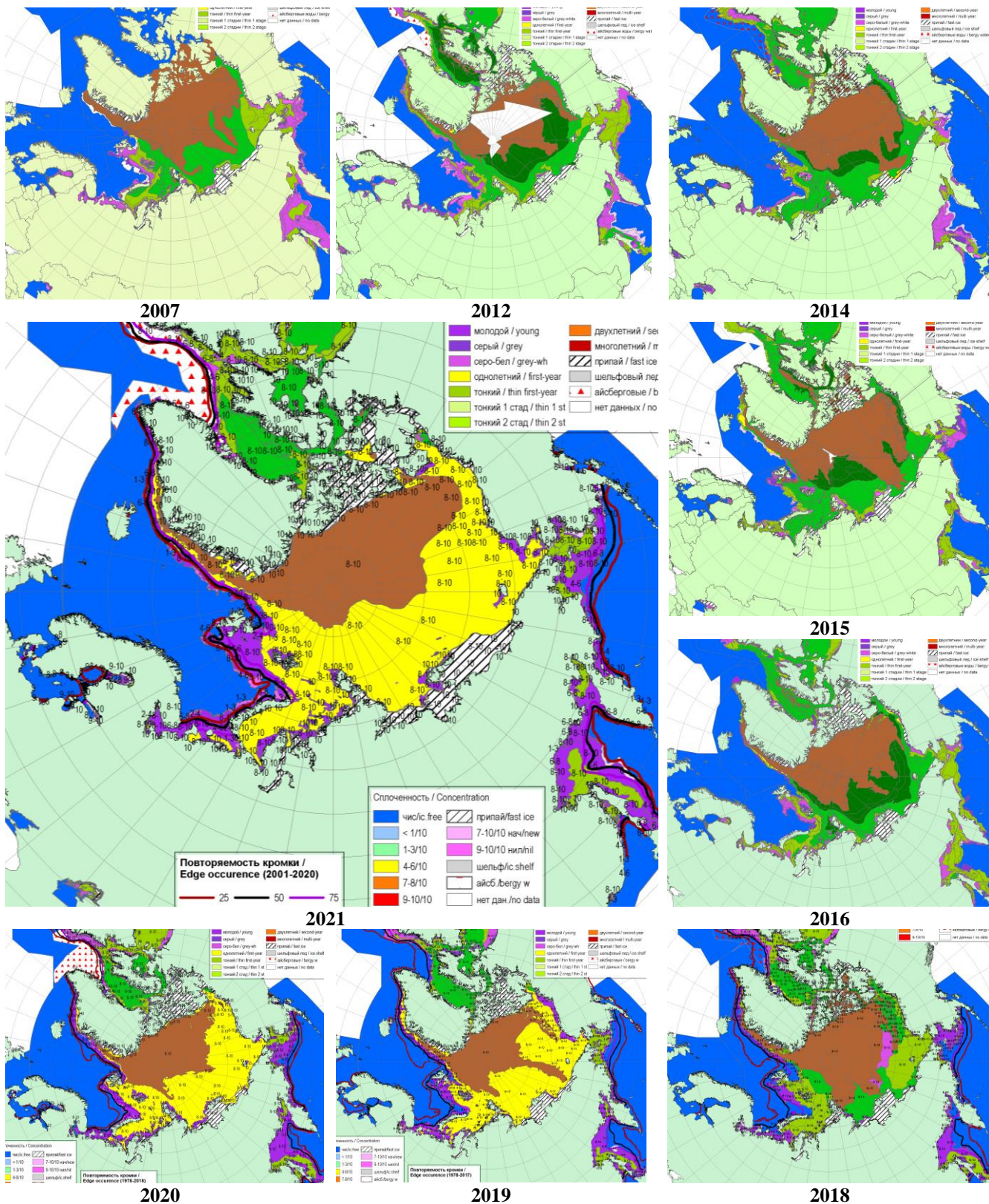
Рисунок 2а – Обзорная ледовая карта САО за 04.02-09.02.2021 г. и аналогичные периоды 2007-2020гг. на основе ледового анализа ААНИИ, НИЦ Планета, Канадской ледовой службы и Национального ледового центра США.
