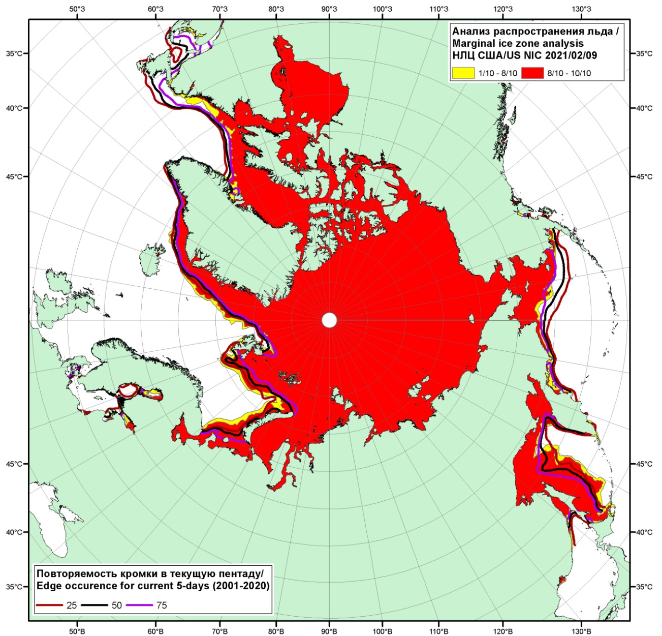
Рисунок 1в – Положение кромки льда и зон разреженных ( <8/10 ) и сплоченных ( \geq 8/10 ) льдов СЛО за 09.02.2021 г. на основе ледового анализа Национального Ледового Центра США и повторяемость кромки за 06-10.02 за период 2001-2020 гг. по наблюдениям SSMR-SSM/I-SSMIS (алгоритм NASATEAM)
