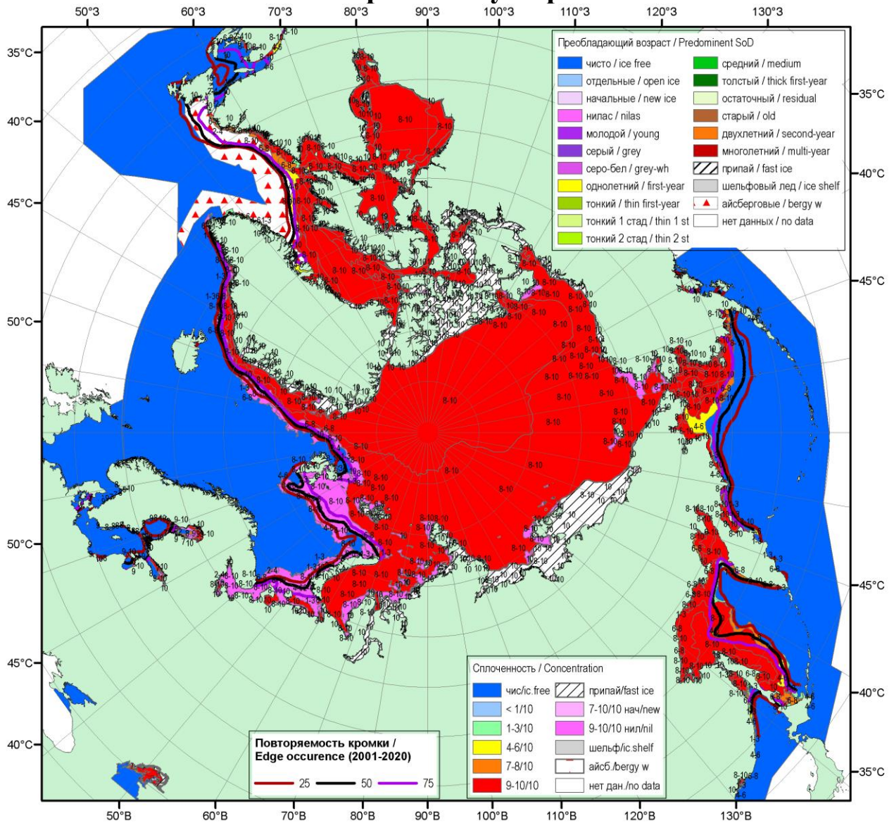
Рисунок 1а – Обзорная ледовая карта СЛЮ за 04.02-09.02.2021 г. (цветовая раскраска по общей сплоченности) на основе ледового анализа ААНИИ (09.02), Национального ледового центра США (04.01) и НИЦ Планета (01-02.02 Каспийское, Азовское моря) и повторяемость кромки за 06-10.02 за период 2001-2020 гг. по наблюдениям SSMR-SSM/I-SSMIS (алгоритм NASATEAM).
