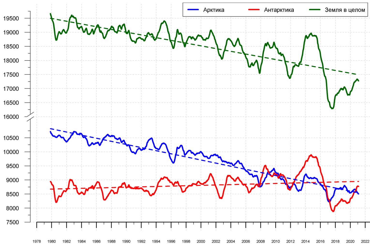
Рисунок 10 – Ежедневные сглаженные окном 365 суток значения приведенной ледовитости (площади морского льда) Арктики, Антарктики и Земли в целом с 26.10.1978 по 07.02.2021 на основе SSMR-SSM/I-SSMIS
