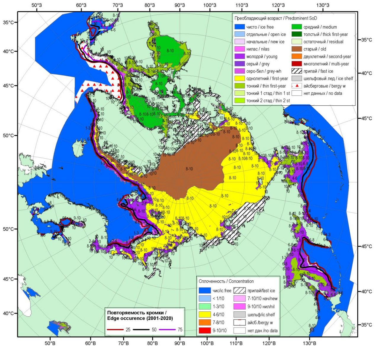
Рисунок 16 – Обзорная ледовая карта СЛО за 28.01-02.02.2021 г. 04.02-09.02.2021 г. (цветовая раскраска по преобладающему возрасту) на основе ледового анализа ААНИИ (09.02), Национального ледового центра США (04.01) и НИЦ Планета (01-02.02 Каспийское, Азовское моря) и повторяемость кромки за 06-10.02 за период 2001-2020 гг. по наблюдениям SSMR-SSM/I-SSMIS (алгоритм NASATEAM).
