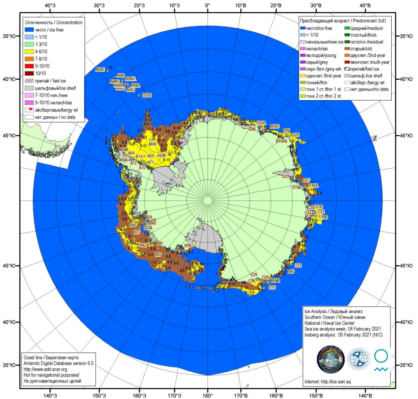
Рисунок 5б – Ледовая карта Южного океана (цветовая окраска по возрасту) и расположение крупных айсбергов на основе информации совместного ледового анализа НЛЦ США, ААНИИ и НМИ (Норвегия) за 04.02.2021.
