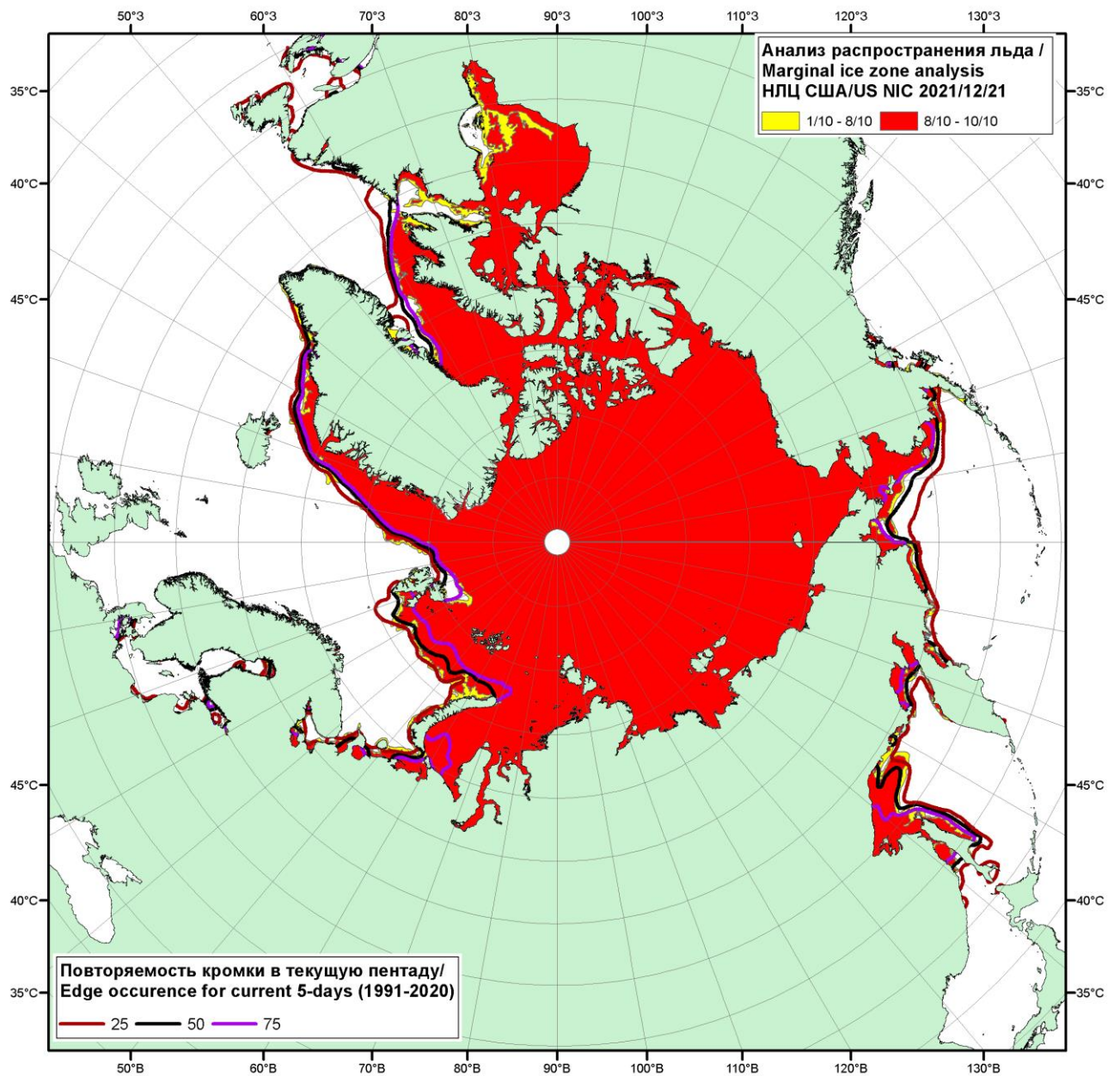
Рисунок 1в – Положение кромки льда и зон разреженных ( <8/10 ) и сплоченных ( \geq 8/10 ) льдов СЛО за 21.12.2021 г. на основе ледового анализа Национального Ледового Центра США и повторяемость кромки за 21-25.12 за период 1991-2020 гг. по наблюдениям SSMR-SSM/I-SSMIS (алгоритм NASATEAM)
