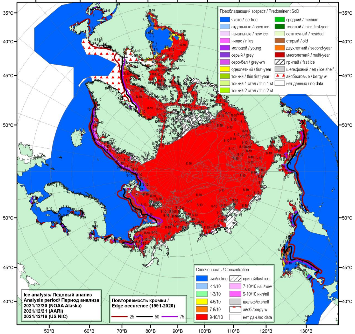
Рисунок 1а – Обзорная ледовая карта СЛЮ за 16.12-21.12.2021 г. (цветовая раскраска по общей сплоченности) на основе ледового анализа ААНИИ (21.12), NOAA Аляска (20.12) и Национального ледового центра США (16.12), и повторяемость кромки за 16.12-20.12 за период 1991-2020гг. по наблюдениям SSMR-SSM/I-SSMIS (алгоритм NASATEAM).
