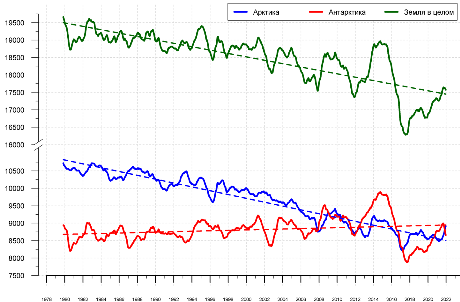
Рисунок 10 – Ежедневные сглаженные окном 365 суток значения приведенной ледовитости (площади морского льда) Арктики, Антарктики и Земли в целом с 26.10.1978 по 19.12.2021 на основе SSMR-SSM/I-SSMIS
