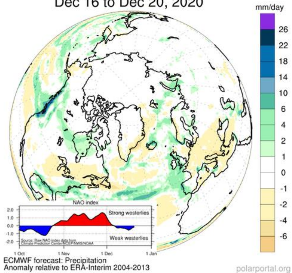
Рисунок 2ж – Аномалии приземной суммы осадков за 16.12 - 20.12 в 2020-2021 гг. относительно периода 2004-2013 гг. ( http://polarportal.dk )
