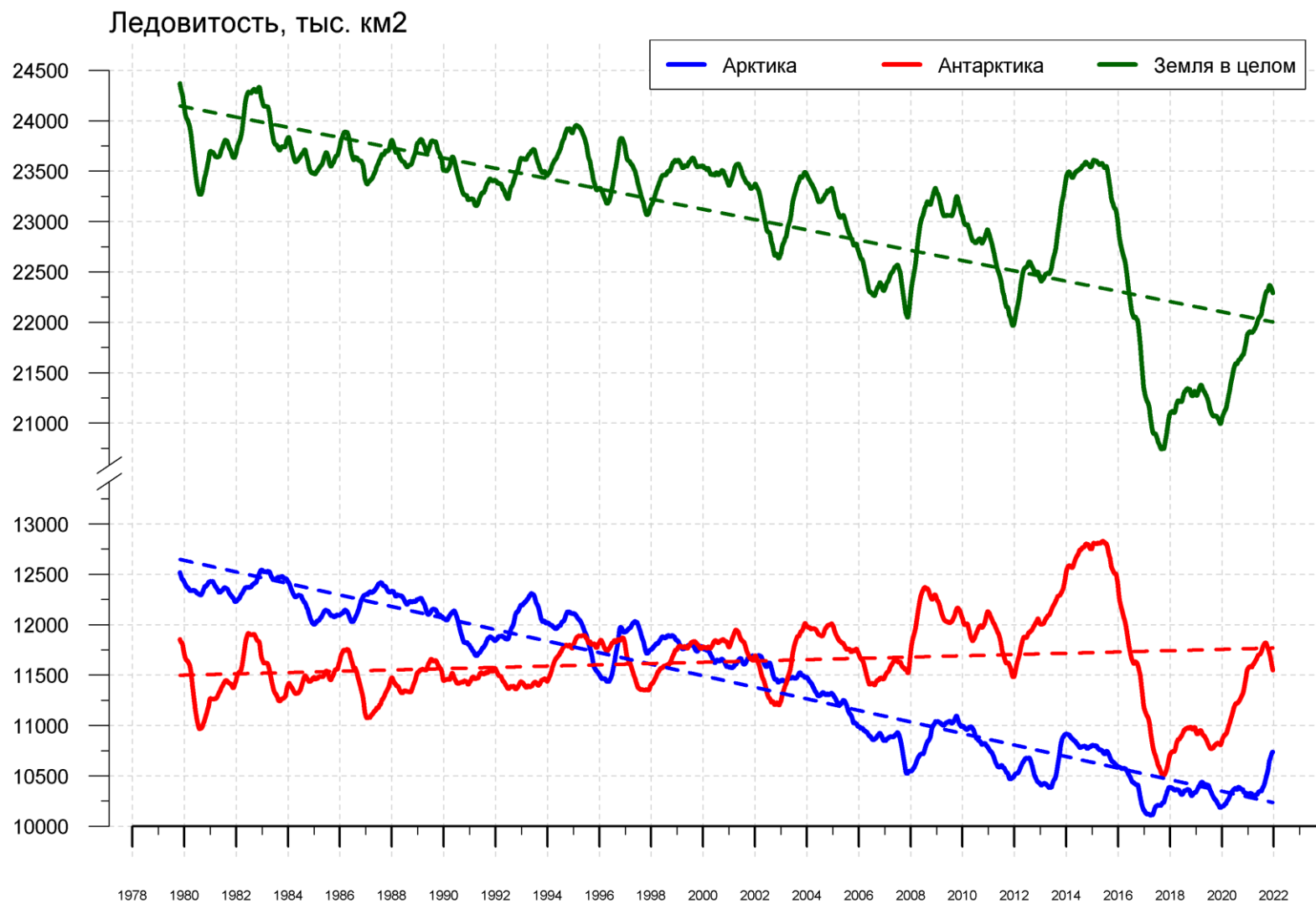
Рисунок 9 – Ежедневные сглаженные окном 365 суток значения ледовитости (площади распространения морского льда) Арктики, Антарктики и Земли в целом с 26.10.1978 по 19.12.2021 на основе SSMR-SSM/I-SSMIS
