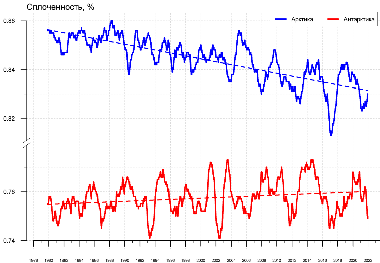
Рисунок 11 – Ежедневные сглаженные окном 365 суток значения средней общей сплоченности Арктики и Антарктики с 07.11.1978 по 19.12.2021 на основе SSMR-SSM/I-SSMIS
