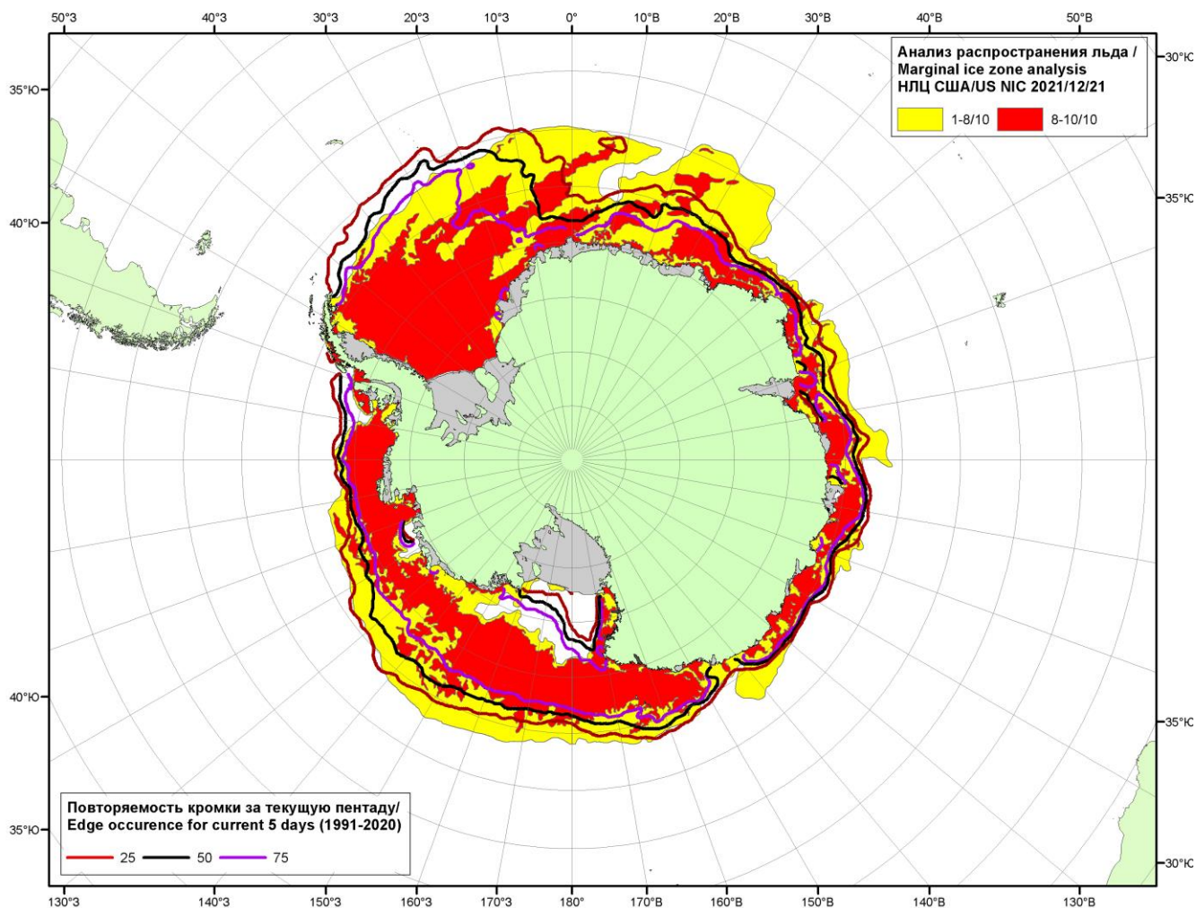
Рисунок 5в – Положение кромки льда и зон разреженных ( <8/10 ) и сплоченных ( \geq 8/10 ) льдов Южного океана за 21.12.2021 г. на основе ледового анализа Национального Ледового Центра США и повторяемость кромки за 21-25.12 за период 1991-2020 гг. по наблюдениям SSMR-SSM/I-SSMIS (алгоритм NASATEAM).
