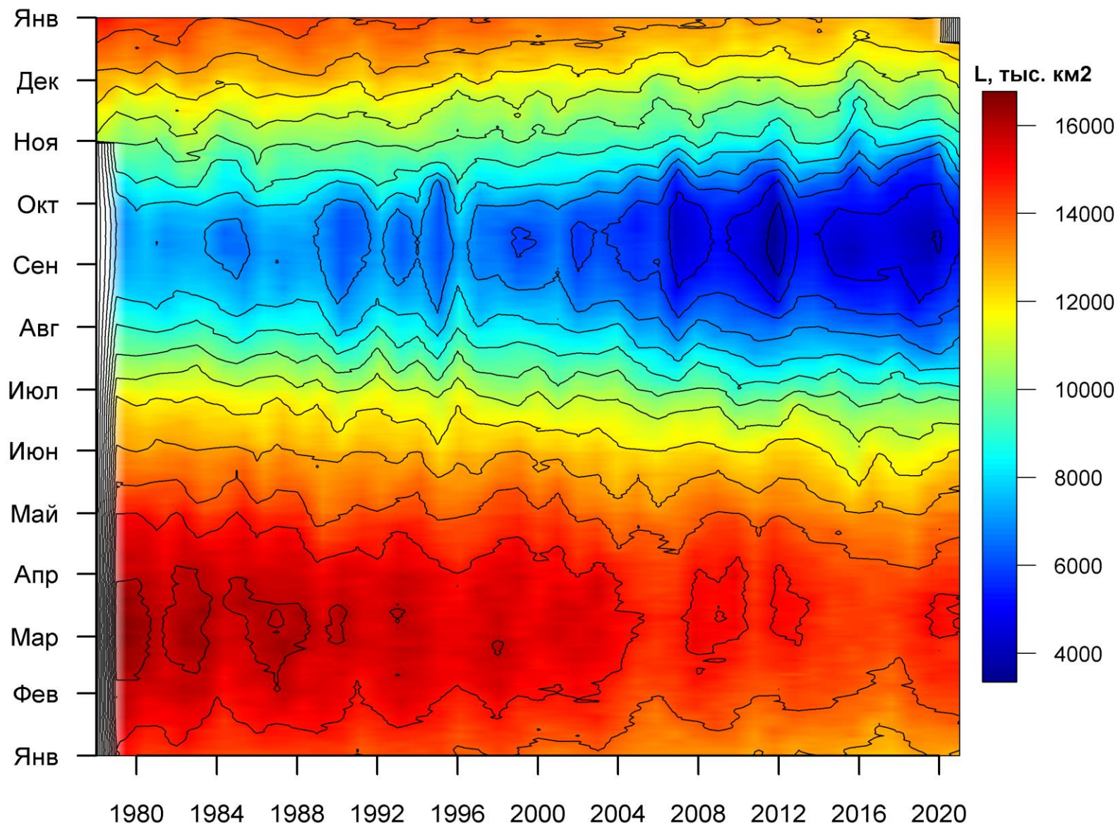
Рисунок 3б – Ежедневные оценки сезонных изменений ледовитости для Северной Полярной Области за период 26.10.1978 – 19.12.2021 на основе расчетов по данным SSMR-SSM/I-SSMIS, алгоритм NASATEAM.
