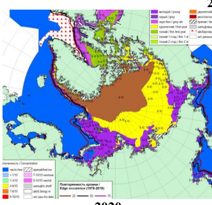
Рисунок 2а – Обзорная ледовая карта СЛО за 16.12-21.12.2021 г. и аналогичные периоды 2007-2020гг. на основе ледового анализа ААНИИ, НИЦ Планета, Канадской ледовой службы и Национального ледового центра США.
