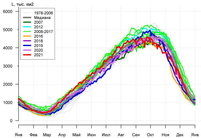
Рисунок 7а – Ежедневные оценки сезонного хода ледовитости Южного Океана и меридиональных секторов за период 26.10.1978 – 19.12.2021 по годам на основе расчетов по данным SSMR-SSM/I-SSMIS, алгоритм NASATEAM: а) Южный Океан, б) Атлантический сектор (60°W-30°E, море Уэдделла), в) Индоокеанский сектор (30°E-150°E, моря Космонавтов, Содружества, Моусона), г) Тихоокеанский сектор (150°E-60°W, моря Росса, Беллинсгаузена)
