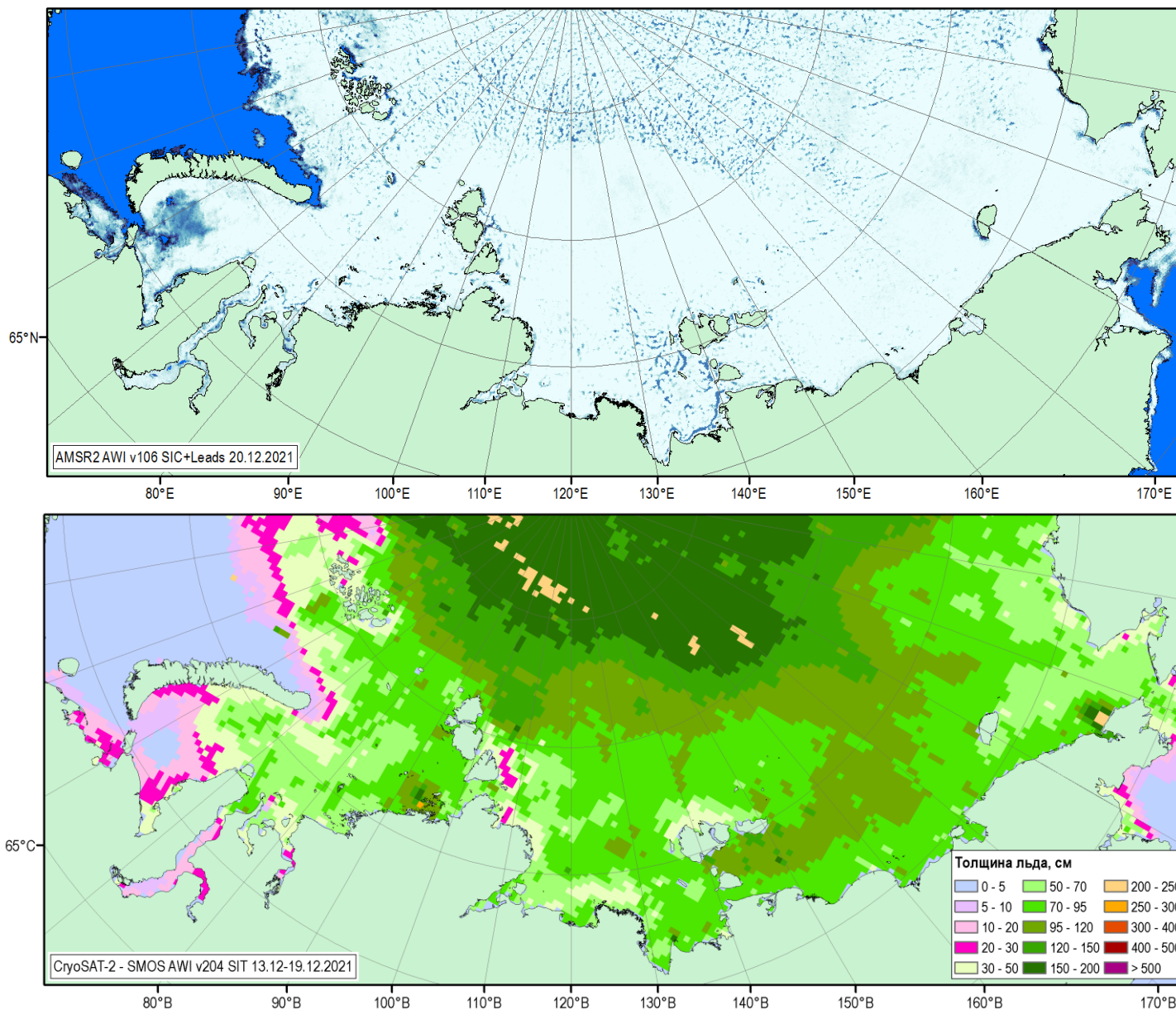
Рисунок 1г – Оценка сплоченности льда и расположения полыней по данным ИСЗ AMSR2 за 20.12.2021 (верх) и оценка толщин льда по данным ИСЗ CryoSAT-2 – SMOS за 13.12-19.12.2021 (AWI SIRAL).
