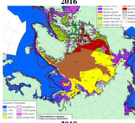
Рисунок 2а – Обзорная ледовая карта СЛО за 16.12-21.12.2021 г. и аналогичные периоды 2007-2020гг. на основе ледового анализа ААНИИ, НИЦ Планета, Канадской ледовой службы и Национального ледового центра США.
