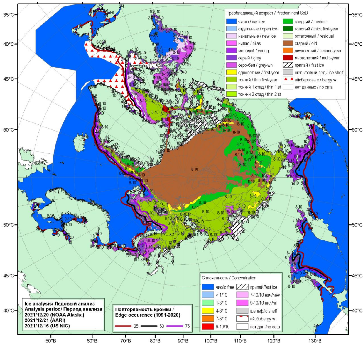
Рисунок 16 – Обзорная ледовая карта СЮ за 16.12-21.12.2021 г. (цветовая раскраска по преобладающему возрасту) на основе ледового анализа ААНИИ (21.12), NOAA Аляска (20.12) и Национального ледового центра США (16.12), и повторяемость кромки за 16.12-20.12 за период 1991-2020гг. по наблюдениям SSMR-SSM/I-SSMIS (алгоритм NASATEAM).
