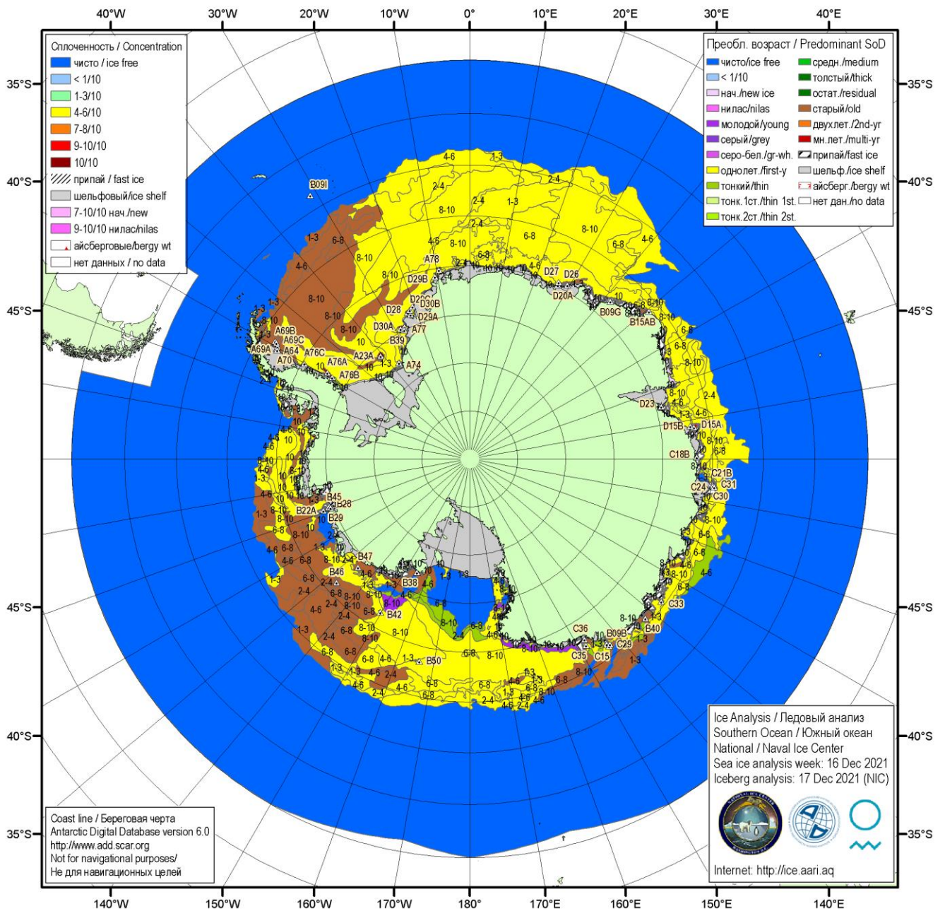
Рисунок 5б – Ледовая карта Южного океана (цветовая окраска по возрасту) и расположение крупных айсбергов на основе информации совместного ледового анализа НЛЦ США, ААНИИ и НМИ (Норвегия) за 16.12.2021.
