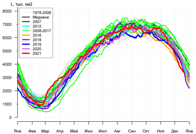
Рисунок 7а – Ежедневные оценки сезонного хода ледовитости Южного Океана и меридиональных секторов за период 26.10.1978 – 19.12.2021 по годам на основе расчетов по данным SSMR-SSM/I-SSMIS, алгоритм NASATEAM: а) Южный Океан, б) Атлантический сектор (60°W-30°E, море Уэдделла), в) Индоокеанский сектор (30°E-150°E, моря Космонавтов, Содружества, Моусона), г) Тихоокеанский сектор (150°E-60°W, моря Росса, Беллинсгаузена)
