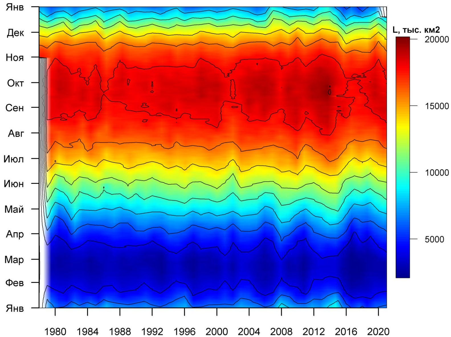
Рисунок 76 – Ежедневные оценки сезонных изменений ледовитости для Южного океана за период 26.10.1978 – 19.12.2021 на основе расчетов по данным SSMR-SSM/I-SSMIS, алгоритм NASATEAM.
