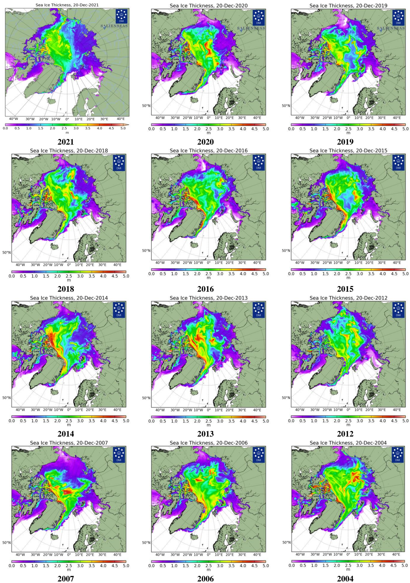
Рисунок 26 – Поля распределения средневзвешенной толщины льда совместной модели морского льда – океана NUCOM/CICE Датского метеорологического института 20.12 за 2004-2021 гг.
