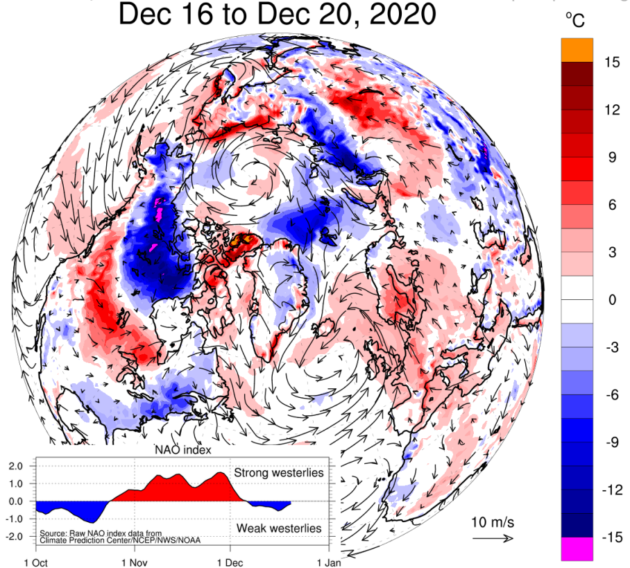
Рисунок 2е – Аномалии приземной температуры воздуха (2м) и осредненные вектора скорости ветра (10 м) за 16.12 - 20.12 в 2020-2021 гг. относительно периода 2004-2013 гг. ( http://polarportal.dk )
