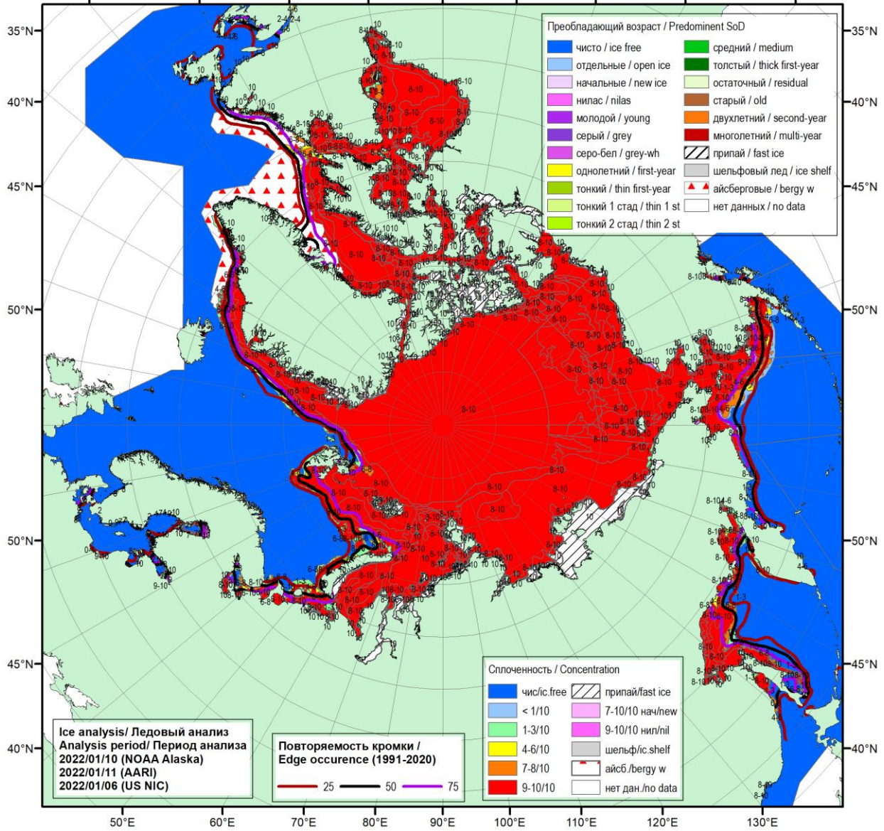
Рисунок 1а – Обзорная ледовая карта СЛЮ за 06.01-11.01.2022 г. (цветовая раскраска по общей сплоченности) на основе ледового анализа ААНИИ (11.01), NOAA Аляска (10.01) и Национального ледового центра США (06.01), и повторяемость кромки за 06.01-10.01 за период 1991-2020гг. по наблюдениям SSMR-SSM/I-SSMIS (алгоритм NASATEAM).
