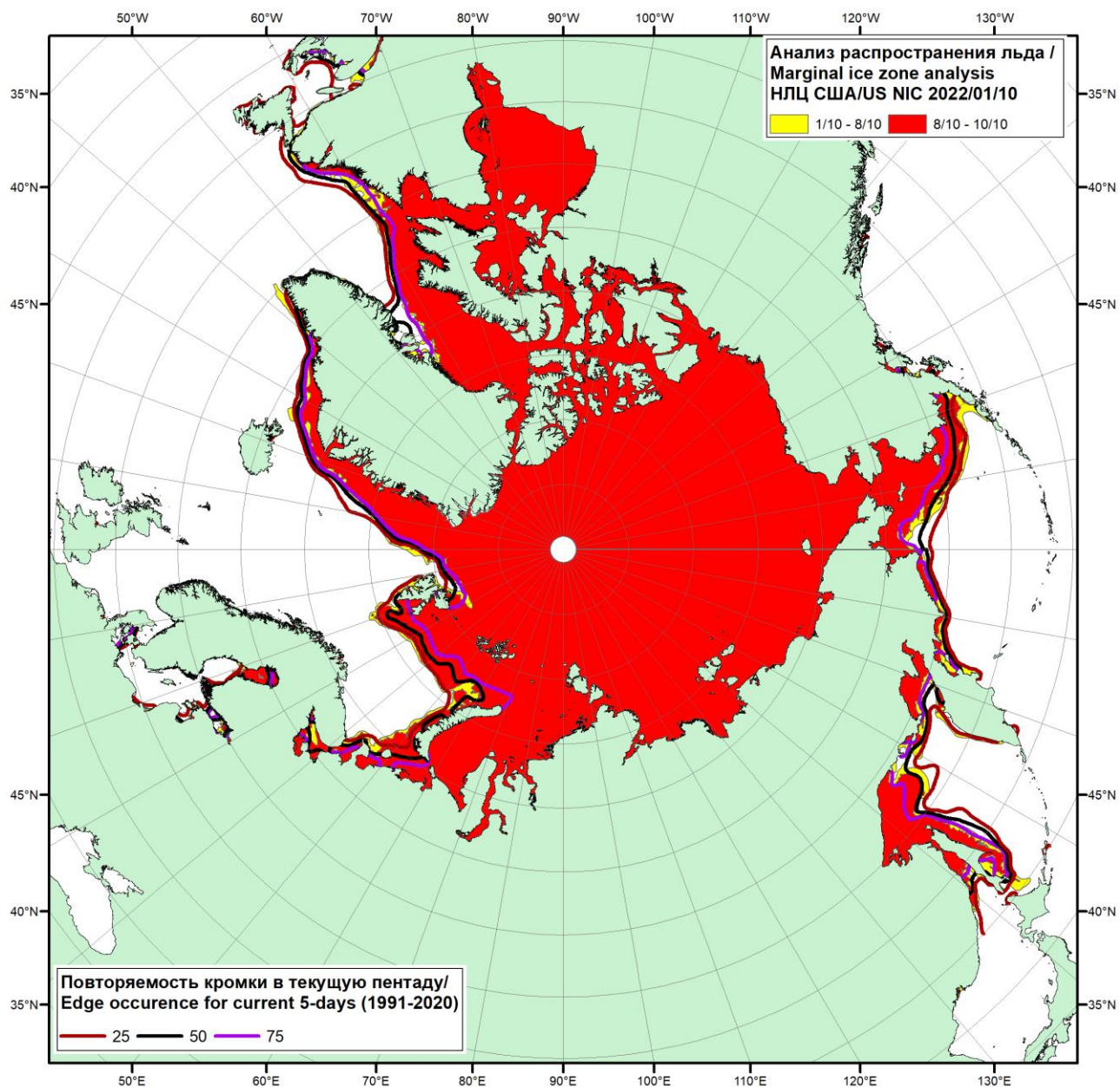
Рисунок 1в – Положение кромки льда и зон разреженных ( <8/10 ) и сплоченных ( \geq 8/10 ) льдов СЛО за 10.01.2022 г. на основе ледового анализа Национального Ледового Центра США и повторяемость кромки за 06.01-10.01 за период 1991-2020 гг. по наблюдениям SSMR-SSM/I-SSMIS (алгоритм NASATEAM)
