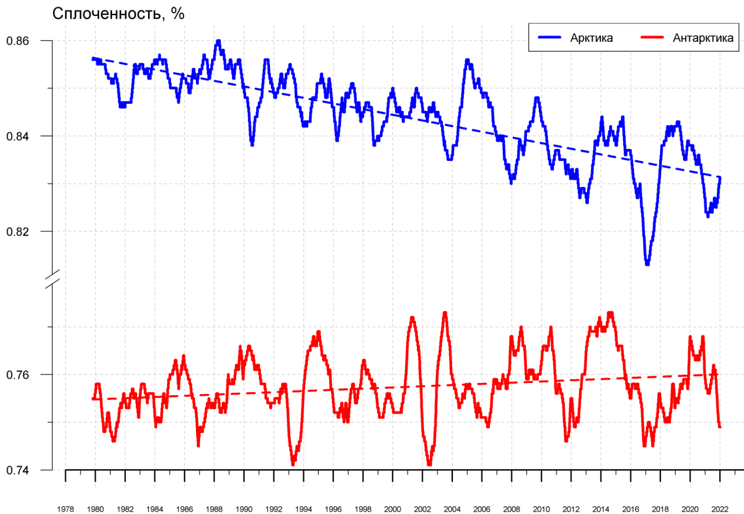
Рисунок 11 – Ежедневные сглаженные окном 365 суток значения средней общей сплоченности Арктики и Антарктики с 07.11.1978 по 09.01.2022 на основе SSMR-SSM/I-SSMIS
