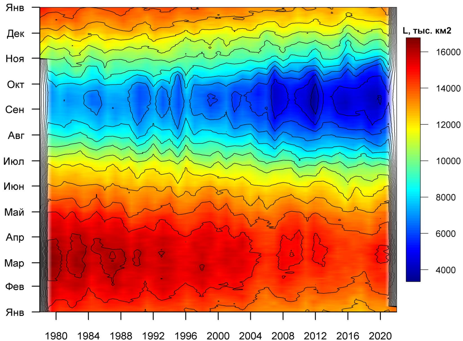
Рисунок 36 – Ежедневные оценки сезонных изменений ледовитости для Северной Полярной Области за период 26.10.1978 – 09.01.2022 на основе расчетов по данным SSMR-SSM/I-SSMIS, алгоритм NASATEAM.
