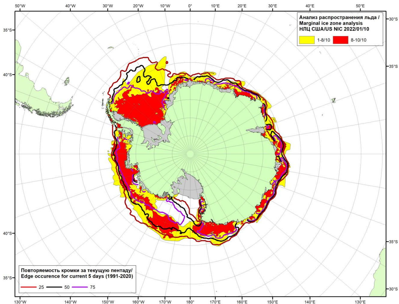
Рисунок 5в – Положение кромки льда и зон разреженных ( <8/10 ) и сплоченных ( \geq 8/10 ) льдов Южного океана за 10.01.2022 г. на основе ледового анализа Национального Ледового Центра США и повторяемость кромки за 06-10.01 за период 1991-2020 гг. по наблюдениям SSMR-SSM/I-SSMIS (алгоритм NASATEAM).
