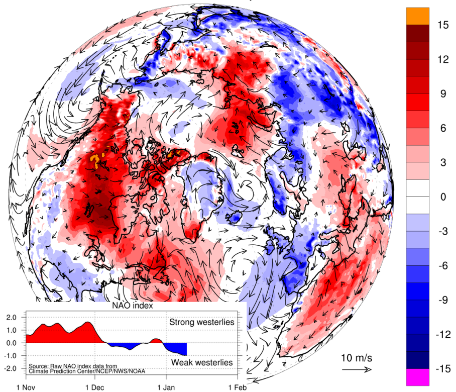
Рисунок 2е – Аномалии приземной температуры воздуха (2м) и осредненные вектора скорости ветра (10 м) за 06.01 - 10.01 в 2021-2022 гг. относительно периода 2004-2013 гг. ( http://polarportal.dk )
