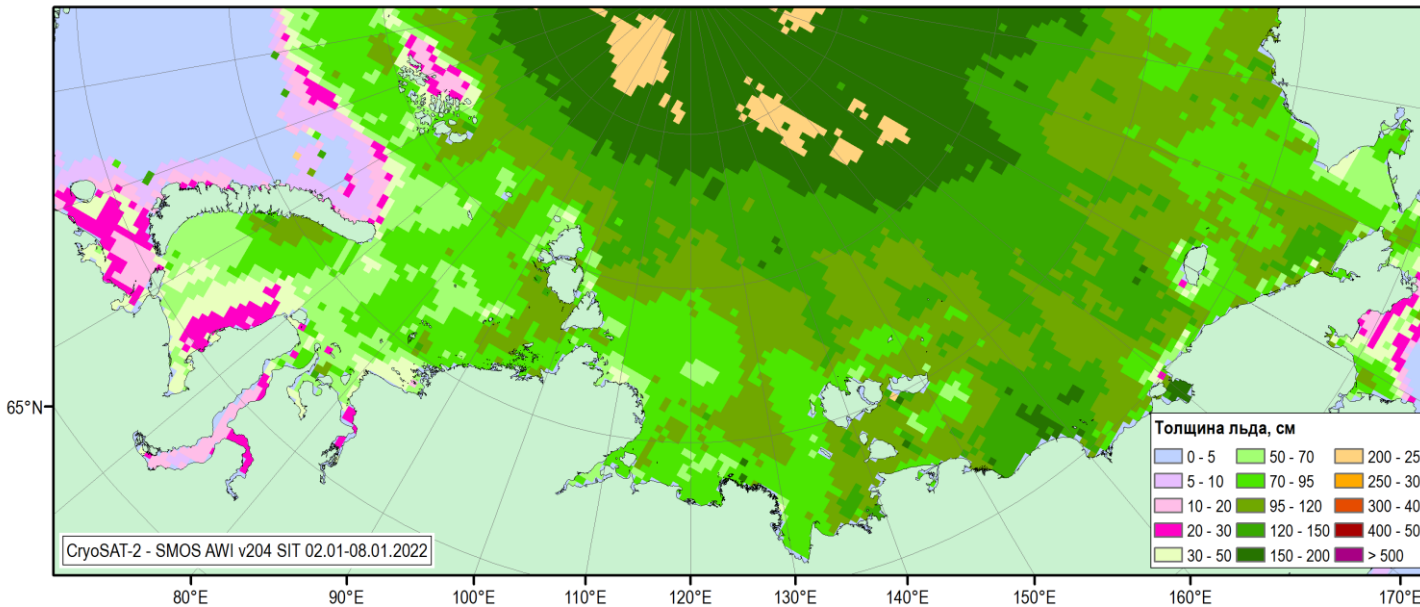
Рисунок 1г – Оценка сплоченности льда и расположения полыней по данным ИСЗ AMSR2 за 09.01.2022 (верх) и оценка толщин льда по данным ИСЗ CryoSAT-2 – SMOS за 02.01-08.01.2022 (AWI SIRAL).
