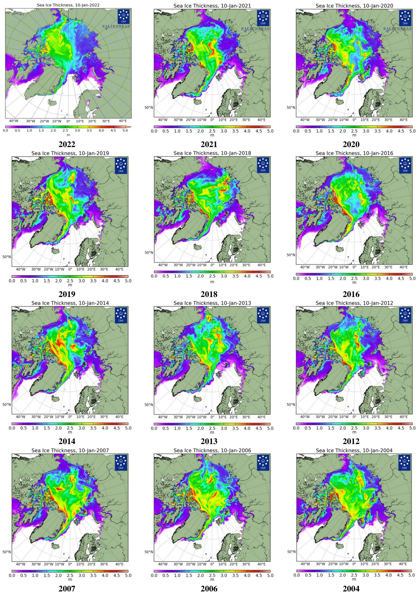
Рисунок 26 – Поля распределения средневзвешенной толщины льда совместной модели морского льда – океана NUCOM/CICE Датского метеорологического института 10.01 за 2004-2022 гг.
