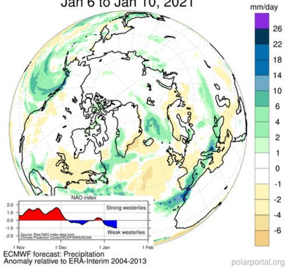
Рисунок 2ж – Аномалии приземной суммы осадков за 06.01 - 10.01 в 2021-2022 гг. относительно периода 2004-2013 гг. ( http://polarportal.dk )
