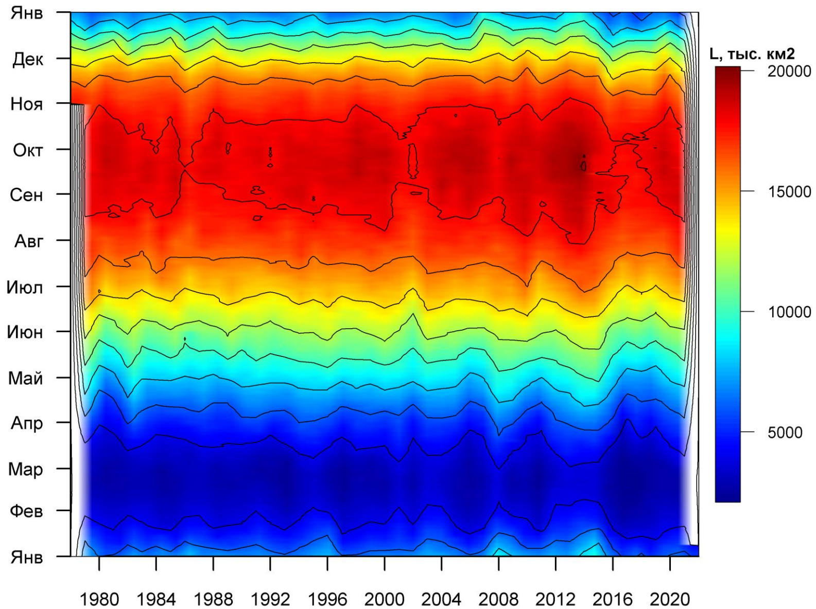
Рисунок 76 – Ежедневные оценки сезонных изменений ледовитости для Южного океана за период 26.10.1978 – 09.01.2022 на основе расчетов по данным SSMR-SSM/I-SSMIS, алгоритм NASATEAM.
