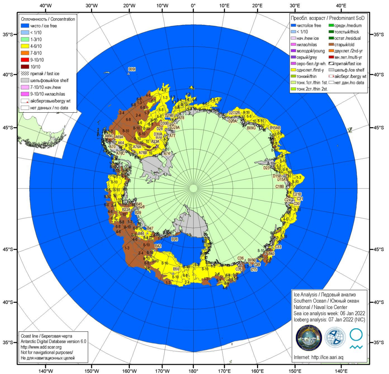
Рисунок 5б – Ледовая карта Южного океана (цветовая окраска по возрасту) и расположение крупных айсбергов на основе информации совместного ледового анализа НЛЦ США, ААНИИ и НМИ (Норвегия) за 06.01.2022.
