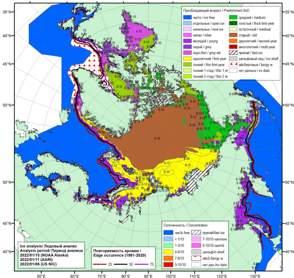
Рисунок 16 – Обзорная ледовая карта СЮ за 06.01-11.01.2022 г. (цветовая раскраска по преобладающему возрасту) на основе ледового анализа ААНИИ (11.01), NOAA Аляска (10.01) и Национального ледового центра США (06.01), и повторяемость кромки за 06.01-10.01 за период 1991-2020гг. по наблюдениям SSMR-SSM/I-SSMIS (алгоритм NASATEAM).
