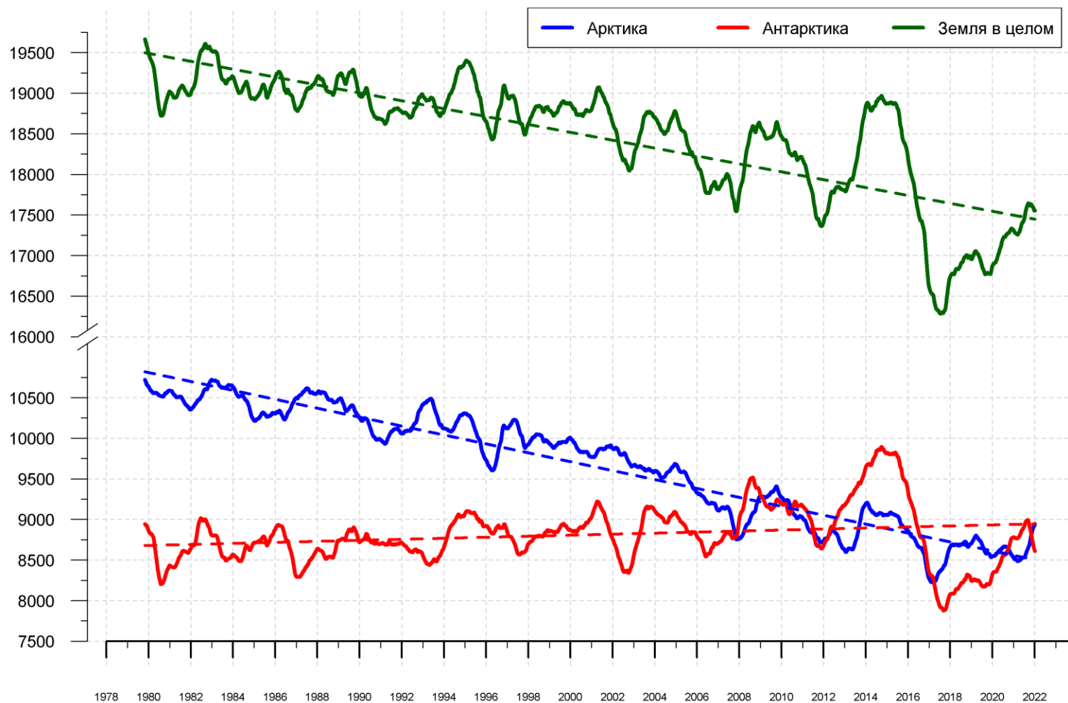
Рисунок 10 – Ежедневные сглаженные окном 365 суток значения приведенной ледовитости (площади морского льда) Арктики, Антарктики и Земли в целом с 26.10.1978 по 09.01.2022 на основе SSMR-SSM/I-SSMIS
