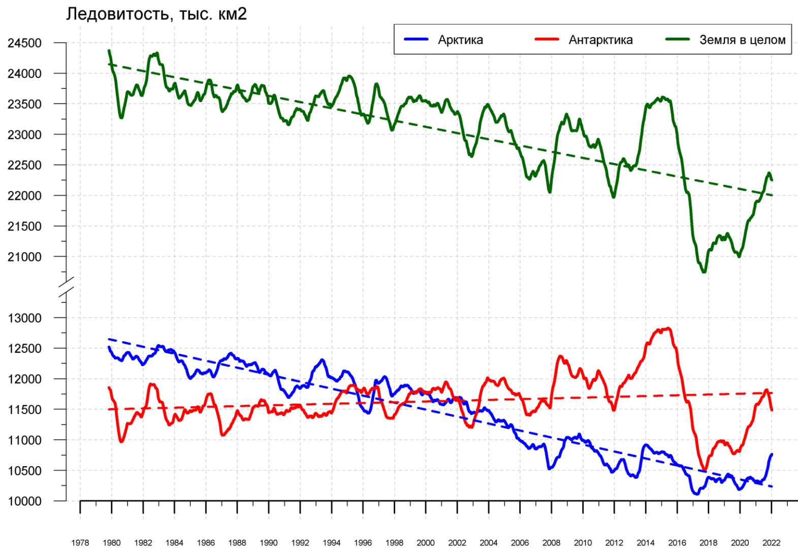
Рисунок 9 – Ежедневные сглаженные окном 365 суток значения ледовитости (площади распространения морского льда) Арктики, Антарктики и Земли в целом с 26.10.1978 по 09.01.2022 на основе SSMR-SSM/I-SSMIS
