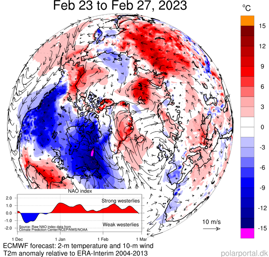
Рисунок 2е – Аномалии приземной температуры воздуха (2м) и осредненные вектора скорости ветра (10 м) за 23.02 – 27.02 в 2023-2024 гг. относительно периода 2004-2013 гг. ( http://polarportal.dk )
