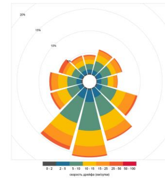
Рисунок 1а – Трек дрейфа ГСН и РСД дрейфующей станции «Северный Полус-41» на 28.02.2024, совмещенные с положением разрежений на основе данных ИСЗ AMSR2 за 27.02.2024 (Leads AWI, v110) и S1A. Красным/зеленым цветом выделены активные буи, синим неактивные буи. Диаграмма скоростей и направлений дрейфа за неделю дана в полярной проекции с осевым меридианом 0°
