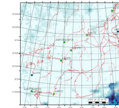
Сеть дрейфующих буев на 2024-02-28 0600UTC. AWI SIC LEADS (v.110) 2024-02-27PM. Обработка: МЦД МП ААНИИ.
