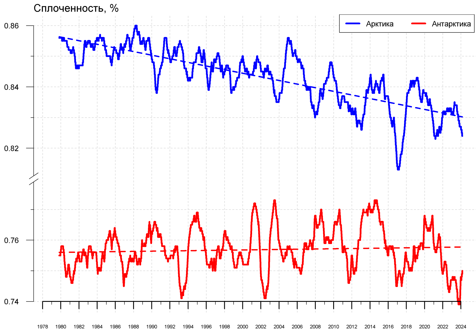
Рисунок 11 – Ежедневные сглаженные окном 365 суток значения средней общей сплоченности Арктики и Антарктики с 07.11.1978 по 25.02.2024 на основе SSMR-SSM/I-SSMIS
