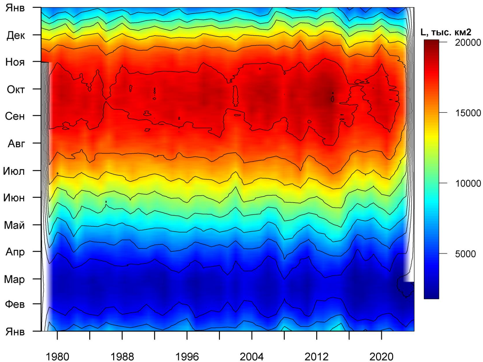
Рисунок 76 – Ежедневные оценки сезонных изменений ледовитости для Южного океана за период 26.10.1978 - 25.02.2024 на основе расчетов по данным SSMR-SSM/I-SSMIS, алгоритм NASATEAM.
