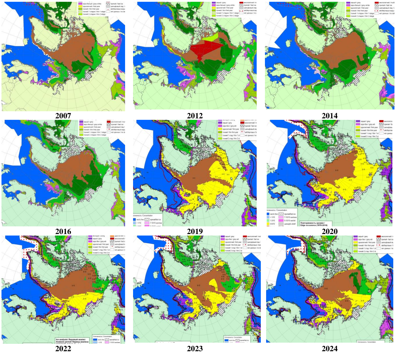
Рисунок 2а – Ледовые условия за 19.02-27.02.2024г. и аналогичные периоды 2007-2023 гг. на основе ледового анализа ААНИИ, НИЦ Планета, Канадской ледовой службы и Национального ледового центра США.
