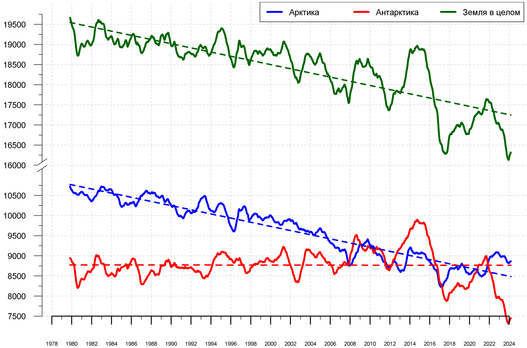
Рисунок 10 – Ежедневные сглаженные окном 365 суток значения приведенной ледовитости (площади морского льда) Арктики, Антарктики и Земли в целом с 26.10.1978 по 25.02.2024 на основе SSMR-SSM/I-SSMIS
