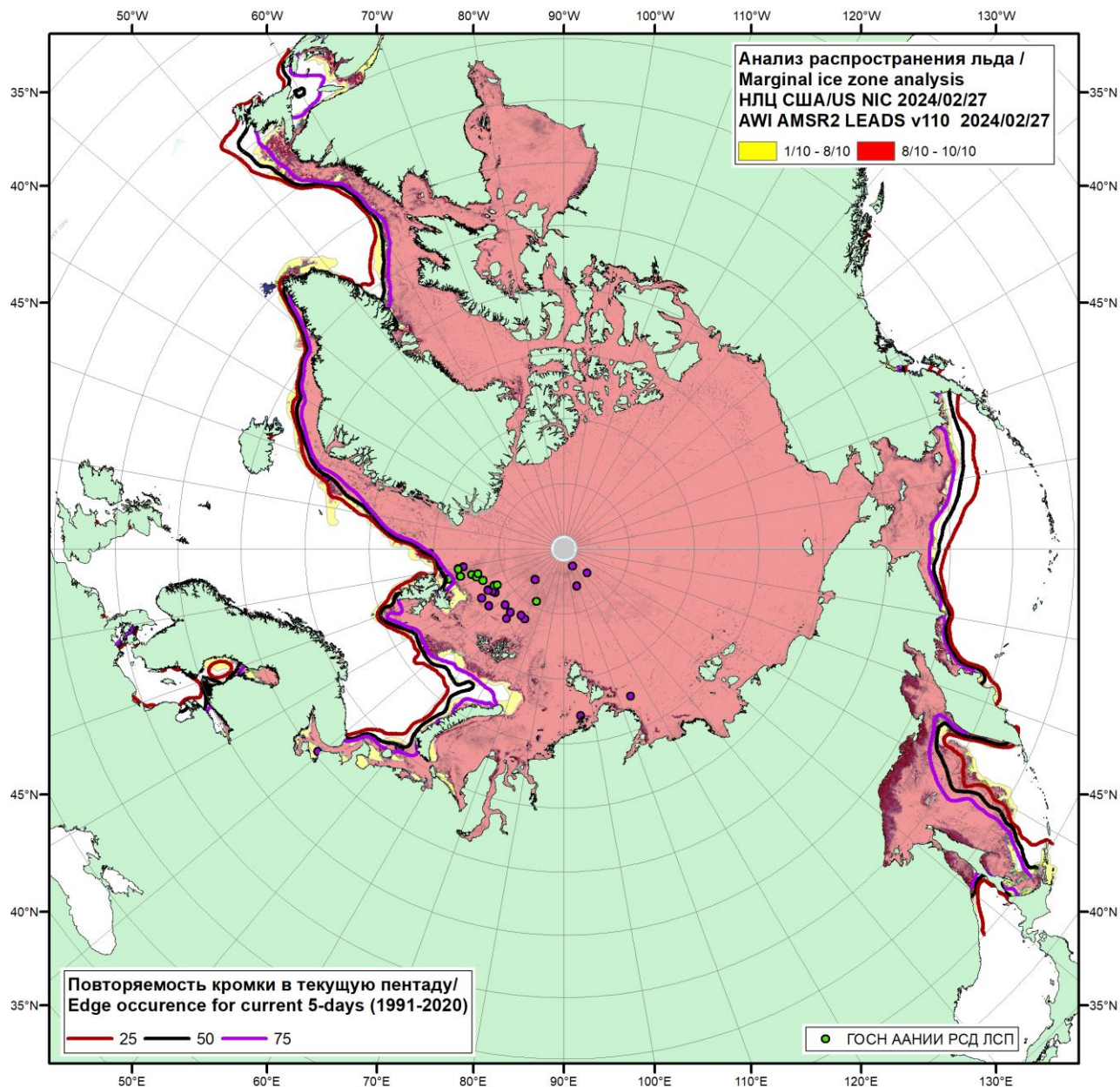
Рисунок 1г – Положение кромки льда и зон разреженных ( <8/10 ) и сплоченных ( \geq 8/10 ) льдов СЛО за 27.02.2024 г. на основе ледового анализа Национального Ледового Центра США и повторяемость кромки за 26-29.02 за период 1991-2020 гг. по наблюдениям SSMR-SSM/I-SSMIS (алгоритм NASATEAM), совмещенное с положением разрежений на основе данных ИСЗ AMSR2 27.02.2024 (AWI, v110) и положение РСД ЛСП на 27.02.2024.
