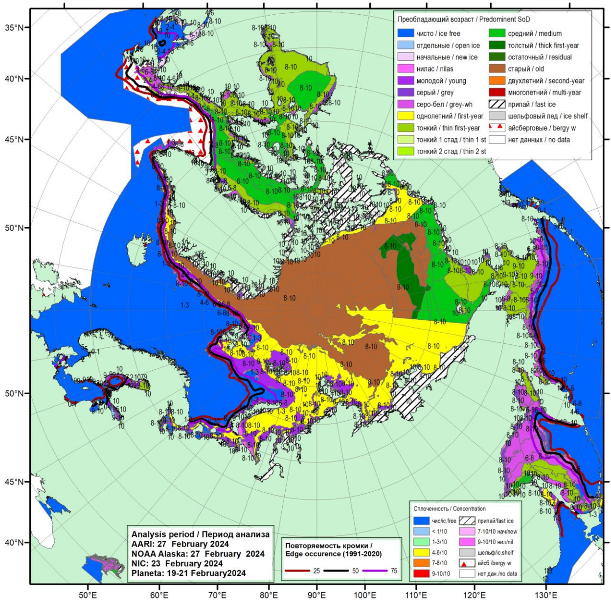
Рисунок 16 – Обзорная ледовая карта СЛО за 19.02 - 28.02.2024 г. (цветовая раскраска по преобладающему возрасту) на основе ледового анализа ААНИИ (27.02), NOAA Аляска (27.02), НИЦ Планета (19-21.02), Национального ледового центра США (23.02) и повторяемость кромки за 26-29.02 за период 1991-2020гг. по наблюдениям SSMR-SSM/I-SSMIS (алгоритм NASATEAM).
