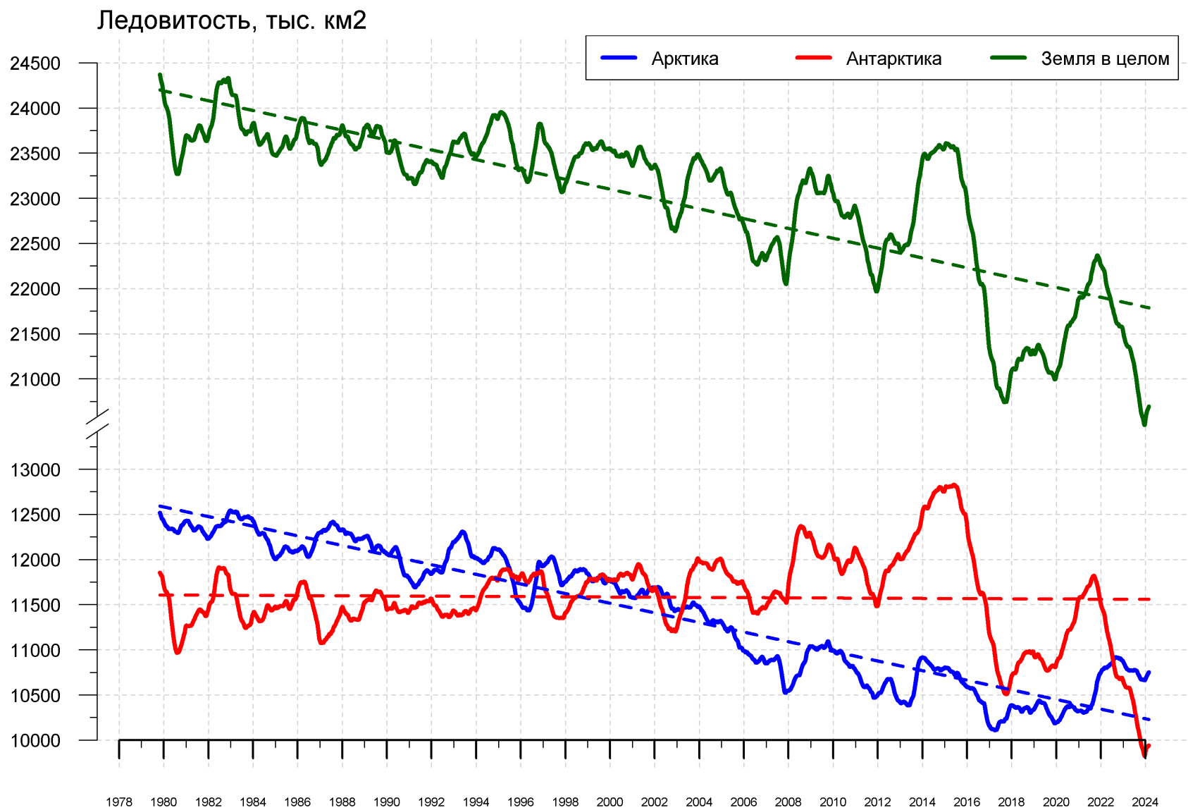
Рисунок 9 – Ежедневные сглаженные окном 365 суток значения ледовитости (площади распространения морского льда) Арктики, Антарктики и Земли в целом с 26.10.1978 по 25.02.2024 на основе SSMR-SSM/I-SSMIS
