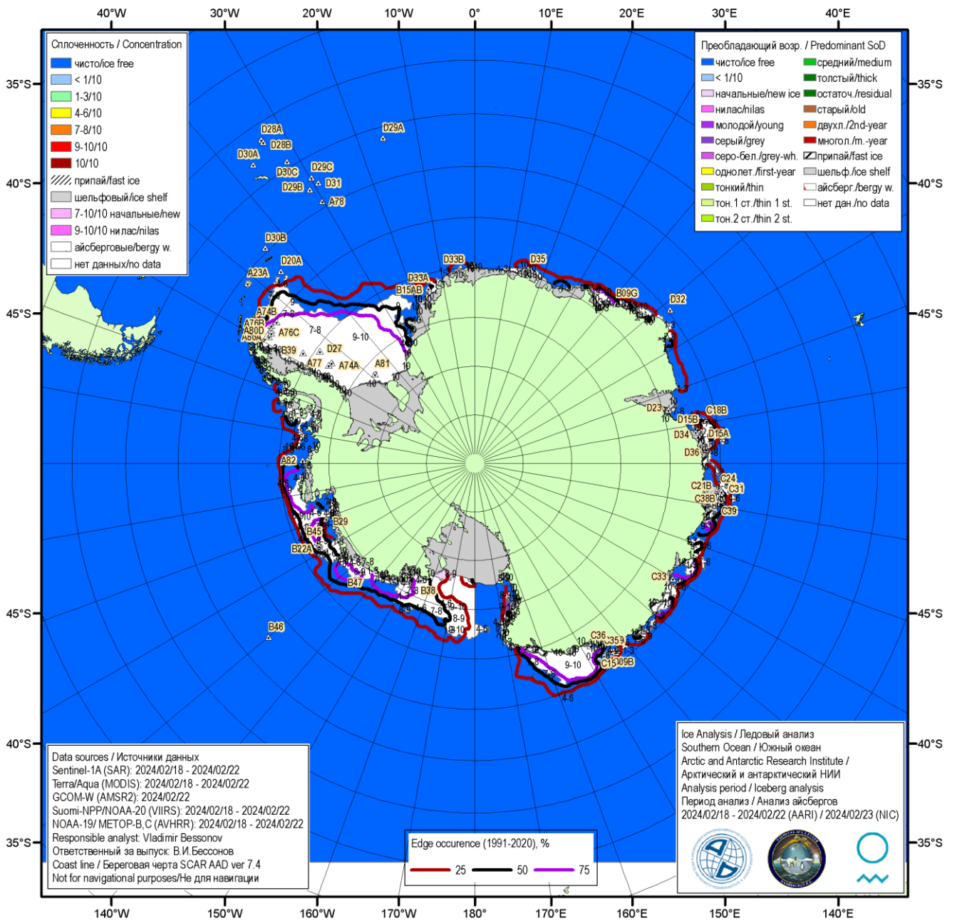
Рисунок 5в – Ледовая карта Южного океана (цветовая окраска по возрасту) и расположение крупных айсбергов на основе ледового анализа за 22.02.2024 в рамках проекта совместного ледового картирования Южного океана ААНИИ, НЛЦ США и НМИ.
