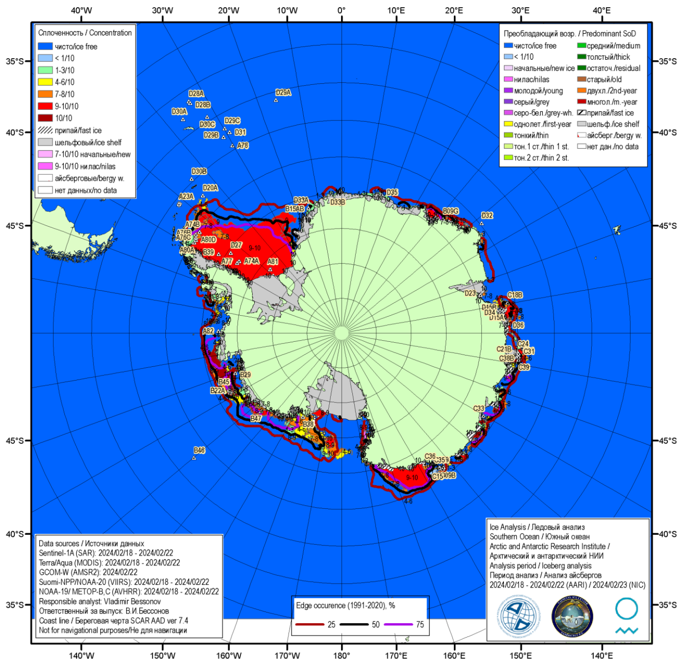
Рисунок 5а – Ледовая карта Южного океана (цветовая окраска по общей сплоченности) и расположение крупных айсбергов на основе ледового анализа за 22.02.2024 в рамках проекта совместного ледового картирования Южного океана ААНИИ, НЛЦ США и НМИ.
