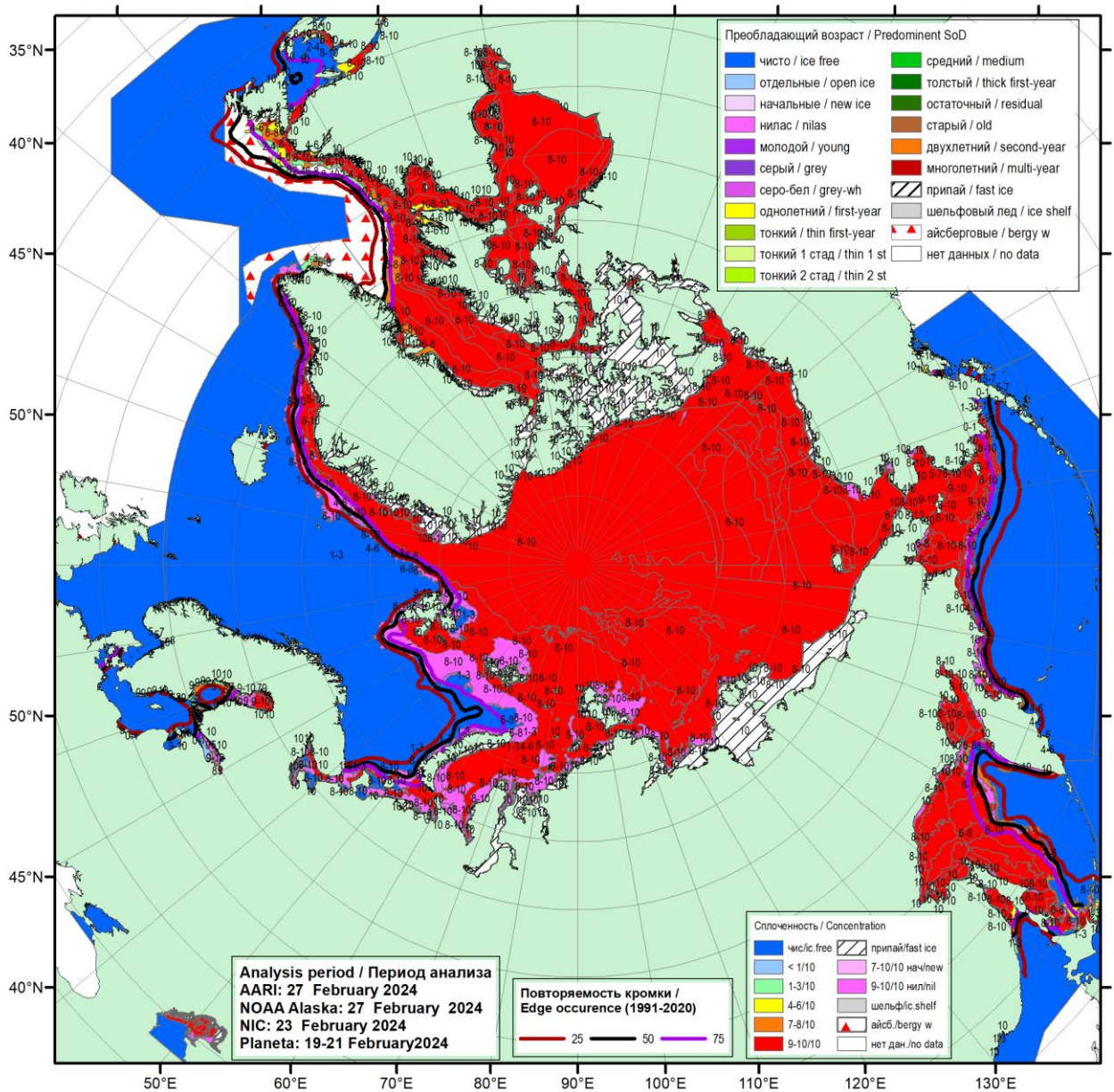
Рисунок 16 – Обзорная ледовая карта СЛО за 19.02 - 28.02.2024 г. (цветовая раскраска по общей сплоченности) на основе ледового анализа ААНИИ (27.02), NOAA Аляска (27.02), НИЦ Планета (19-21.02), Национального ледового центра США (23.02) и повторяемость кромки за 26-29.02 за период 1991-2020гг. по наблюдениям SSMR-SSM/I-SSMIS (алгоритм NASATEAM).
