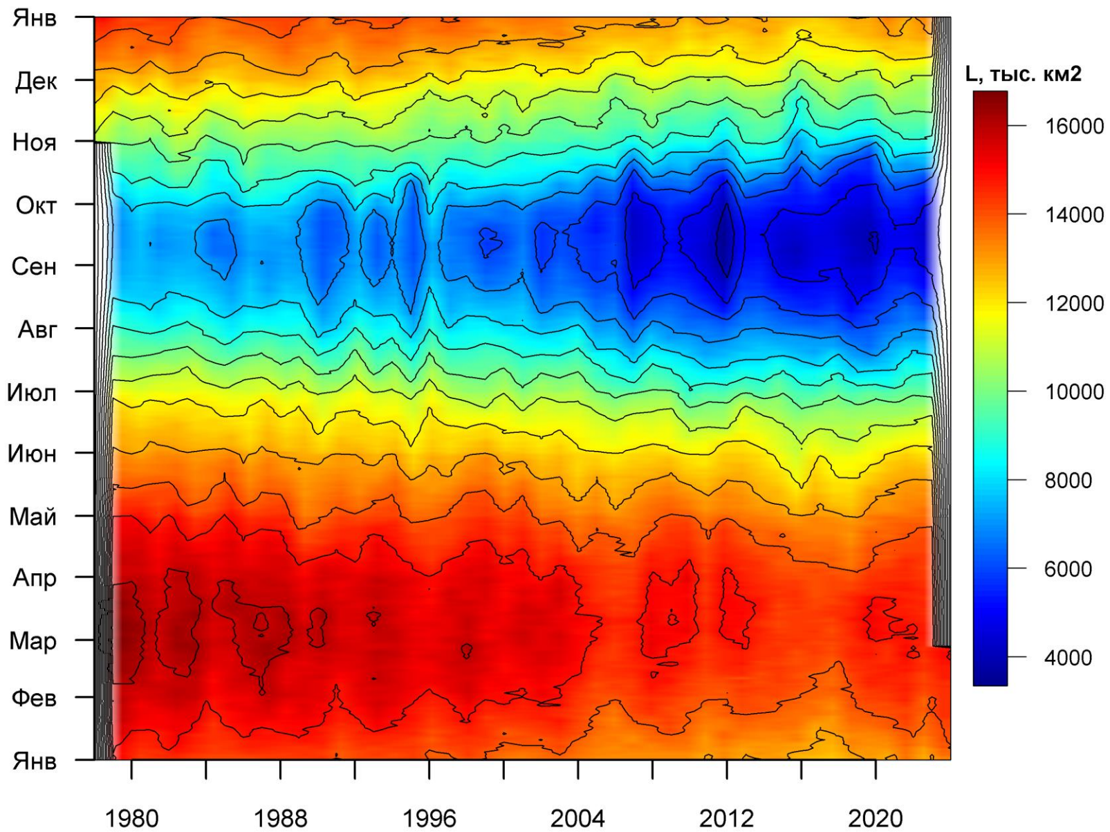
Рисунок 36 – Ежедневные оценки сезонных изменений ледовитости для Северной Полярной Области за период 26.10.1978 – 25.02.2024 на основе расчетов по данным SSMR-SSM/I-SSMIS, алгоритм NASATEAM.
