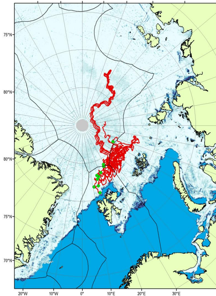
Сеть дрейфующих буев на 2024-02-28 0600UTC. AWI SIC LEADS (v.110) 2024-02-27PM. Обработка: МЦД МП ААНИИ.
