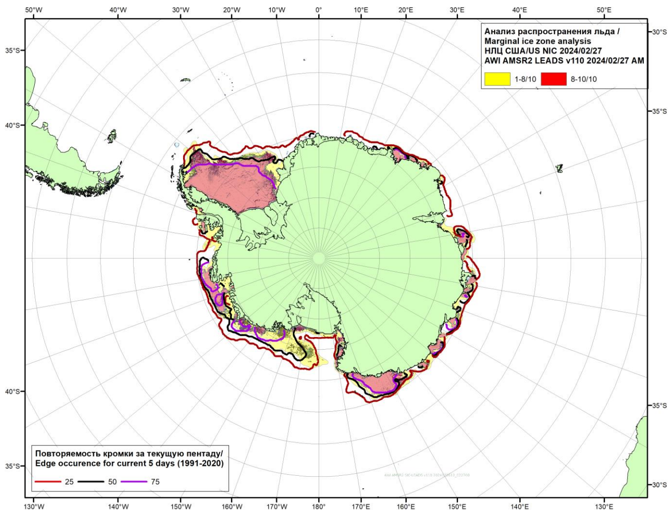
Рисунок 5в – Положение кромки льда и зон разреженных ( <8/10 ) и сплоченных ( \geq 8/10 ) льдов Южного океана за 27.02.2024 г. на основе ледового анализа Национального Ледового Центра США и повторяемость кромки за 26-29.02 за период 1991-2020 гг. по наблюдениям SSMR-SSM/I-SSMIS (алгоритм NASATEAM), совмещенное с положением разрежений на основе данных ИСЗ AMSR2 за 27.02.2024 (AWI, v110).
