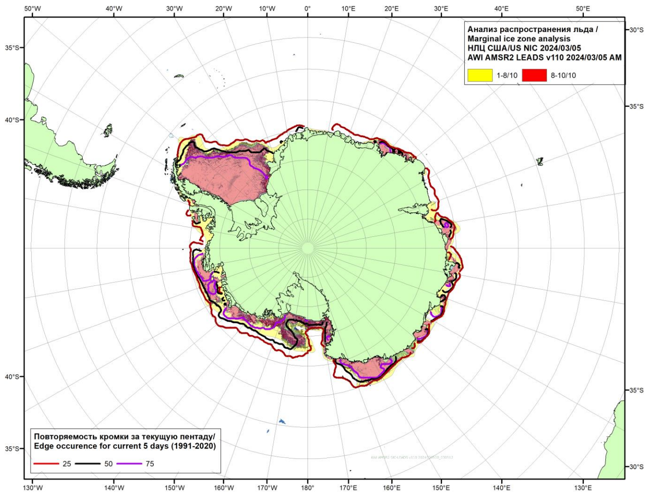
Рисунок 5в – Положение кромки льда и зон разреженных ( <8/10 ) и сплоченных ( \geq 8/10 ) льдов Южного океана за 05.03.2024 г. на основе ледового анализа Национального Ледового Центра США и повторяемость кромки за 01-05.03 за период 1991-2020 гг. по наблюдениям SSMR-SSM/I-SSMIS (алгоритм NASATEAM), совмещенное с положением разрежений на основе данных ИСЗ AMSR2 за 05.03.2024 (AWI, v110).
