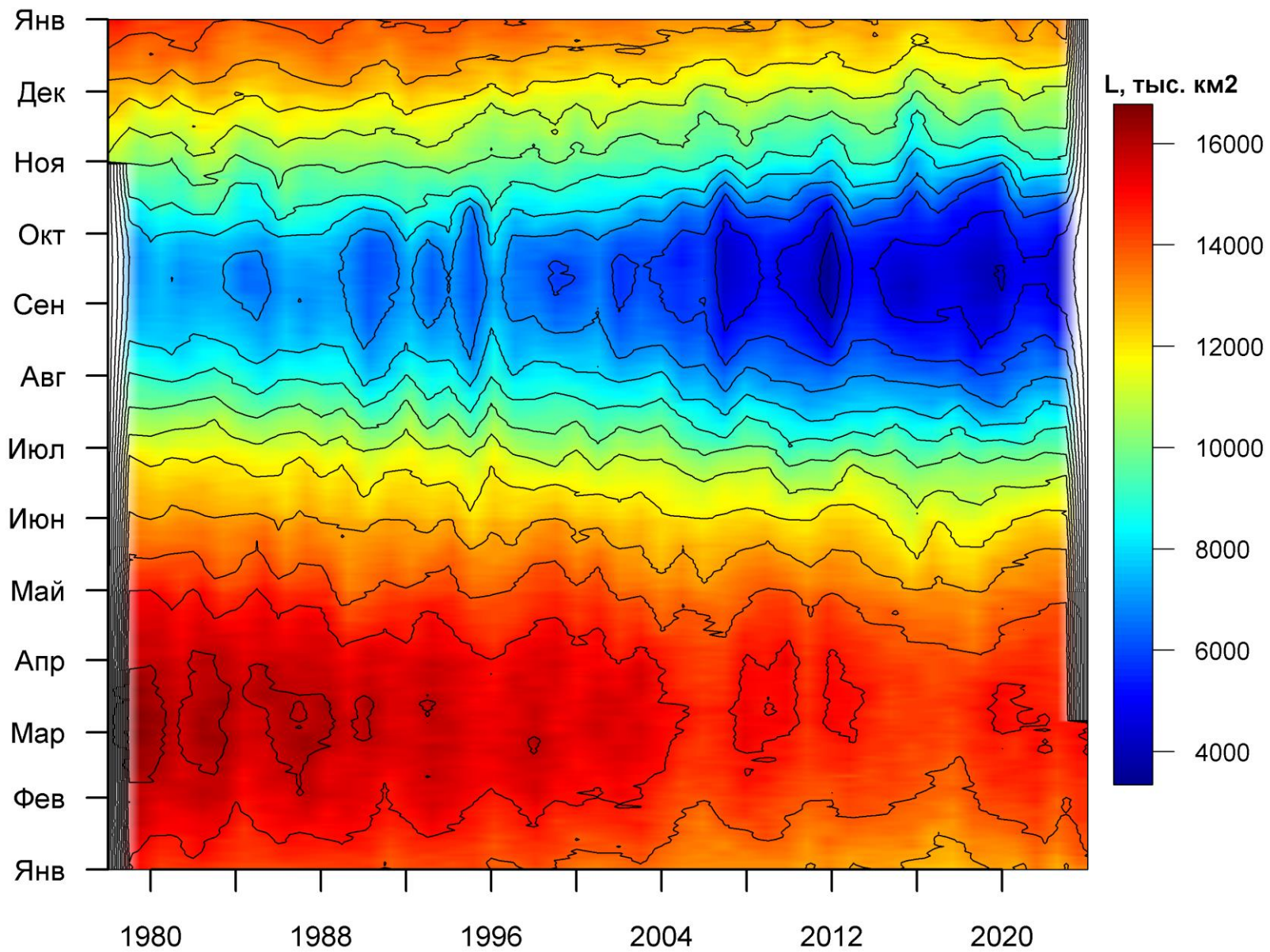
Рисунок 36 – Ежедневные оценки сезонных изменений ледовитости для Северной Полярной Области за период 26.10.1978 – 03.03.2024 на основе расчетов по данным SSMR-SSM/I-SSMIS, алгоритм NASATEAM.
