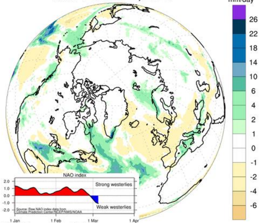
Рисунок 2ж – Аномалии приземной суммы осадков 01.03 – 05.03 в 2023-2024 гг. относительно периода 2004-2013 гг. ( http://polarportal.dk )
