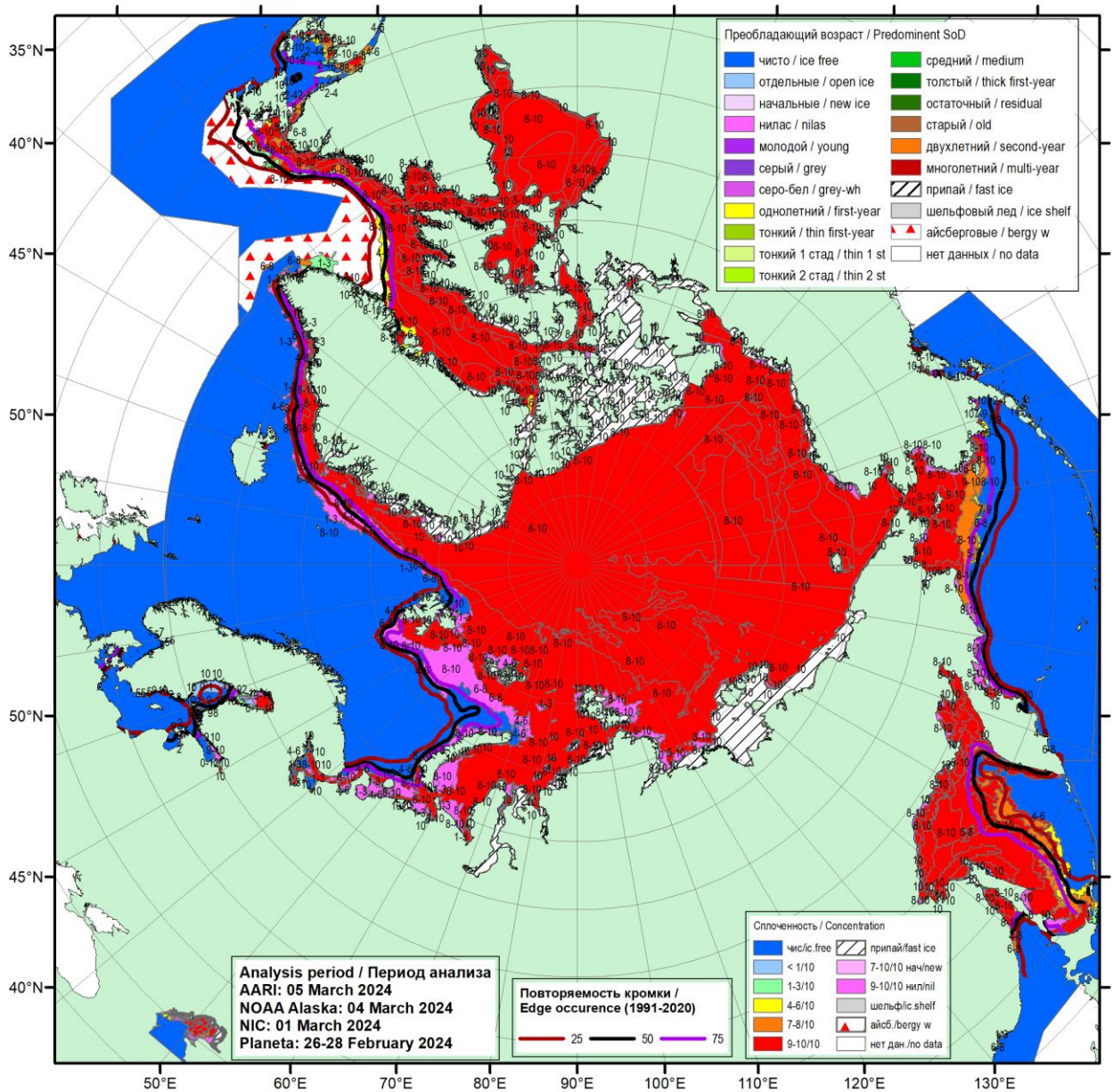
Рисунок 16 – Обзорная ледовая карта СЛО за 26.02 - 05.03.2024 г. (цветовая раскраска по общей сплоченности) на основе ледового анализа ААНИИ (05.03), НОАА Аляска (04.03), НИЦ Планета (26-28.02), Национального ледового центра США (01.03) и повторяемость кромки за 01-05.03 за период 1991-2020гг. по наблюдениям SSMR-SSM/I-SSMIS (алгоритм NASATEAM).
