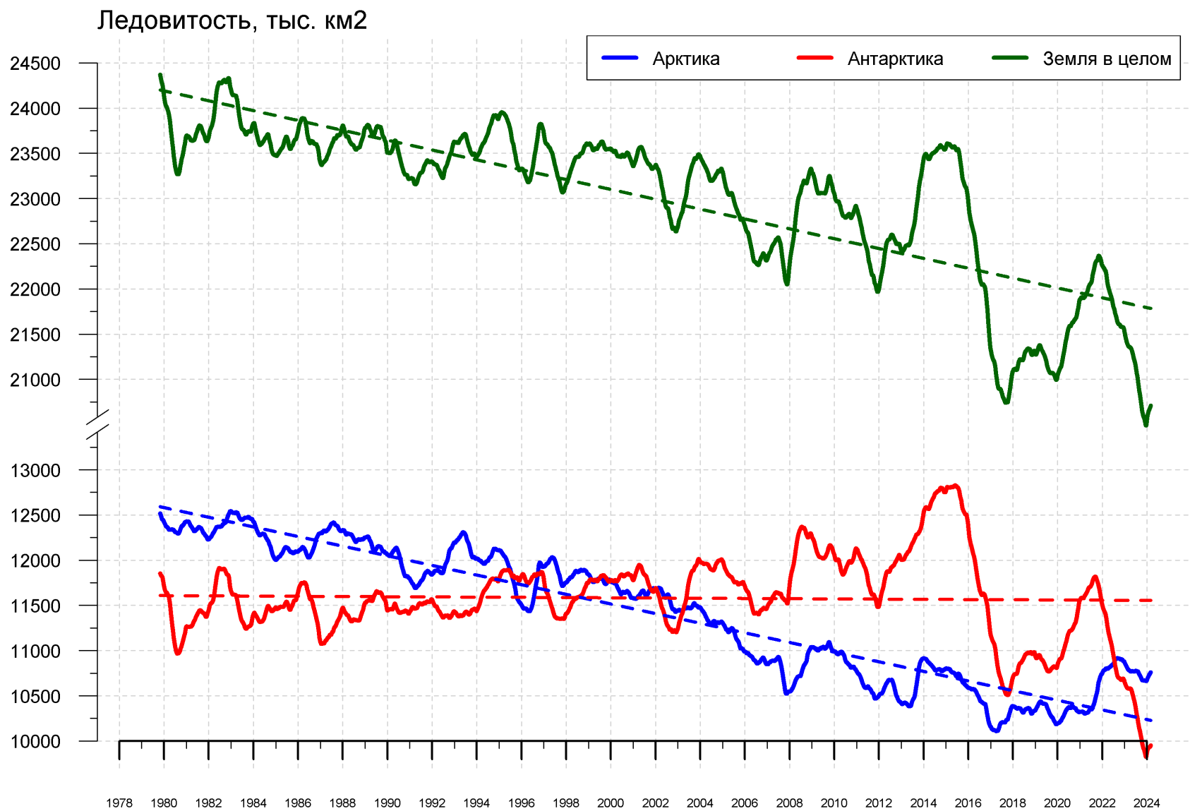
Рисунок 9 – Ежедневные сглаженные окном 365 суток значения ледовитости (площади распространения морского льда) Арктики, Антарктики и Земли в целом с 26.10.1978 по 03.03.2024 на основе SSMR-SSM/I-SSMIS
