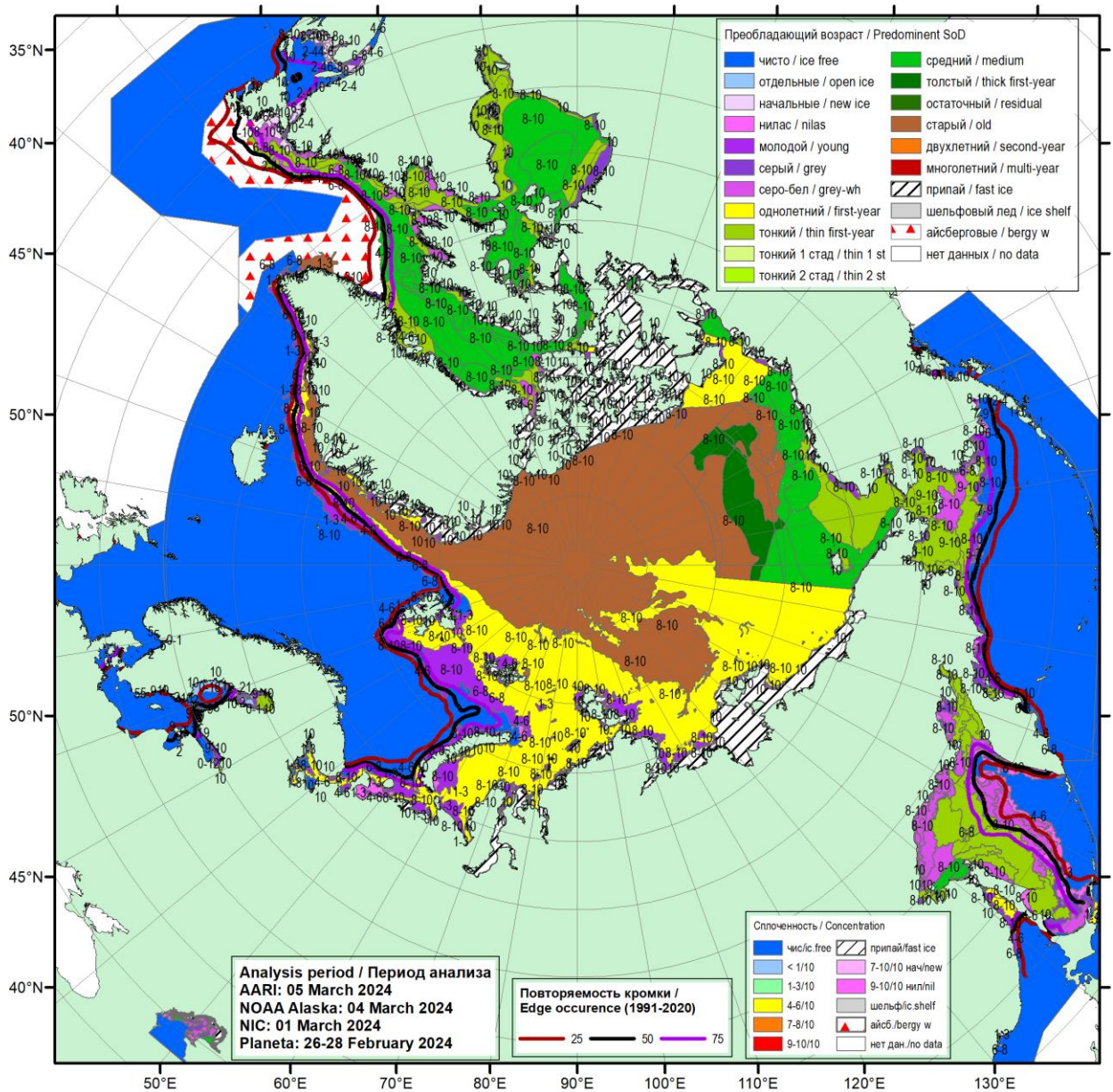
Рисунок 16 – Обзорная ледовая карта СЛО за 26.02 - 05.03.2024 г. (цветовая раскраска по преобладающему возрасту) на основе ледового анализа ААНИИ (05.03), NOAA Аляска (04.03), НИЦ Планета (26-28.02), Национального ледового центра США (01.03) и повторяемость кромки за 01-05.03 за период 1991-2020гг. по наблюдениям SSMR-SSM/I-SSMIS (алгоритм NASATEAM).
