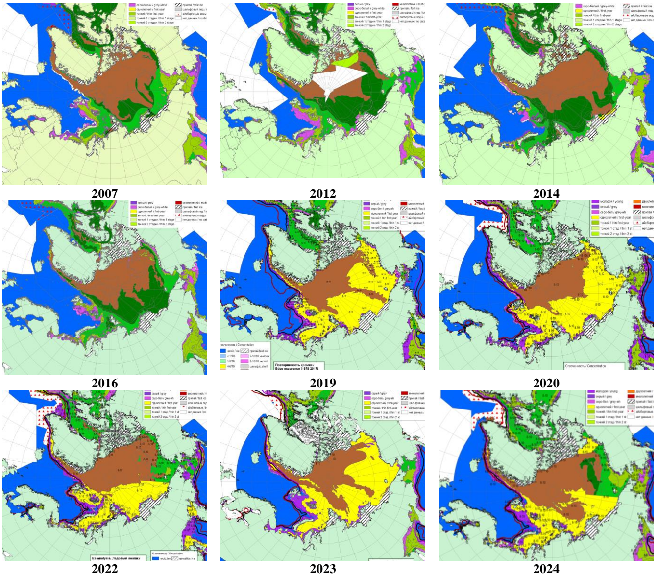
Рисунок 2а – Ледовые условия за 26.02-05.03.2024г. и аналогичные периоды 2007-2023 гг. на основе ледового анализа ААНИИ, НИЦ Планета, Канадской ледовой службы и Национального ледового центра США.
