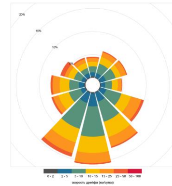
Рисунок 1а – Трек дрейфа ГСН и РСД дрейфующей станции «Северный Полус-41» на 28.02.2024, совмещенные с положением разрежений на основе данных ИСЗ AMSR2 за 27.02.2024 (Leads AWI, v110) и S1A. Красным/зеленым цветом выделены активные буи, синим неактивные буи. Диаграмма скоростей и направлений дрейфа за неделю дана в полярной проекции с осевым меридианом 0°
