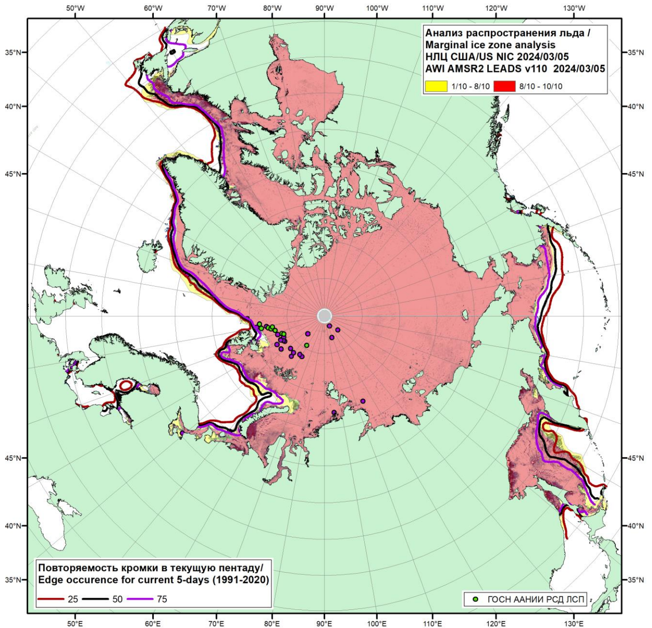
Рисунок 1г – Положение кромки льда и зон разреженных (<8/10) и сплоченных (≥8/10) льдов СЛО за 05.03.2024 г. на основе ледового анализа Национального Ледового Центра США и повторяемость кромки за 01-05.03 за период 1991-2020 гг. по наблюдениям SSMR-SSM/I-SSMIS (алгоритм NASATEAM), совмещенное с положением разрежений на основе данных ИСЗ AMSR2 05.03.2024 (AWI, v110) и положение РСД ЛСП на 06.03.2024.
