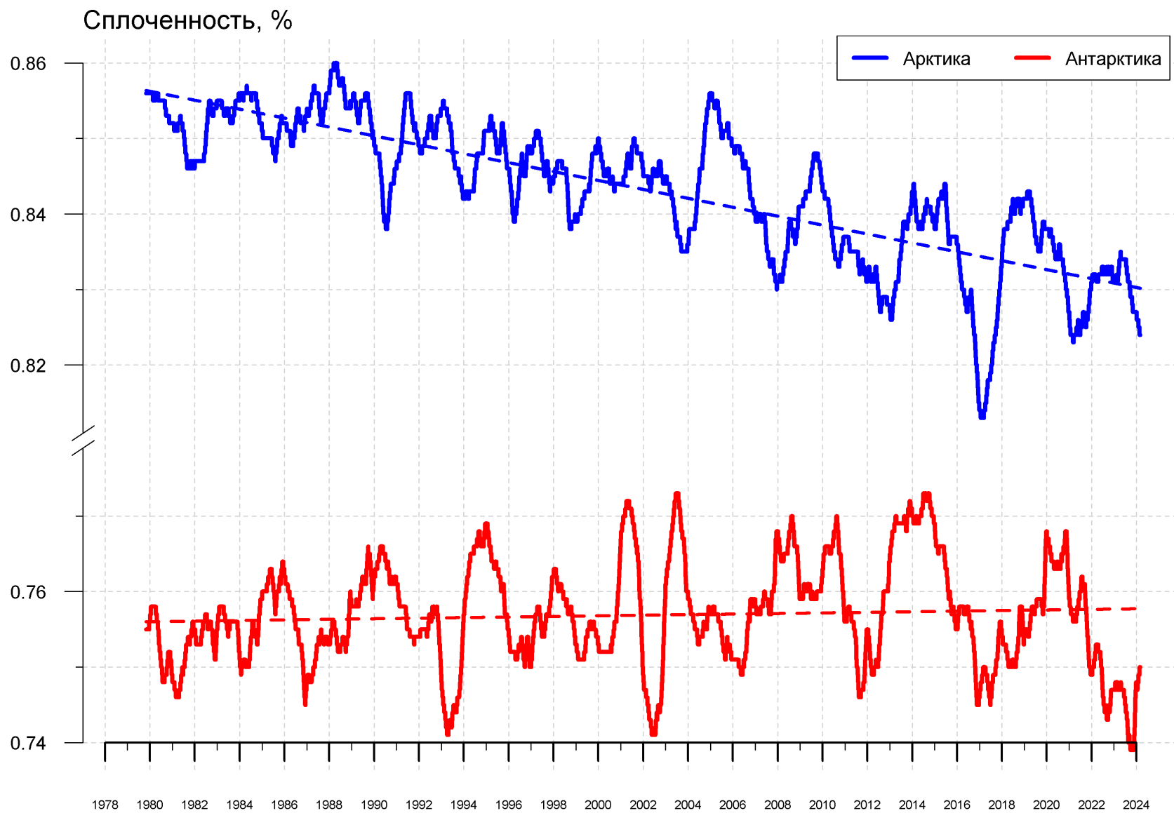
Рисунок 11 – Ежедневные сглаженные окном 365 суток значения средней общей сплоченности Арктики и Антарктики с 07.11.1978 по 03.03.2024 на основе SSMR-SSM/I-SSMIS
