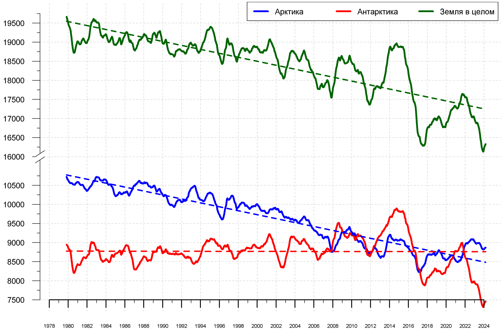
Рисунок 10 – Ежедневные сглаженные окном 365 суток значения приведенной ледовитости (площади морского льда) Арктики, Антарктики и Земли в целом с 26.10.1978 по 03.03.2024 на основе SSMR-SSM/I-SSMIS
