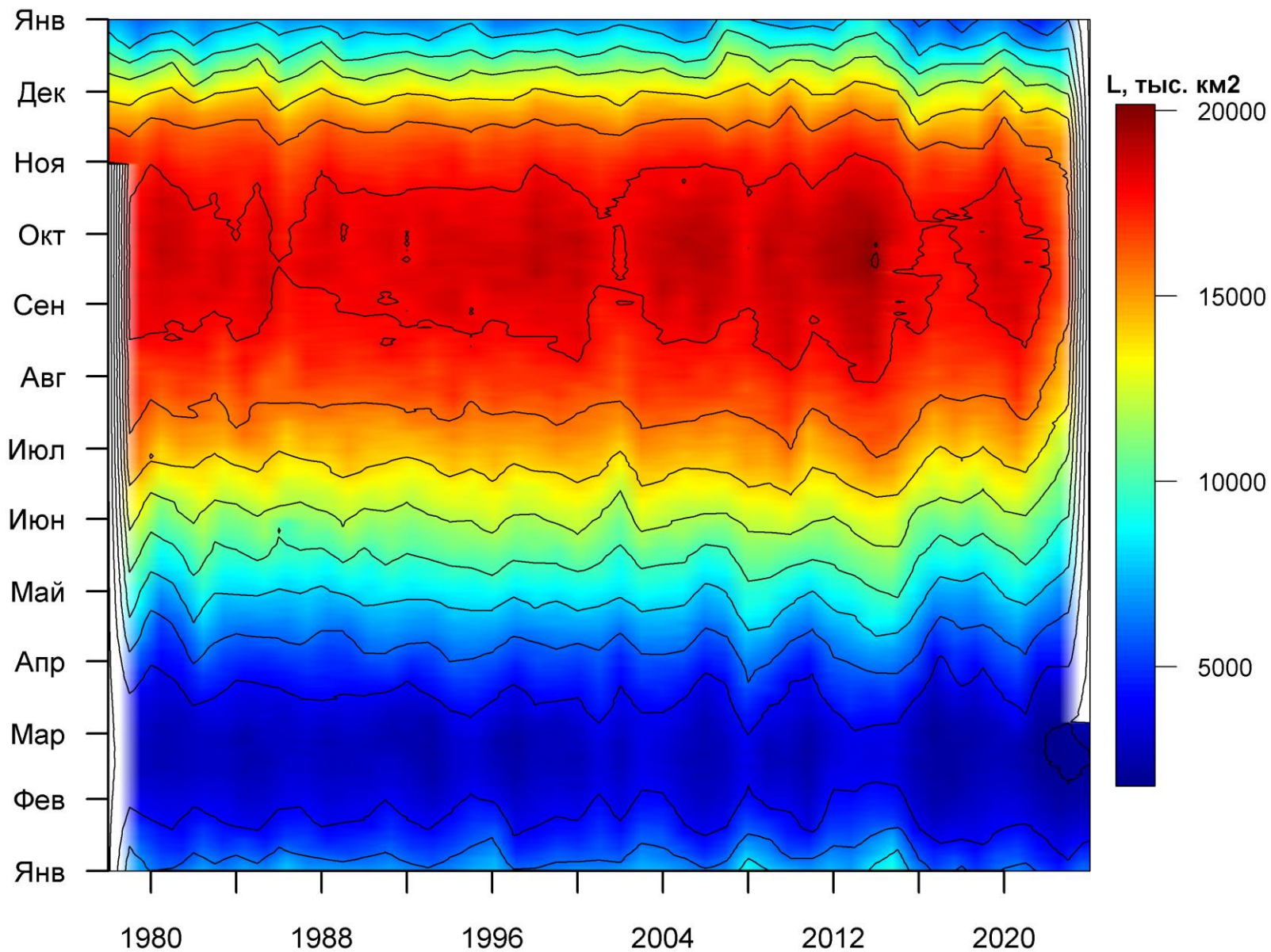
Рисунок 76 – Ежедневные оценки сезонных изменений ледовитости для Южного океана за период 26.10.1978 - 03.03.2024 на основе расчетов по данным SSMR-SSM/I-SSMIS, алгоритм NASATEAM.
