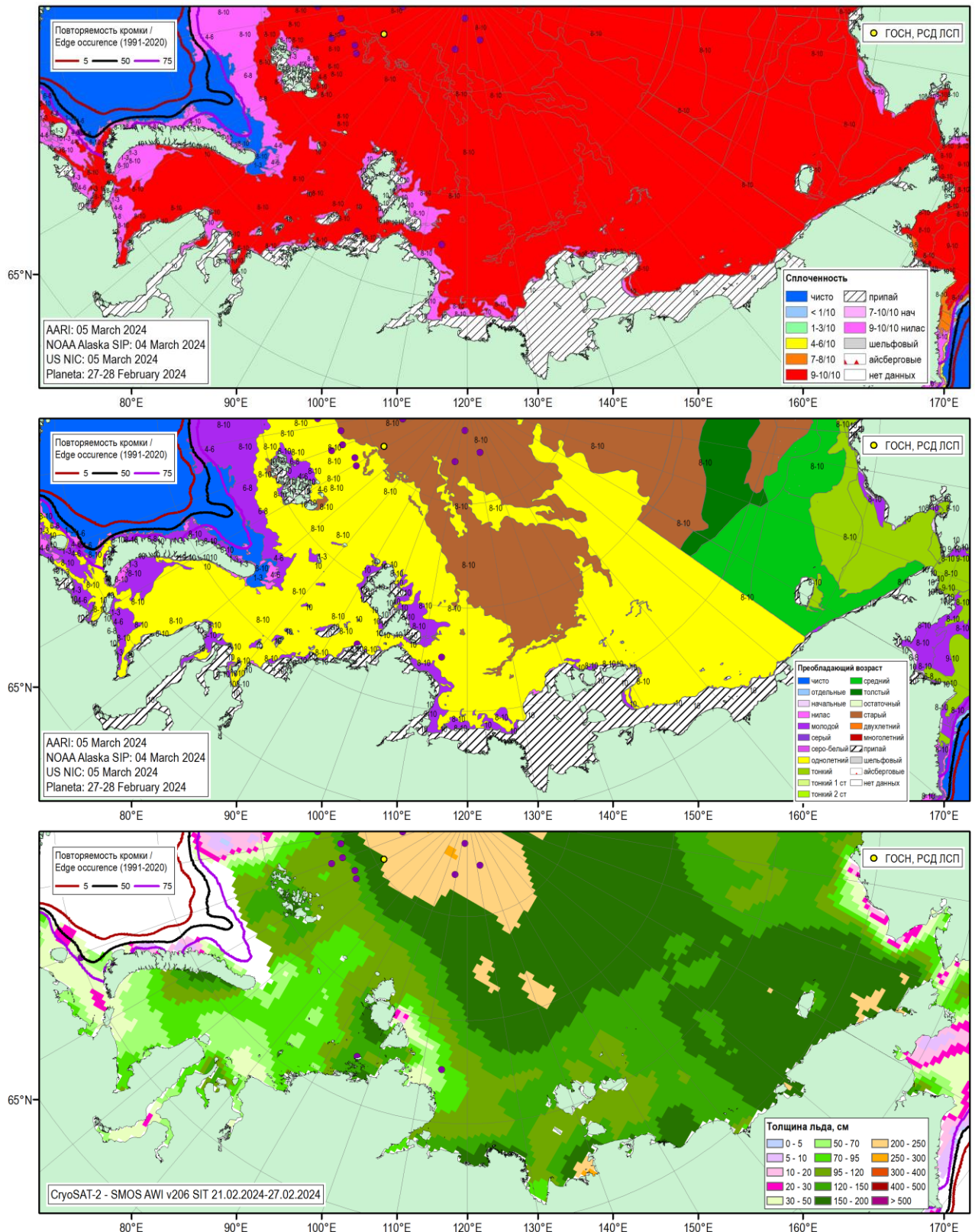
Рисунок 1д – Обзорная ледовая карта СМП за 05.03.2024 г. (цветовая раскраска по общей сплоченности – верх, по преобладающему возрасту - низ) на основе ледового анализа ААНИИ (05.03), NOAA Аляска (04.03), НИЦ Планета (26-28.02), Национального ледового центра США (01.03), оценка толщин льда по данным CryoSAT-2-SMOS AWI v206 за 21.02-27.02.2024 и повторяемость кромки за 01-05.03 за период 1991-2020гг. по наблюдениям SSMR-SSM/I-SSMIS (алгоритм NASATEAM), положение РСД ЛСП на 06.03.2024.
