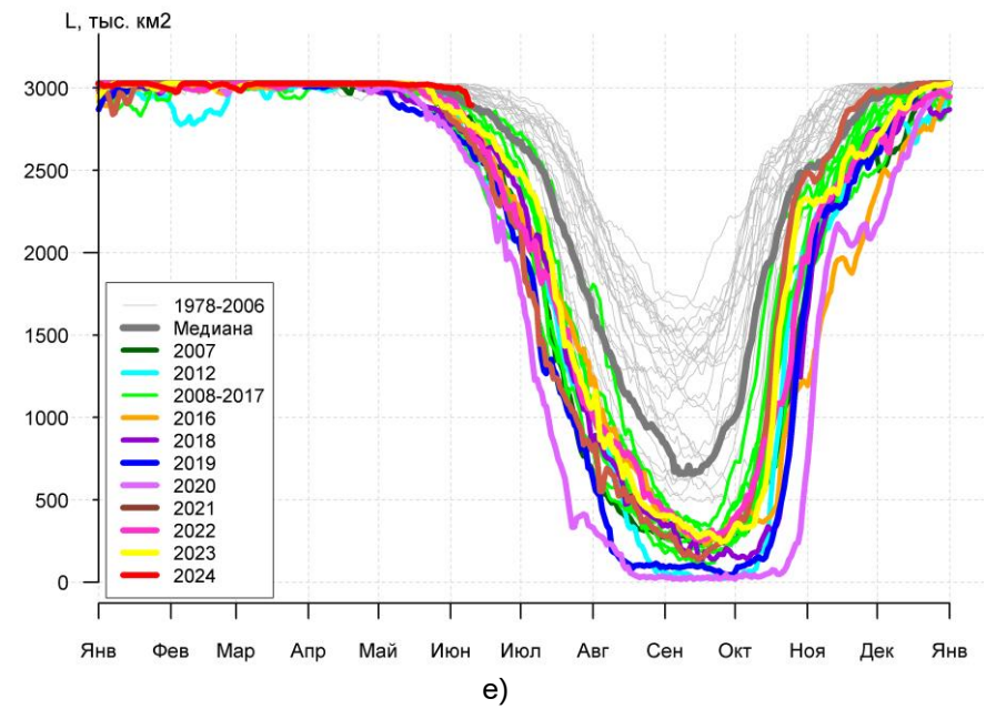
Рисунок 3а – Ежедневные оценки сезонного хода ледовитости для Северной Полярной Области и трех меридиональных секторов за период 26.10.1978 – 09.06.2024 по годам на основе расчетов по данным SSMR-SSM/I-SSMIS, алгоритмы NASATEAM: а) Северная полярная область, б) сектор 45°W-95°E (Гренландское – Карское моря), в) сектор 95°E-170°W (моря Лаптевых – Чукотское и Берингово, Охотское), г) сектор 170°W-45°W (море Бофорта и Канадская Арктика), д) Северный Ледовитый океан, е) Северный морской путь (Карское - Чукотское моря).
