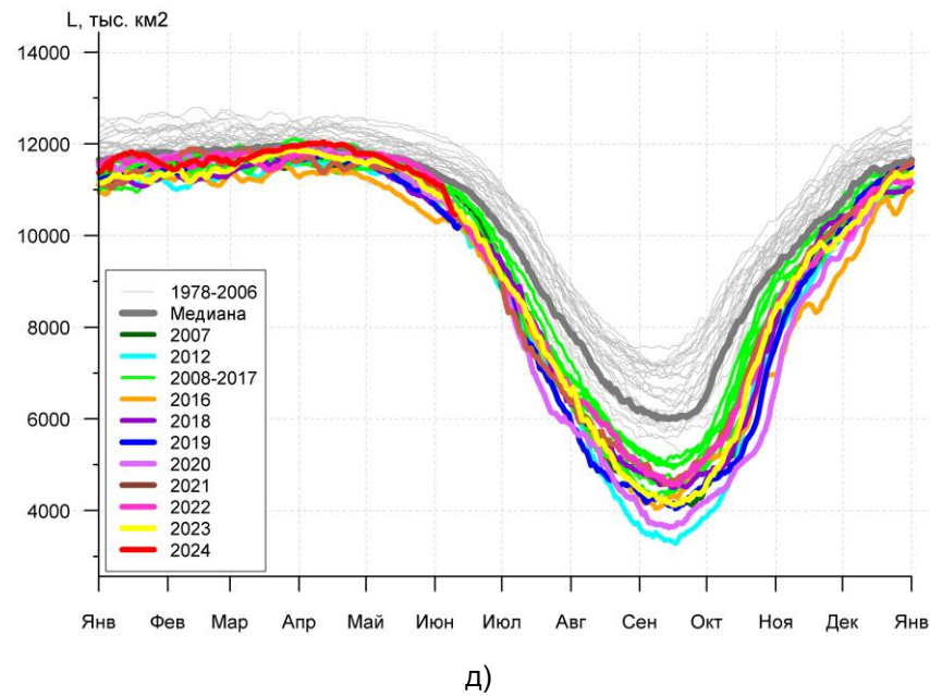
Рисунок 3а – Ежедневные оценки сезонного хода ледовитости для Северной Полярной Области и трех меридиональных секторов за период 26.10.1978 – 09.06.2024 по годам на основе расчетов по данным SSMR-SSM/I-SSMIS, алгоритмы NASATEAM: а) Северная полярная область, б) сектор 45°W-95°E (Гренландское – Карское моря), в) сектор 95°E-170°W (моря Лаптевых – Чукотское и Берингово, Охотское), г) сектор 170°W-45°W (море Бофорта и Канадская Арктика), д) Северный Ледовитый океан, е) Северный морской путь (Карское - Чукотское моря).
