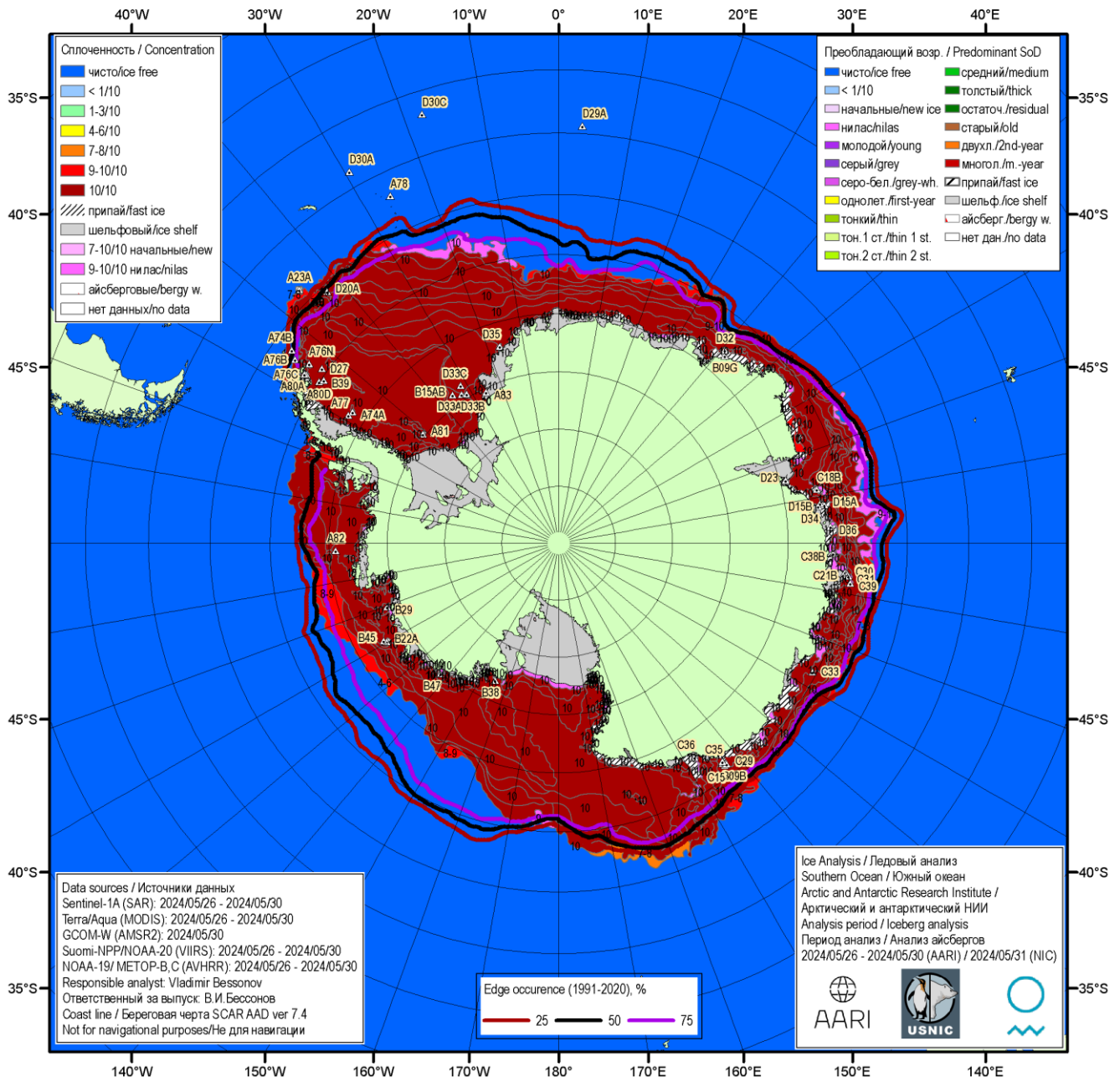
Рисунок 5а – Ледовая карта Южного океана (цветовая окраска по общей сплоченности) и расположение крупных айсбергов на основе ледового анализа за 30.05.2024 в рамках проекта совместного ледового картирования Южного океана ААНИИ, НЛЦ США и НМИ.
