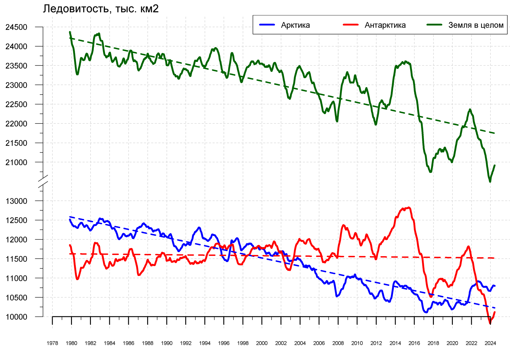
Рисунок 10 – Ежедневные сглаженные окном 365 суток значения приведенной ледовитости (площади морского льда) Арктики, Антарктики и Земли в целом с 26.10.1978 по 09.06.2024 на основе SSMR-SSM/I-SSMIS
