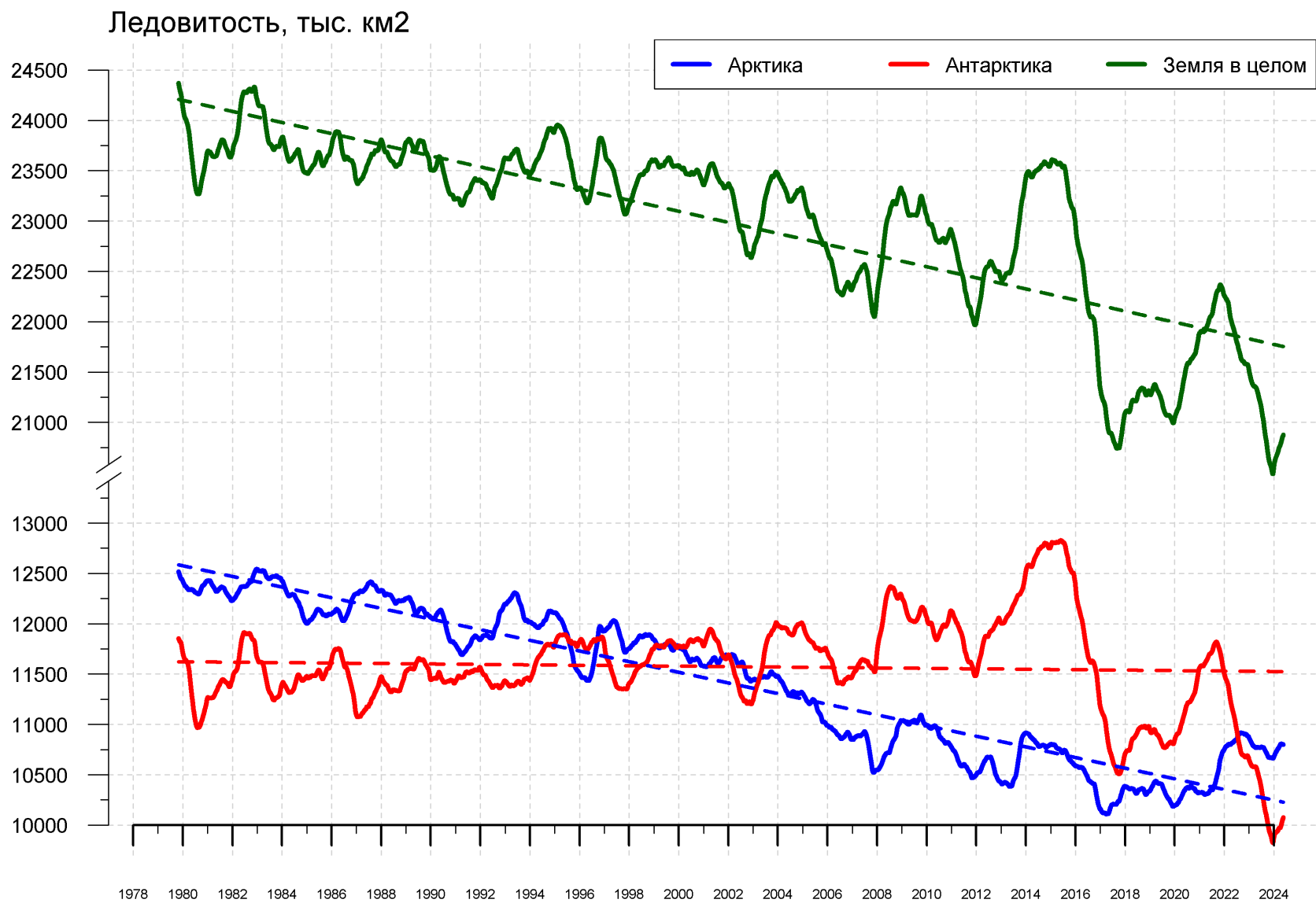
Рисунок 9 – Ежедневные сглаженные окном 365 суток значения ледовитости (площади распространения морского льда) Арктики, Антарктики и Земли в целом с 26.10.1978 по 09.06.2024 на основе SSMR-SSM/I-SSMIS
