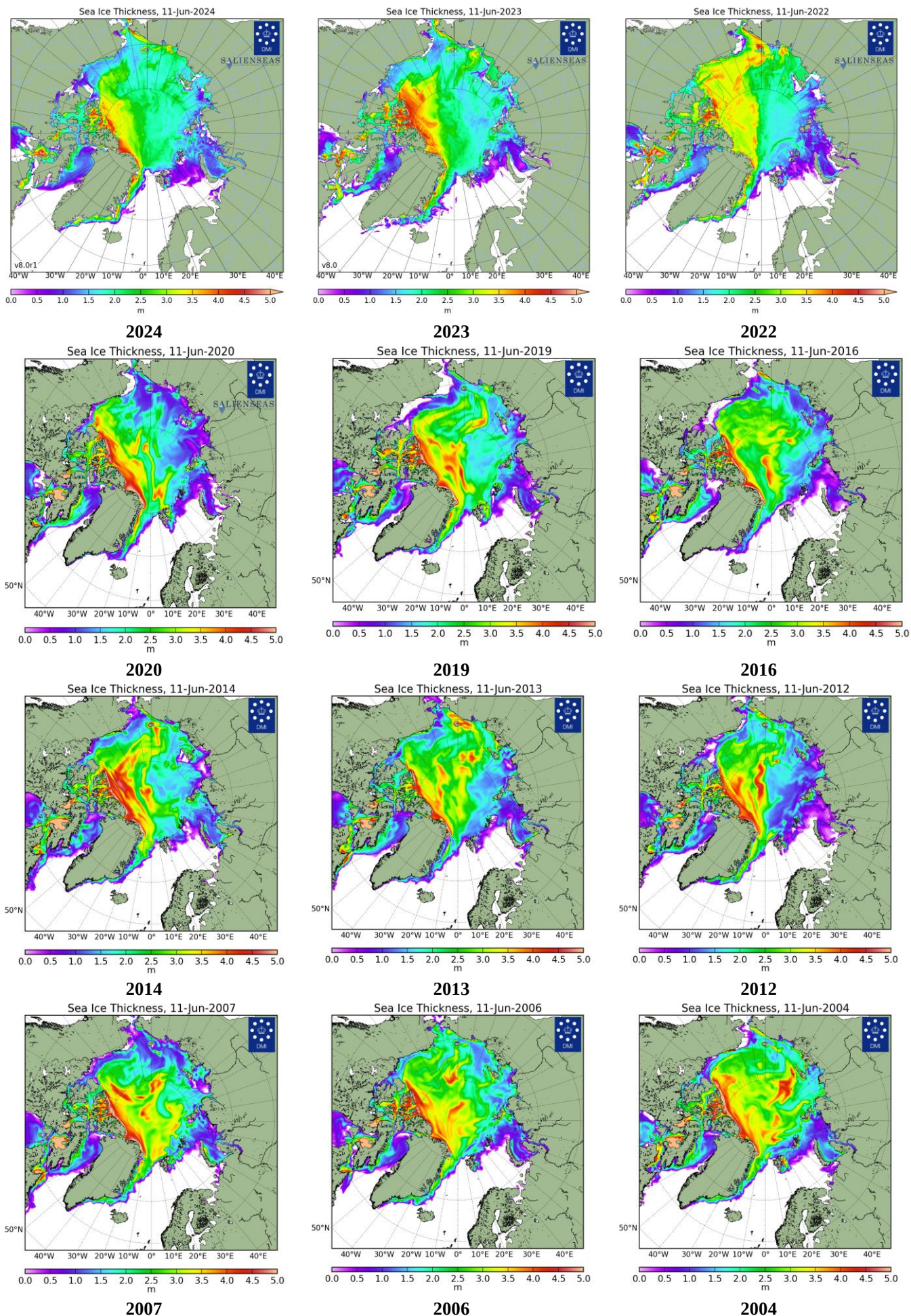
Рисунок 26 – Поля распределения средневзвешенной толщины льда совместной модели морского льда – океана HUSCOM/CICE Датского метеорологического института 11.06 за 2004-2024 гг.
