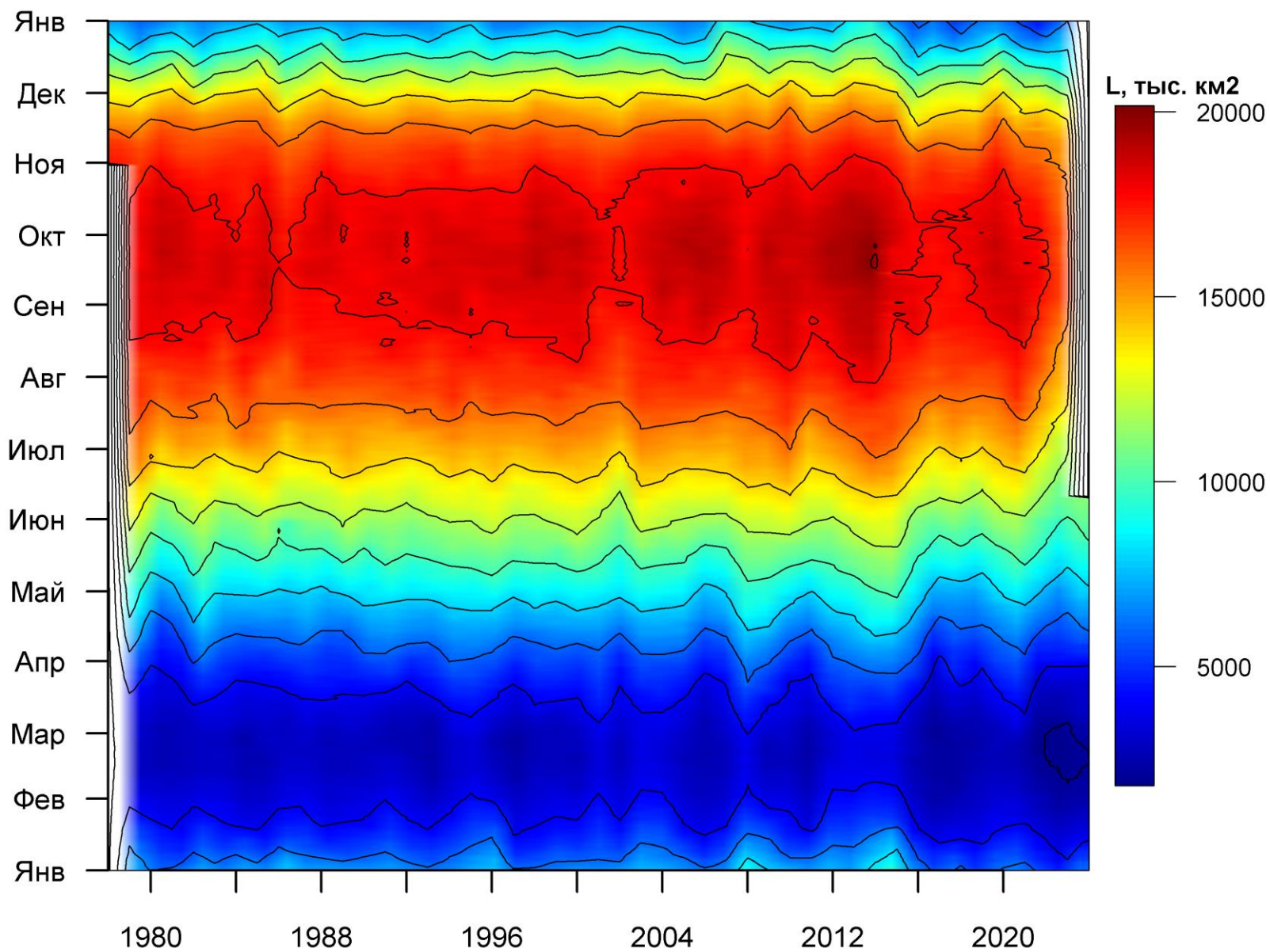
Рисунок 76 – Ежедневные оценки сезонных изменений ледовитости для Южного океана за период 26.10.1978 - 09.06.2024 на основе расчетов по данным SSMR-SSM/I-SSMIS, алгоритм NASATEAM.
