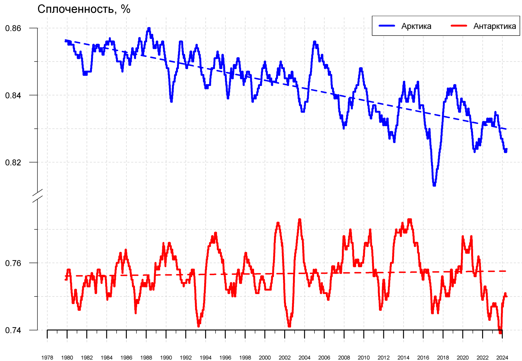
Рисунок 11 – Ежедневные сглаженные окном 365 суток значения средней общей сплоченности Арктики и Антарктики с 07.11.1978 по 09.06.2024 на основе SSMR-SSM/I-SSMIS
