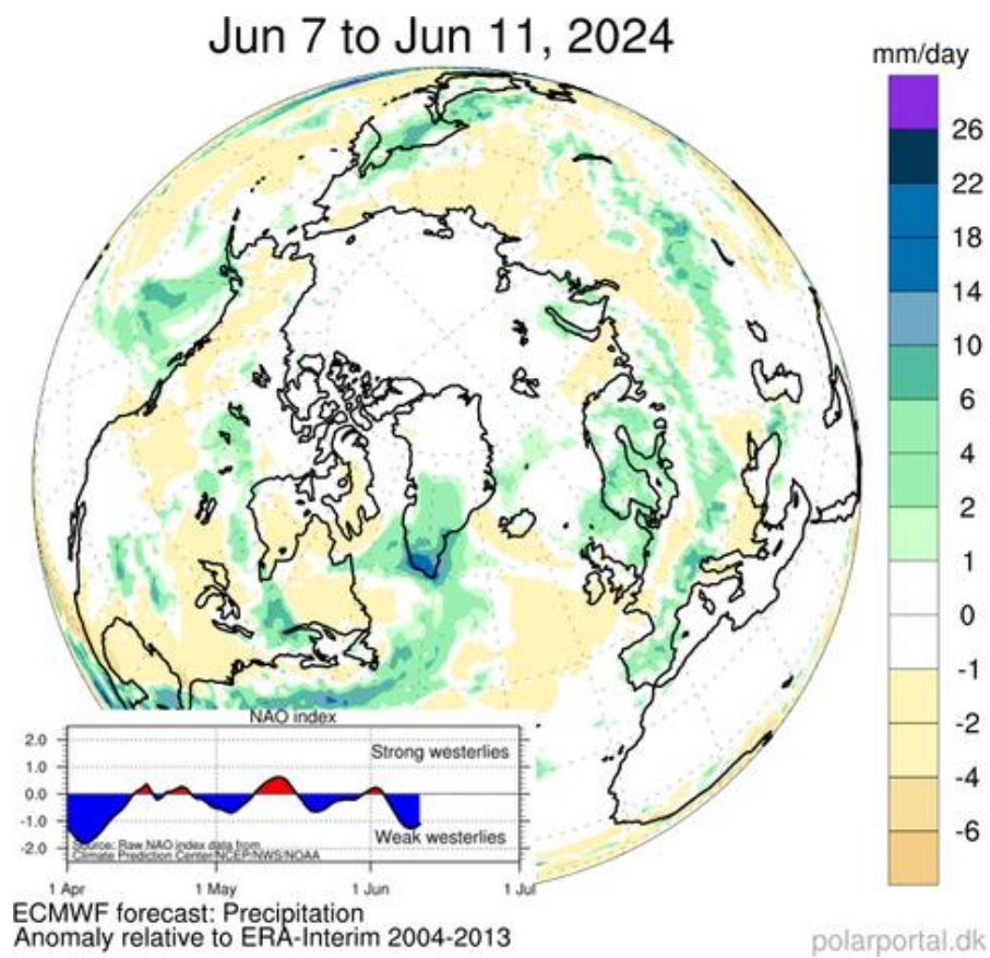
Рисунок 2ж – Аномалии приземной суммы осадков 07.06 – 11.06.2024 гг. относительно периода 2004-2013 гг. ( http://polarportal.dk )
