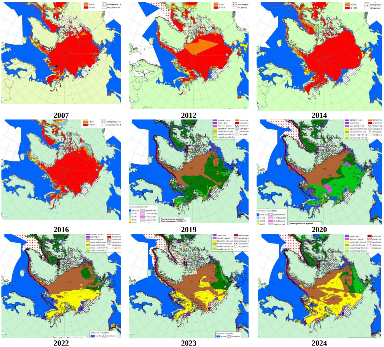
Рисунок 2а – Ледовые условия за 06.06-11.06.2024г. и аналогичные периоды 2007-2023 гг. на основе ледового анализа ААНИИ, НИЦ Планета, Канадской ледовой службы и Национального ледового центра США.
