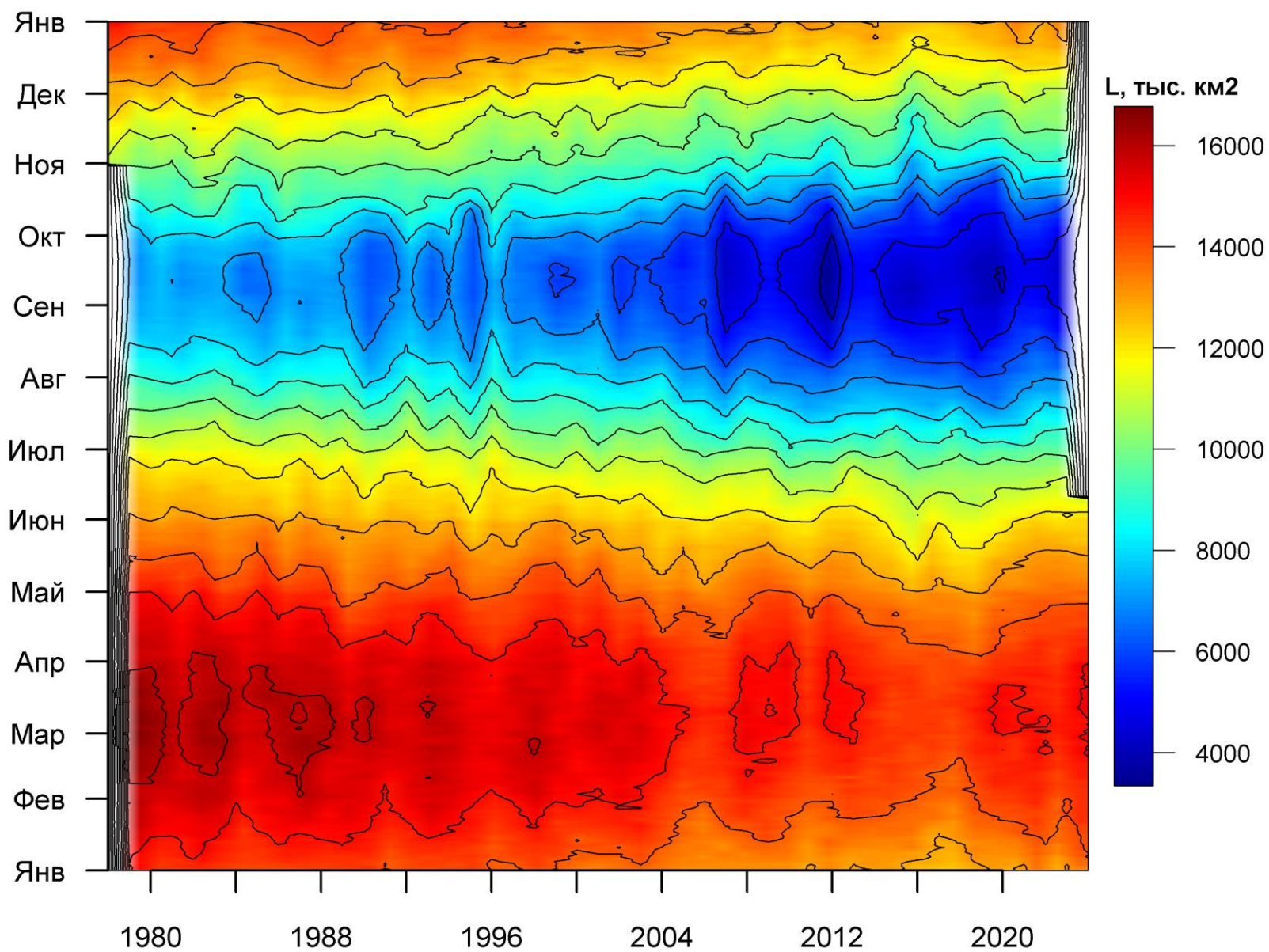
Рисунок 36 – Ежедневные оценки сезонных изменений ледовитости для Северной Полярной Области за период 26.10.1978 – 09.06.2024 на основе расчетов по данным SSMR-SSM/I-SSMIS, алгоритм NASATEAM.
