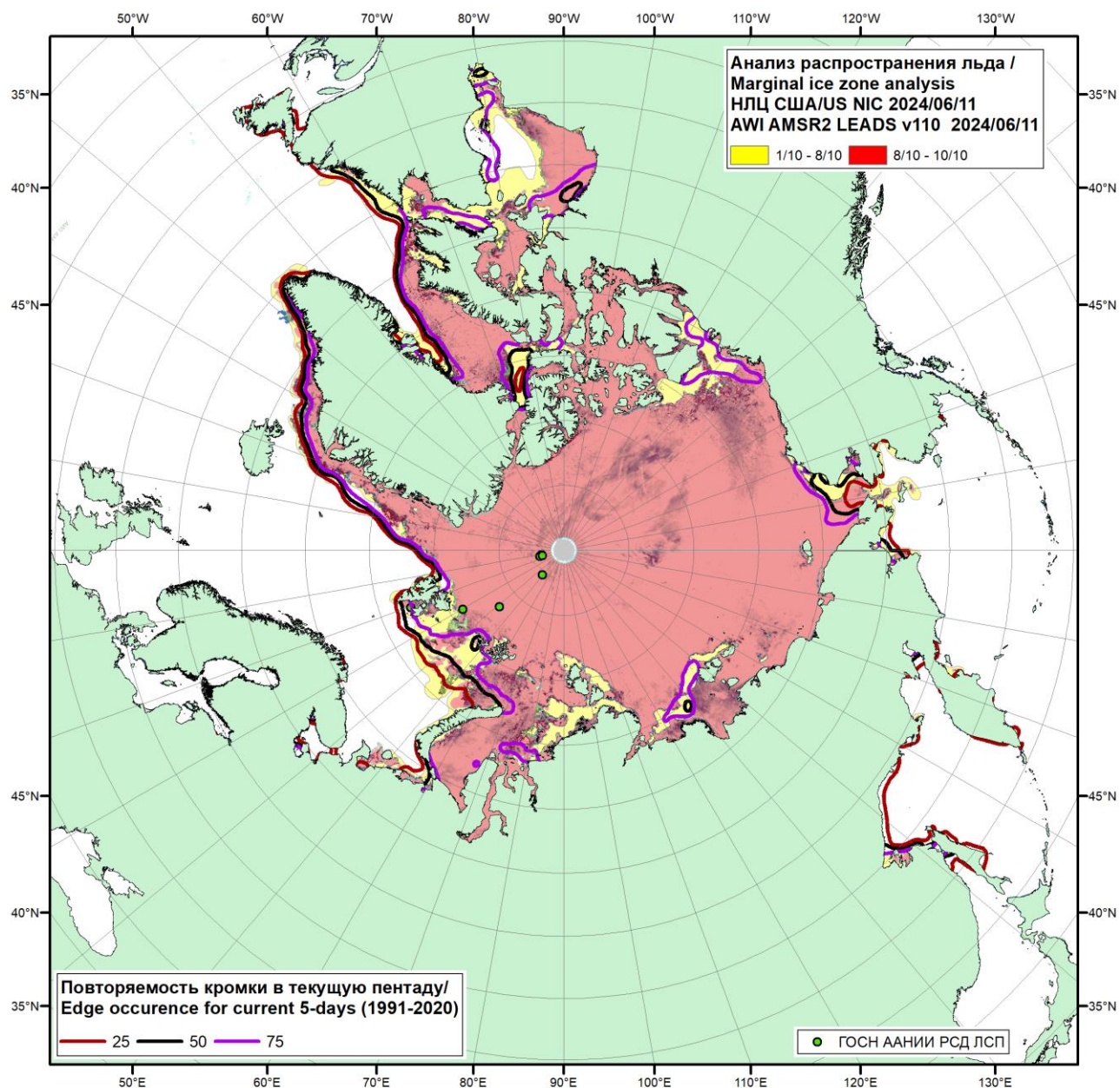
Рисунок 1г – Положение кромки льда и зон разреженных ( <8/10 ) и сплоченных ( \geq 8/10 ) льдов СЛО за 11.06.2024 г. на основе ледового анализа Национального Ледового Центра США и повторяемость кромки за 11-15.06 за период 1991-2020 гг. по наблюдениям SSMR-SSM/I-SSMIS (алгоритм NASATEAM), совмещенное с положением разрежений на основе данных ИСЗ AMSR2 11.06.2024 (AWI, v110) и положение РСД ЛСП на 11.06.2024.
