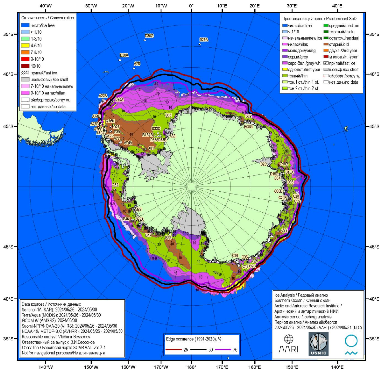
Рисунок 5в – Ледовая карта Южного океана (цветовая окраска по возрасту) и расположение крупных айсбергов на основе ледового анализа за 30.05.2024 в рамках проекта совместного ледового картирования Южного океана ААНИИ, НЛЦ США и НМИ.
