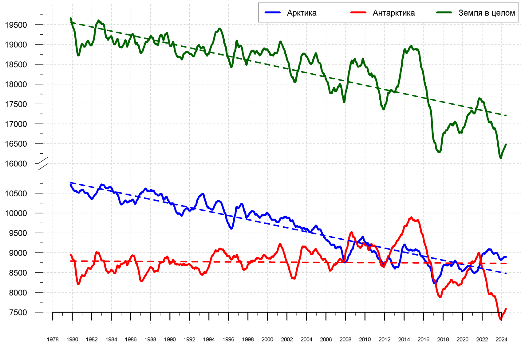
Рисунок 11 – Ежедневные сглаженные окном 365 суток значения средней общей сплоченности Арктики и Антарктики с 07.11.1978 по 09.06.2024 на основе SSMR-SSM/I-SSMIS
