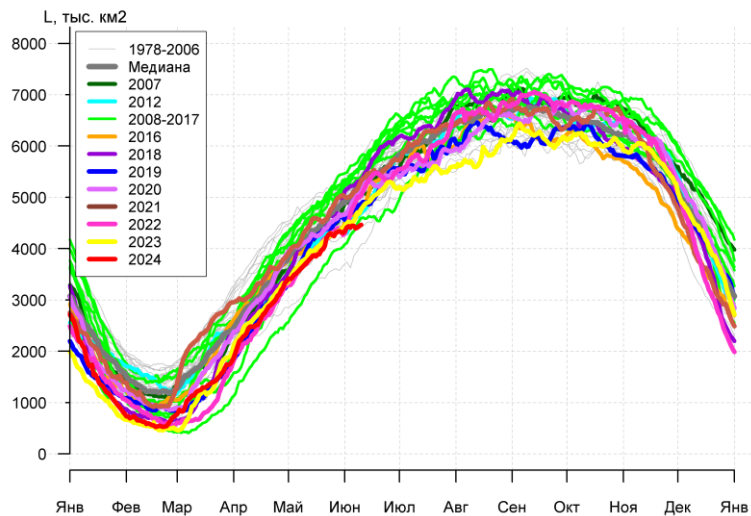
Рисунок 7а – Ежедневные оценки сезонного хода ледовитости Южного Океана и меридиональных секторов за период 26.10.1978 – 09.06.2024 по годам на основе расчетов по данным SSMR-SSM/I-SSMIS, алгоритм NASATEAM: а) Южный Океан, б) Атлантический сектор (60°W-30°E, море Уэдделла), в) Индоокеанский сектор (30°E-150°E, моря Космонавтов, Содружества, Моусона), г) Тихоокеанский сектор (150°E-60°W, моря Росса, Беллинсгаузена)
