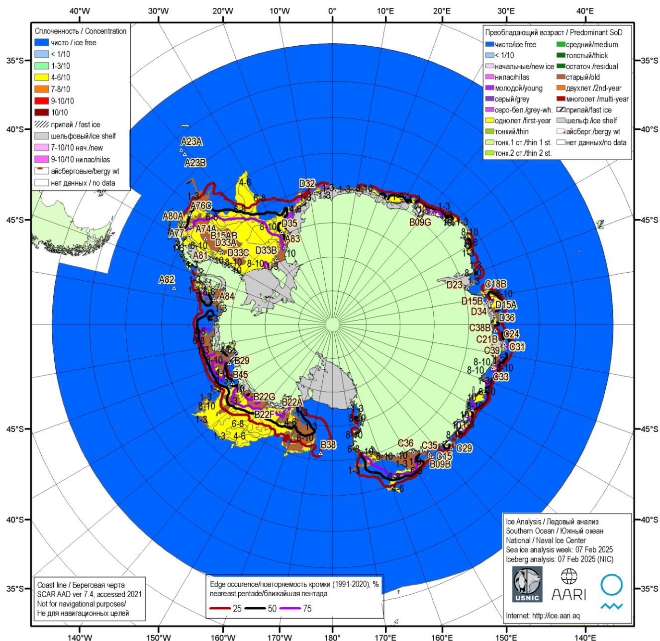
Рисунок 56 – Ледовая карта Южного океана (цветовая окраска по возрасту) и расположение крупных айсбергов на основе ледового анализа за 07.02.2025 в рамках проекта совместного ледового картирования Южного океана ААНИИ, НЛЦ США и НМИ и повторяемость кромки за 06-10.02 за период 1991-2020 гг. по наблюдениям SSMR-SSM/I-SSMIS (алгоритм NASATEAM)
