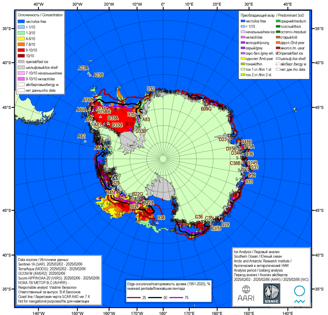
Рисунок 5а – Ледовая карта Южного океана (цветовая окраска по общей сплоченности) и расположение крупных айсбергов на основе ледового анализа за 07.02.2025 в рамках проекта совместного ледового картирования Южного океана ААНИИ, НЛЦ США и НМИ и повторяемость кромки за 06-10.02 за период 1991-2020 гг. по наблюдениям SSMR-SSM/I-SSMIS (алгоритм NASATEAM)
