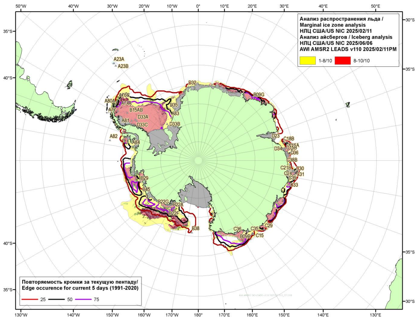
Рисунок 5в – Положение кромки льда и зон разреженных ( <8/10 ) и сплоченных ( \geq 8/10 ) льдов Южного океана за 11.02.2025 г. и расположение крупных айсбергов за 07.02.2025 на основе ледового анализа Национального Ледового Центра США, повторяемость кромки за 11-15.02 за период 1991-2020 гг. по наблюдениям SSMR-SSM/I-SSMIS (алгоритм NASATEAM), совмещенное с положением разрежений на основе данных ИСЗ AMSR2 за 11.02.2025 (AWI, v110).
