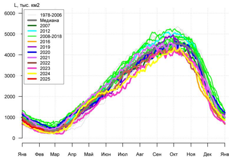
Рисунок 7а – Ежедневные оценки сезонного хода ледовитости Южного Океана и меридиональных секторов за период 26.10.1978 – 09.02.2025 по годам на основе расчетов по данным SSMR-SSM/I-SSMIS, алгоритм NASATEAM: а) Южный Океан, б) Атлантический сектор (60°W-30°E, море Уэдделла), в) Индоокеанский сектор (30°E-150°E, моря Космонавтов, Содружества, Моусона), г) Тихоокеанский сектор (150°E-60°W, моря Росса, Беллингаузена)
