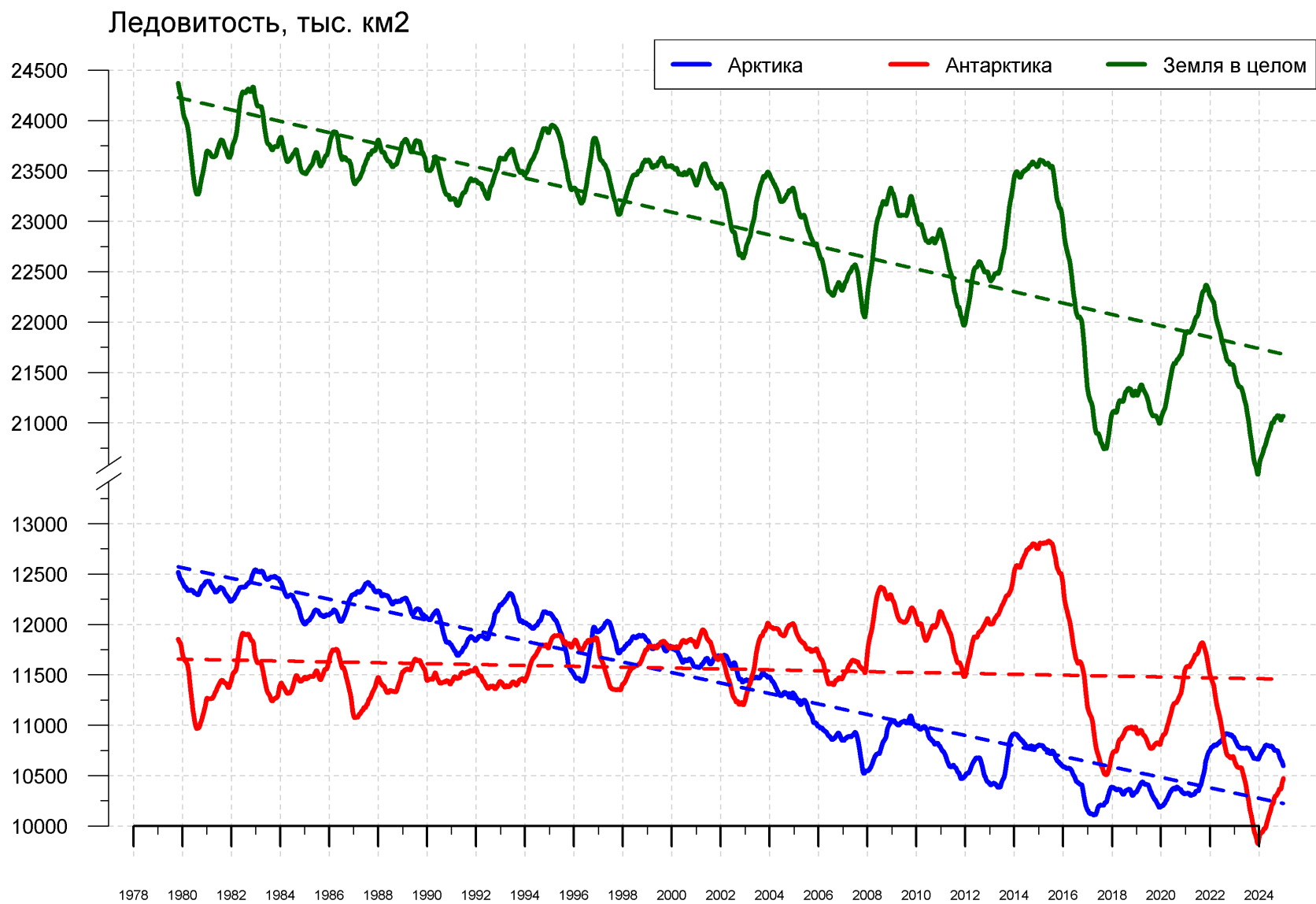
Рисунок 9 – Ежедневные сглаженные окном 365 суток значения ледовитости (площади распространения морского льда) Арктики, Антарктики и Земли в целом с 26.10.1978 по 09.02.2024 на основе SSMR-SSM/I-SSMIS
