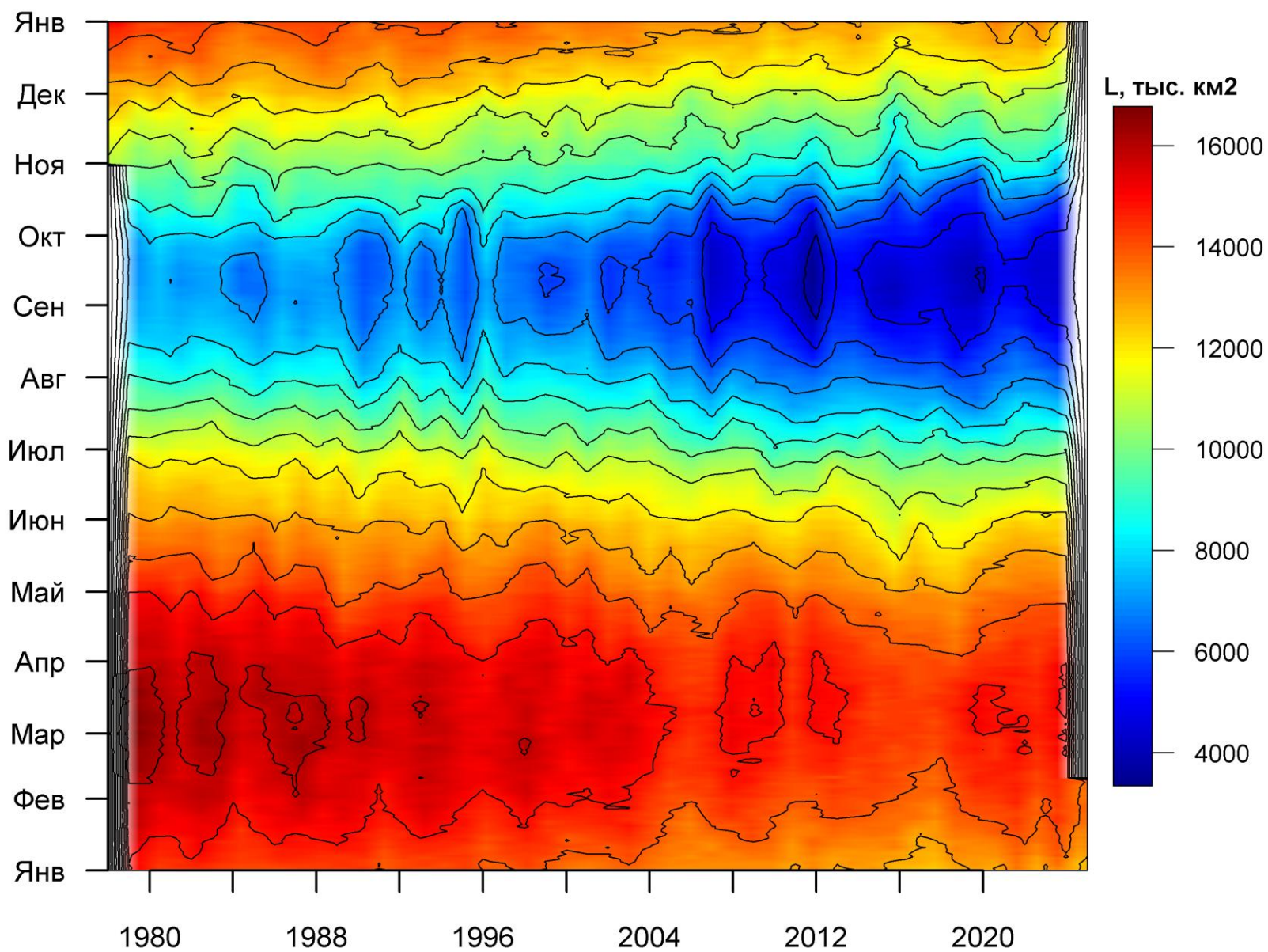
Рисунок 36 – Ежедневные оценки сезонных изменений ледовитости для Северной Полярной Области за период 26.10.1978 – 09.02.2025 на основе расчетов по данным SSMR-SSM/I-SSMIS, алгоритм NASATEAM.
