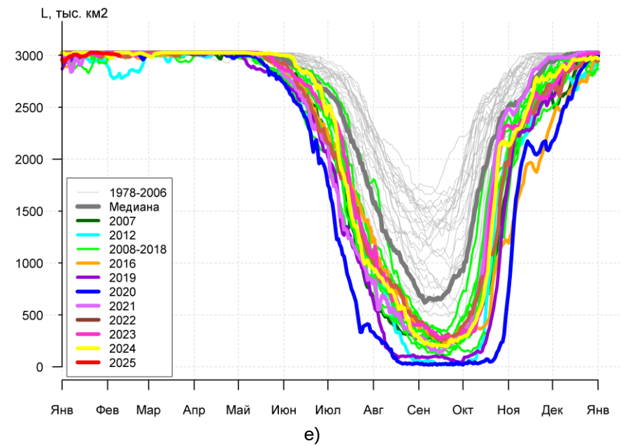
Рисунок 3а – Ежедневные оценки сезонного хода ледовитости для Северной Полярной Области и трех меридиональных секторов, СЛО и морей СМП за период 26.10.1978 – 09.02.2025 по годам на основе расчетов по данным SSMR-SSM/I-SSMIS, алгоритмы NASATEAM: а) Северная полярная область, б) сектор 45°W-95°E (Гренландское – Карское моря), в) сектор 95°E-170°W (моря Лаптевых – Чукотское и Берингово, Охотское), г) сектор 170°W-45°W (море Бофорта и Канадская Арктика), д) Северный Ледовитый океан, е) Северный морской путь (Карское - Чукотское моря).
