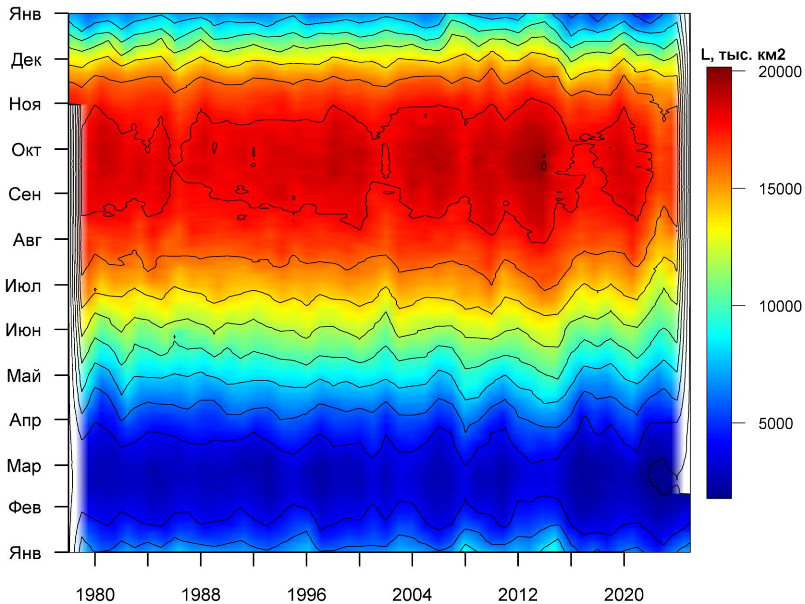
Рисунок 76 – Ежедневные оценки сезонных изменений ледовитости для Южного океана за период 26.10.1978 - 09.02.2025 на основе расчетов по данным SSMR-SSM/I-SSMIS, алгоритм NASATEAM.
