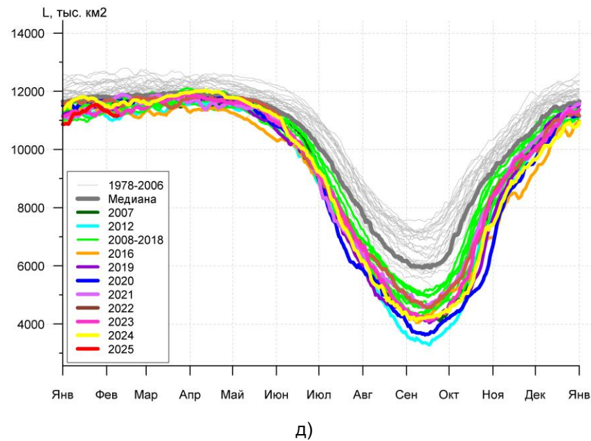
Рисунок 3а – Ежедневные оценки сезонного хода ледовитости для Северной Полярной Области и трех меридиональных секторов, СЛО и морей СМП за период 26.10.1978 – 09.02.2025 по годам на основе расчетов по данным SSMR-SSM/I-SSMIS, алгоритмы NASATEAM: а) Северная полярная область, б) сектор 45°W-95°E (Гренландское – Карское моря), в) сектор 95°E-170°W (моря Лаптевых – Чукотское и Берингово, Охотское), г) сектор 170°W-45°W (море Бофорта и Канадская Арктика), д) Северный Ледовитый океан, е) Северный морской путь (Карское - Чукотское моря).
