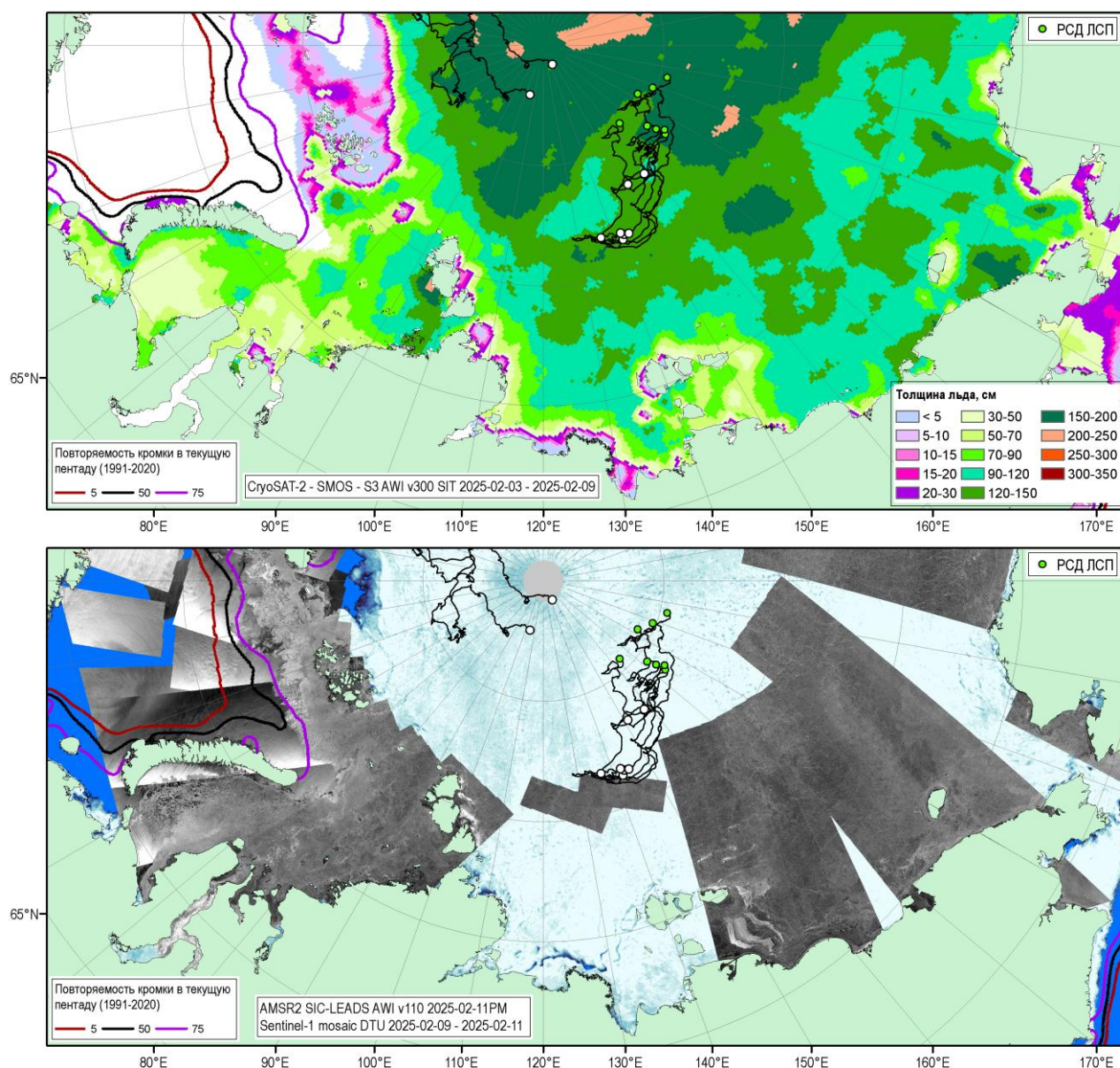
Рисунок 1е - Оценка толщины льда на акватории СМП на основе данных ИСЗ CryoSat-2-SMOS-S3 за 03.02.2025-09.02.2025 (AWI, ver.300), мозаика радиолокационных снимком ИСЗ Sentinel-1A за 09-11.02.2025 (DTU), оценка положения полыней на основе данных AMSR2 (AWI v110) за 11.02.2025, повторяемость кромки за 06-10/11-15.02 за период 1991-2020 гг. по наблюдениям SSMR-SSM/I-SSMIS (алгоритм NASATEAM) и положение РСН СП-42 на 08МСК 12.02.2025
