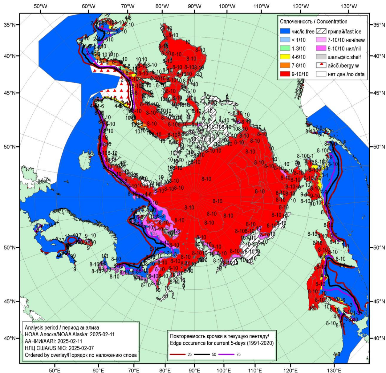
Рисунок 1а – Обзорная ледовая карта СЛО за 2025.02.07 – 2025.02.11 г. (цветовая раскраска по общей сплоченности) на основе ледового анализа NOAA Аляска (11.02.2025), ААНИИ (11.03.2025), Национального ледового центра США (07.02.2025) и повторяемость кромки за 11-15.02 за период 1991-2020 гг. по наблюдениям SSMR-SSM/I-SSMIS (алгоритм NASATEAM).
