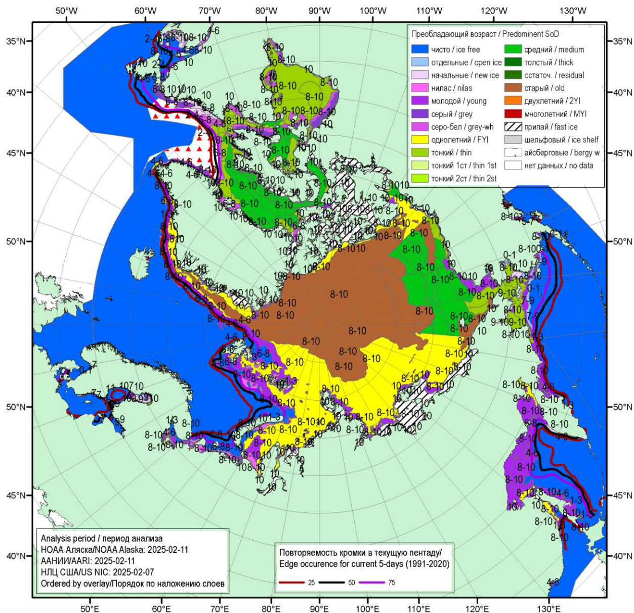
Рисунок 16 – Обзорная ледовая карта СЛО за 2025.02.07 – 2025.02.11 г. (цветовая раскраска по преобладающему возрасту) на основе ледового анализа NOAA Аляска (11.02.2025), ААНИИ (11.02.2025), Национального ледового центра США (07.02.2025) и повторяемость кромки за 11-15.02 за период 1991-2020 гг. по наблюдениям SSMR-SSM/I-SSMIS (алгоритм NASATEAM).
