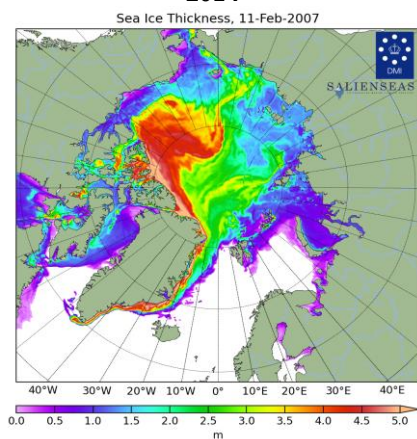
Рисунок 26 – Поля распределения средневзвешенной толщины льда совместной модели морского льда – океана HYCOM/CICE Датского метеорологического института 11.02 за 2005-2025 гг.
