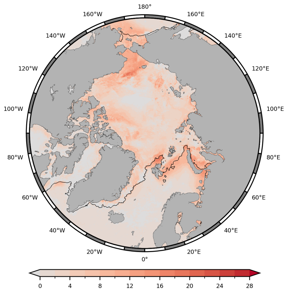
Рисунок 2в – Аномалия температуры поверхности морского льда и океана (к периоду 1991-2020 гг.) Датского метеорологического института за 09-11.02.2025 гг. ( http://polarportal.dk/en/sea-ice-and-icebergs/sea-ice-temperature/#c8099 )
