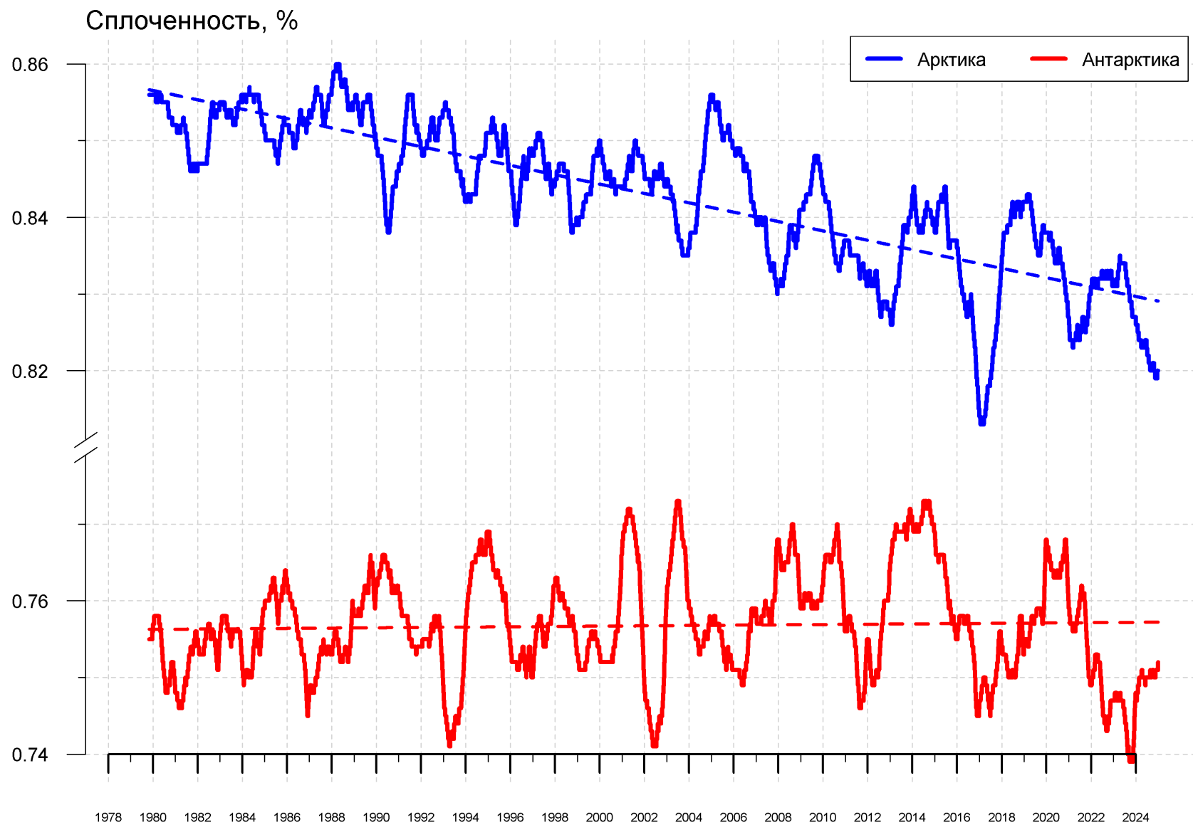
Рисунок 11 – Ежедневные сглаженные окном 365 суток значения средней общей сплоченности Арктики и Антарктики с 07.11.1978 по 09.02.2024 на основе SSMR-SSM/I-SSMIS
