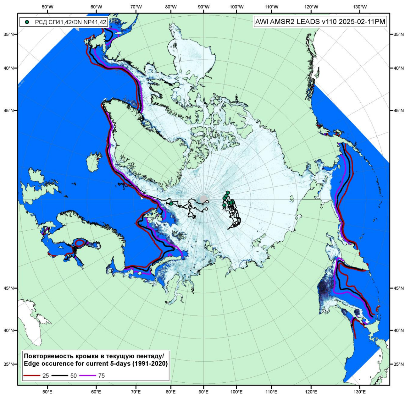
Рисунок 1г – Положение разрежений на основе данных ИСЗ AMSR2 2025-02-11PM (AWI, v110), повторяемость кромки за 11-15.02 за период 1991-2020 гг. по наблюдениям SSMR-SSM/I-SSMIS (алгоритм NASATEAM) и положение РСН СП-42 на 12.02.2025 г. 08:00МСК.
