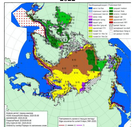
Рисунок 1ж – Ледовые условия за 02.05 - 06.05.2025. и аналогичные периоды 2007-2024 гг. на основе ледового анализа ААНИИ, НИЦ Планета, Канадской ледовой службы, Национального ледового центра США и НОАА Аляска [4, 10, 12, 23, 17].
