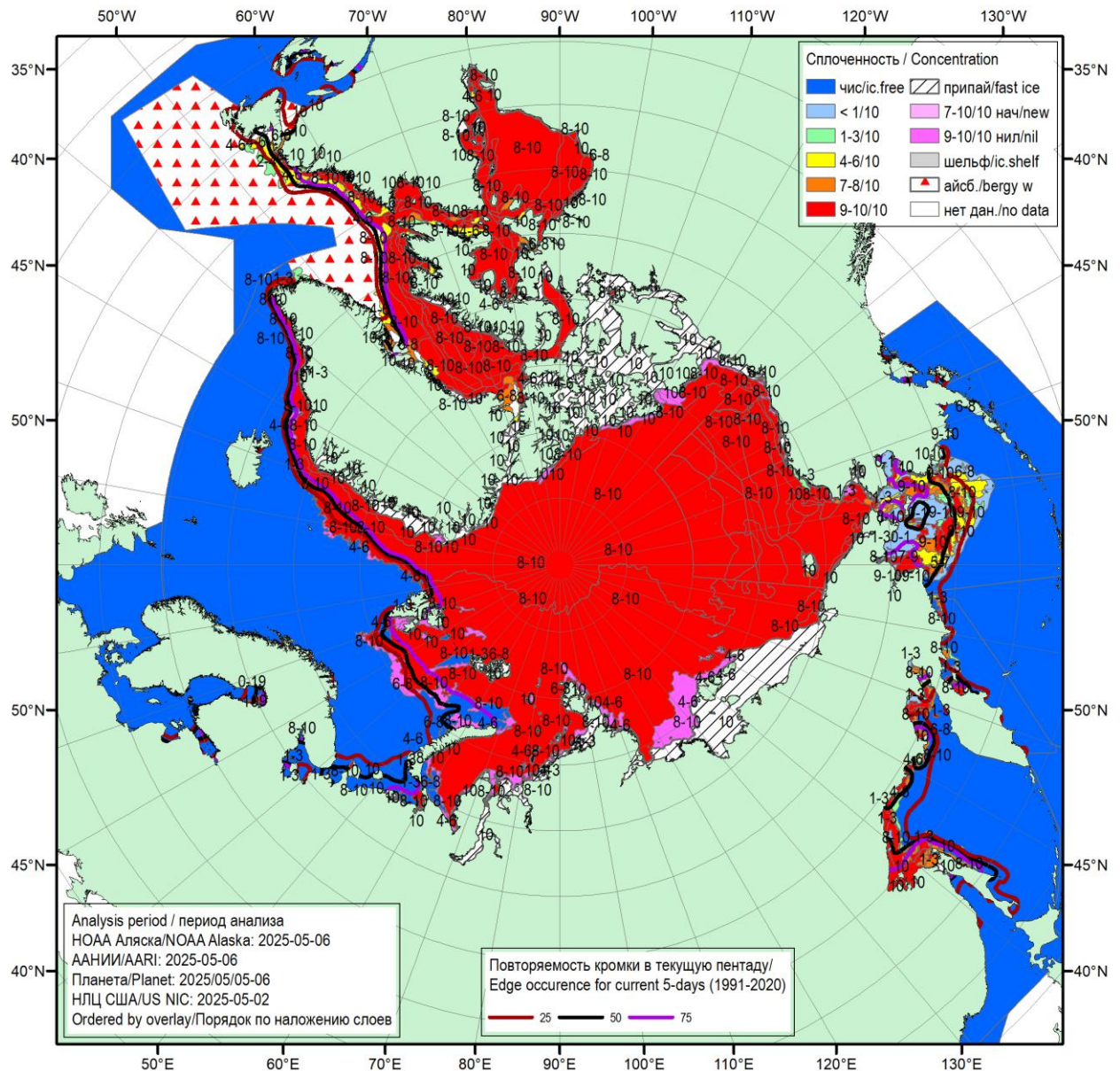
Рисунок 1а – Обзорная ледовая карта СЛО за 02.05.2025 – 06.05.2025 (цветовая раскраска по общей сплоченности) на основе ледового анализа NOAA Аляска (06.05.2025), ААНИИ (06.05.2025), НИЦ Планета (05-06.05.2025), Национального ледового центра США (02.05.2025) и повторяемость кромки за ближайшую пентаду за период 1991-2020 гг. по наблюдениям SSMR-SSM/I-SSMIS (алгоритм NASATEAM) [4, 10, 23, 17].
