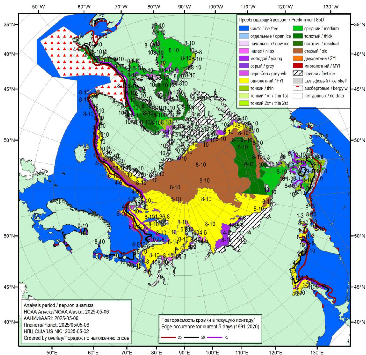
Рисунок 16 – Обзорная ледовая карта СЛО за 02.05.2025 – 06.05.2025 (цветовая раскраска по преобладающему возрасту) на основе ледового анализа НОАА Аляска (06.05.2025), АНИИ (06.05.2025), НИЦ Планета (05-06.05.2025), Национального ледового центра США (02.05.2025) и повторяемость кромки за ближайшую пентаду за период 1991-2020 гг. по наблюдениям SSMR-SSM/I-SSMIS (алгоритм NASATEAM) [4, 10, 23, 17].
