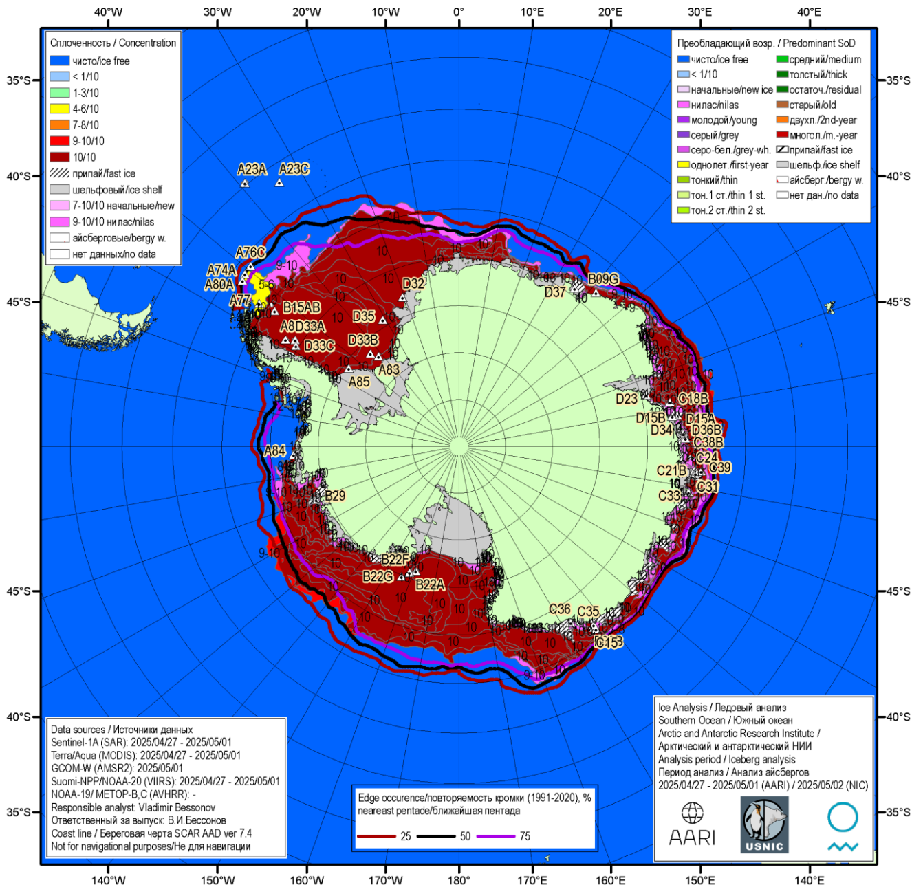
Рисунок 5а – Ледовая карта Южного океана (цветовая окраска по общей сплоченности) и расположение крупных айсбергов на основе ледового анализа за 01.05.2025 в рамках проекта совместного ледового картирования Южного океана ААНИИ, НЛЦ США и НМИ и повторяемость кромки за ближайшую пентаду за период 1991-2020 гг. по наблюдениям SSMR-SSM/I-SSMIS (алгоритм NASATEAM) [5, 10, 17, 21]
