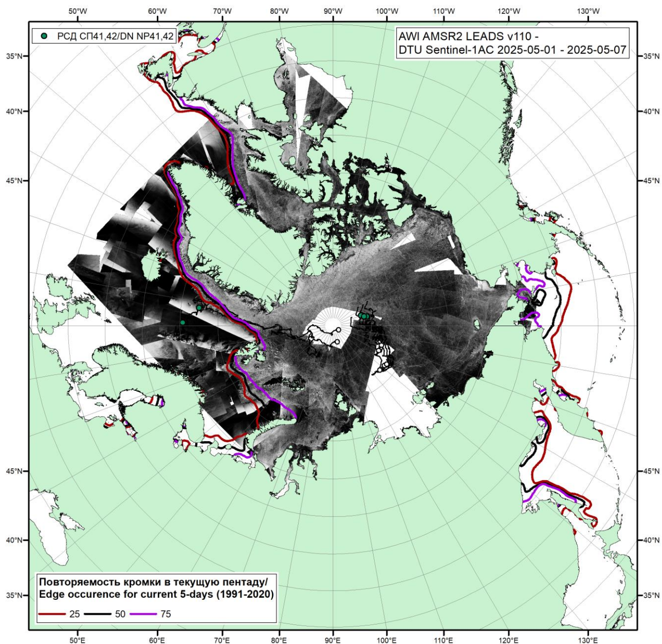
Рисунок 1г – Мозаика радиолокационных снимком ИСЗ Sentinel-1AC за 01.05-07.05.2025 г (DTU), повторяемость кромки за ближайшую пентаду 1991-2020 гг. по наблюдениям SSMR-SSM/I-SSMIS (алгоритм NASATEAM) и положение РСН СП-42 на 07.05.2025 г. 08:00МСК.
