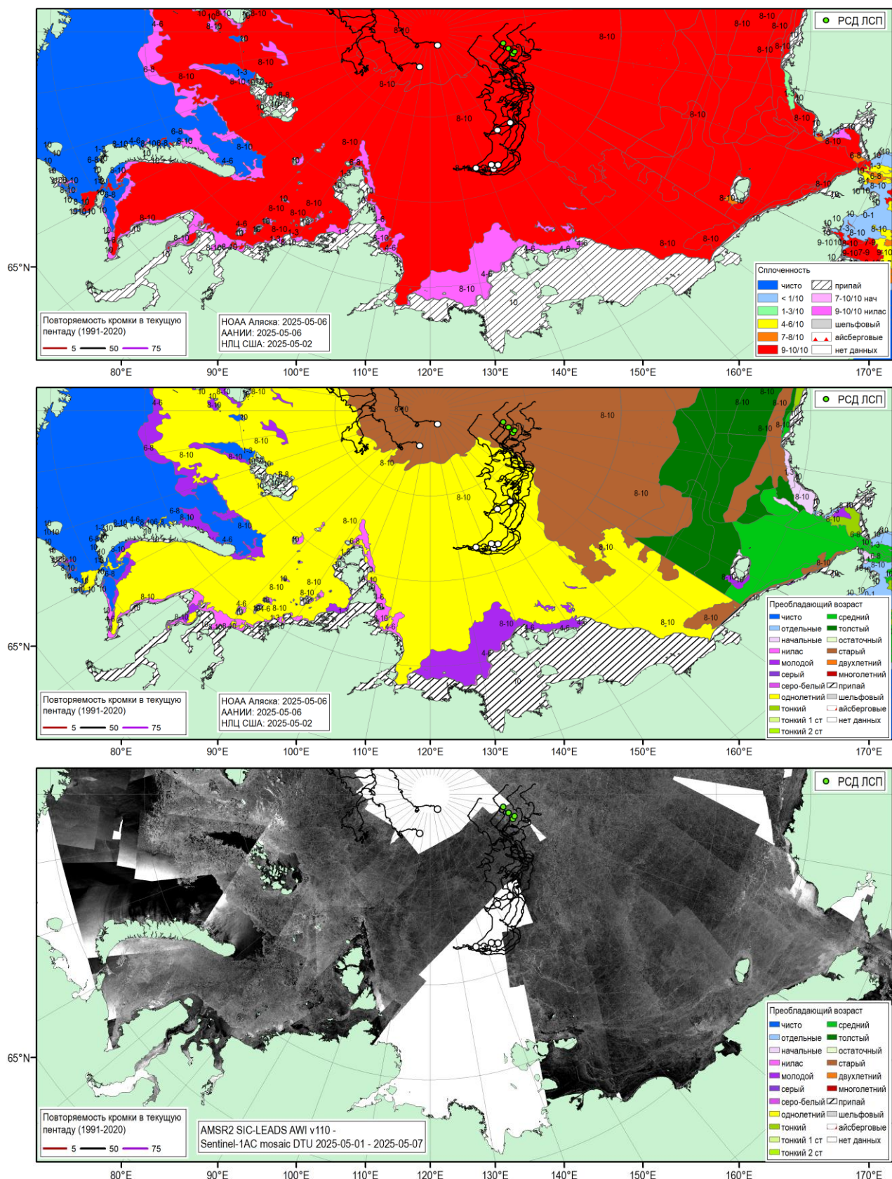
Рисунок 1д – Обзорная ледовая карта СМП за 06.05.2025 г. на основе ледового анализа НОАА Аляска (06.05.2025), ААНИИ (06.05.2025), мозаика радиолокационных снимком ИСЗ Sentinel-1AC за 01.05-07.05.2025 (DTU), повторяемость кромки за ближайшую пентаду 1991-2020 гг. по наблюдениям SSMR-SSM/I-SSMIS (алгоритм NASATEAM) и положение РСН СП-42 на 08МСК 07.05.2025 [27, 28, 17].
