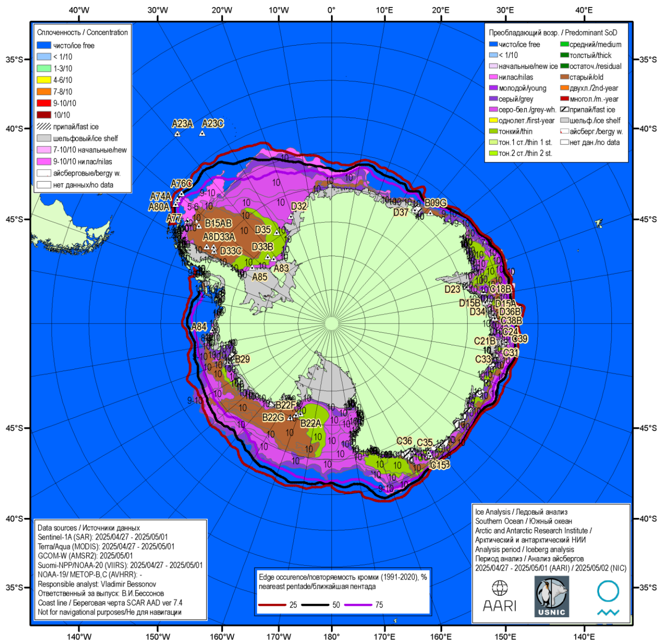
Рисунок 56 – Ледовая карта Южного океана (цветовая окраска по возрасту) и расположение крупных айсбергов на основе ледового анализа за 01.05.2025 в рамках проекта совместного ледового картирования Южного океана ААНИИ, НЛЦ США и НМИ и повторяемость кромки за ближайшую пентаду за период 1991-2020 гг. по наблюдениям SSMR-SSM/I-SSMIS (алгоритм NASATEAM) [5, 10, 17, 21].
