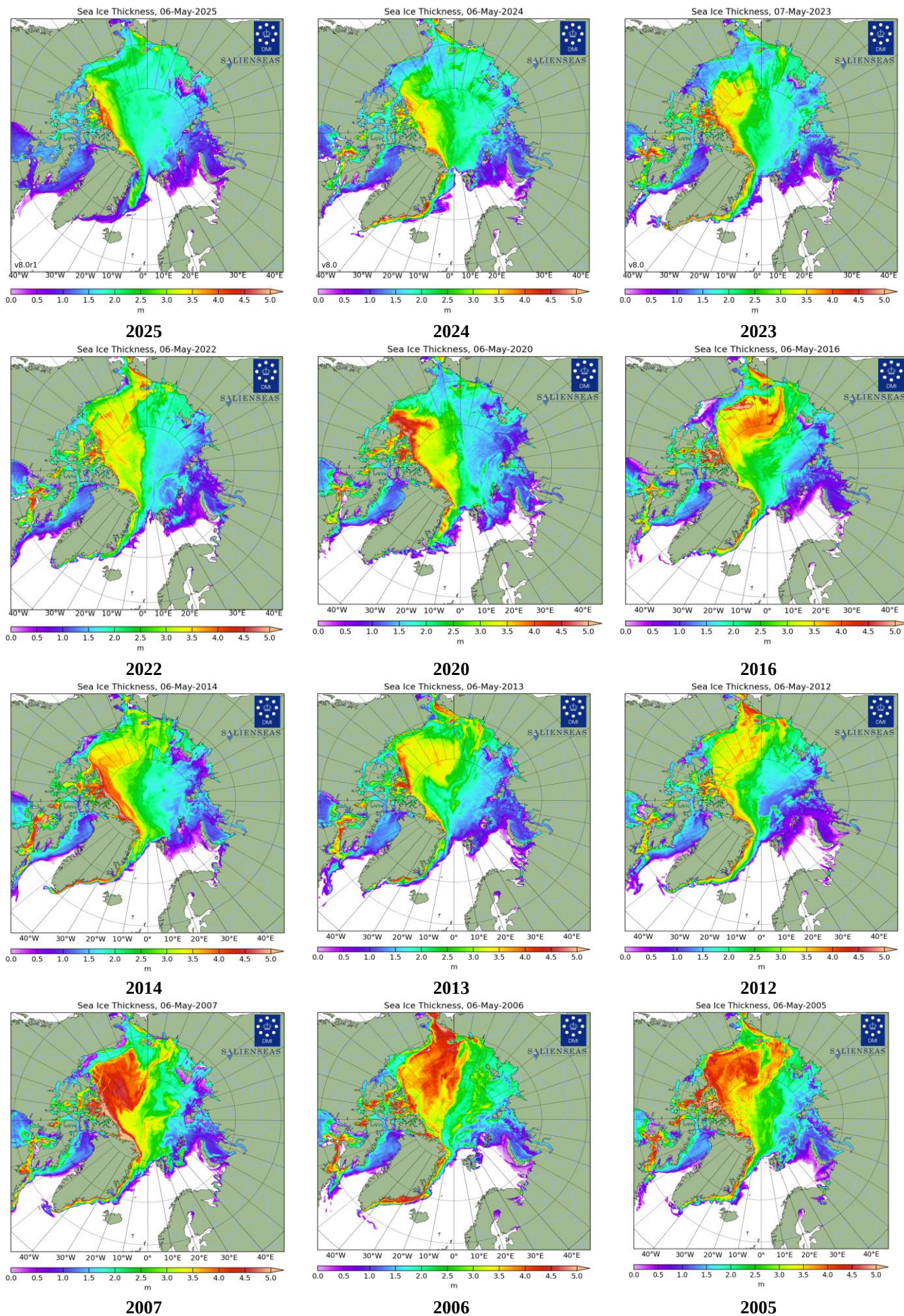
Рисунок 26 – Поля распределения средневзвешенной толщины льда совместной модели морского льда – океана HYCOM/CICE Датского метеорологического института 06.05 за 2005-2025 гг. [22].
