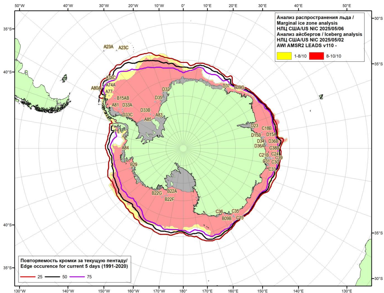
Рисунок 5в – Положение кромки льда и зон разреженных ( <8/10 ) и сплоченных ( \geq 8/10 ) льдов Южного океана за 06.05.2025 г. и расположение крупных айсбергов за 02.05.2025 на основе ледового анализа Национального Ледового Центра США, повторяемость кромки за ближайшую пентаду за период 1991-2020 гг. по наблюдениям SSMR-SSM/I-SSMIS (алгоритм NASATEAM), совмещенное с положением разрежений на основе данных ИСЗ AMSR2 за 29.04.2025 (AWI, v110) [10, 17, 24]
