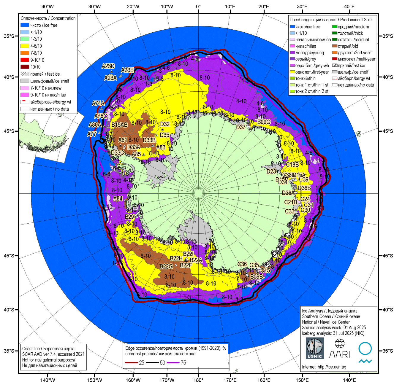
Рисунок 56 – Ледовая карта Южного океана (цветовая окраска по возрасту) и расположение крупных айсбергов на основе ледового анализа за 01.08.2025 в рамках проекта совместного ледового картирования Южного океана ААНИИ, НЛЦ США и НМИ и повторяемость кромки за ближайшую пентаду за период 1991-2020 гг. по наблюдениям SSMR-SSM/I-SSMIS (алгоритм NASATEAM) [5, 10, 17, 21].
