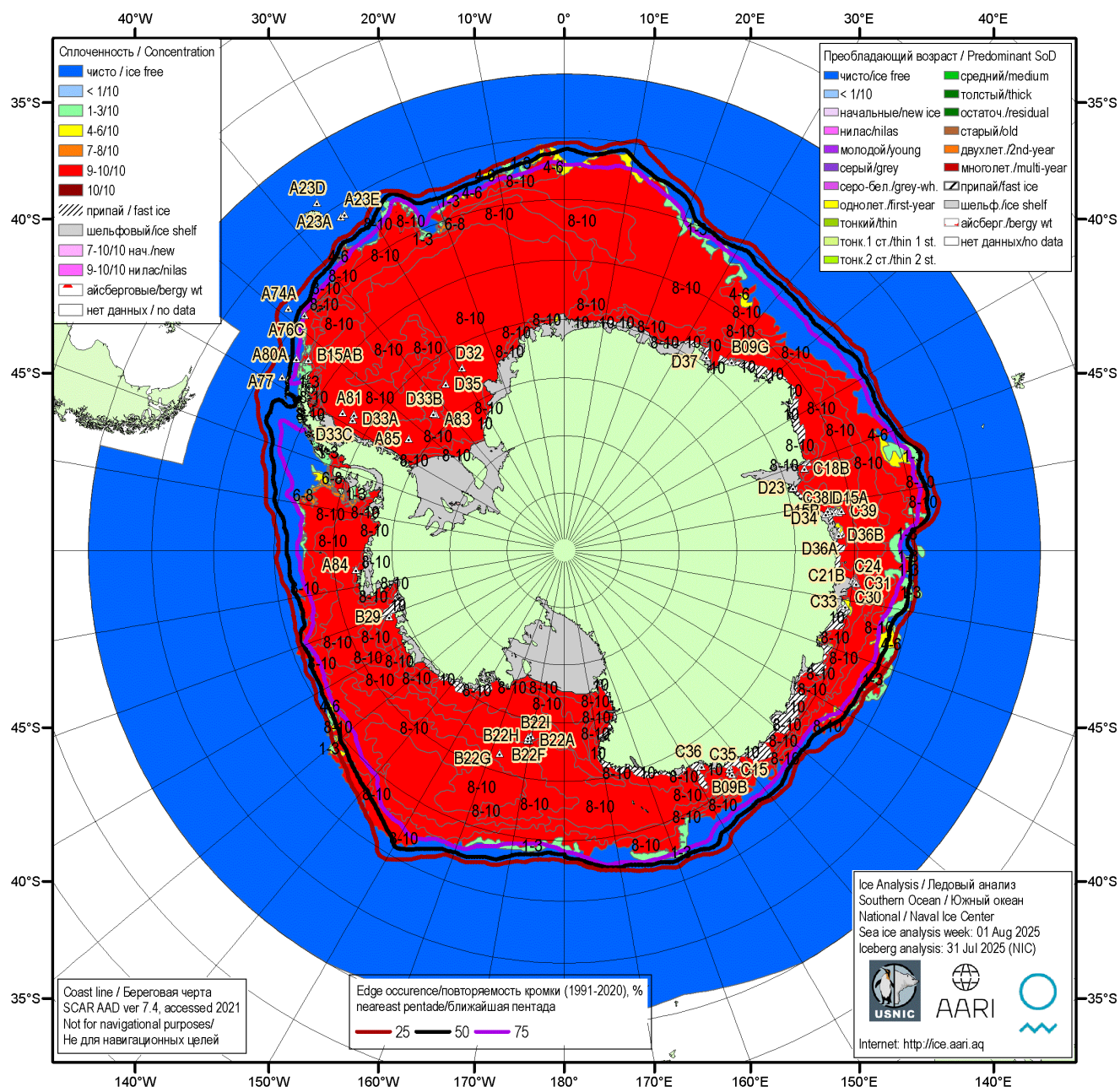
Рисунок 5а – Ледовая карта Южного океана (цветовая окраска по общей сплоченности) и расположение крупных айсбергов на основе ледового анализа за 01.08.2025 в рамках проекта совместного ледового картирования Южного океана ААНИИ, НЛЦ США и НМИ и повторяемость кромки за ближайшую пентаду за период 1991-2020 гг. по наблюдениям SSMR-SSM/I-SSMIS (алгоритм NASATEAM) [5, 10, 17, 21]
