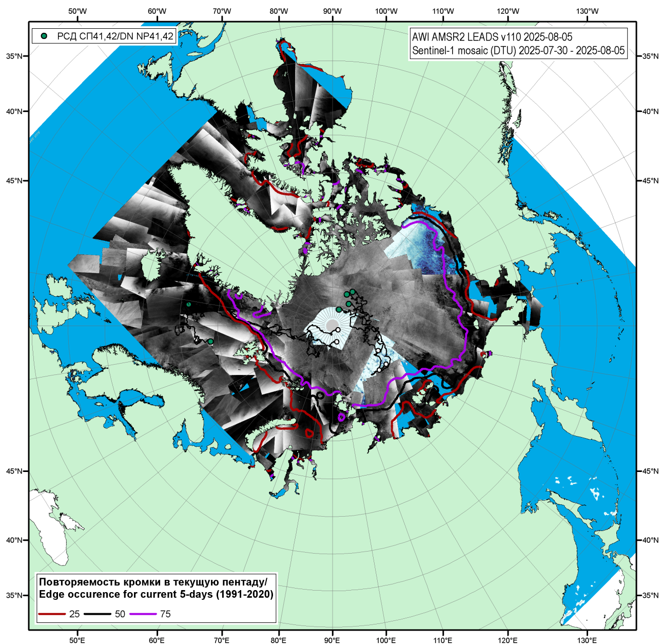
Рисунок 1г – Мозаика снимков Sentinel-1 (DTU) за 30.07.2025 – 05.08.2025, положение крупных полыней по данным AMSR2 за 05.08.2025 (AWI v110), повторяемость кромки за соответствующий 5-дневный период за 1991-2020 гг. по наблюдениям SSMR-SSM/I-SSMIS (алгоритм NASATEAM) и положение РСН СП-42 на 06.08.2025 г. 08:00МСК.
