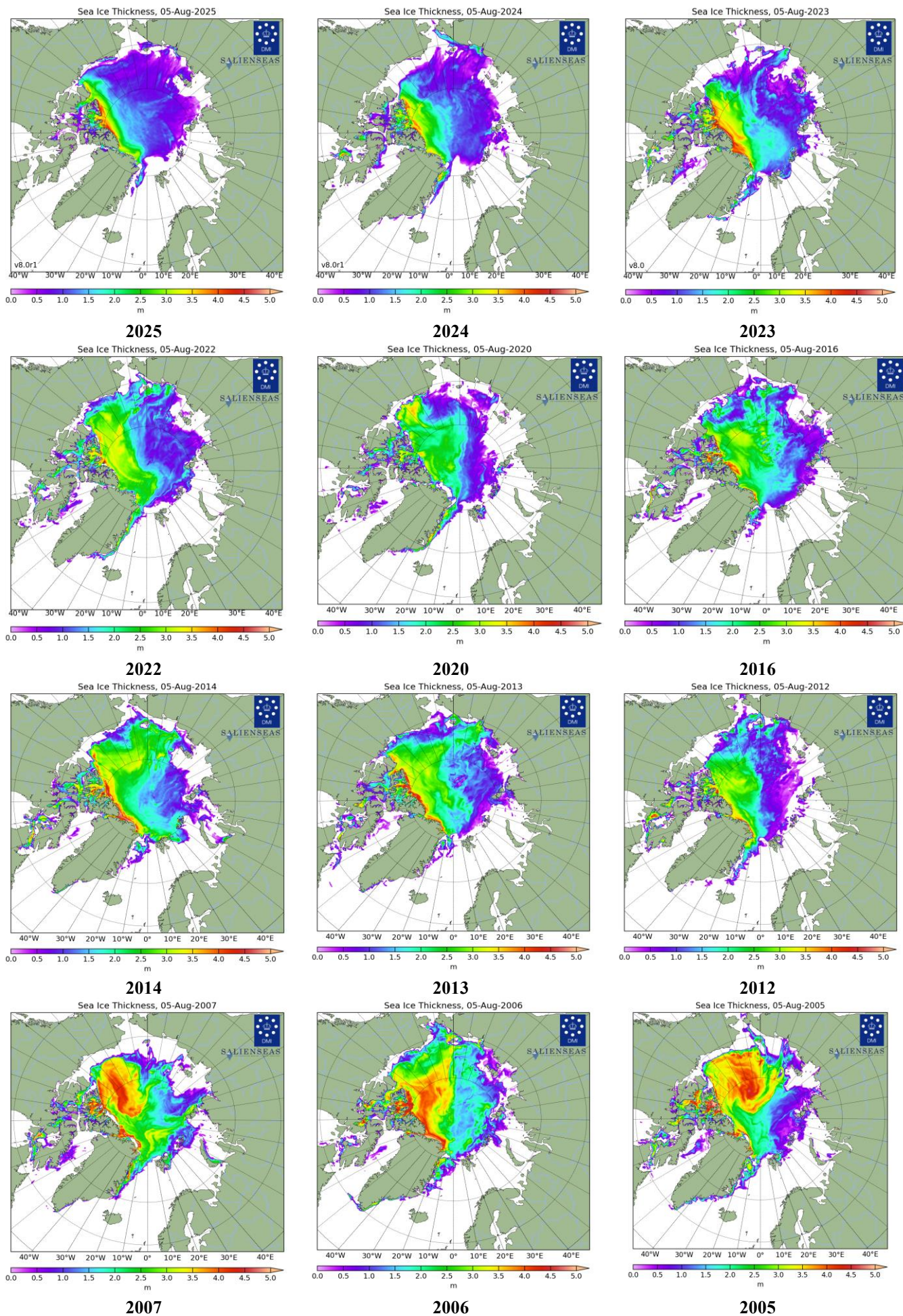
Рисунок 26 – Поля распределения средневзвешенной толщины льда совместной модели морского льда – океана HYCOM/CICE Датского метеорологического института 05.08 за 2005-2025 гг. [22].
