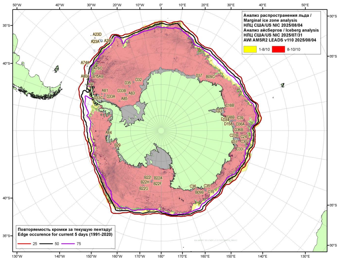
Рисунок 5в – Положение кромки льда и зон разреженных ( <8/10 ) и сплошных ( \geq 8/10 ) льдов Южного океана за 04.08.2025 г. и расположение крупных айсбергов за 31.07.2025 на основе ледового анализа Национального Ледового Центра США, повторяемость кромки за ближайшую пентаду за период 1991-2020 гг. по наблюдениям SSMR-SSM/I-SSMIS (алгоритм NASATEAM), совмещенное с положением разрежений на основе данных ИСЗ AMSR2 за 04.08.2025 (AWI, v110) [10, 17, 24]
