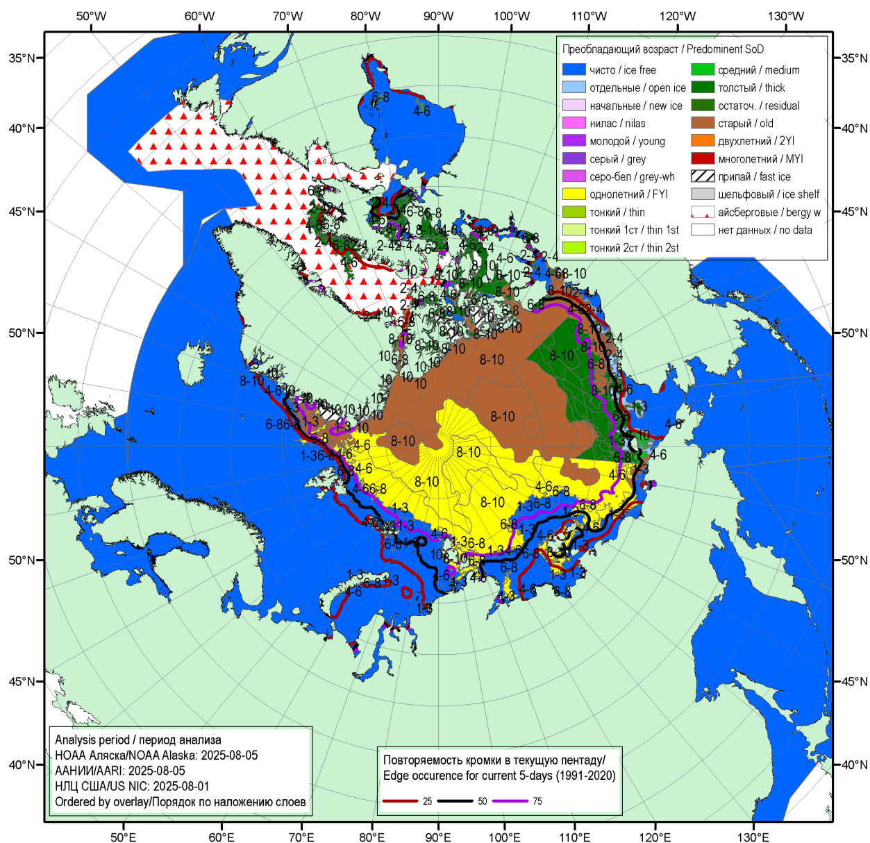
Рисунок 16 – Обзорная ледовая карта СЛО за 01.08.2025 – 05.08.2025 (цветовая раскраска по преобладающему возрасту) на основе ледового анализа NOAA Аляска, ААНИИ и Национального ледового центра США и повторяемость кромки за соответствующий 5-дневный период за 1991-2020 гг. по наблюдениям SSMR-SSM/I-SSMIS (алгоритм NASATEAM) [4, 10, 23, 17].
