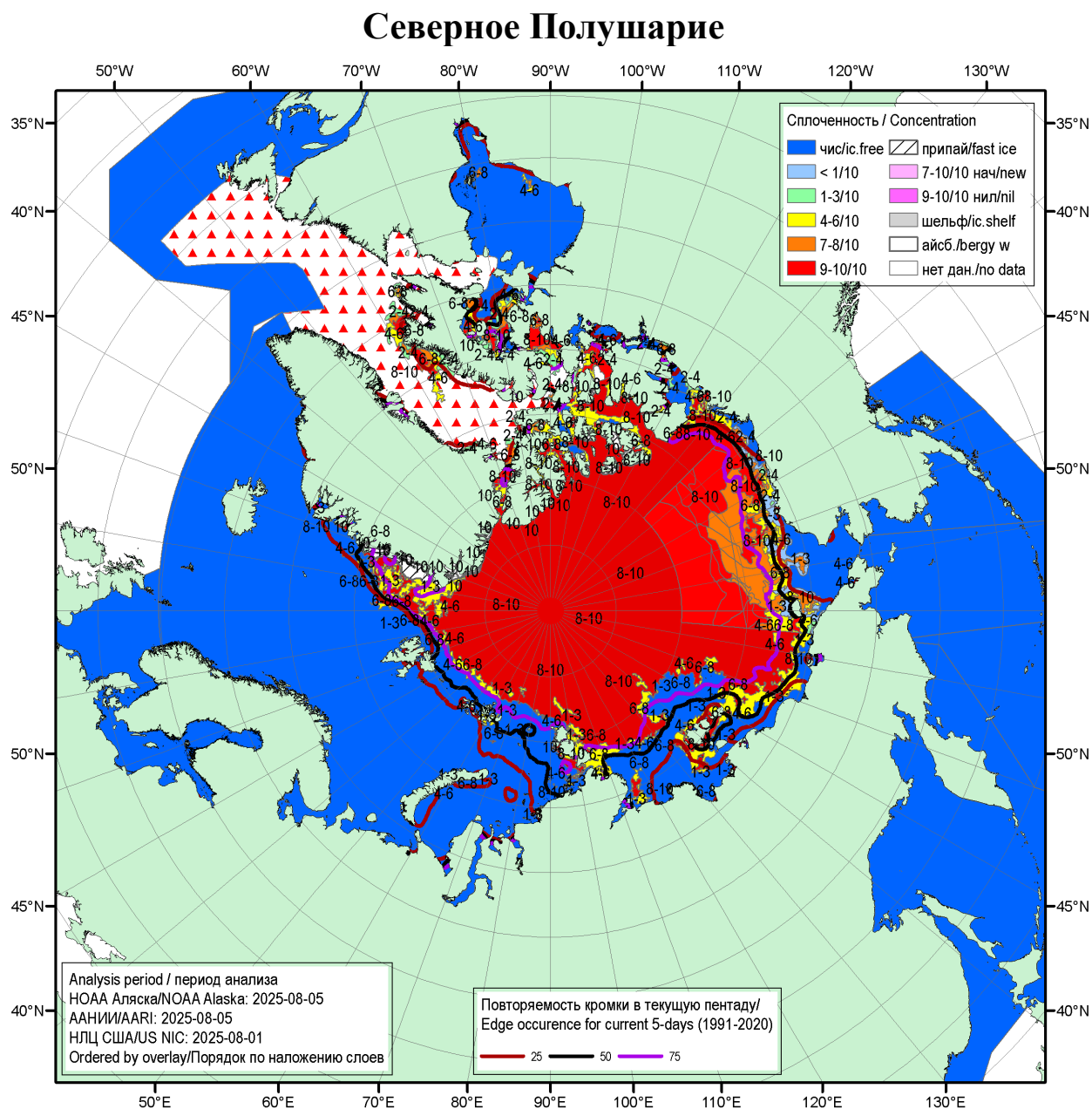
Рисунок 1а – Обзорная ледовая карта СЛО за 01.08.2025 – 05.08.2025 (цветовая раскраска по общей сплоченности) на основе ледового анализа NOAA Аляска, ААНИИ и Национального ледового центра США и повторяемость кромки за соответствующий 5-дневный период за 1991-2020 гг. по наблюдениям SSMR-SSM/I-SSMIS (алгоритм NASATEAM) [4, 10, 23, 17].
