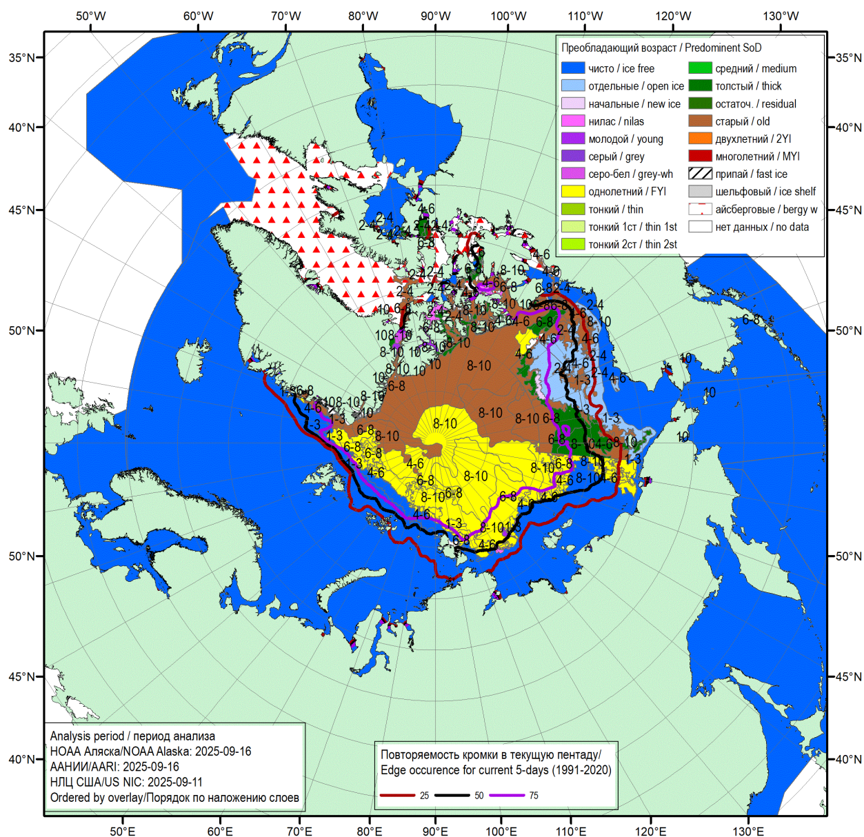
Рисунок 16 – Обзорная ледовая карта СЛО за 11.09.2025 – 16.09.2025 (цветовая раскраска по преобладающему возрасту) на основе ледового анализа НОАА Аляска, ААНИИ и Национального ледового центра США и повторяемость кромки за соответствующий 5-дневный период за 1991-2020 гг. по наблюдениям SSMR-SSM/I-SSMIS (алгоритм NASATEAM) [4, 10, 23, 17].
