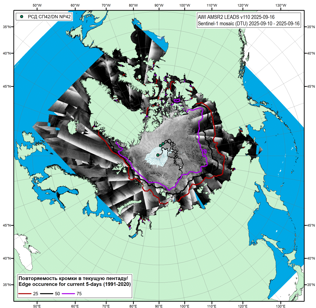
Рисунок 1г – Мозаика снимков Sentinel-1 (DTU) за 10.09.2025 – 16.09.2025, положение крупных полыней по данным AMSR2 за 16.09.2025 (AWI v110), повторяемость кромки за соответствующий 5-дневный период за 1991-2020 гг. по наблюдениям SSMR-SSM/I-SSMIS (алгоритм NASATEAM) и положение РСН СП-42 на 16.09.2025 г. 18:00МСК.
