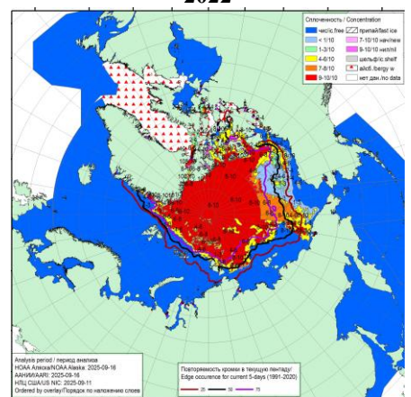
Рисунок 1ж – Ледовые условия за 11.09 - 16.09.2025. и аналогичные периоды 2007-2024 гг. на основе ледового анализа ААНИИ, НИЦ Планета, Канадской ледовой службы, Национального ледового центра США и НОАА Аляска [4, 10, 12, 23, 17].
