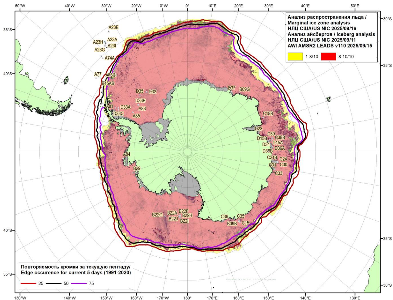
Рисунок 5в – Положение кромки льда и зон разреженных ( <8/10 ) и сплоченных ( \geq 8/10 ) льдов Южного океана за 16.09.2025 г. и расположение крупных айсбергов за 11.09.2025 на основе ледового анализа Национального Ледового Центра США, повторяемость кромки за ближайшую пентаду за период 1991-2020 гг. по наблюдениям SSMR-SSM/I-SSMIS (алгоритм NASATEAM), совмещенное с положением разрежений на основе данных ИСЗ AMSR2 за 16.09.2025 (AWI, v110) [10, 17, 24]
