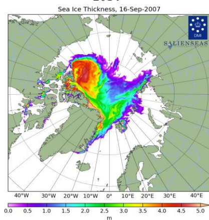
Рисунок 26 – Поля распределения средневзвешенной толщины льда совместной модели морского льда – океана HYCOM/CICE Датского метеорологического института 16.09 за 2005-2025 гг. [22].
