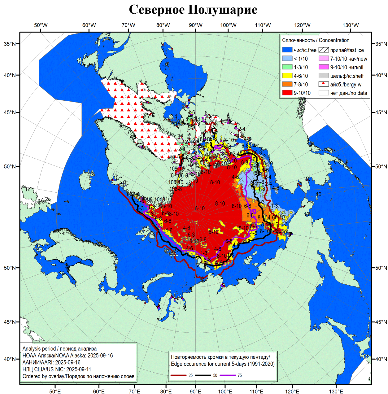
Рисунок 1а – Обзорная ледовая карта СЛО за 11.09.2025 – 16.09.2025 (цветовая раскраска по общей сплоченности) на основе ледового анализа НОАА Аляска, ААНИИ и Национального ледового центра США и повторяемость кромки за соответствующий 5-дневный период за 1991-2020 гг. по наблюдениям SSMR-SSM/I-SSMIS (алгоритм NASATEAM) [4, 10, 23, 17].
