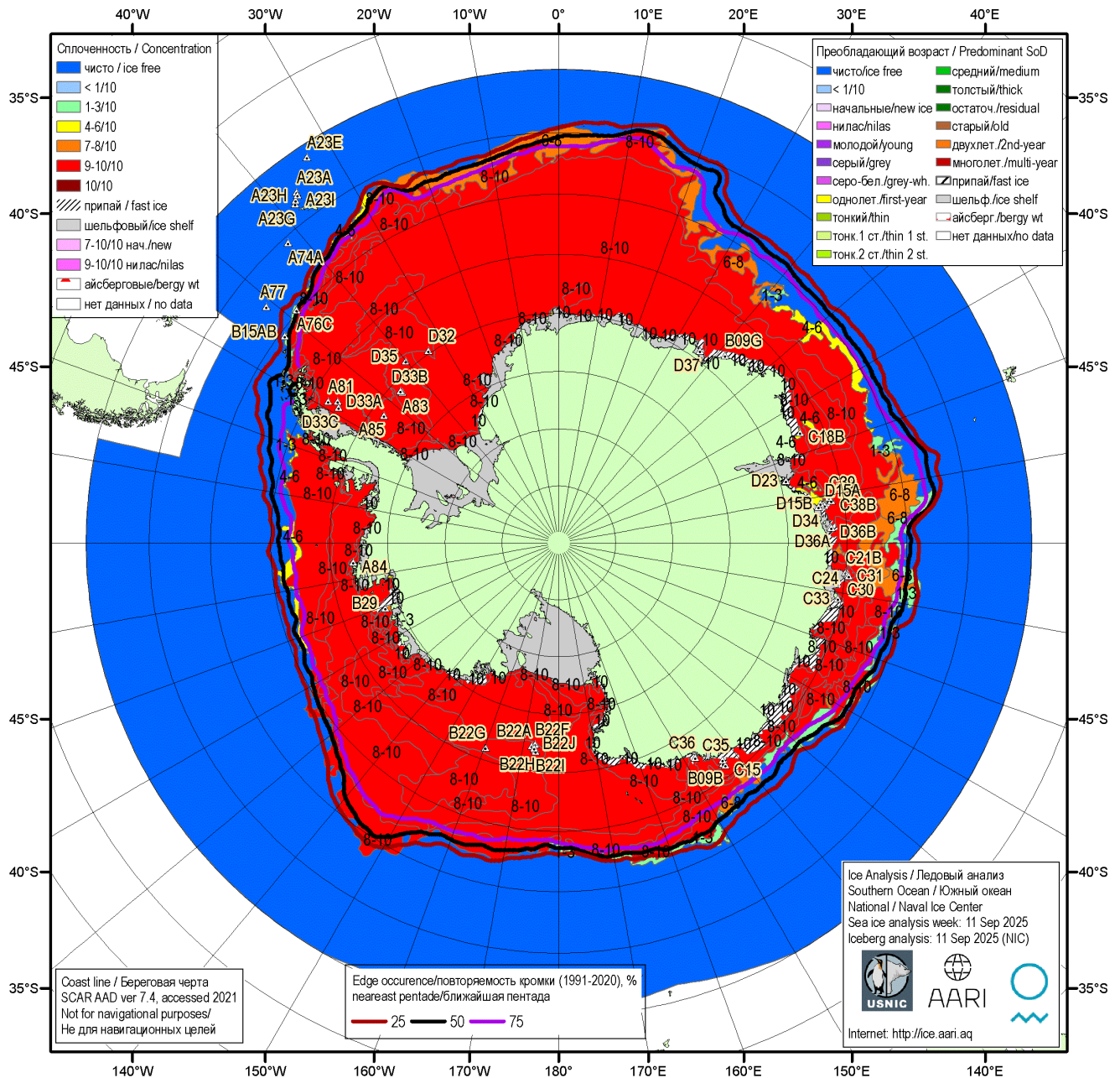
Рисунок 5а – Ледовая карта Южного океана (цветовая окраска по общей сплоченности) и расположение крупных айсбергов на основе ледового анализа за 11.09.2025 в рамках проекта совместного ледового картирования Южного океана ААНИИ, НЛЦ США и НМИ и повторяемость кромки за ближайшую пентаду за период 1991-2020 гг. по наблюдениям SSMR-SSM/I-SSMIS (алгоритм NASATEAM) [5, 10, 17, 21]
