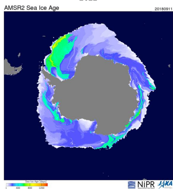
Рисунок 5г – Оценка возраста льда (сутки) на 11.09 за 2018 – 2025 гг. по данным JAXA-NIPR [29]
