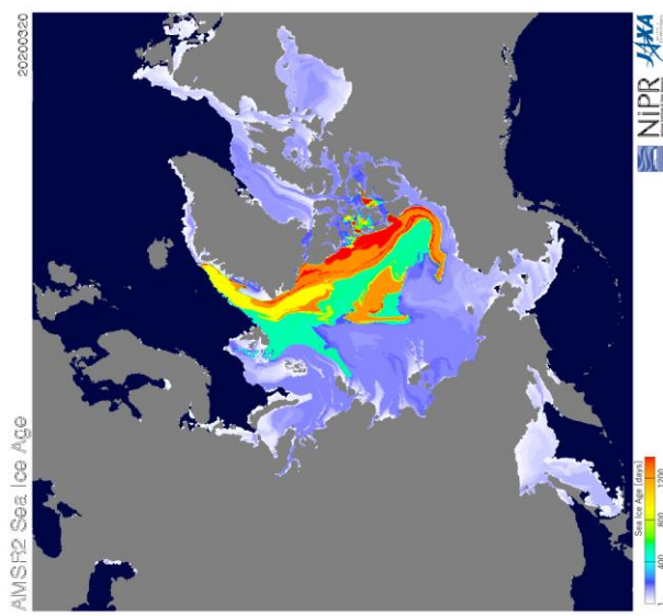
Рисунок 46 – Оценка возраста льда (сутки) на 20.03 за 1818 – 2026 гг. по данным JAXA-NIPR [29]
