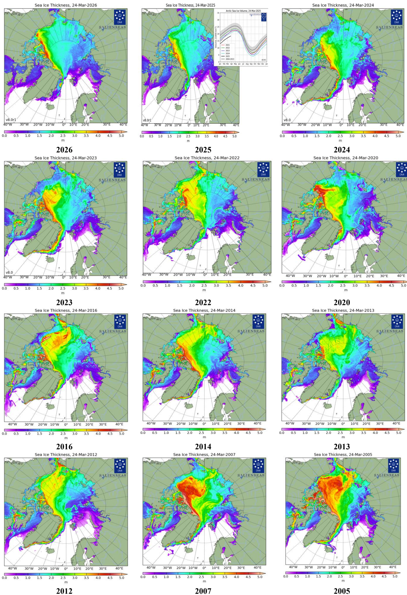
Рисунок 4в – Поля распределения средневзвешенной толщины льда совместной модели морского льда – океана NUSOM/CICE Датского метеорологического института 24.03 за 2005-2026 гг. [22].
