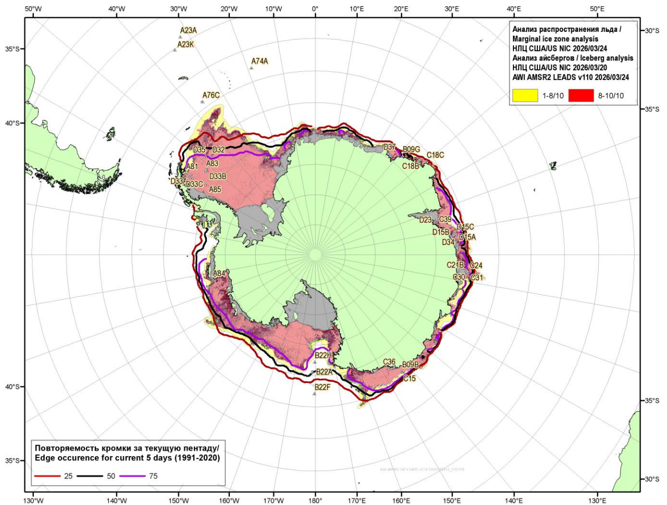
Рисунок 7в – Положение кромки льда и зон разреженных ( <8/10 ) и сплоченных ( \geq 8/10 ) льдов Южного океана за 24.03.2026 г. и расположение крупных айсбергов за 20.03.2026 на основе ледового анализа Национального Ледового Центра США, повторяемость кромки за ближайшую пентаду за период 1991-2020 гг. по наблюдениям SSMR-SSM/I-SSMIS (алгоритм NASATEAM), совмещенное с положением разрежений на основе данных ИСЗ AMSR2 за 24.03.2026 (AWI, v110) [10, 17, 24]
