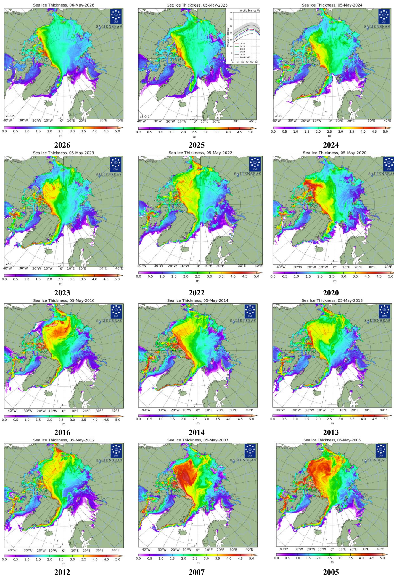
Рисунок 4в – Поля распределения средневзвешенной толщины льда совместной модели морского льда – океана NUSOM/CICE Датского метеорологического института 05.05 за 2005-2026 гг. [22].
