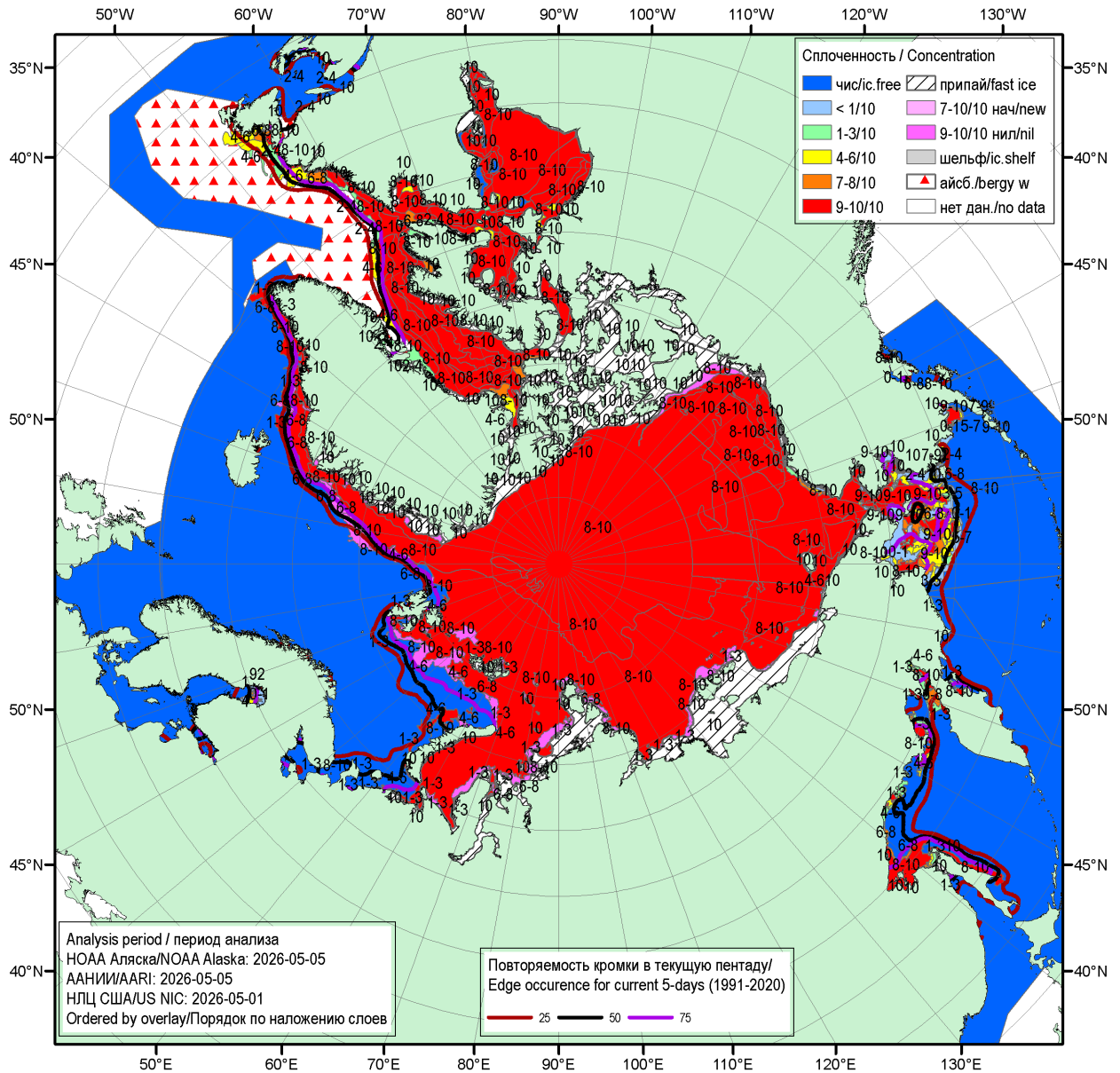
Рисунок 1а – Обзорная ледовая карта СЛО за 01.05.2026 – 05.05.2026 (цветовая раскраска по общей сплоченности) на основе ледового анализа НОАА Аляска, ААНИИ и Национального ледового центра США и повторяемость кромки за соответствующий 5-дневный период за 1991-2020 гг. по наблюдениям SSMR-SSM/I-SSMIS (алгоритм NASATEAM) [4, 10, 23, 17].
