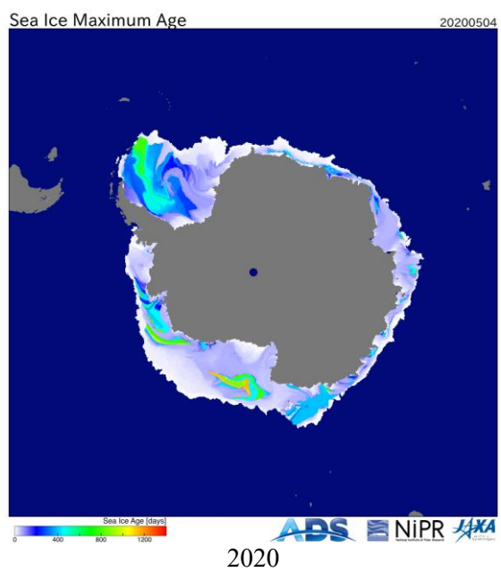
Рисунок 86 – Оценка максимального возраста льда (сутки) на 04.05 за 2018 – 2026 гг. по данным JAXA-NiPR [29]
