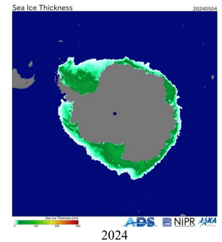
Рисунок 8а - Оценка толщины льда и степени разрушенности на основе данных пассивного микроволнового зондирования AMSR2 04.05 в 2018 – 2026 гг. [29].
