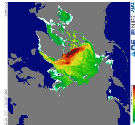
Рисунок 2а - Оценка толщины льда и степени разрушенности на основе данных пассивного микроволнового зондирования AMSR2 04.05 в 2018 – 2026 гг. [29].
