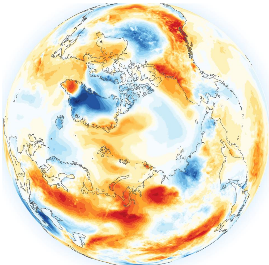
Рисунок 5а – Аномалия приземной температуры воздуха (2м) и температуры поверхности моря на 04.05.2026 г. относительно периода 1991-2020 гг. - The Copernicus Climate Change Service (C3S) , implemented by the European Centre for Medium-Range Weather Forecasts (ECMWF) on behalf of the European Commission is part of the European Union's space programme
