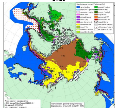
Рисунок 4а – Ледовые условия за 01.05 - 05.05.2026. и аналогичные периоды 2007-2025 гг. на основе ледового анализа ААНИИ, НИЦ Планета, Канадской ледовой службы, Национального ледового центра США и НОАА Аляска [4, 10, 12, 23, 17].
