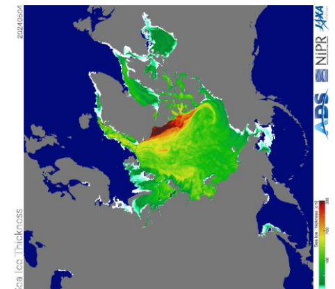
Рисунок 2а - Оценка толщины льда и степени разрушенности на основе данных пассивного микроволнового зондирования AMSR2 04.05 в 2018 – 2026 гг. [29].
