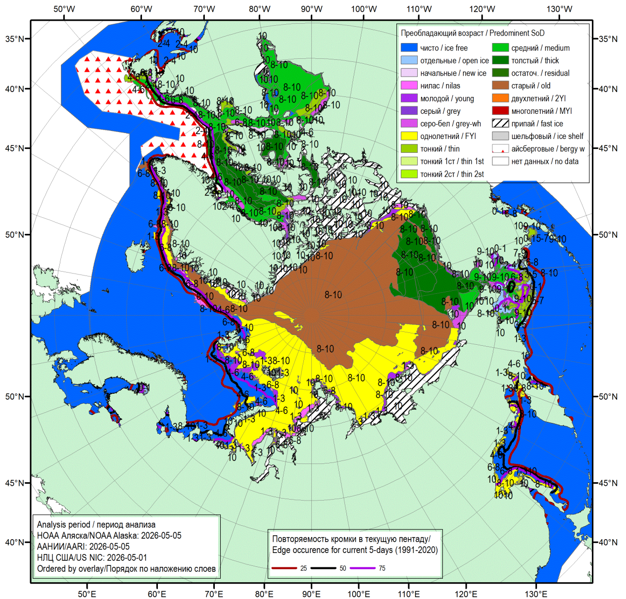
Рисунок 16 – Обзорная ледовая карта СЛО за 01.05.2026 – 05.05.2026 (цветовая раскраска по преобладающему возрасту) на основе ледового анализа НОАА Аляска, ААНИИ и Национального ледового центра США и повторяемость кромки за соответствующий 5-дневный период за 1991-2020 гг. по наблюдениям SSMR-SSM/I-SSMIS (алгоритм NASATEAM) [4, 10, 23, 17].
