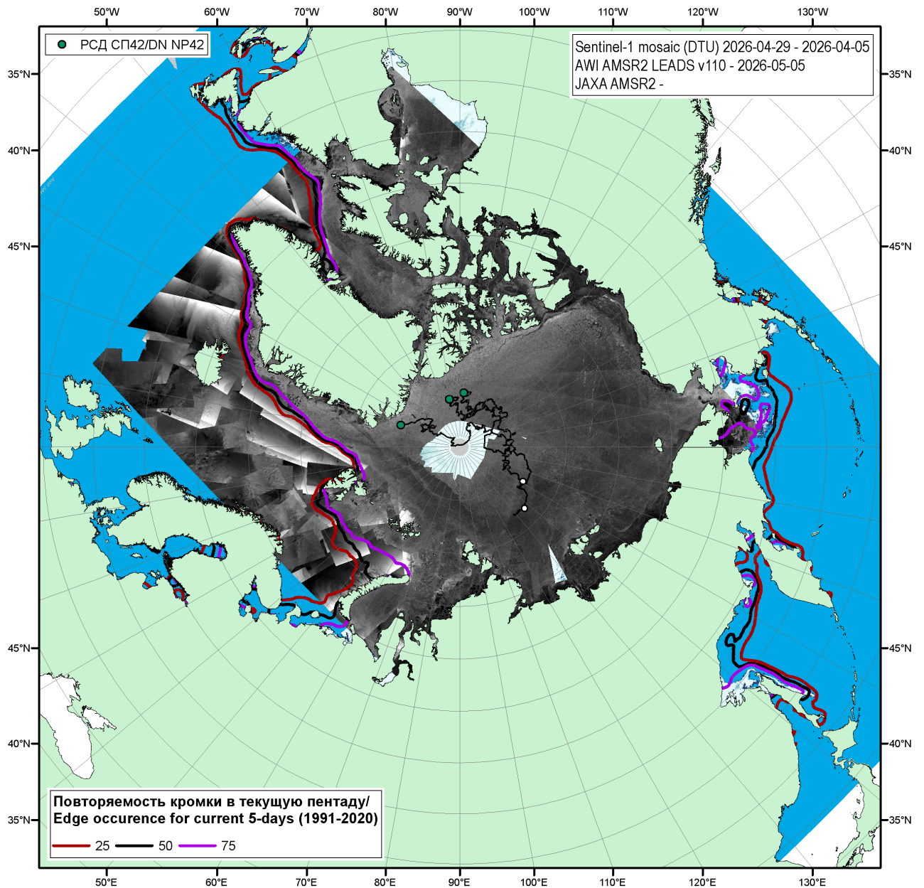
Рисунок 1в – Мозаика снимков Sentinel-1 (DTU) за 29.04.2026 – 05.05.2026, общая сплоченность и оценка положения полыней за 05.05.2026 г. по данным AMSR2 (AWI-JAXA), повторяемость кромки за соответствующий 5-дневный период за 1991-2020 гг. по наблюдениям SSMR-SSM/I-SSMIS (алгоритм NASATEAM) и положение РСН СП-42 на 06.05.2025 г. 08:00МСК.
