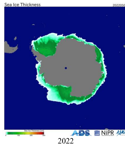
Рисунок 8а - Оценка толщины льда и степени разрушенности на основе данных пассивного микроволнового зондирования AMSR2 04.05 в 2018 – 2026 гг. [29].
