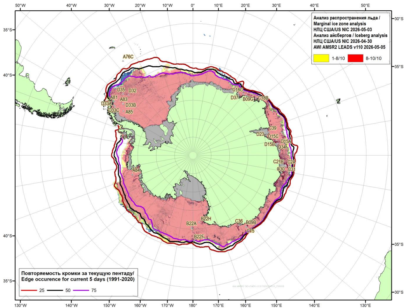
Рисунок 7в – Положение кромки льда и зон разреженных ( <8/10 ) и сплоченных ( \geq 8/10 ) льдов Южного океана за 03.05.2026 и расположение крупных айсбергов за 30.04.2026 на основе ледового анализа Национального Ледового Центра США, повторяемость кромки за ближайшую пентаду за период 1991-2020 гг. по наблюдениям SSMR-SSM/I-SSMIS (алгоритм NASATEAM), совмещенное с положением разрежений на основе данных ИСЗ AMSR2 за 05.05.2026 (AWI-JAXA, v110) [10, 17, 24]
