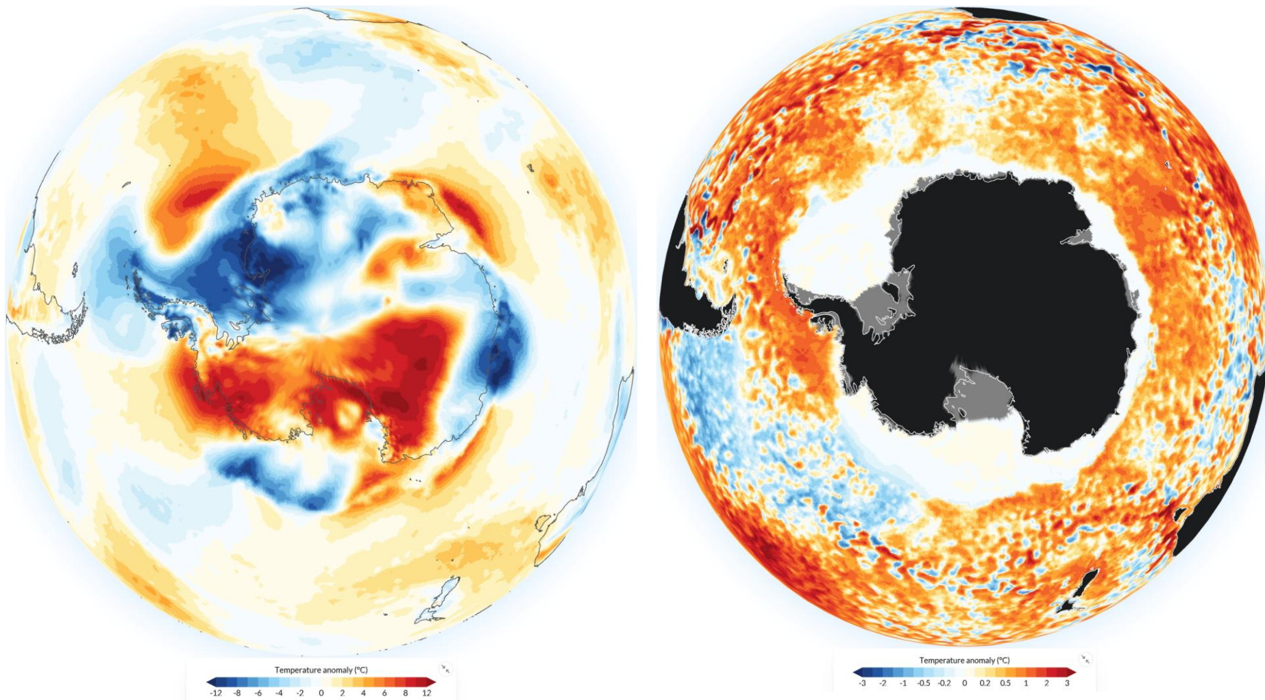
Рисунок 9 – Аномалия приземной температуры воздуха (2м) на 04.05.2026 г. относительно периода 1991-2020 гг. - The Copernicus Climate Change Service (C3S) , implemented by the European Centre for Medium-Range Weather Forecasts (ECMWF) on behalf of the European Commission is part of the European Union's space programme.
