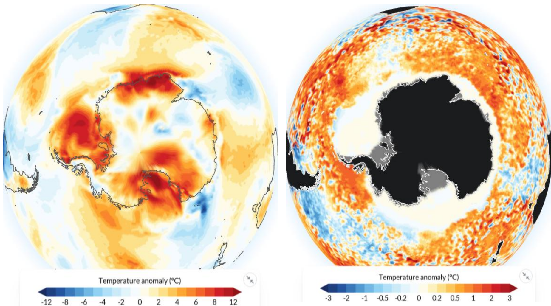
Рисунок 9 – Аномалия приземной температуры воздуха (2м) на 11.05.2026 г. относительно периода 1991-2020 гг. - The Copernicus Climate Change Service (C3S) , implemented by the European Centre for Medium-Range Weather Forecasts (ECMWF) on behalf of the European Commission is part of the European Union's space programme.
