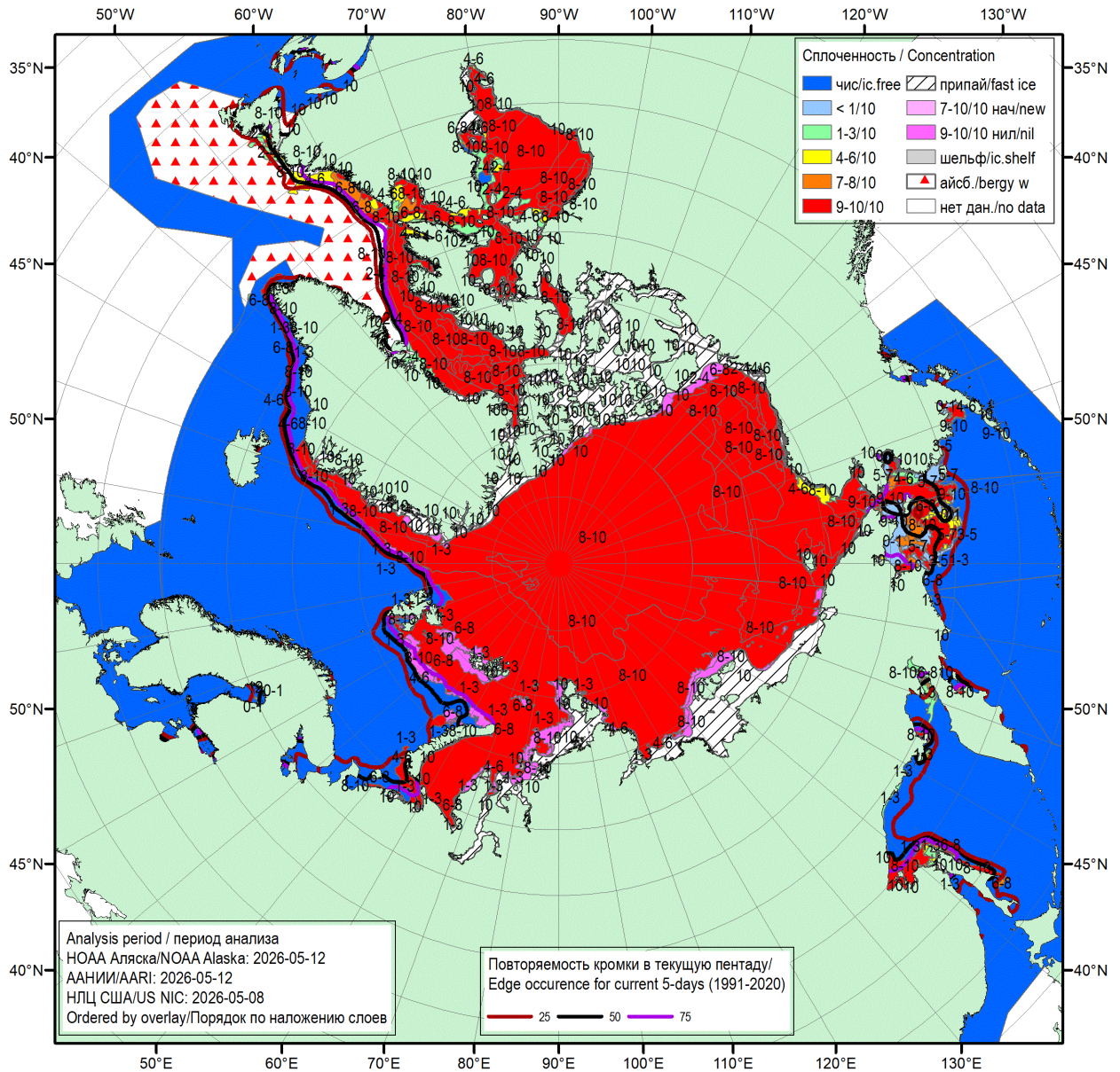
Рисунок 1а – Обзорная ледовая карта СЛО за 08.05.2026 – 12.05.2026 (цветовая раскраска по общей сплоченности) на основе ледового анализа NOAA Аляска, ААНИИ и Национального ледового центра США и повторяемость кромки за соответствующий 5-дневный период за 1991-2020 гг. по наблюдениям SSMR-SSM/I-SSMIS (алгоритм NASATEAM) [4, 10, 23, 17].
