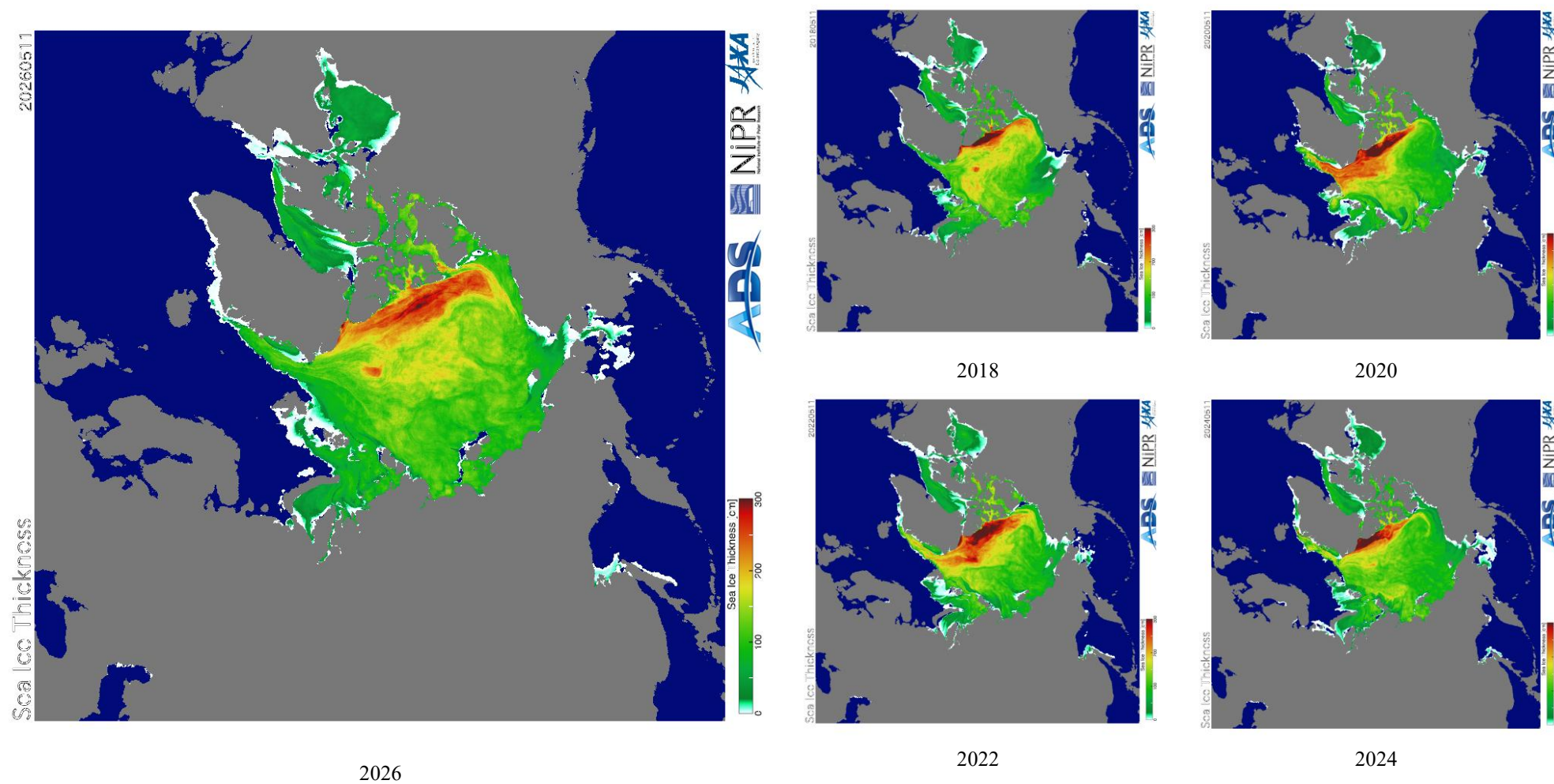
Рисунок 2а - Оценка толщины льда и степени разрушенности на основе данных пассивного микроволнового зондирования AMSR2 11.05 в 2018 – 2026 гг. [29].
