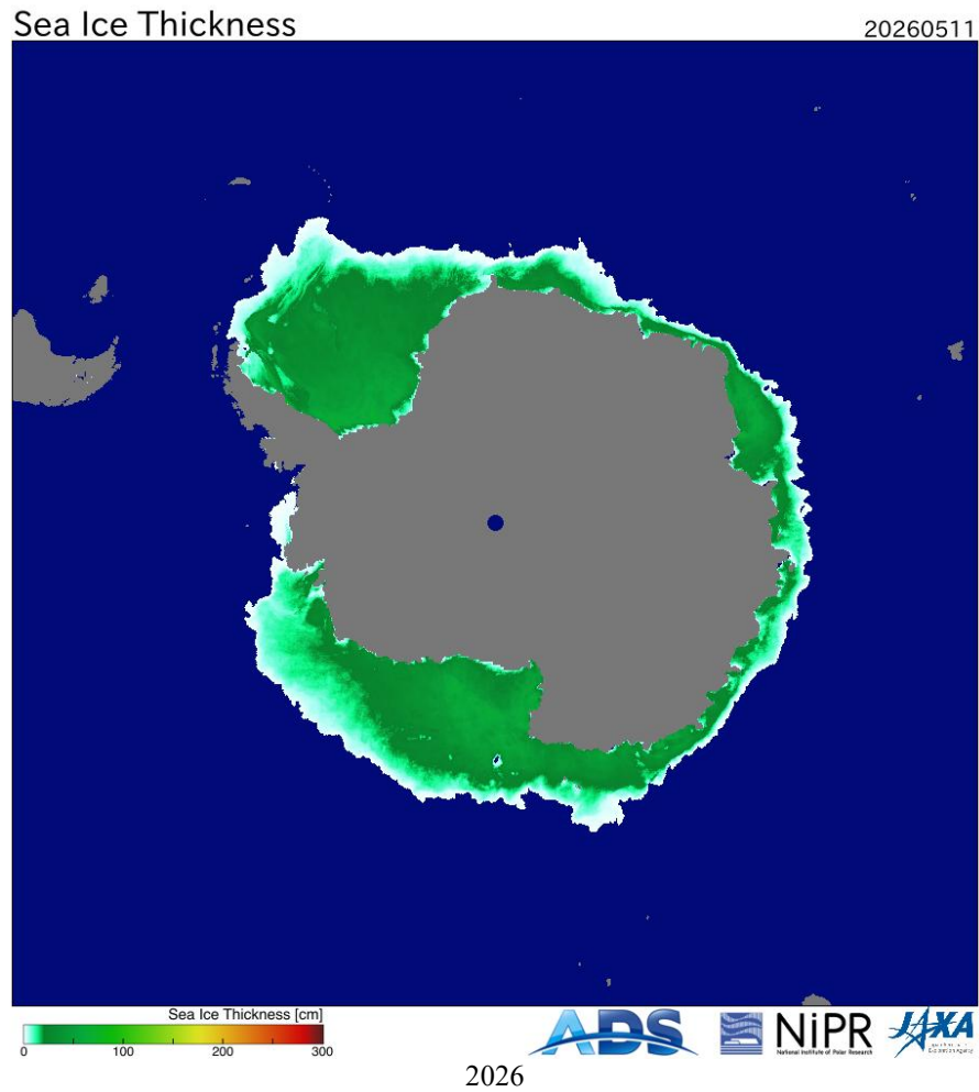
Рисунок 8а - Оценка толщины льда и степени разрушенности на основе данных пассивного микроволнового зондирования AMSR2 11.05 в 2018 – 2026 гг. [29].
