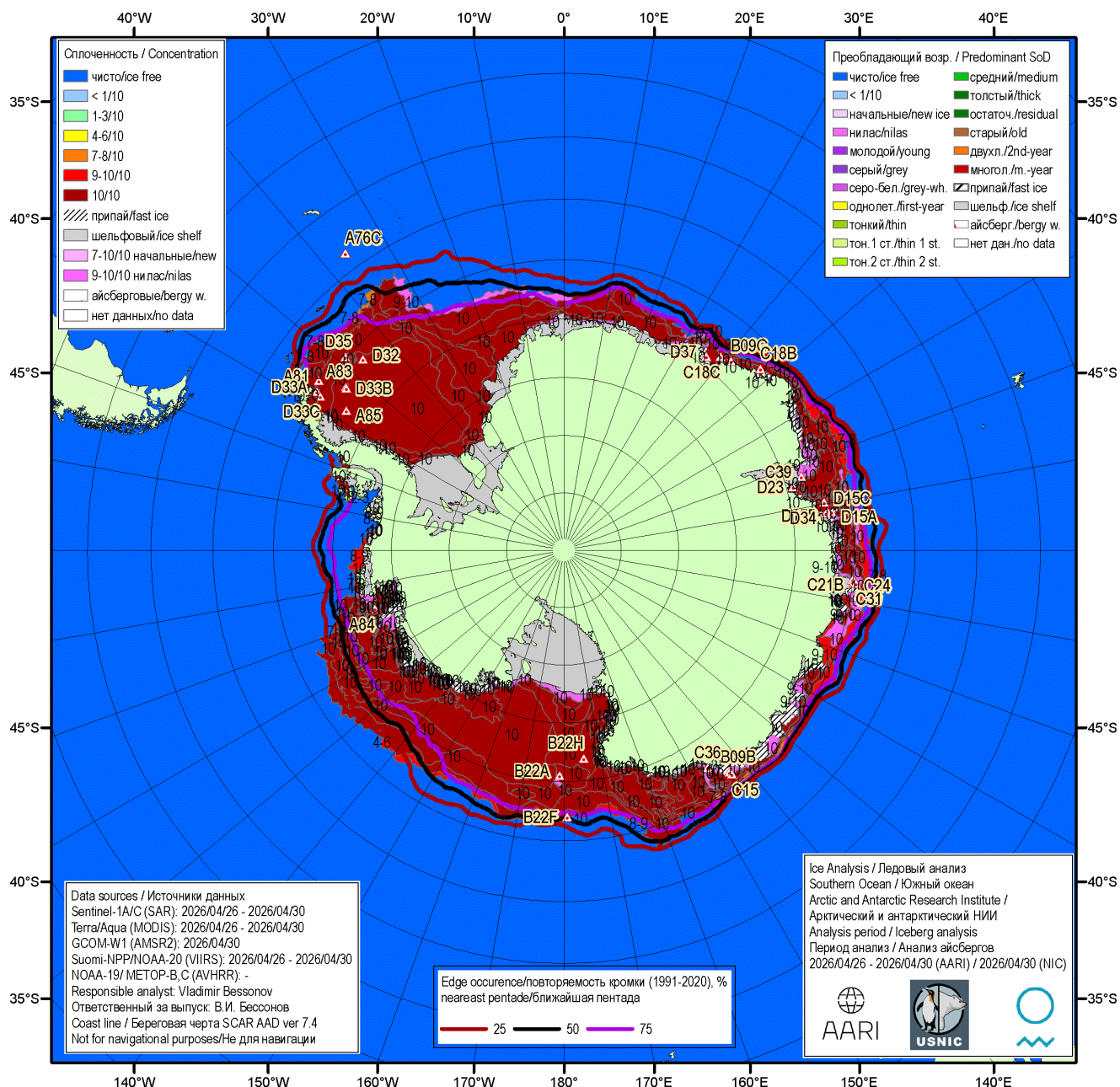
Рисунок 7а – Ледовая карта Южного океана (цветовая окраска по общей сплоченности) и расположение крупных айсбергов на основе ледового анализа за 30.04.2026 в рамках проекта совместного ледового картирования Южного океана ААНИИ, НЛЦ США и НМИ и повторяемость кромки за ближайшую пентаду за период 1991-2020 гг. по наблюдениям SSMR-SSM/I-SSMIS (алгоритм NASATEAM) [5, 10, 17, 21]
