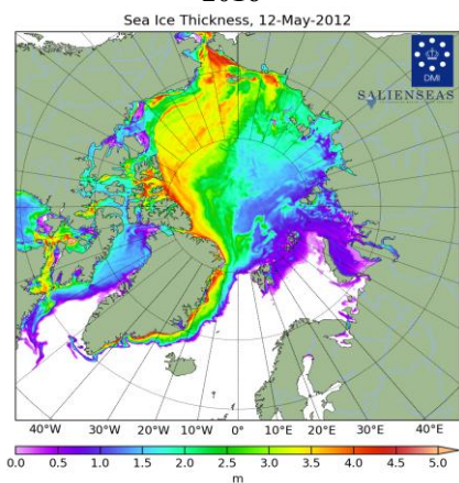
Рисунок 4в – Поля распределения средневзвешенной толщины льда совместной модели морского льда – океана NUSOM/CICE Датского метеорологического института 12.05 за 2005-2026 гг. [22].
