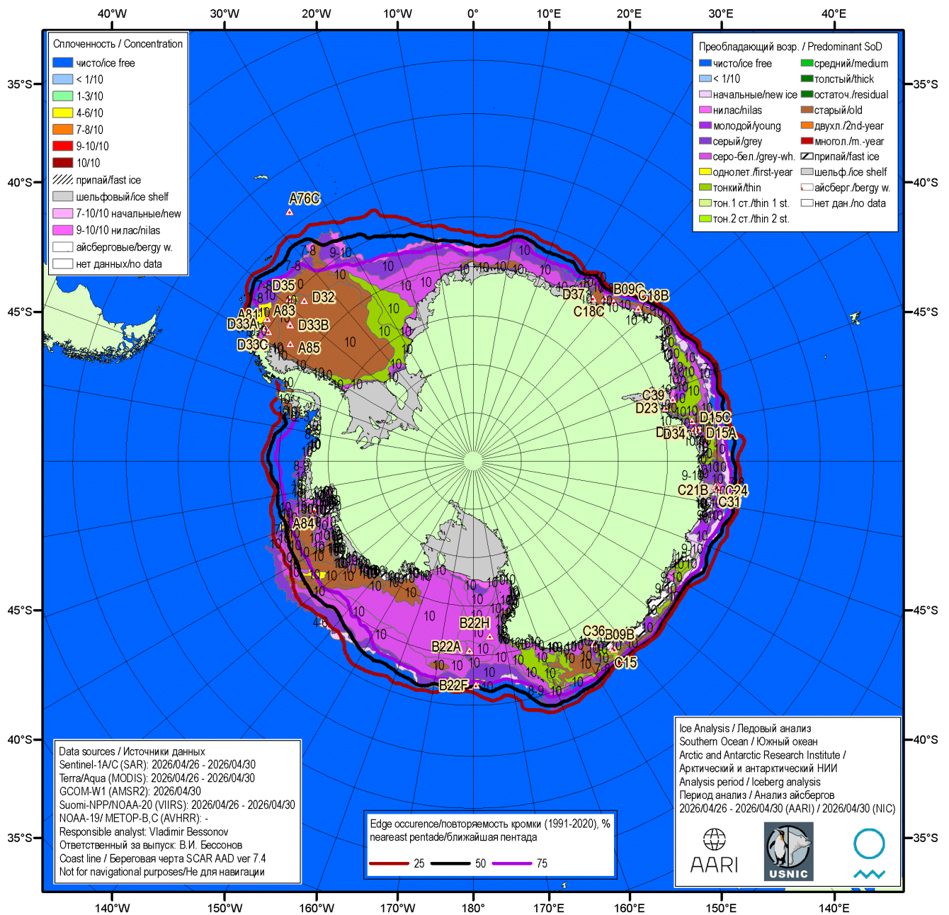
Рисунок 76 – Ледовая карта Южного океана (цветовая окраска по возрасту) и расположение крупных айсбергов на основе ледового анализа за 30.04.2026 в рамках проекта совместного ледового картирования Южного океана ААНИИ, НЛЦ США и НМИ и повторяемость кромки за ближайшую пентаду за период 1991-2020 гг. по наблюдениям SSMR-SSM/I-SSMIS (алгоритм NASATEAM) [5, 10, 17, 21].
