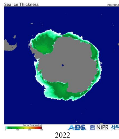
Рисунок 8а - Оценка толщины льда и степени разрушенности на основе данных пассивного микроволнового зондирования AMSR2 11.05 в 2018 – 2026 гг. [29].
