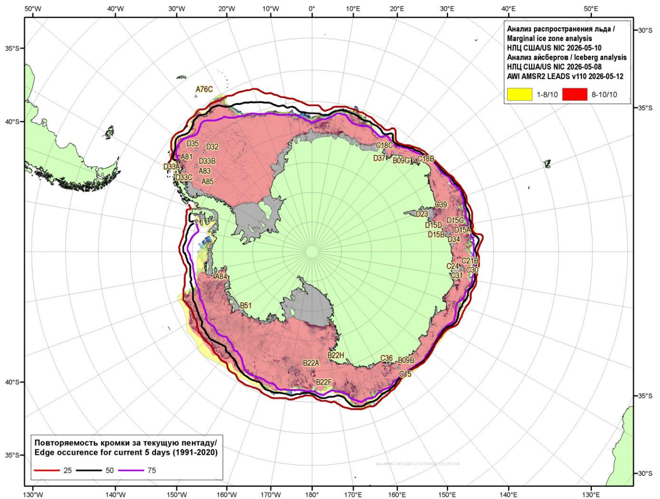
Рисунок 7в – Положение кромки льда и зон разреженных ( < 8/10 ) и сплоченных ( \geq 8/10 ) льдов Южного океана за 10.05.2026 и расположение крупных айсбергов за 08.05.2026 на основе ледового анализа Национального Ледового Центра США, повторяемость кромки за ближайшую пентаду за период 1991-2020 гг. по наблюдениям SSMR-SSM/I-SSMIS (алгоритм NASATEAM), совмещенное с положением разрежений на основе данных ИСЗ AMSR2 за 12.05.2026 (AWI-JAXA, v110) [10, 17, 24]
