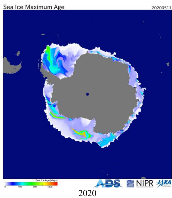
Рисунок 86 – Оценка максимального возраста льда (сутки) на 11.05 за 2018 – 2026 гг. по данным JAXA-NIPR [29]
