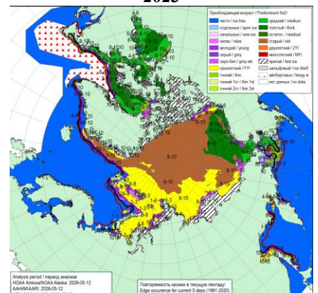
Рисунок 4а – Ледовые условия за 08.05 - 12.05.2026. и аналогичные периоды 2007-2025 гг. на основе ледового анализа ААНИИ, НИЦ Планета, Канадской ледовой службы, Национального ледового центра США и НОАА Аляска [4, 10, 12, 23, 17].
