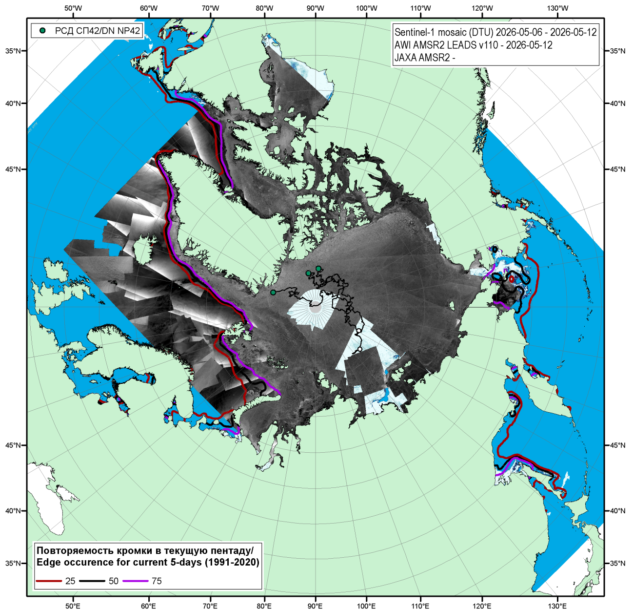
Рисунок 1в – Мозаика снимков Sentinel-1 (DTU) за 06.05.2026 – 12.05.2026, общая сплоченность и оценка положения полыней за 12.05.2026 г. по данным AMSR2 (AWI-JAXA), повторяемость кромки за соответствующий 5-дневный период за 1991-2020 гг. по наблюдениям SSMR-SSM/I-SSMIS (алгоритм NASATEAM) и положение РСН СП-42 на 13.05.2025 г. 08:00МСК.
