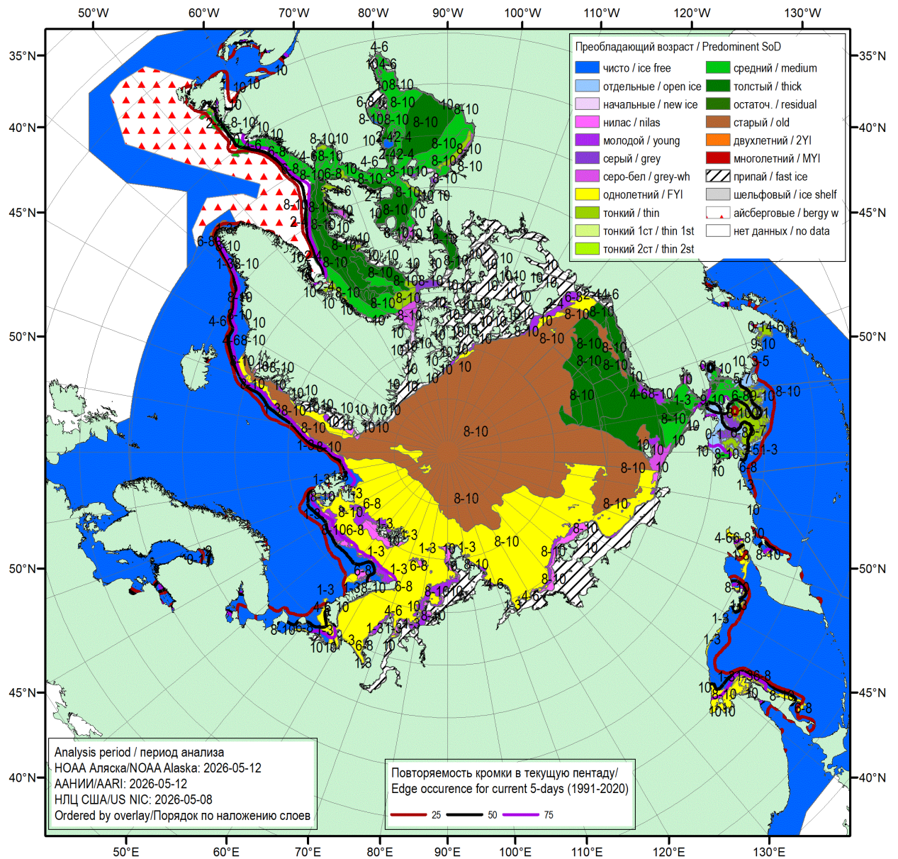
Рисунок 16 – Обзорная ледовая карта СЛО за 08.05.2026 – 12.05.2026 (цветовая раскраска по преобладающему возрасту) на основе ледового анализа NOAA Аляска, ААНИИ и Национального ледового центра США и повторяемость кромки за соответствующий 5-дневный период за 1991-2020 гг. по наблюдениям SSMR-SSM/I-SSMIS (алгоритм NASATEAM) [4, 10, 23, 17].
