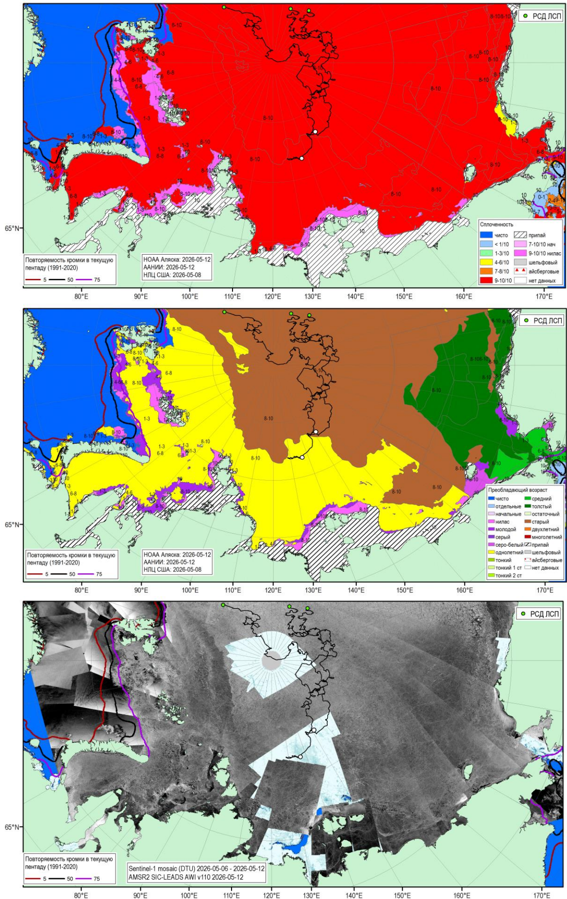
Рисунок 3 - Обзорная ледовая карта СМП за 08.05-12.05.2026 г., мозаика радиолокационных снимком ИСЗ Sentinel-1AC за 06.05-12.05.2026 (DTU) с оценкой положения польшей за 12.05.2026 г. по данным AMSR2 (AWI-JAXA), повторяемость кромки за соответствующий 5-дневный период 1991-2020 гг. по наблюдениям SSMR-SSM/I-SSMIS (алгоритм NASATEAM) и положение РСН СП-42 на 13.05.2026 0800МСК [27, 28, 17].
