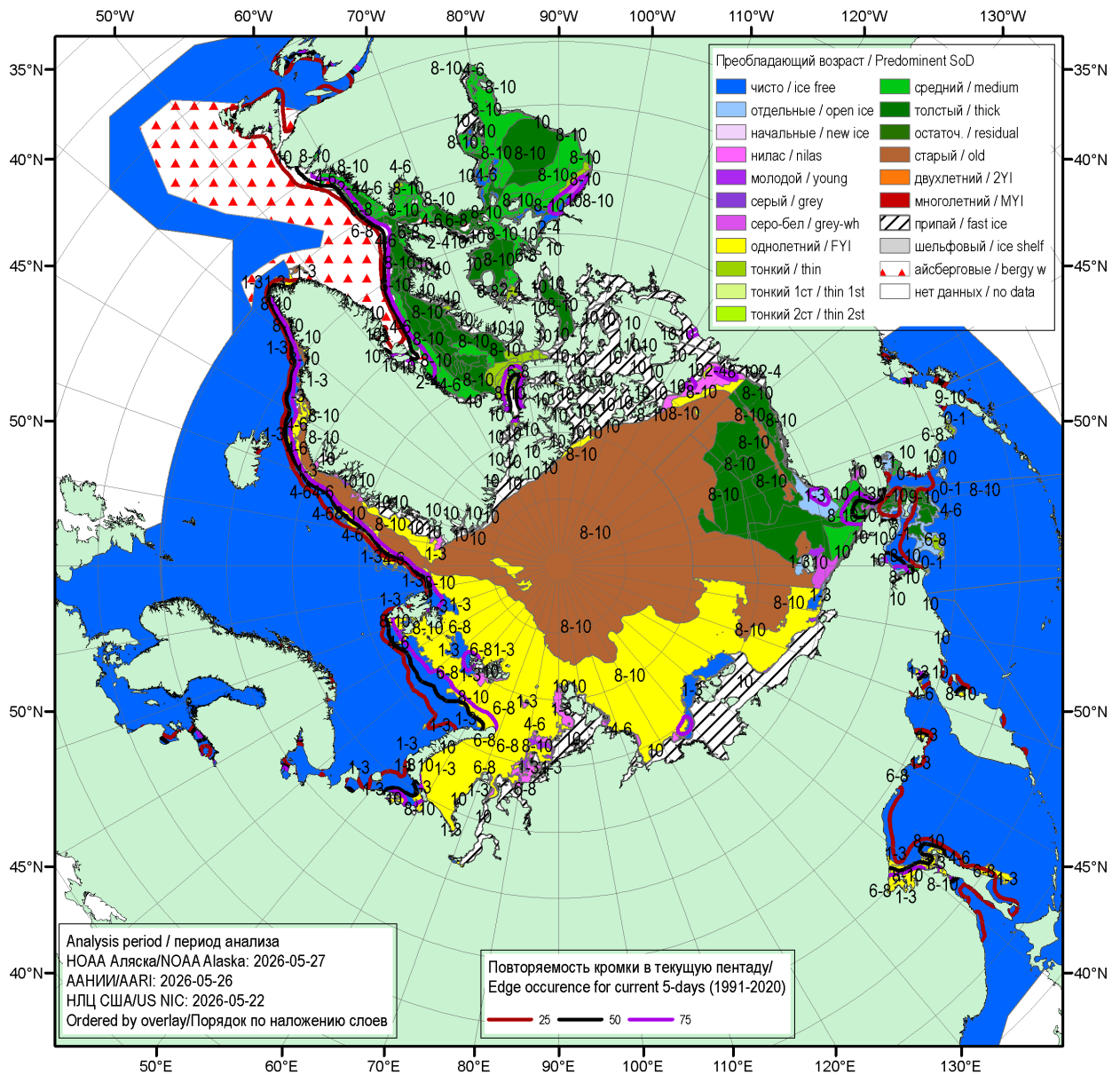
Рисунок 16 – Обзорная ледовая карта СЛО за 22.05.2026 – 27.05.2026 (цветовая раскраска по преобладающему возрасту) на основе ледового анализа NOAA Аляска, ААНИИ и Национального ледового центра США и повторяемость кромки за соответствующий 5-дневный период за 1991-2020 гг. по наблюдениям SSMR-SSM/I-SSMIS (алгоритм NASATEAM) [4, 10, 23, 17].
