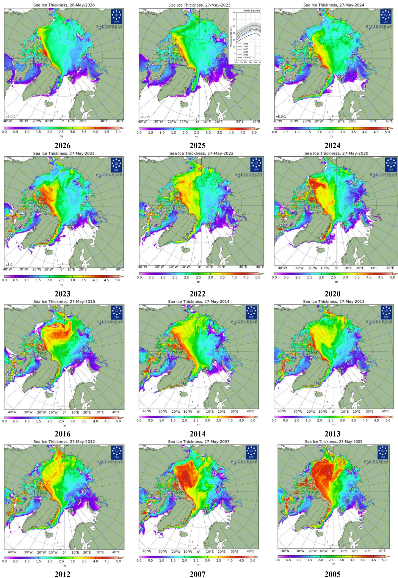
Рисунок 4в – Поля распределения средневзвешенной толщины льда совместной модели морского льда – океана NUSOM/CICE Датского метеорологического института 26-27.05 за 2005-2026 гг. [22].
