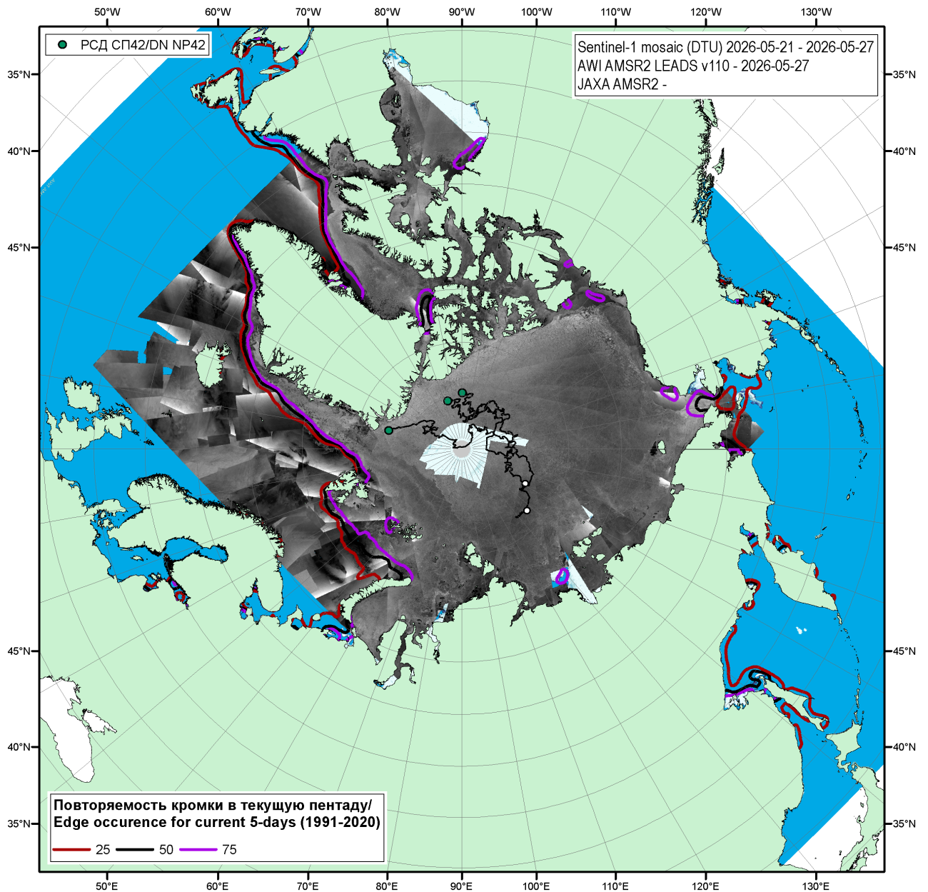
Рисунок 1в – Мозаика снимков Sentinel-1 (DTU) за 21.05.2026 – 27.05.2026, общая сплоченность и оценка положения полыней за 27.05.2026 г. по данным AMSR2 (AWI-JAXA), повторяемость кромки за соответствующий 5-дневный период за 1991-2020 гг. по наблюдениям SSMR-SSM/I-SSMIS (алгоритм NASATEAM) и положение РСН СП-42 на 28.05.2025 г. 06:00МСК.
