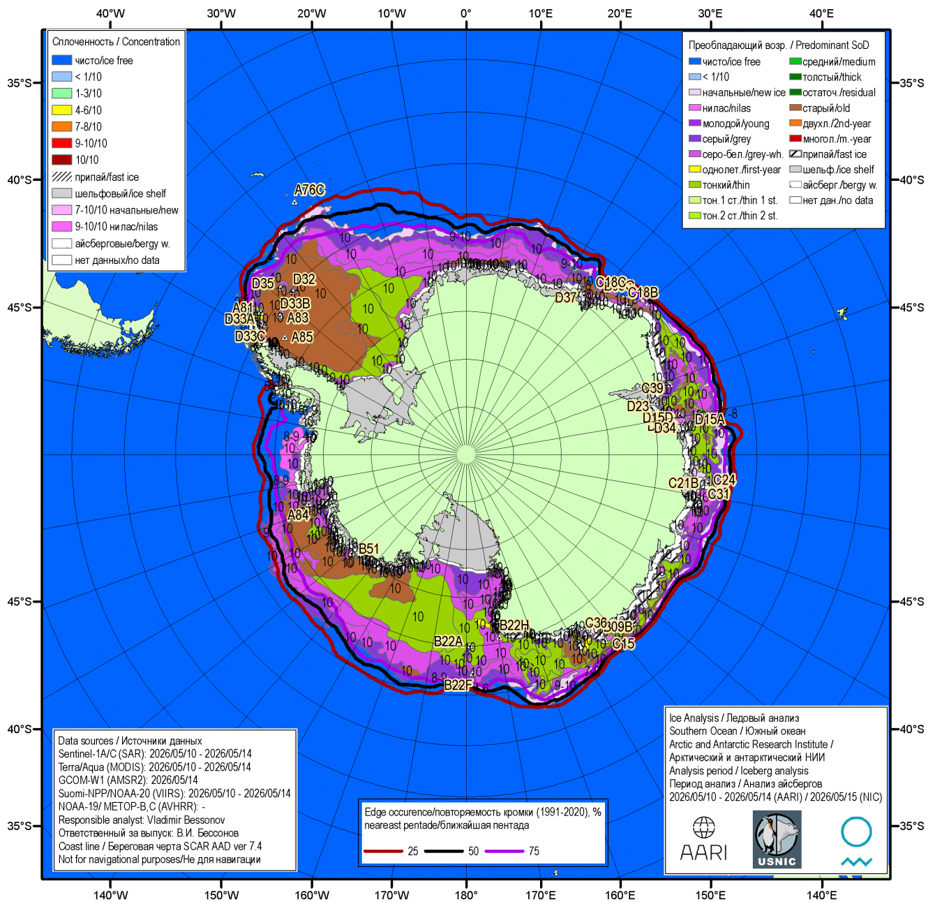
Рисунок 76 – Ледовая карта Южного океана (цветовая окраска по возрасту) и расположение крупных айсбергов на основе ледового анализа за 14.05.2026 в рамках проекта совместного ледового картирования Южного океана ААНИИ, НЛЦ США и НМИ и повторяемость кромки за ближайшую пентаду за период 1991-2020 гг. по наблюдениям SSMR-SSM/I-SSMIS (алгоритм NASATEAM) [5, 10, 17, 21].
