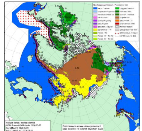
Рисунок 4а – Ледовые условия за 22.05 - 27.05.2026. и аналогичные периоды 2007-2025 гг. на основе ледового анализа ААНИИ, НИЦ Планета, Канадской ледовой службы, Национального ледового центра США и НОАА Аляска [4, 10, 12, 23, 17].
