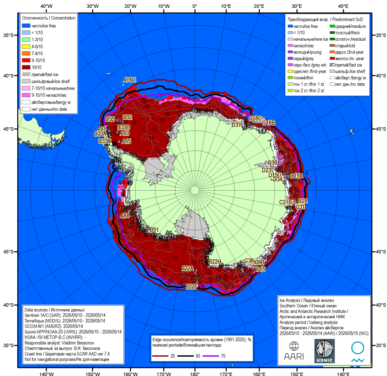
Рисунок 7а – Ледовая карта Южного океана (цветовая окраска по общей сплоченности) и расположение крупных айсбергов на основе ледового анализа за 14.05.2026 в рамках проекта совместного ледового картирования Южного океана ААНИИ, НЛЦ США и НМИ и повторяемость кромки за ближайшую пентаду за период 1991-2020 гг. по наблюдениям SSMR-SSM/I-SSMIS (алгоритм NASATEAM) [5, 10, 17, 21]
