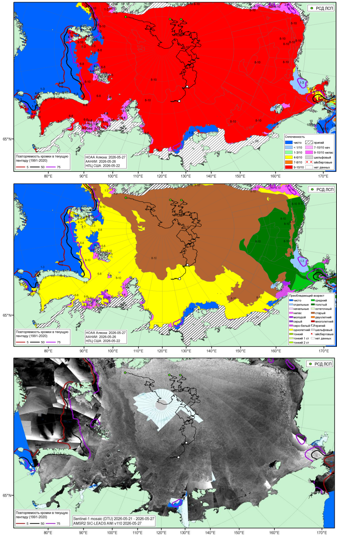
Рисунок 3 - Обзорная ледовая карта СМП за 22.05-27.05.2026 г., мозаика радиолокационных снимком ИСЗ Sentinel-1AC за 21.05-27.05.2026 (DTU) с оценкой положения польшей за 27.05.2026 г. по данным AMSR2 (AWI-JAXA), повторяемость кромки за соответствующий 5-дневный период 1991-2020 гг. по наблюдениям SSMR-SSM/I-SSMIS (алгоритм NASATEAM) и положение РСН СП-42 на 28.05.2026 0600МСК [27, 28, 17].
