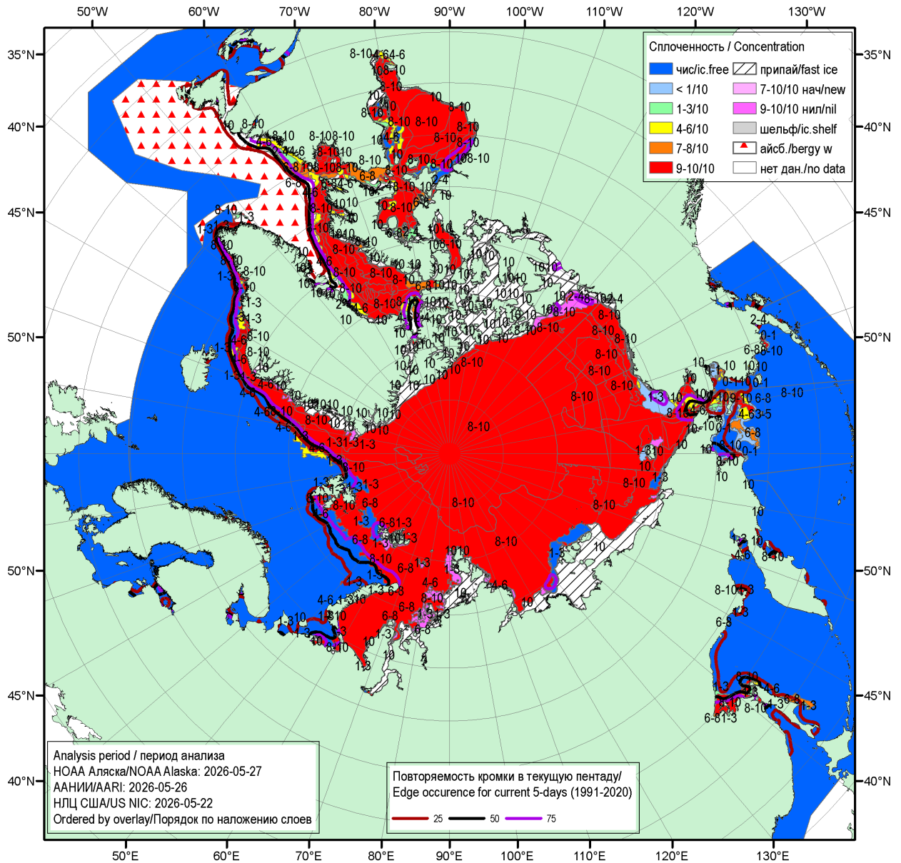
Рисунок 1а – Обзорная ледовая карта СЛО за 22.05.2026 – 27.05.2026 (цветовая раскраска по общей сплоченности) на основе ледового анализа NOAA Аляска, ААНИИ и Национального ледового центра США и повторяемость кромки за соответствующий 5-дневный период за 1991-2020 гг. по наблюдениям SSMR-SSM/I-SSMIS (алгоритм NASATEAM) [4, 10, 23, 17].
