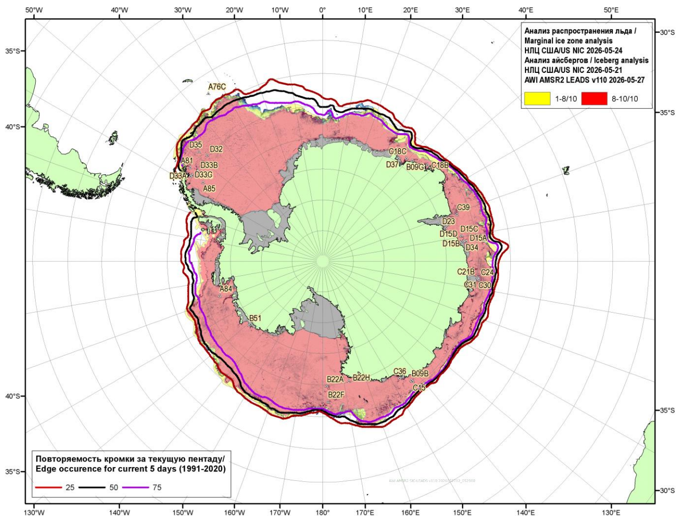
Рисунок 7в – Положение кромки льда и зон разреженных ( < 8/10 ) и сплоченных ( \geq 8/10 ) льдов Южного океана за 24.05.2026 и расположение крупных айсбергов за 21.05.2026 на основе ледового анализа Национального Ледового Центра США, повторяемость кромки за ближайшую пентаду за период 1991-2020 гг. по наблюдениям SSMR-SSM/I-SSMIS (алгоритм NASATEAM), совмещенное с положением разрежений на основе данных ИСЗ AMSR2 за 27.05.2026 (AWI-JAXA, v110) [10, 17, 24]
