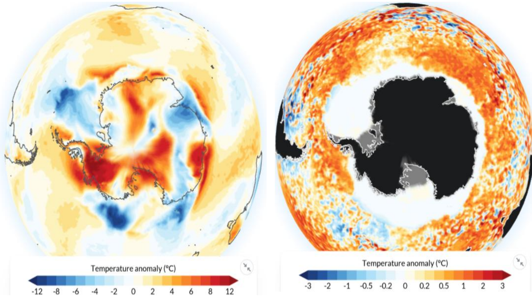
Рисунок 9 – Аномалия приземной температуры воздуха (2м) на 26.05.2026 г. относительно периода 1991-2020 гг. - The Copernicus Climate Change Service (C3S) , implemented by the European Centre for Medium-Range Weather Forecasts (ECMWF) on behalf of the European Commission is part of the European Union's space programme.
