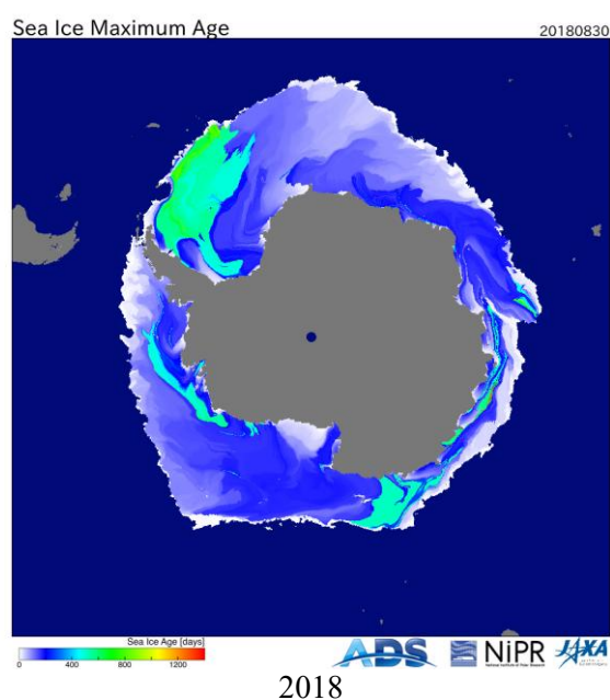
Рисунок 86 – Оценка максимального возраста льда (сутки) на 30.08 за 2018 – 2026 гг. по данным JAXA-NIPR [29]
