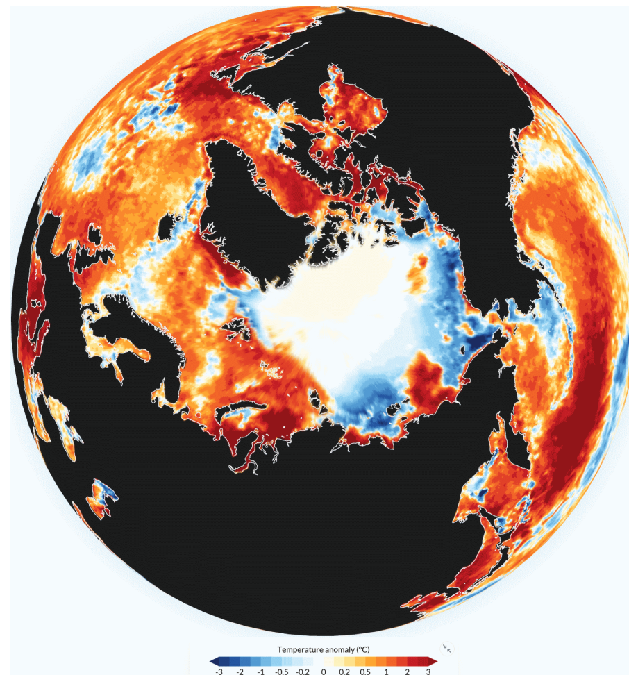
Рисунок 5а – Аномалия приземной температуры воздуха (2м) и температуры поверхности моря на 31.08.2026 г. относительно периода 1991-2020 гг. - The Copernicus Climate Change Service (C3S) , implemented by the European Centre for Medium-Range Weather Forecasts (ECMWF) on behalf of the European Commission is part of the European Union's space programme
