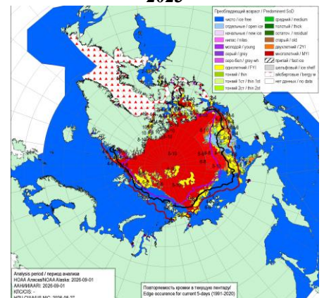
Рисунок 4а – Ледовые условия за 27.08 - 01.09.2026. и аналогичные периоды 2007-2025 гг. на основе ледового анализа ААНИИ, НИЦ Планета, Канадской ледовой службы, Национального ледового центра США и НОАА Аляска [4, 10, 12, 23, 17].
