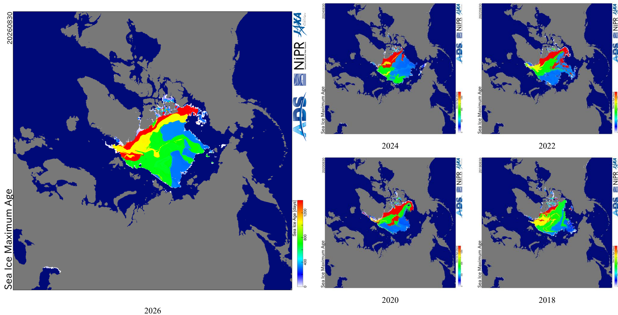
Рисунок 46 – Оценка максимального возраста льда (сутки) на 30.08 за 2018 – 2026 гг. по данным JAXA-NIPR [29]
