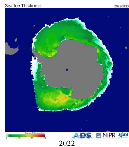
Рисунок 8а - Оценка толщины льда на основе данных пассивного микроволнового зондирования AMSR2 30.08 в 2018 – 2026 гг. [29].
