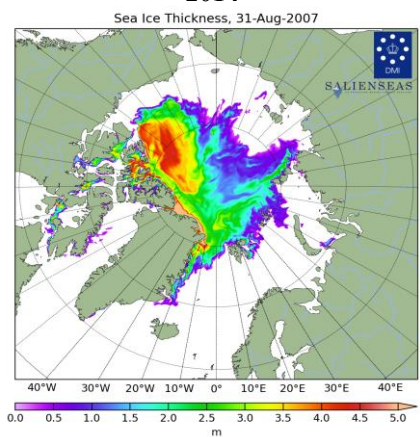
Рисунок 4в – Поля распределения средневзвешенной толщины льда совместной модели морского льда – океана HYCOM/CICE Датского метеорологического института 31.08 за 2005-2026 гг. [22].
