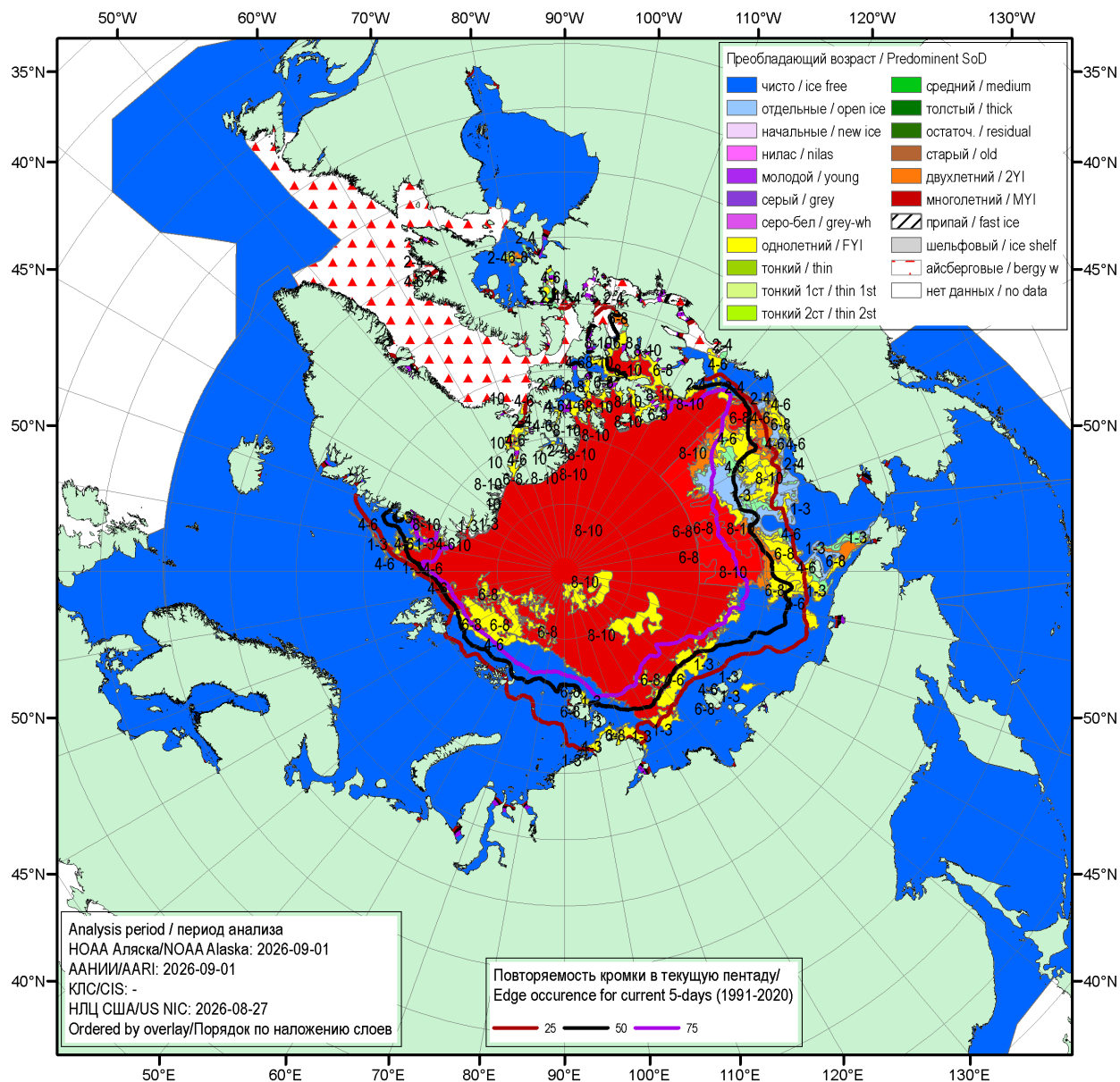
Рисунок 1а – Обзорная ледовая карта СЛО за 27.08.2026 – 01.09.2026 (цветовая раскраска по общей сплоченности) на основе ледового анализа НОАА Аляска, ААНИИ и Национального ледового центра США и повторяемость кромки за соответствующий 5-дневный период за 1991-2020 гг. по наблюдениям SSMR-SSM/I-SSMIS (алгоритм NASATEAM) [4, 10, 23, 17].
