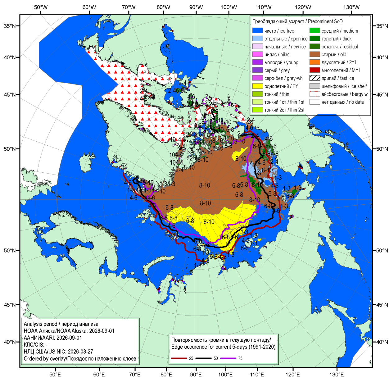
Рисунок 16 – Обзорная ледовая карта СЛО за 27.08.2026 – 01.09.2026 (цветовая раскраска по преобладающему возрасту) на основе ледового анализа NOAA Аляска, ААНИИ и Национального ледового центра США и повторяемость кромки за соответствующий 5-дневный период за 1991-2020 гг. по наблюдениям SSMR-SSM/I-SSMIS (алгоритм NASATEAM) [4, 10, 23, 17].
