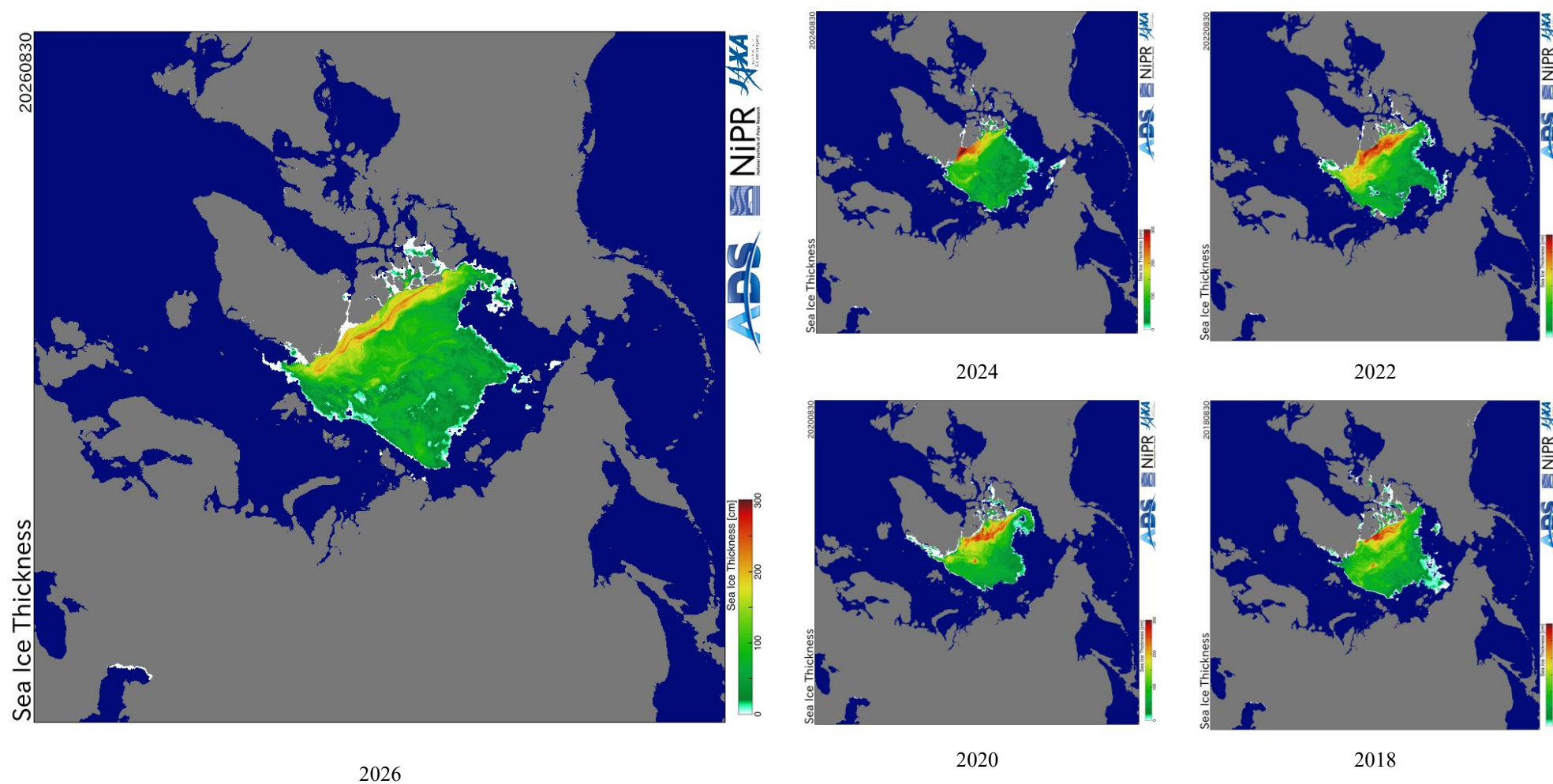
Рисунок 2а - Оценка толщины льда на основе данных пассивного микроволнового зондирования AMSR2 30.08 в 2018 – 2026 гг. [29].
