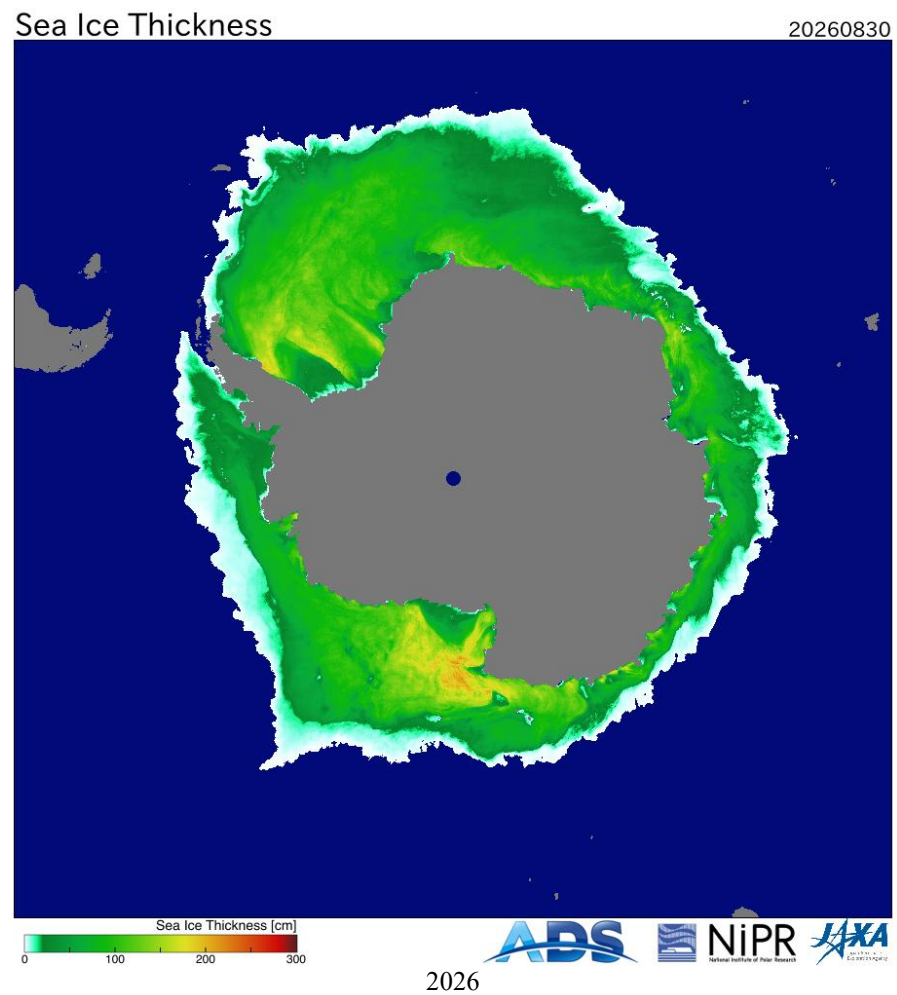
Рисунок 8а - Оценка толщины льда на основе данных пассивного микроволнового зондирования AMSR2 30.08 в 2018 – 2026 гг. [29].
