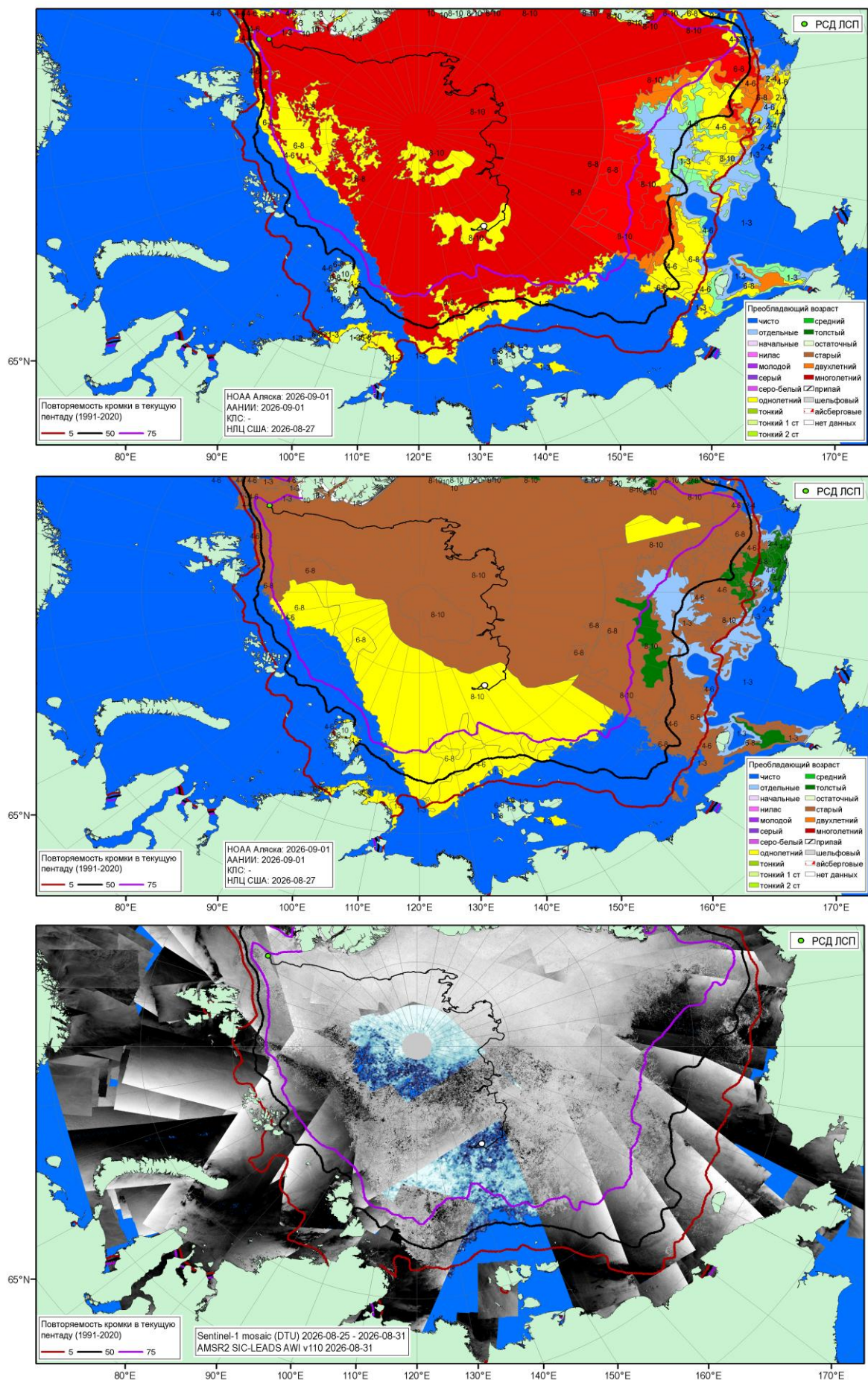
Рисунок 3 - Обзорная ледовая карта ЧМП за 27.08-01.09.2026 г., мозаика радиолокационных снимком ИСЗ Sentinel-1AC за 25.08-31.08.2026 (DTU) с оценкой положения полыней за 31.08.2026 г. по данным AMSR2 (AWI-JAXA), повторяемость кромки за соответствующий 5-дневный период 1991-2020 гг. по наблюдениям SSMR-SSM/I-SSMIS (алгоритм NASATEAM) и положение РСН СП-42 на 01.09.2026 0600МСК [27, 28, 17].
