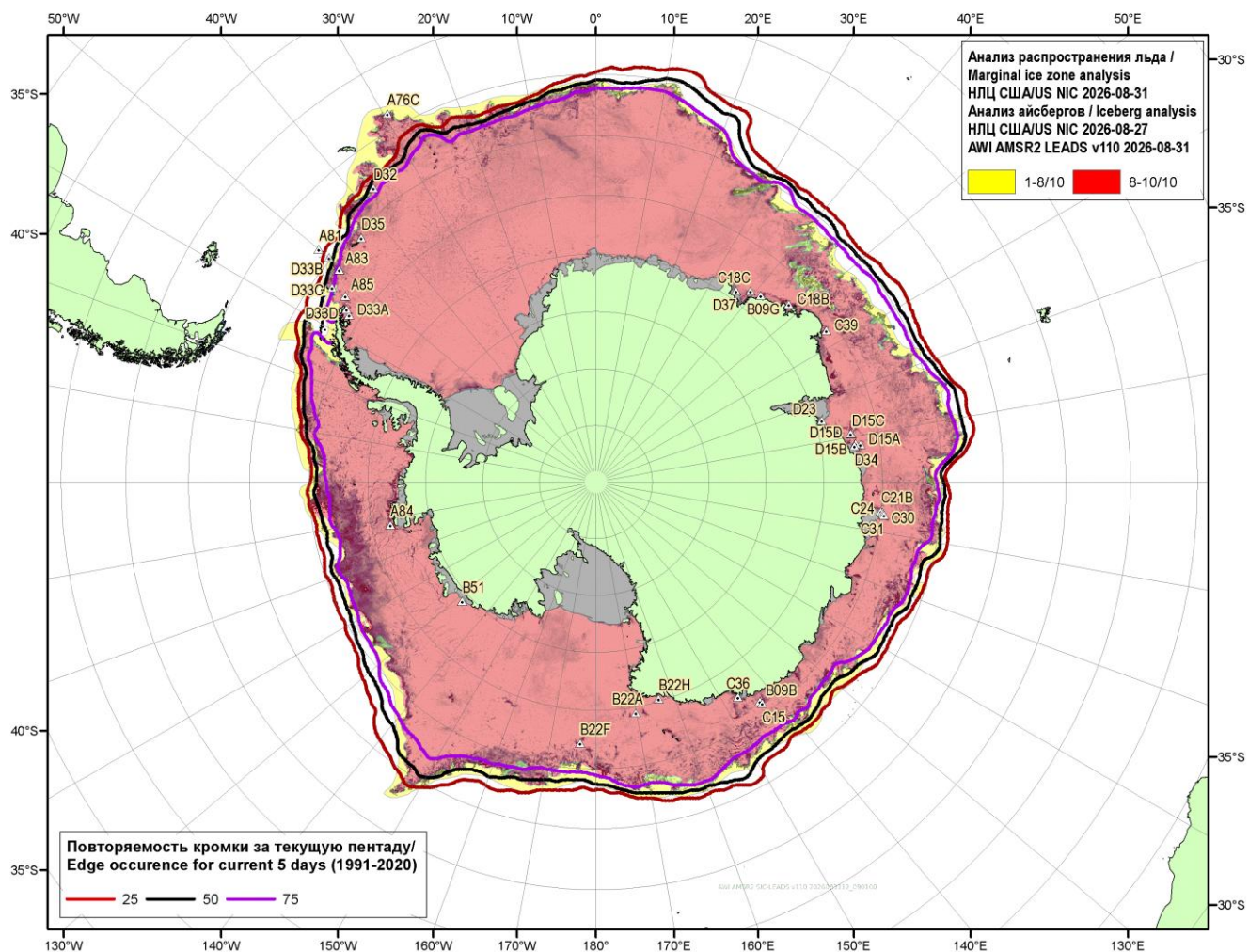
Рисунок 7в – Положение кромки льда и зон разреженных ( <8/10 ) и сплошных ( \geq 8/10 ) льдов Южного океана за 31.08.2026 и расположение крупных айсбергов за 27.08.2026 на основе ледового анализа Национального Ледового Центра США, повторяемость кромки за ближайшую пентаду за период 1991-2020 гг. по наблюдениям SSMR-SSM/I-SSMIS (алгоритм NASATEAM), совмещенное с положением разрежений на основе данных ИСЗ AMSR2 за 31.08.2026 (AWI-JAXA, v110) [10, 17, 24]
