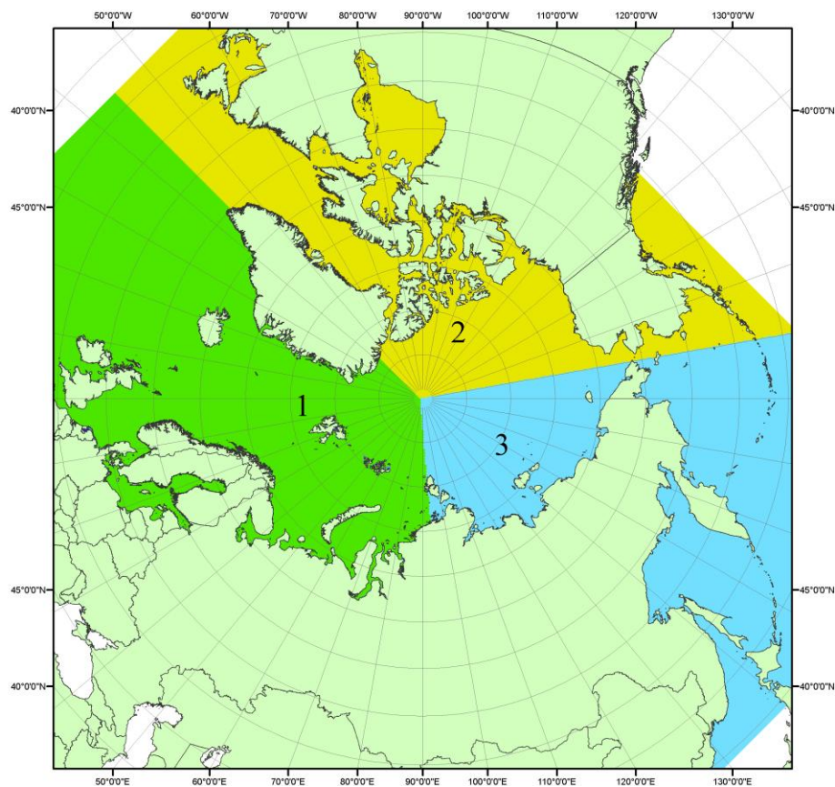
Рисунок П1 – Секторальное деление северной полярной области. 1 - Сектор 45^{\circ} W- 95^{\circ} E (Гренландское - Карское моря); 2 - Сектор 170^{\circ} W- 45^{\circ} W (море Бофорта и Канадская Арктика); 3 - Сектор 95^{\circ} E- 170^{\circ} W (моря Лаптевых - Чукотское, Берингово, Охотское, Японское)
