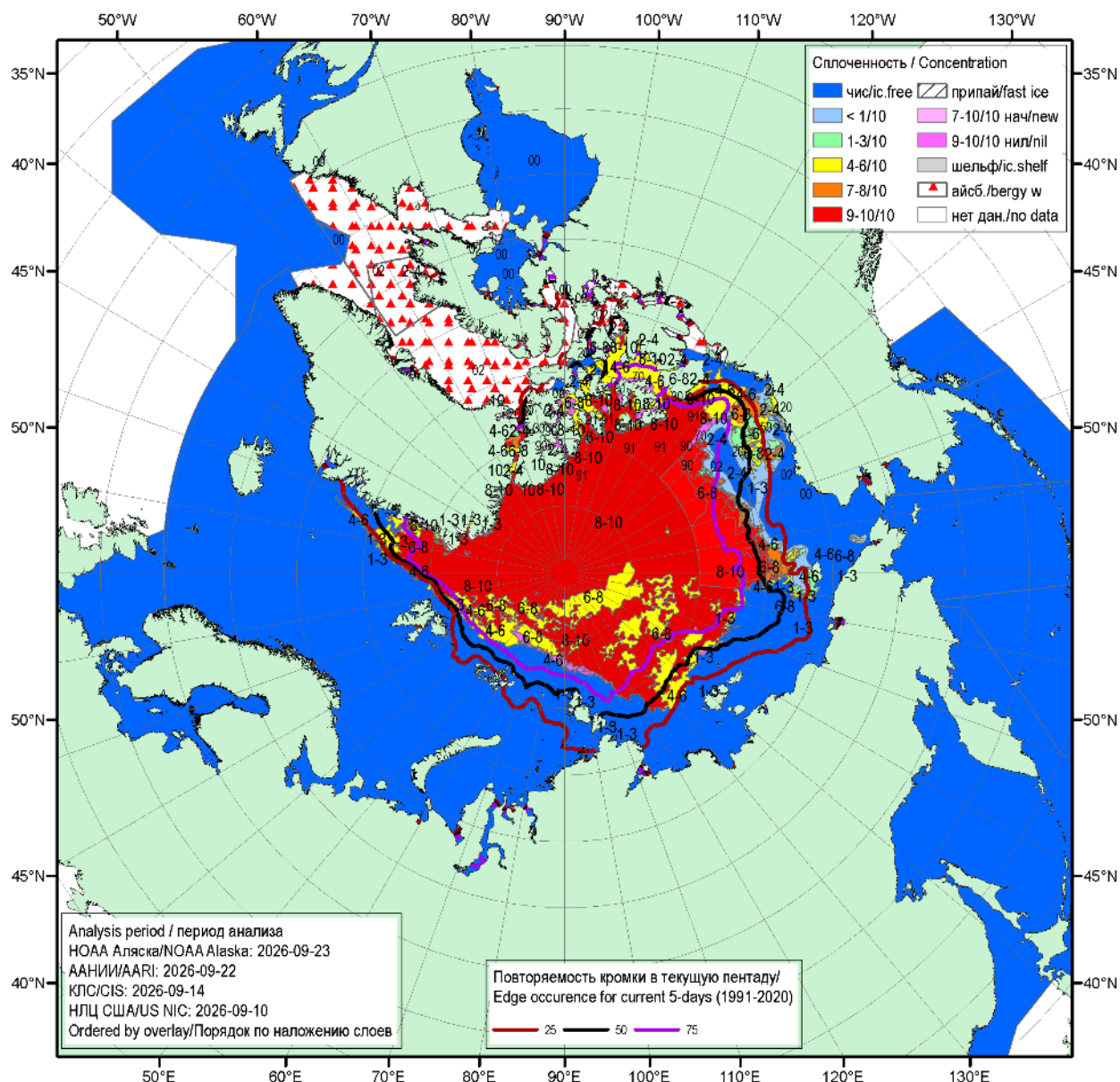
Рисунок 1а – Обзорная ледовая карта СЛО за 10.09.2026 – 23.09.2026 (цветовая раскраска по общей сплоченности) на основе ледового анализа NOAA Аляска, ААНИИ, Канадской ледовой службы и Национального ледового центра США и повторяемость кромки за соответствующий 5-дневный период за 1991-2020 гг. по наблюдениям SSMR-SSM/I-SSMIS (алгоритм NASATEAM) [4, 10, 23, 17].
