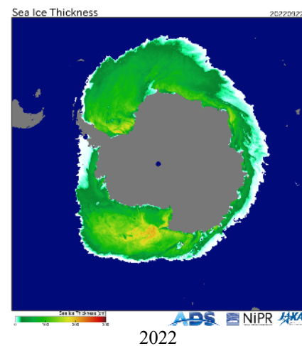
Рисунок 8а - Оценка толщины льда на основе данных пассивного микроволнового зондирования AMSR2 22.09 в 2018 – 2026 гг. [29].
