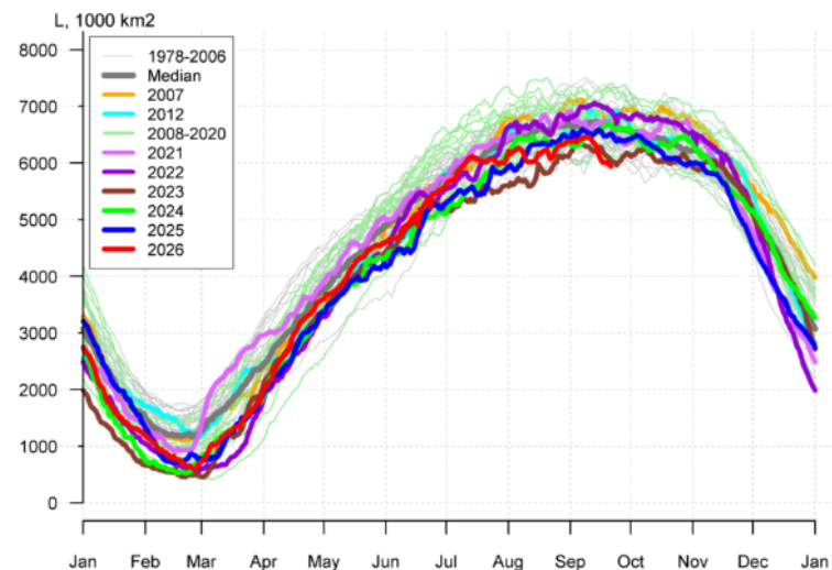
Рисунок 10а – Ежедневные оценки сезонного хода ледовитости Южного Океана и меридиональных секторов за период 26.10.1978 – последний доступный срок по годам на основе расчетов по данным SSMR-SSM/I-SSMIS, алгоритм NASATEAM: а) Южный Океан, б) Атлантический сектор (60°W-30°E, море Уэдделла), в) Индоокеанский сектор (30°E-150°E, моря Космонавтов, Содружества, Моусона), г) Тихоокеанский сектор (150°E-60°W, моря Росса, Беллингаузена) [13-17]
