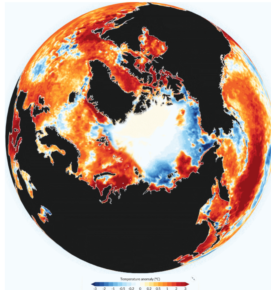
Рисунок 5а – Аномалия приземной температуры воздуха (2м) и температуры поверхности моря на 22.09.2026 г. относительно периода 1991-2020 гг. - The Copernicus Climate Change Service (C3S) , implemented by the European Centre for Medium-Range Weather Forecasts (ECMWF) on behalf of the European Commission is part of the European Union's space programme
