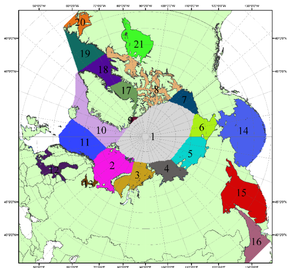
Рисунок П3 – моря северной полярной области. 1 – Арктический бассейн; 2 – Баренцево море; 3 – Карское море; 4 – море Лаптевых; 5 – Восточно-Сибирское море; 6 – Чукотское море; 7 – море Бофорта; 8 – Канадский архипелаг; 9 – море Линкольна; 10 – Гренландское море; 11 – Норвежское море; 12 – Балтийское море; 13 – Белое море; 14 – Берингово море; 15 – Охотское море; 16 – Японское море; 17 – море Баффина; 18 – Дейвисов пролив; 19 – море Лабрадор; 20 – залив Святого Лаврентия; 21 – Гудзонов залив.
