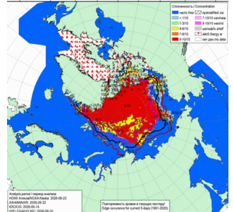
Рисунок 4а – Ледовые условия за 10.09 - 23.09.2026. и аналогичные периоды 2007-2025 гг. на основе ледового анализа ААНИИ, НИЦ Планета, Канадской ледовой службы, Национального ледового центра США и НОАА Аляска [4, 10, 12, 23, 17].
