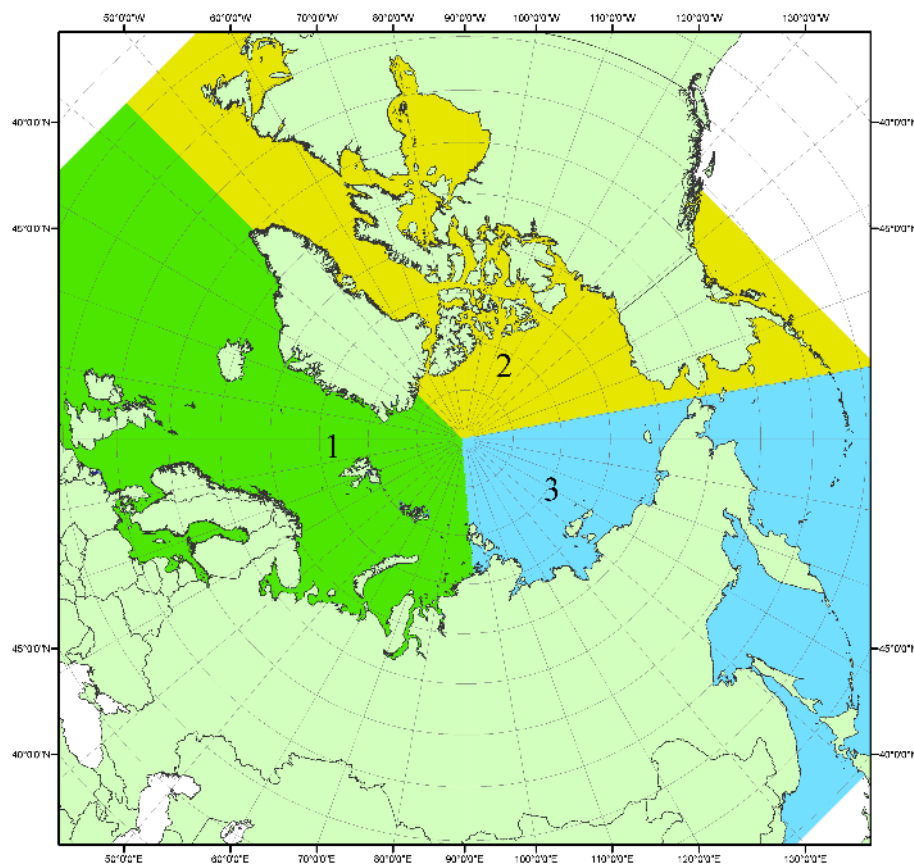
Рисунок П1 – Секторальное деление северной полярной области. 1 - Сектор 45^\circ\text{W} - 95^\circ\text{E} (Гренландское - Карское моря); 2 - Сектор 170^\circ\text{W} - 45^\circ\text{W} (море Бофорта и Канадская Арктика); 3 - Сектор 95^\circ\text{E} - 170^\circ\text{W} (моря Лаптевых - Чукотское, Берингово, Охотское, Японское)
