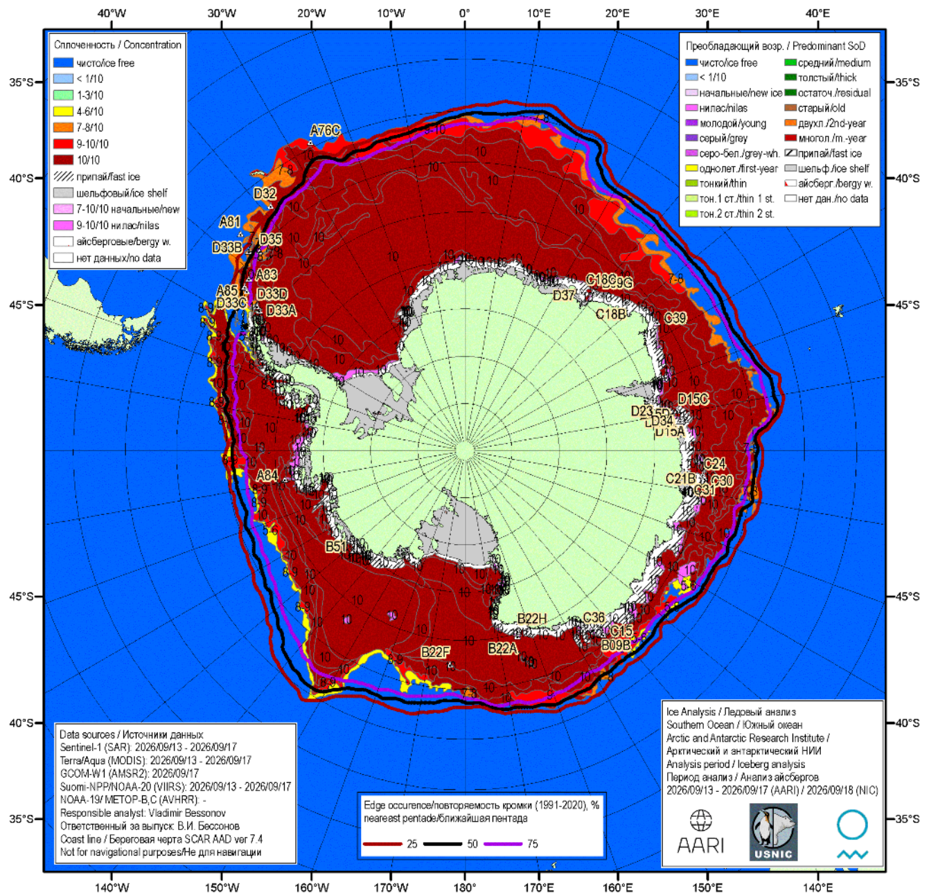
Рисунок 7а – Ледовая карта Южного океана (цветовая окраска по общей сплоченности) и расположение крупных айсбергов на основе ледового анализа за 17.09.2026 в рамках проекта совместного ледового картирования Южного океана ААНИИ, НЛЦ США и НМИ и повторяемость кромки за ближайшую пентаду за период 1991-2020 гг. по наблюдениям SSMR-SSM/I-SSMIS (алгоритм NASATEAM) [5, 10, 17, 21]
