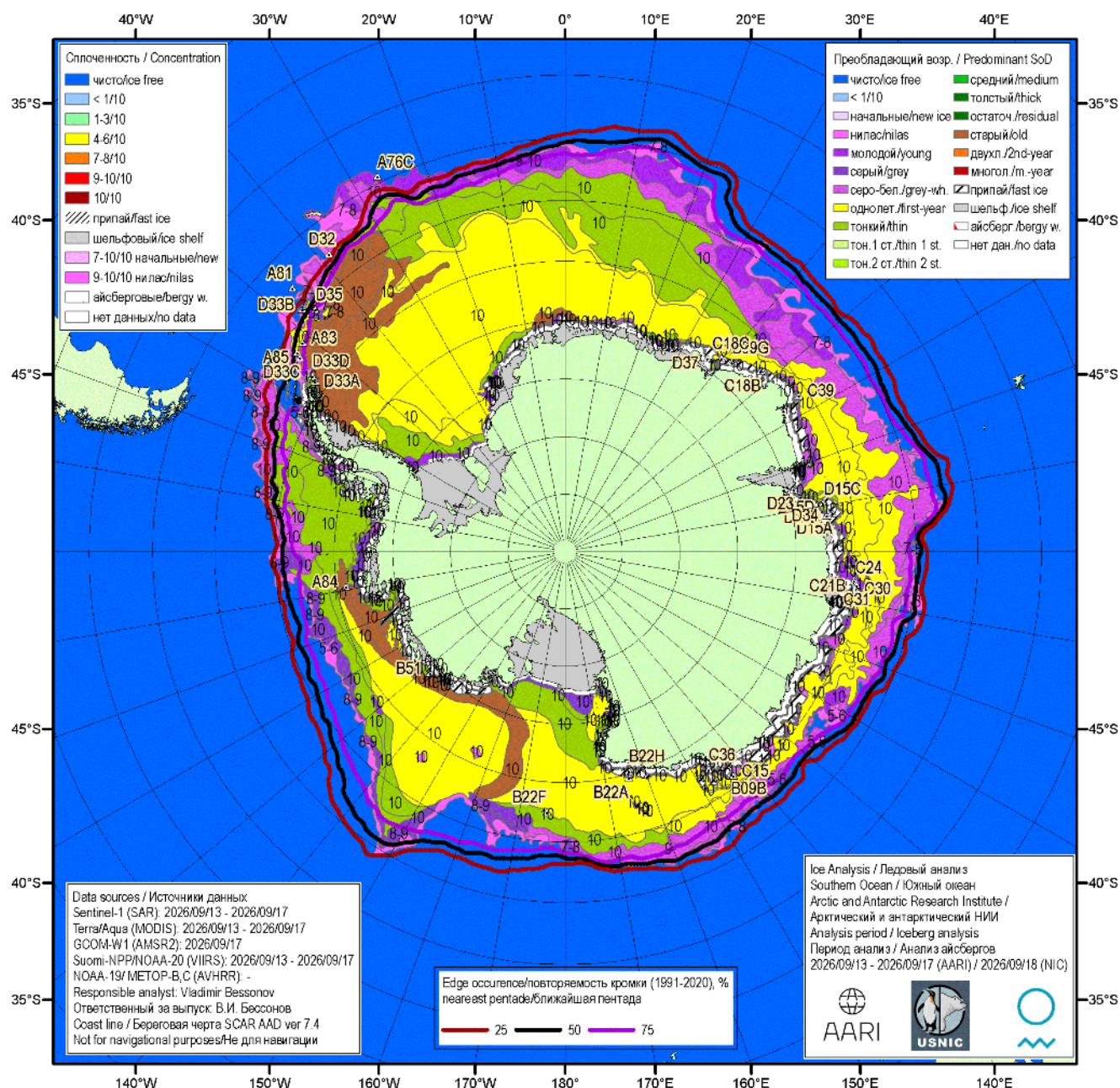
Рисунок 76 – Ледовая карта Южного океана (цветовая окраска по возрасту) и расположение крупных айсбергов на основе ледового анализа за 17.09.2026 в рамках проекта совместного ледового картирования Южного океана ААНИИ, НЛЦ США и НМИ и повторяемость кромки за ближайшую пентаду за период 1991-2020 гг. по наблюдениям SSMR-SSM/I-SSMIS (алгоритм NASATEAM) [5, 10, 17, 21].
