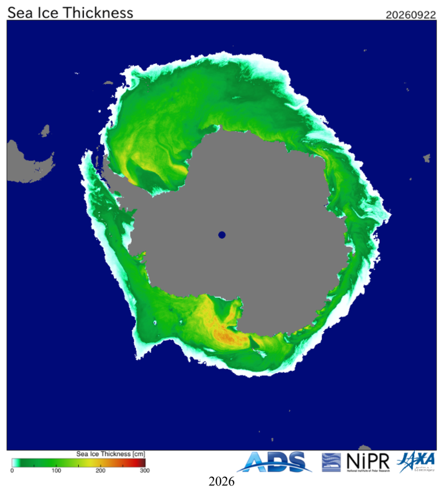
Рисунок 8а - Оценка толщины льда на основе данных пассивного микроволнового зондирования AMSR2 22.09 в 2018 – 2026 гг. [29].
