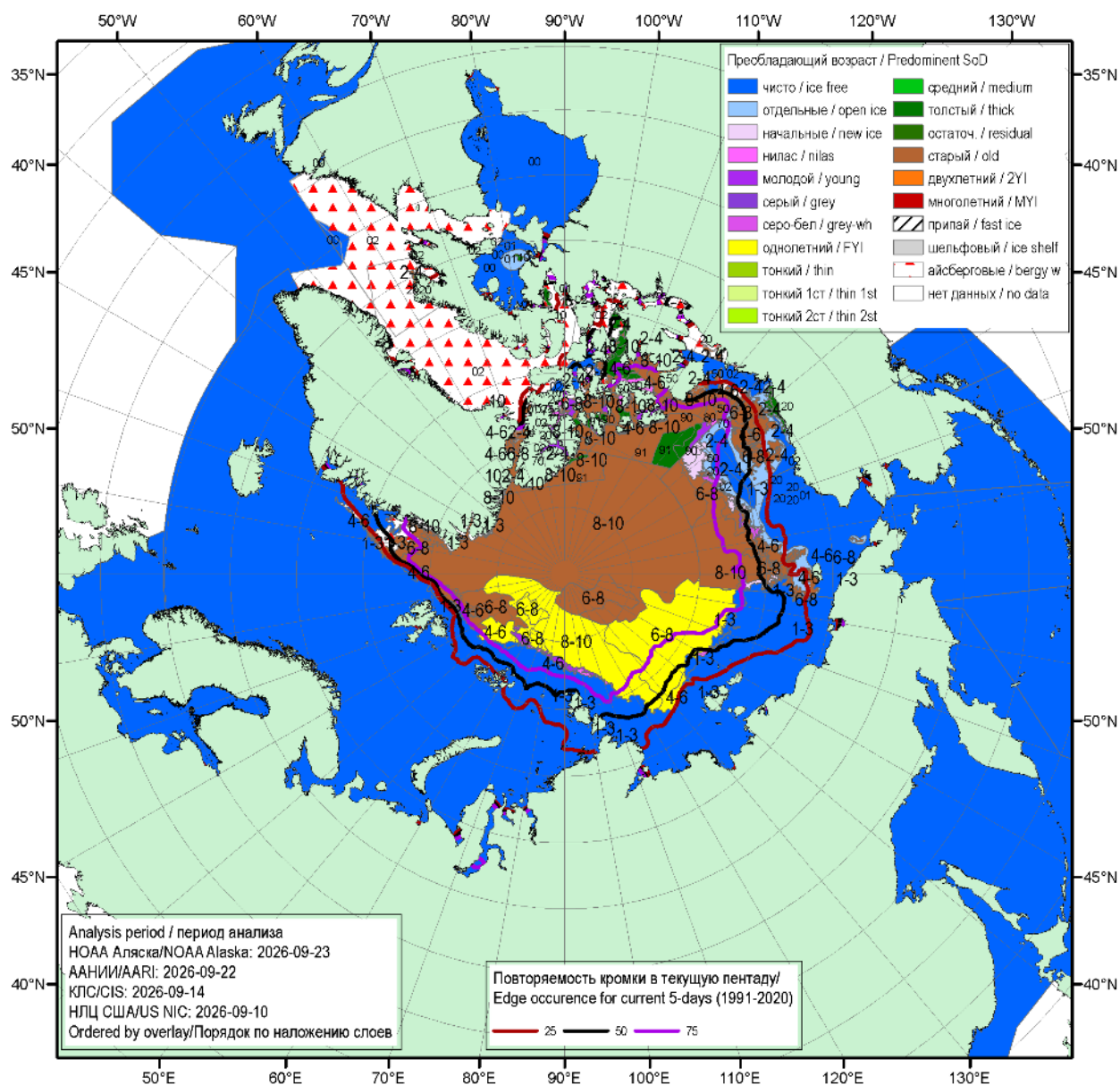
Рисунок 16 – Обзорная ледовая карта СЛО за 10.09.2026 – 23.09.2026 (цветовая раскраска по преобладающему возрасту) на основе ледового анализа НОАА Аляска, ААНИИ, Канадской ледовой службы и Национального ледового центра США и повторяемость кромки за соответствующий 5-дневный период за 1991-2020 гг. по наблюдениям SSMR-SSM/I-SSMIS (алгоритм NASATEAM) [4, 10, 23, 17].
