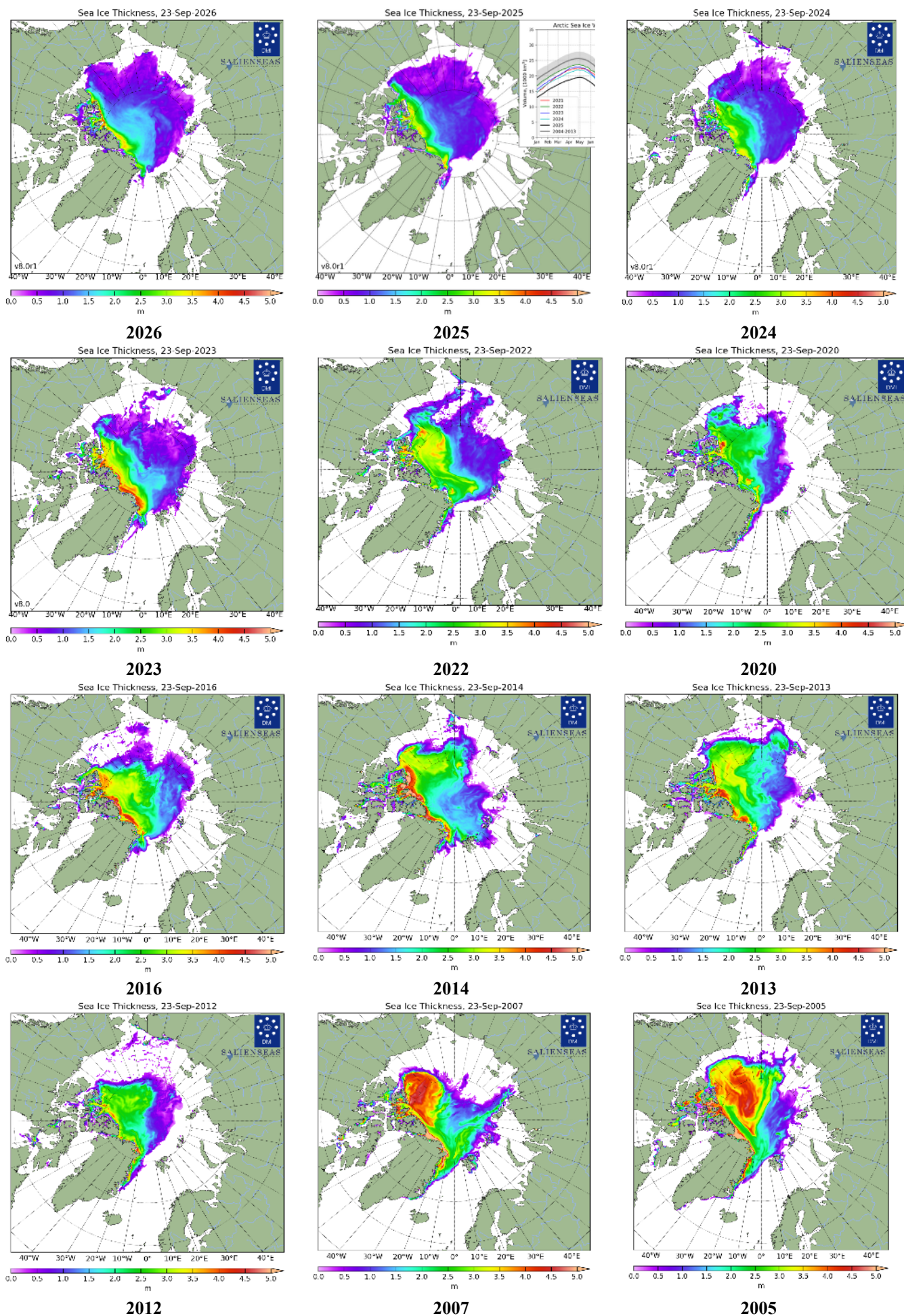
Рисунок 4в – Поля распределения средневзвешенной толщины льда совместной модели морского льда – океана HYCOM/CICE Датского метеорологического института 23.09 за 2005-2026 гг. [22].
