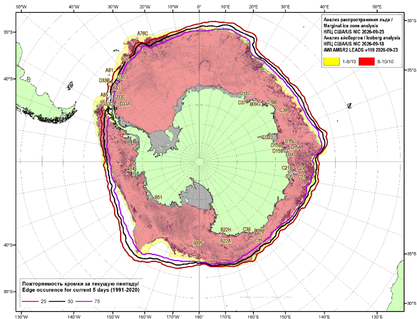
Рисунок 7в – Положение кромки льда и зон разреженных ( <8/10 ) и сплоченных ( \geq 8/10 ) льдов Южного океана за 23.09.2026 и расположение крупных айсбергов за 18.09.2026 на основе ледового анализа Национального Ледового Центра США, повторяемость кромки за ближайшую пентаду за период 1991-2020 гг. по наблюдениям SSMR-SSM/I-SSMIS (алгоритм NASATEAM), совмещенное с положением разрежений на основе данных ИСЗ AMSR2 за 23.09.2026 (AWI-JAXA, v110) [10, 17, 24]
