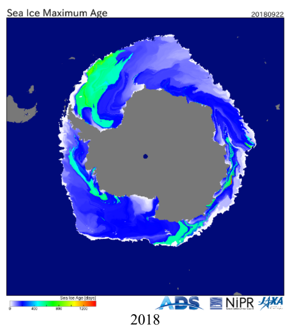
Рисунок 86 – Оценка максимального возраста льда (сутки) на 22.09 за 2018 – 2026 гг. по данным JAXA-NIPR [29]
