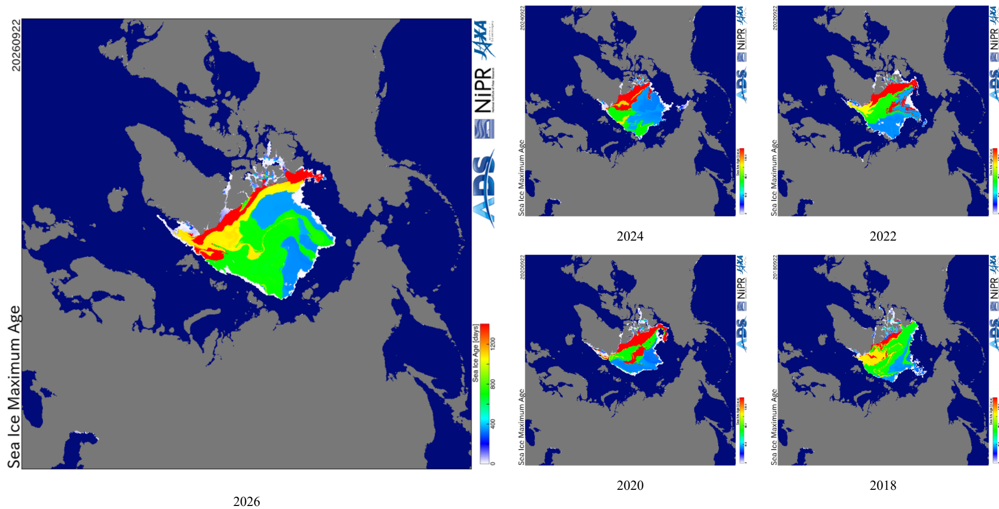
Рисунок 46 – Оценка максимального возраста льда (сутки) на 22.09 за 2018 – 2026 гг. по данным JAXA-NIPR [29]
