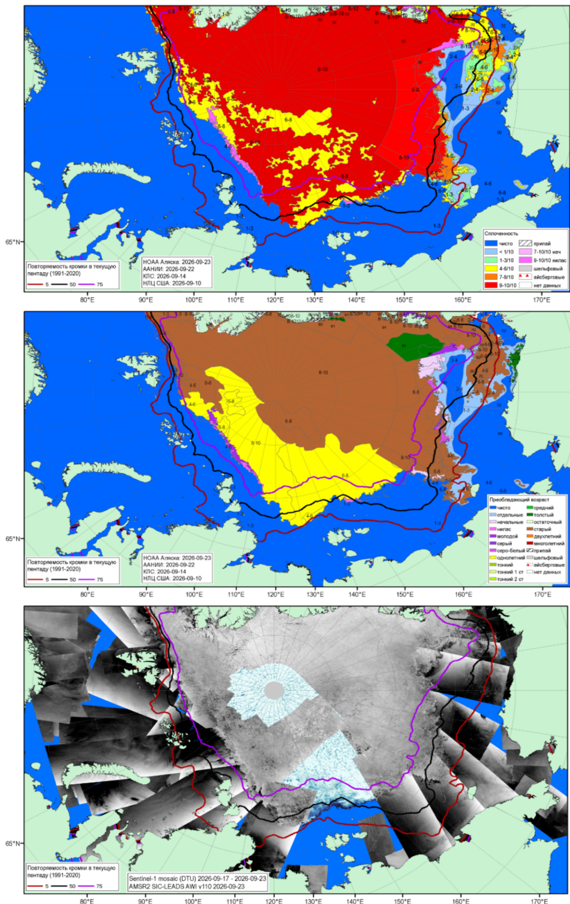
Рисунок 3 - Обзорная ледовая карта МП за 10.09-23.09.2026 г., мозаика радиолокационных снимком ИСЗ Sentinel-1AC за 17.09-23.09.2026 (DTU) с оценкой положения полыней за 23.09.2026 г. по данным AMSR2 (AWI-JAXA), повторяемость кромки за соответствующий 5-дневный период 1991-2020 гг. по наблюдениям SSMR-SSM/I-SSMIS (алгоритм NASATEAM) и положение РЧН СП-42 на 24.09.2026 0600МСК [27, 28, 17].
