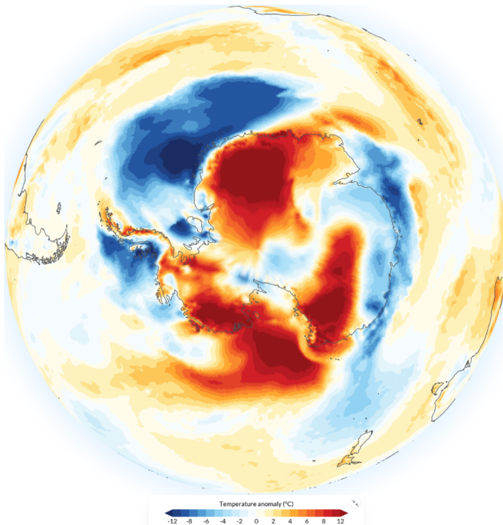
Рисунок 9 – Аномалия приземной температуры воздуха (2м) на 22.09.2026 г. относительно периода 1991-2020 гг. - The Copernicus Climate Change Service (C3S) , implemented by the European Centre for Medium-Range Weather Forecasts (ECMWF) on behalf of the European Commission is part of the European Union's space programme.
