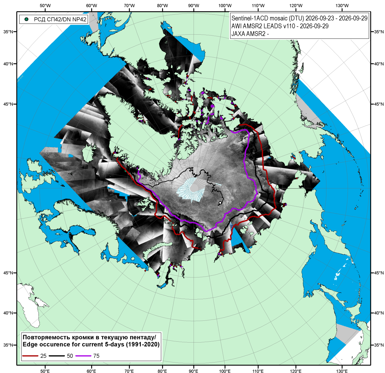
Рисунок 1в – Мозаика снимков Sentinel-1CD (DTU) за 23.09.2026 – 29.09.2026, общая сплоченность и оценка положения полыней за 29.09.2026 г. по данным AMSR2 (AWI-JAXA), повторяемость кромки за соответствующий 5-дневный период за 1991-2020 гг. по наблюдениям SSMR-SSM/I-SSMIS (алгоритм NASATEAM) и положение РСН СП-42 на 30.09.2025 г. 06:00МСК.
