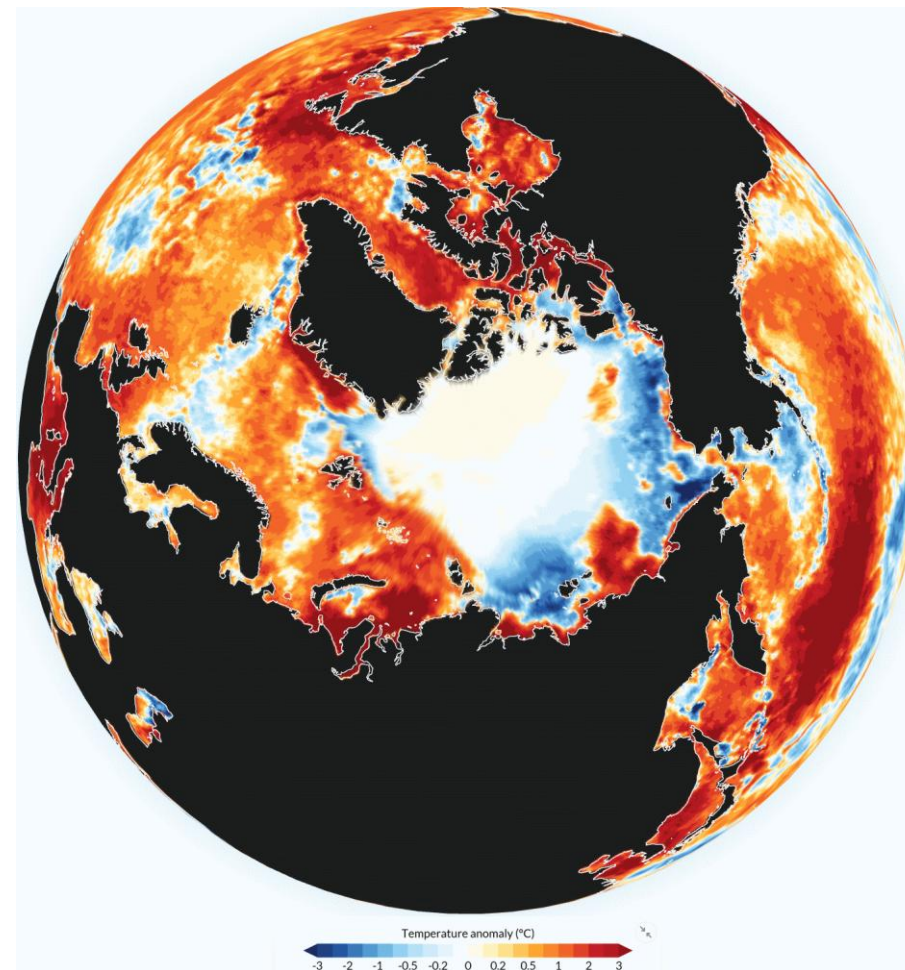
Рисунок 5а – Аномалия приземной температуры воздуха (2м) и температуры поверхности моря на 28.09.2026 г. относительно периода 1991-2020 гг. - The Copernicus Climate Change Service (C3S) , implemented by the European Centre for Medium-Range Weather Forecasts (ECMWF) on behalf of the European Commission is part of the European Union's space programme
