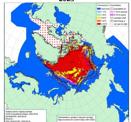
Рисунок 4а – Ледовые условия за 24.09 - 29.09.2026. и аналогичные периоды 2007-2025 гг. на основе ледового анализа ААНИИ, НИЦ Планета, Канадской ледовой службы, Национального ледового центра США и НОАА Аляска [4, 10, 12, 23, 17].
