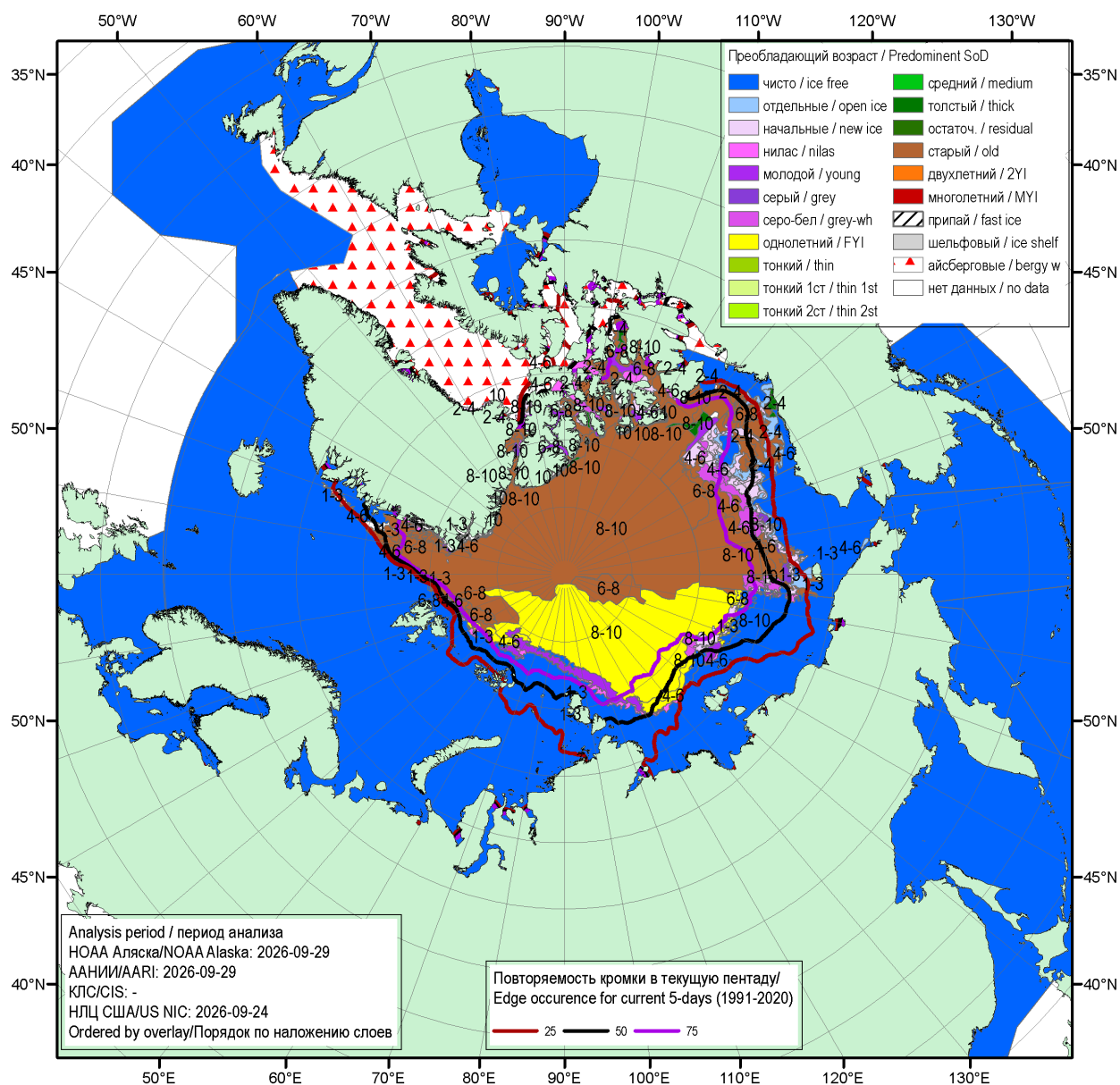
Рисунок 16 – Обзорная ледовая карта СЛО за 24.09.2026 – 29.09.2026 (цветовая раскраска по преобладающему возрасту) на основе ледового анализа НОАА Аляска, ААНИИ и Национального ледового центра США и повторяемость кромки за соответствующий 5-дневный период за 1991-2020 гг. по наблюдениям SSMR-SSM/I-SSMIS (алгоритм NASATEAM) [4, 10, 23, 17].
