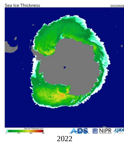
Рисунок 8а - Оценка толщины льда на основе данных пассивного микроволнового зондирования AMSR2 28.09 в 2018 – 2026 гг. [29].
