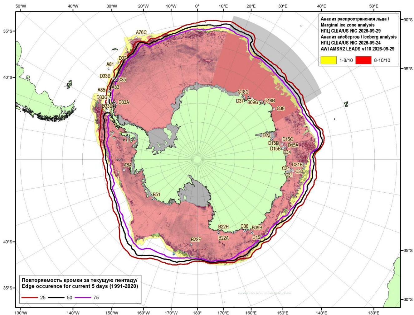
Рисунок 7в – Положение кромки льда и зон разреженных ( <8/10 ) и сплошных ( \geq 8/10 ) льдов Южного океана за 29.09.2026 и расположение крупных айсбергов за 24.09.2026 на основе ледового анализа Национального Ледового Центра США, повторяемость кромки за ближайшую пентаду за период 1991-2020 гг. по наблюдениям SSMR-SSM/I-SSMIS (алгоритм NASATEAM), совмещенное с положением разрежений на основе данных ИСЗ AMSR2 за 29.09.2026 (AWI-JAXA, v110) [10, 17, 24]
