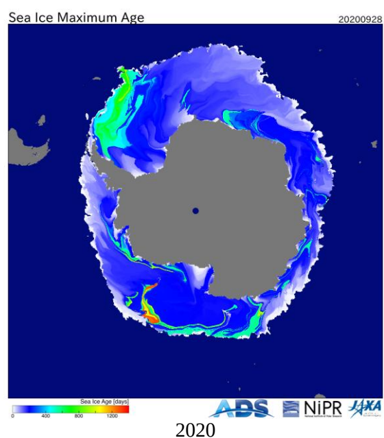
Рисунок 86 – Оценка максимального возраста льда (сутки) на 28.09 за 2018 – 2026 гг. по данным JAXA-NIPR [29]
