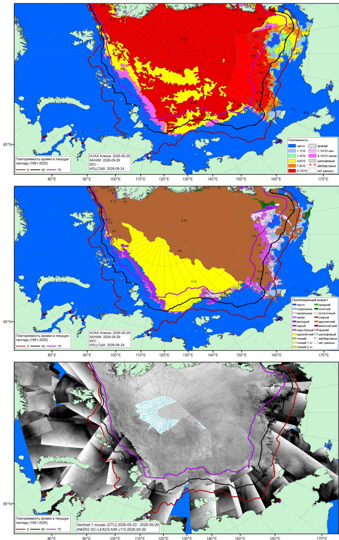
Рисунок 3 - Обзорная ледовая карта ЦМП за 24.09-29.09.2026 г., мозаика радиолокационных снимком ИСЗ Sentinel-1AC за 23.09-29.09.2026 (DTU) с оценкой положения полыней за 29.09.2026 г. по данным AMSR2 (AWI-JAXA), повторяемость кромки за соответствующий 5-дневный период 1991-2020 гг. по наблюдениям SSMR-SSM/I-SSMIS (алгоритм NASATEAM) и положение РСН СП-42 на 30.09.2026 0600МСК [27, 28, 17].
