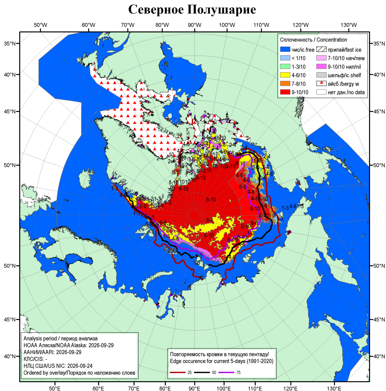
Рисунок 1а – Обзорная ледовая карта СЛО за 24.09.2026 – 29.09.2026 (цветовая раскраска по общей сплоченности) на основе ледового анализа NOAA Аляска, ААНИИ и Национального ледового центра США и повторяемость кромки за соответствующий 5-дневный период за 1991-2020 гг. по наблюдениям SSMR-SSM/I-SSMIS (алгоритм NASATEAM) [4, 10, 23, 17].
