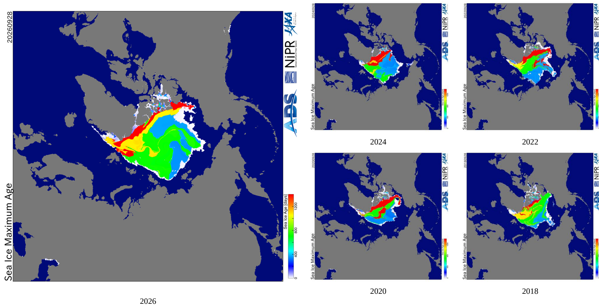
Рисунок 46 – Оценка максимального возраста льда (сутки) на 28.09 за 2018 – 2026 гг. по данным JAXA-NIPR [29]
