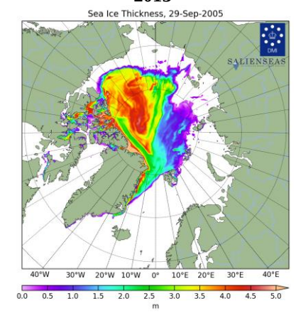
Рисунок 4в – Поля распределения средневзвешенной толщины льда совместной модели морского льда – океана HYCOM/CICE Датского метеорологического института 29.09 за 2005-2026 гг. [22].
