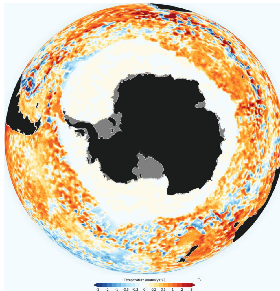
Рисунок 9 – Аномалия приземной температуры воздуха (2м) на 28.09.2026 г. относительно периода 1991-2020 гг. - The Copernicus Climate Change Service (C3S) , implemented by the European Centre for Medium-Range Weather Forecasts (ECMWF) on behalf of the European Commission is part of the European Union's space programme.
