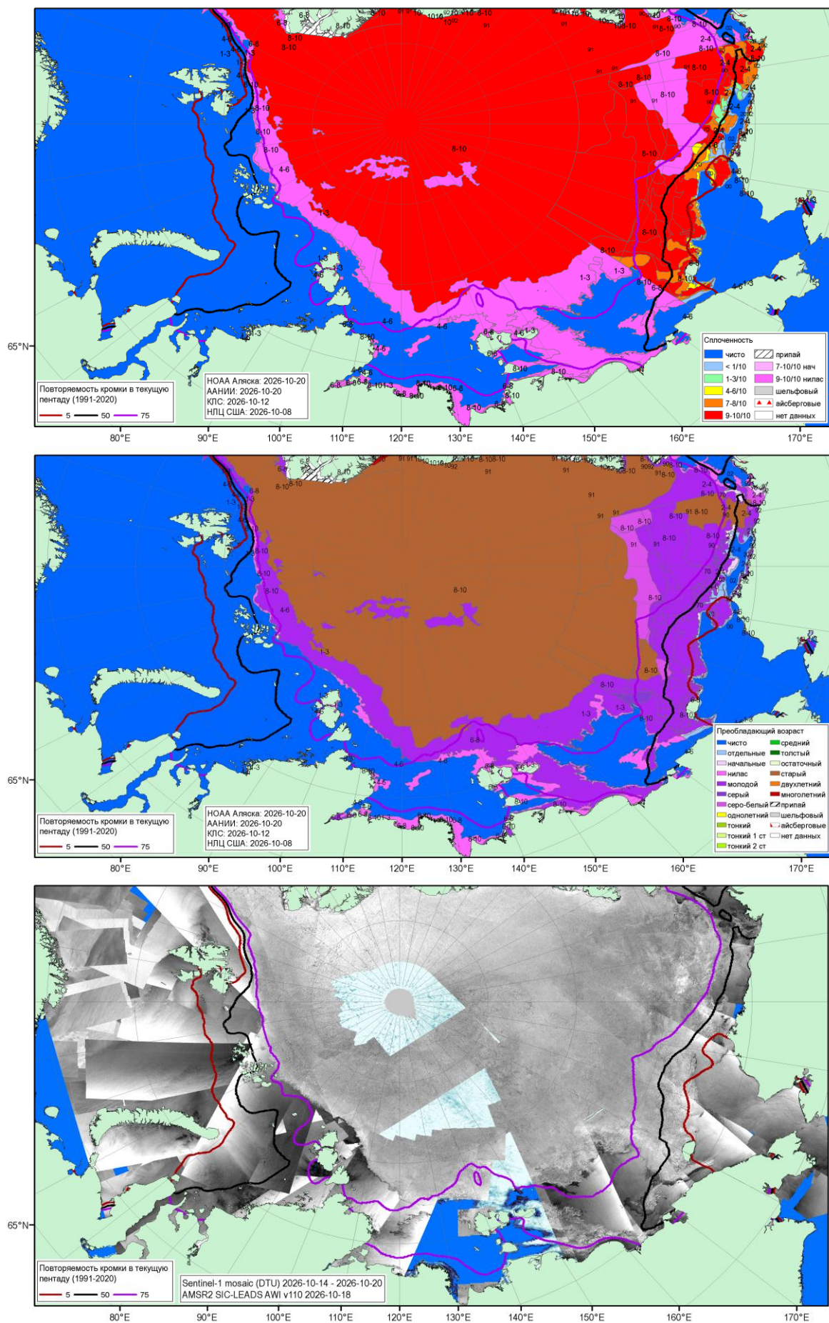
Рисунок 3 - Обзорная ледовая карта МП за 08.10-20.10.2026 г., мозаика радиолокационных снимком ИСЗ Sentinel-1AC за 14.10-20.10.2026 (DTU) с оценкой положения полыней за 18.10.2026 г. по данным AMSR2 (AWI-JAXA) и повторяемость кромки за соответствующий 5-дневный период 1991-2020 гг. по наблюдениям SSMR-SSM/I-SSMIS (алгоритм NASATEAM) [27, 28, 17].
