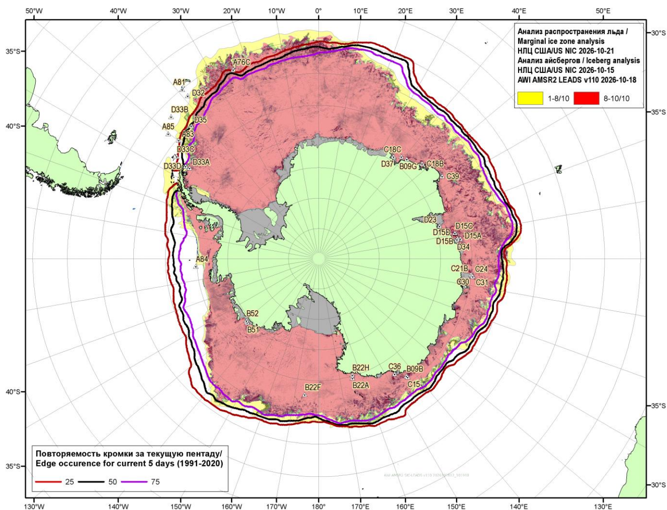
Рисунок 7в – Положение кромки льда и зон разреженных ( <8/10 ) и сплоченных ( \geq 8/10 ) льдов Южного океана за 21.10.2026 и расположение крупных айсбергов за 15.10.2026 на основе ледового анализа Национального Ледового Центра США, повторяемость кромки за ближайшую пентаду за период 1991-2020 гг. по наблюдениям SSMR-SSM/I-SSMIS (алгоритм NASATEAM), совмещенное с положением разрежений на основе данных ИСЗ AMSR2 за 18.10.2026 (AWI-JAXA, v110) [10, 17, 24]
