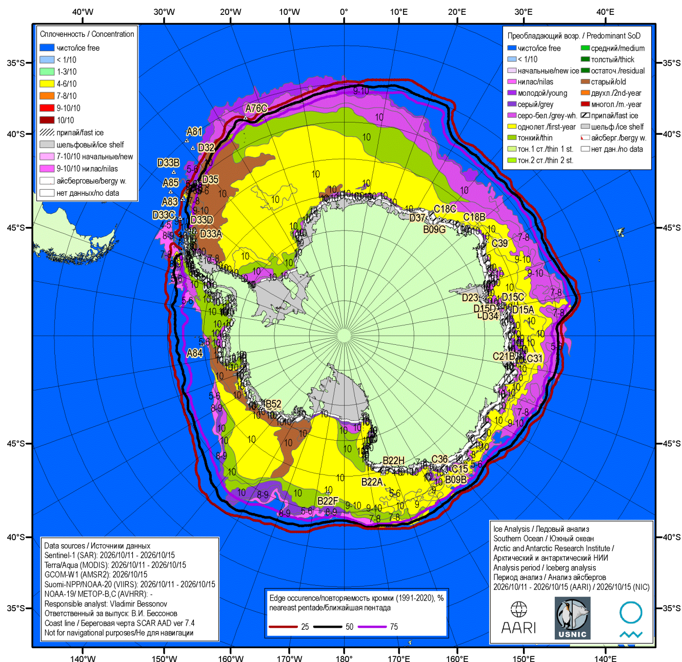
Рисунок 76 – Ледовая карта Южного океана (цветовая окраска по возрасту) и расположение крупных айсбергов на основе ледового анализа за 15.10.2026 в рамках проекта совместного ледового картирования Южного океана ААНИИ, НЛЦ США и НМИ и повторяемость кромки за ближайшую пентаду за период 1991-2020 гг. по наблюдениям SSMR-SSM/I-SSMIS (алгоритм NASATEAM) [5, 10, 17, 21].
