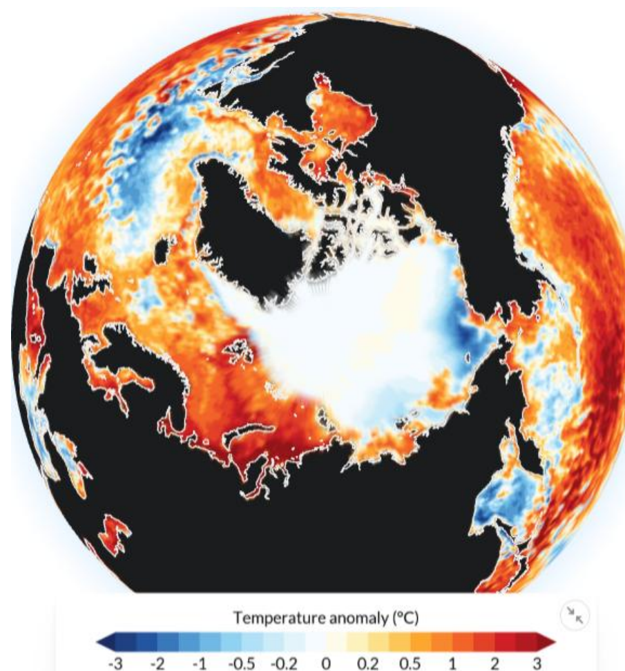
Рисунок 5а – Аномалия приземной температуры воздуха (2м) и температуры поверхности моря на 20.10.2026 г. относительно периода 1991-2020 гг. - The Copernicus Climate Change Service (C3S) , implemented by the European Centre for Medium-Range Weather Forecasts (ECMWF) on behalf of the European Commission is part of the European Union's space programme
