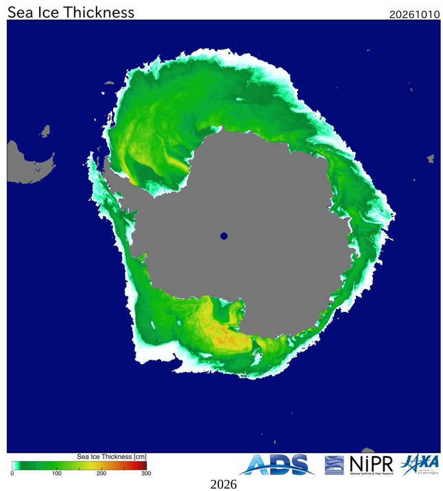
Рисунок 8а - Оценка толщины льда на основе данных пассивного микроволнового зондирования AMSR2 10.10 в 2018 – 2026 гг. [29].
