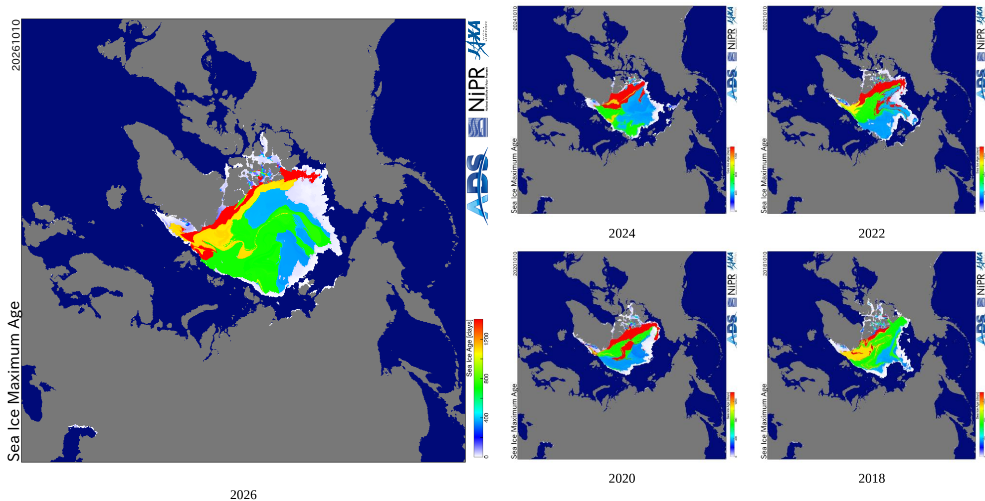
Рисунок 46 – Оценка максимального возраста льда (сутки) на 10.10 за 2018 – 2026 гг. по данным JAXA-NIPR [29]
