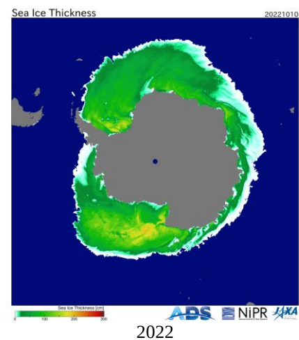
Рисунок 8а - Оценка толщины льда на основе данных пассивного микроволнового зондирования AMSR2 10.10 в 2018 – 2026 гг. [29].
