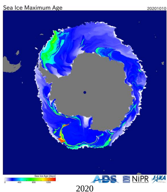
Рисунок 86 – Оценка максимального возраста льда (сутки) на 10.10 за 2018 – 2026 гг. по данным JAXA-NIPR [29]
