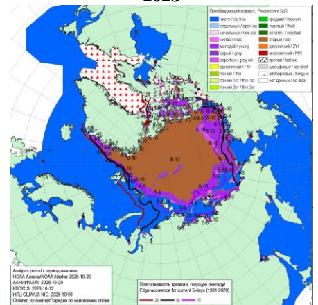
Рисунок 4а – Ледовые условия за 08.10 - 20.10.2026 и аналогичные периоды 2007-2025 гг. на основе ледового анализа ААНИИ, НИЦ Планета, Канадской ледовой службы, Национального ледового центра США и НОАА Аляска [4, 10, 12, 23, 17].
