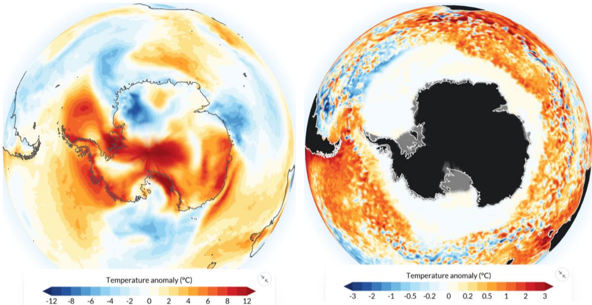
Рисунок 9 – Аномалия приземной температуры воздуха (2м) на 20.10.2026 г. относительно периода 1991-2020 гг. - The Copernicus Climate Change Service (C3S) , implemented by the European Centre for Medium-Range Weather Forecasts (ECMWF) on behalf of the European Commission is part of the European Union's space programme.
