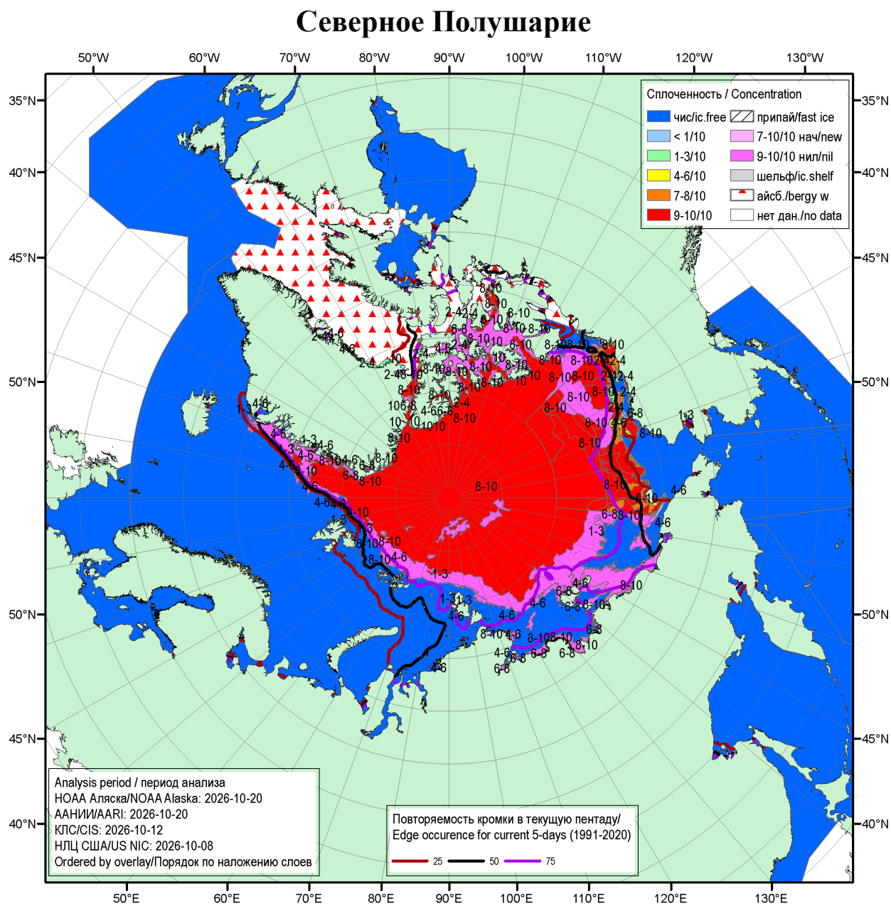
Рисунок 1а – Обзорная ледовая карта СЛО за 08.10.2026 – 20.10.2026 (цветовая раскраска по общей сплоченности) на основе ледового анализа NOAA Аляска, ААНИИ, Канадской ледовой службы и Национального ледового центра США и повторяемость кромки за соответствующий 5-дневный период за 1991-2020 гг. по наблюдениям SSMR-SSM/I-SSMIS (алгоритм NASATEAM) [4, 10, 23, 17].
