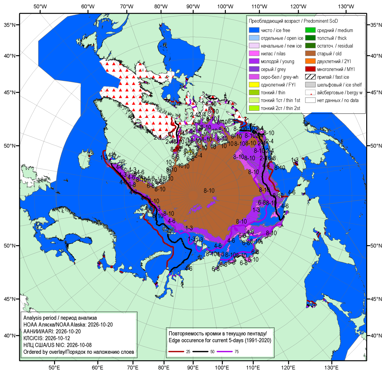
Рисунок 16 – Обзорная ледовая карта СЛО за 08.10.2026 – 20.10.2026 (цветовая раскраска по преобладающему возрасту) на основе ледового анализа НОАА Аляска, ААНИИ, Канадской ледовой службы и Национального ледового центра США и повторяемость кромки за соответствующий 5-дневный период за 1991-2020 гг. по наблюдениям SSMR-SSM/I-SSMIS (алгоритм NASATEAM) [4, 10, 23, 17].
