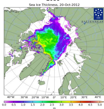
Рисунок 4в – Поля распределения средневзвешенной толщины льда совместной модели морского льда – океана HYCOM/CICE Датского метеорологического института 20.10 за 2005-2026 гг. [22].
