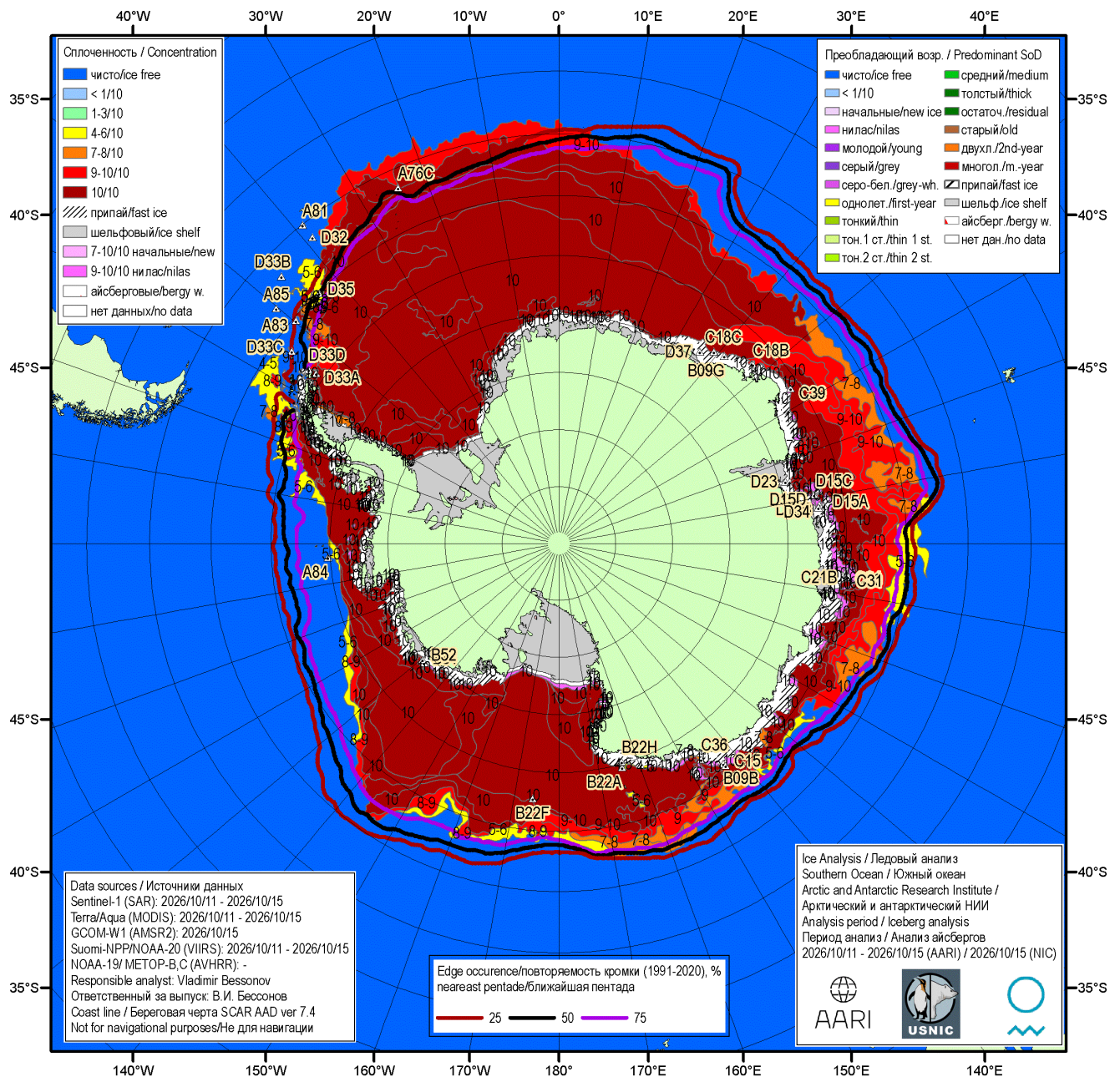
Рисунок 7а – Ледовая карта Южного океана (цветовая окраска по общей сплоченности) и расположение крупных айсбергов на основе ледового анализа за 15.10.2026 в рамках проекта совместного ледового картирования Южного океана ААНИИ, НЛЦ США и НМИ и повторяемость кромки за ближайшую пентаду за период 1991-2020 гг. по наблюдениям SSMR-SSM/I-SSMIS (алгоритм NASATEAM) [5, 10, 17, 21]
