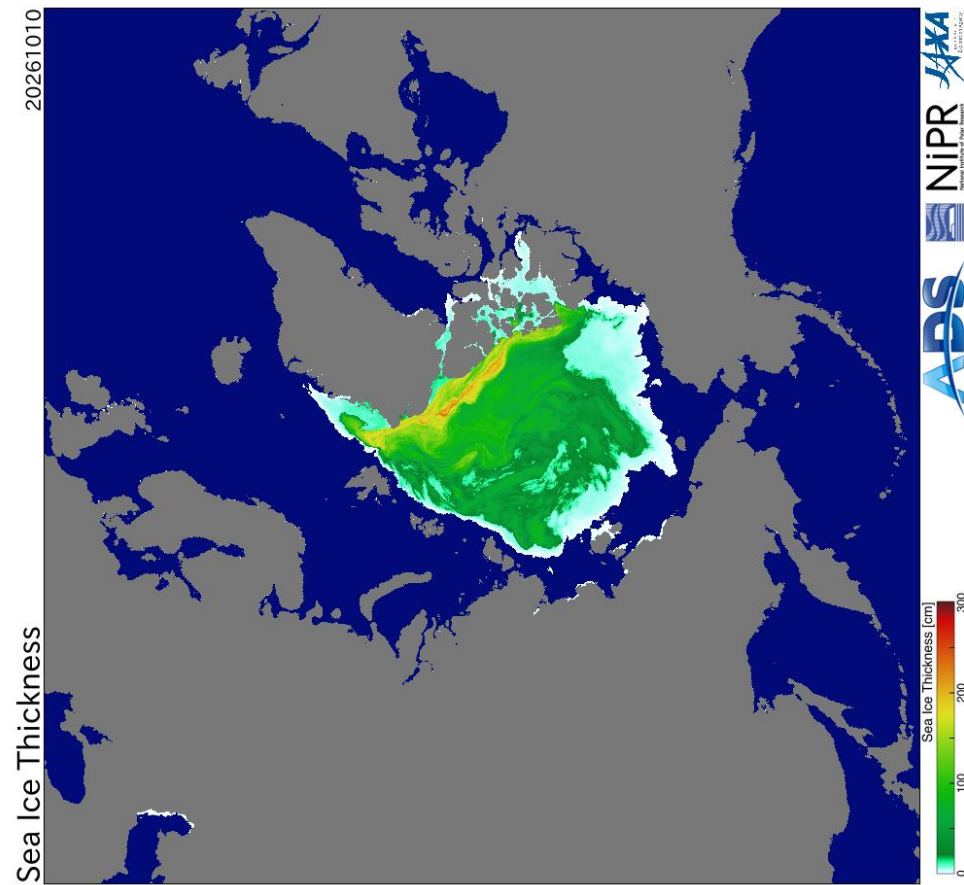
Рисунок 2а - Оценка толщины льда на основе данных пассивного микроволнового зондирования AMSR2 10.10 в 2018 – 2026 гг. [29].
