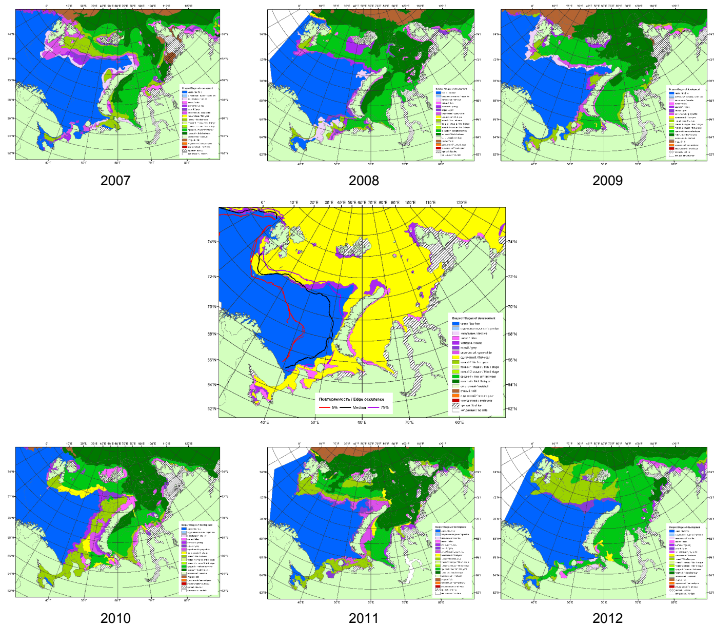
Рисунок 4 – Обзорная ледовая карта акваторий нац. парка «Русская Арктика» за 16.04.2013 г. и аналогичные периоды 2007-2012 гг. на основе ледового анализа ААНИИ и Национального ледового центра США.
