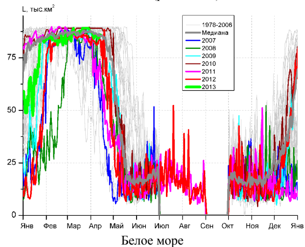
Рисунок 5 – Ежедневные оценки сезонного хода ледовитости для акваторий (рис.7) нац. парка «Русская Арктика» за период 26.10.1978 - 14.04.2013 по годам на основе расчетов по данным SSMR-SSM/I-SSMIS, алгоритм NASATEAM.
