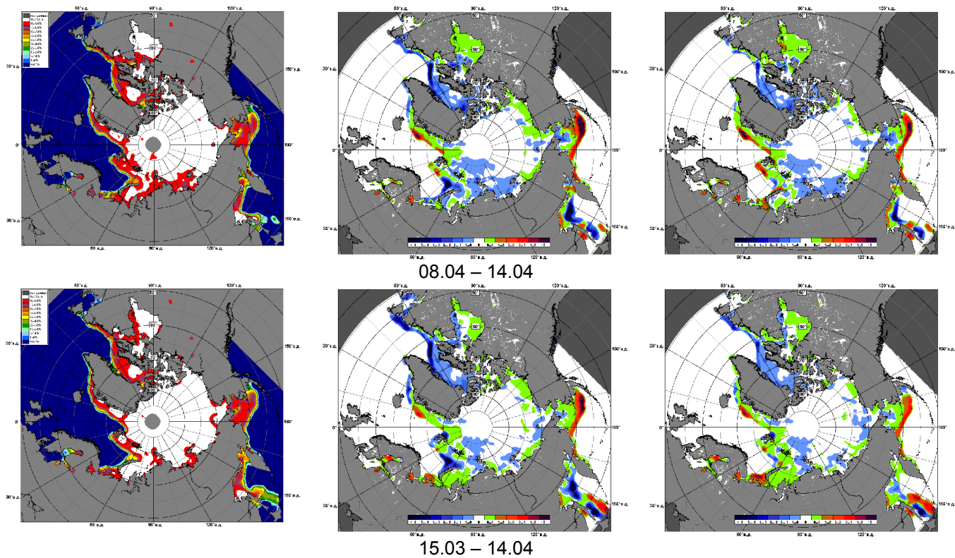
Рисунок 6 – Медианные распределения сплоченности льда за периоды 8 – 14 апреля и 15 марта – 14 апреля 2013 г. (слева) и её разности относительно медианного распределения за те же месяца за периоды 1979-2013 (центр) и 2003-2013 гг. (справа) на основе расчетов по данным SSMR-SSM/I-SSMIS, алгоритм NASATEAM.
