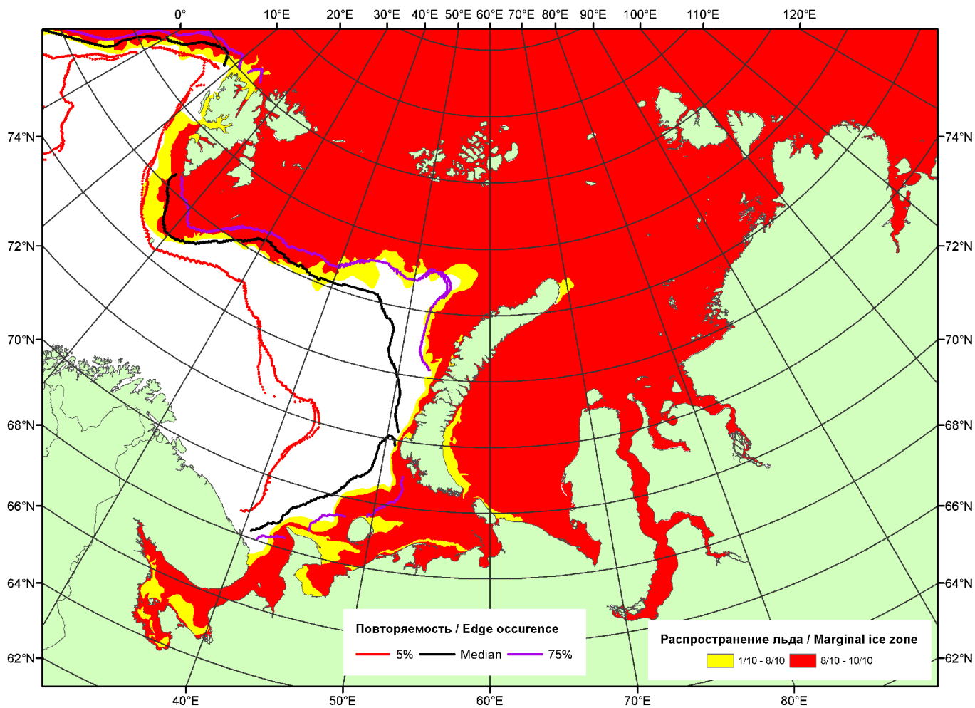
Рисунок 2 – Положение кромки льда (районов безледокольного плавания) и сплоченных льдов акваторий нац. парка «Русская Арктика» за 15.04.2013 г. на основе ледового анализа Национального Ледового Центра США и повторяемость кромки за 11.04-15.04 за период 1979-2012 гг. по наблюдениям SSMR-SSM/I-SSMIS (алгоритм NASATEAM)
