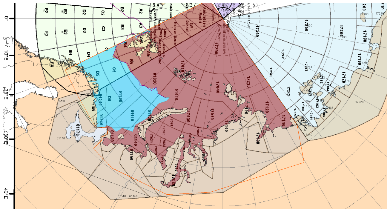
Рисунок 3 – Положение кромки льда (районов безледокольного плавания) в МЕТЗОНах XX-XXI на 16.04.2013 1200UTC
