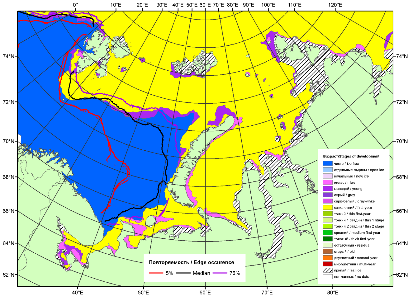
Рисунок 1 – Обзорная ледовая карта акваторий нац. парка «Русская Арктика» за 16.04.2013 г. на основе ледового анализа ААНИИ (16.04.2013) и повторяемость кромки за 16-20.04 за период 1979-2012 гг. по наблюдениям SSMR-SSM/I-SSMIS (алгоритм NASATEAM).
