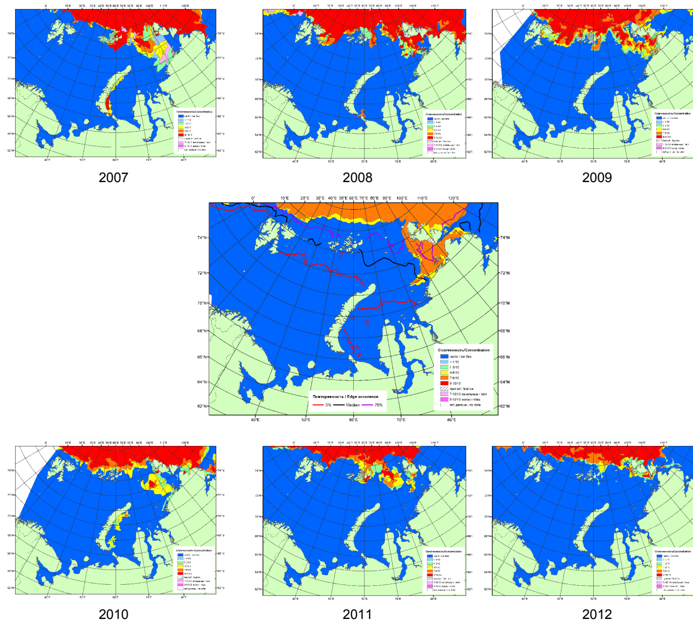
Рисунок 4 – Обзорная ледовая карта акваторий нац. парка «Русская Арктика» за 13.08.2013 г. и аналогичные периоды 2007-2012 гг. на основе ледового анализа ААНИИ и Национального ледового центра США.
