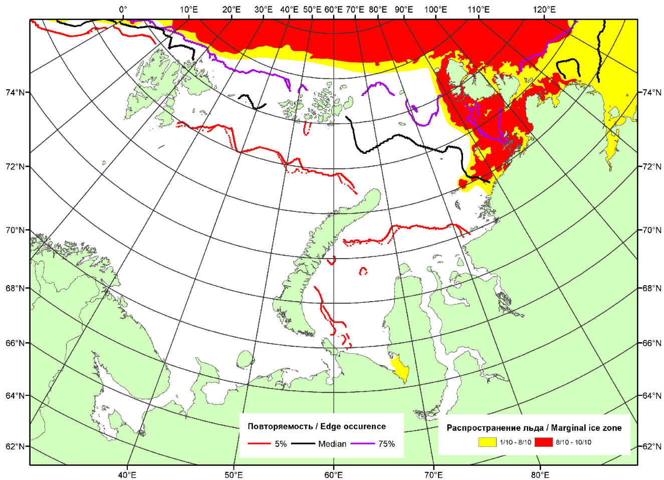
Рисунок 2 – Положение кромки льда (районов безледокольного плавания) и сплоченных льдов акваторий нац. парка «Русская Арктика» за 12.08.2013 г. на основе ледового анализа Национального Ледового Центра США и повторяемость кромки за 11.08-15.08 за период 1979-2012 гг. по наблюдениям SSMR-SSM/I-SSMIS (алгоритм NASATEAM)
