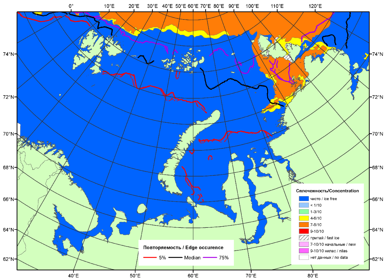
Рисунок 1 – Обзорная ледовая карта акваторий нац. парка «Русская Арктика» за 13.08.2013 г. на основе ледового анализа ААНИИ (13.08.2013) и повторяемость кромки за 11-15.08 за период 1979-2012 гг. по наблюдениям SSMR-SSM/I-SSMIS (алгоритм NASATEAM).
