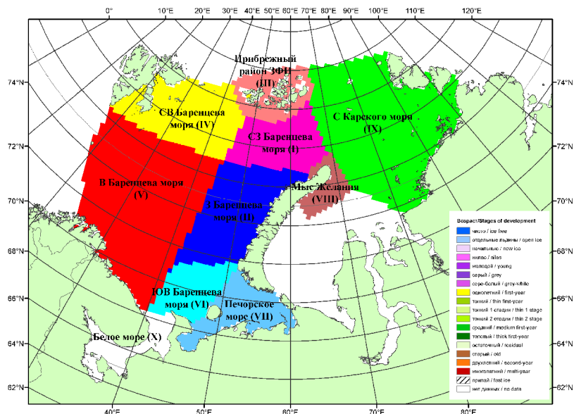
Рисунок 7 – Принятое районирование (акватории) национального парка «Русская Арктика» для расчета ледовитостей
