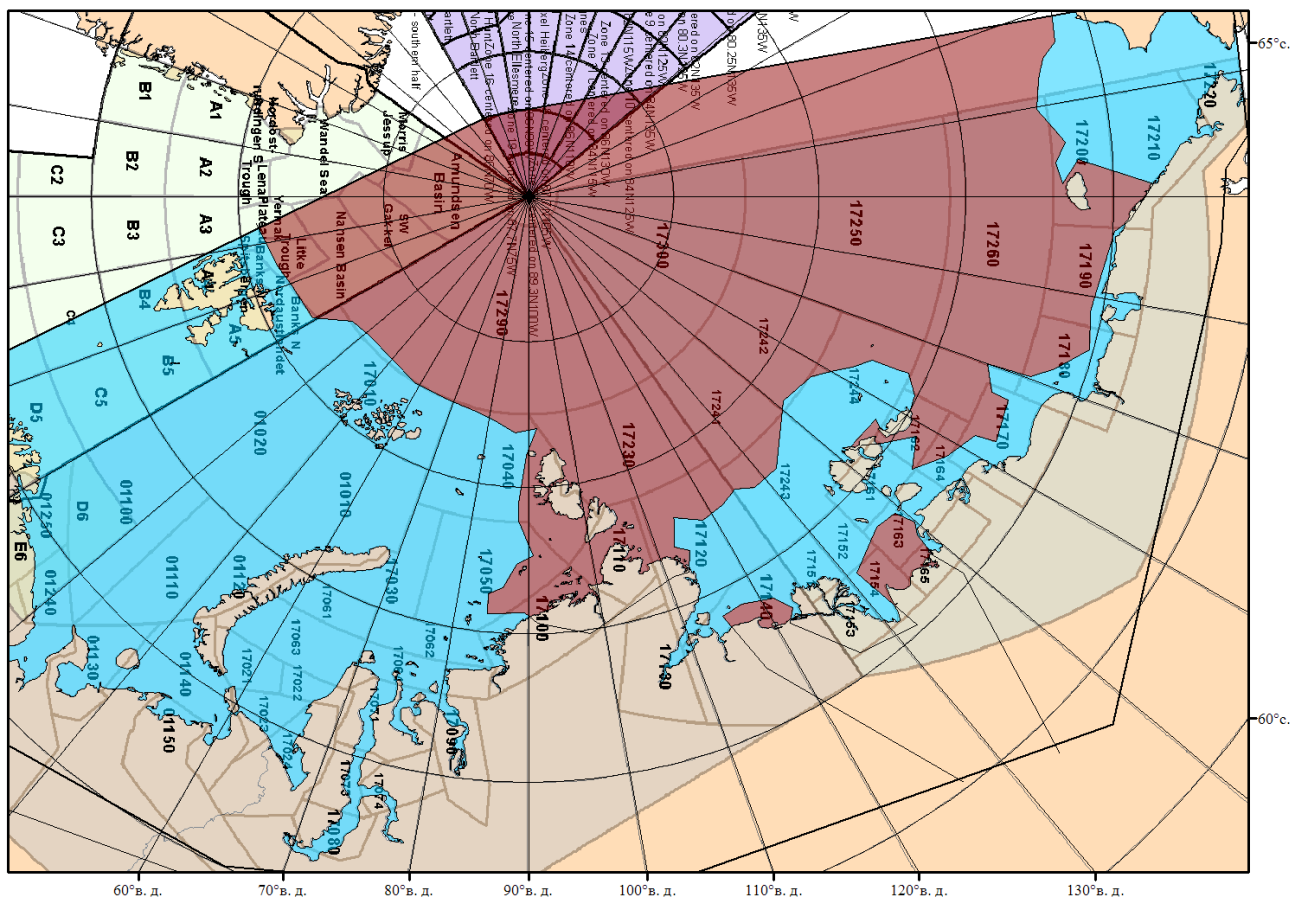
Рисунок 3 – Положение кромки льда (районов безледокольного плавания) в МЕТЗОНах XX-XXI на 13.08.2013 1200UTC
