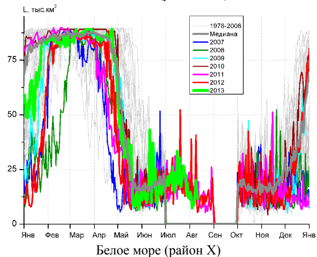
Рисунок 5 – Ежедневные оценки сезонного хода ледовитости для акваторий (рис.7) нац. парка «Русская Арктика» за период 26.10.1978 - 11.08.2013 по годам на основе расчетов по данным SSMR-SSM/I-SSMIS, алгоритм NASATEAM.
