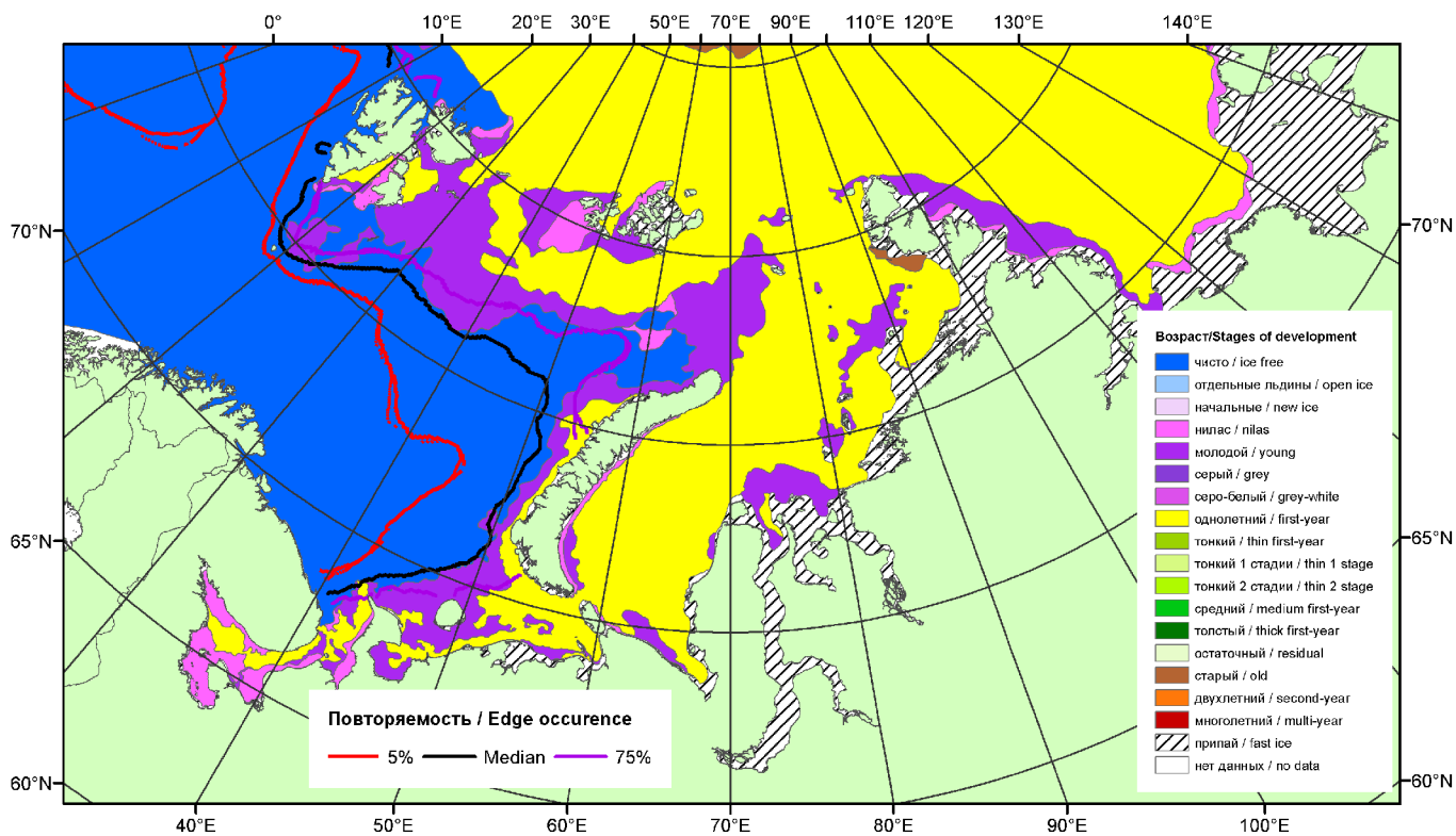
Рисунок 1 – Обзорная ледовая карта акваторий нац. парка «Русская Арктика» и заповедных территорий Таймыра за 18.03.2014 г. на основе ледового анализа ААНИИ (18.03.2014) и повторяемость кромки за 16-20.03 за период 1979-2012 гг. по наблюдениям SSMR-SSM/I-SSMIS (алгоритм NASATEAM).
