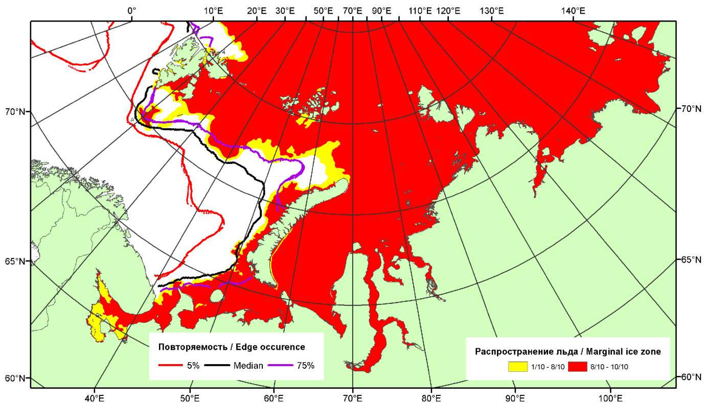
Рисунок 2 – Положение кромки льда (районов безледокольного плавания) и сплоченных льдов акваторий нац. парка «Русская Арктика» и заповедных территорий Таймыра за 17.03.2014 г. на основе ледового анализа Национального Ледового Центра США и повторяемость кромки за 16-20.03 за период 1979-2012 гг. по наблюдениям SSMR-SSM/I-SSMIS (алгоритм NASATEAM)
