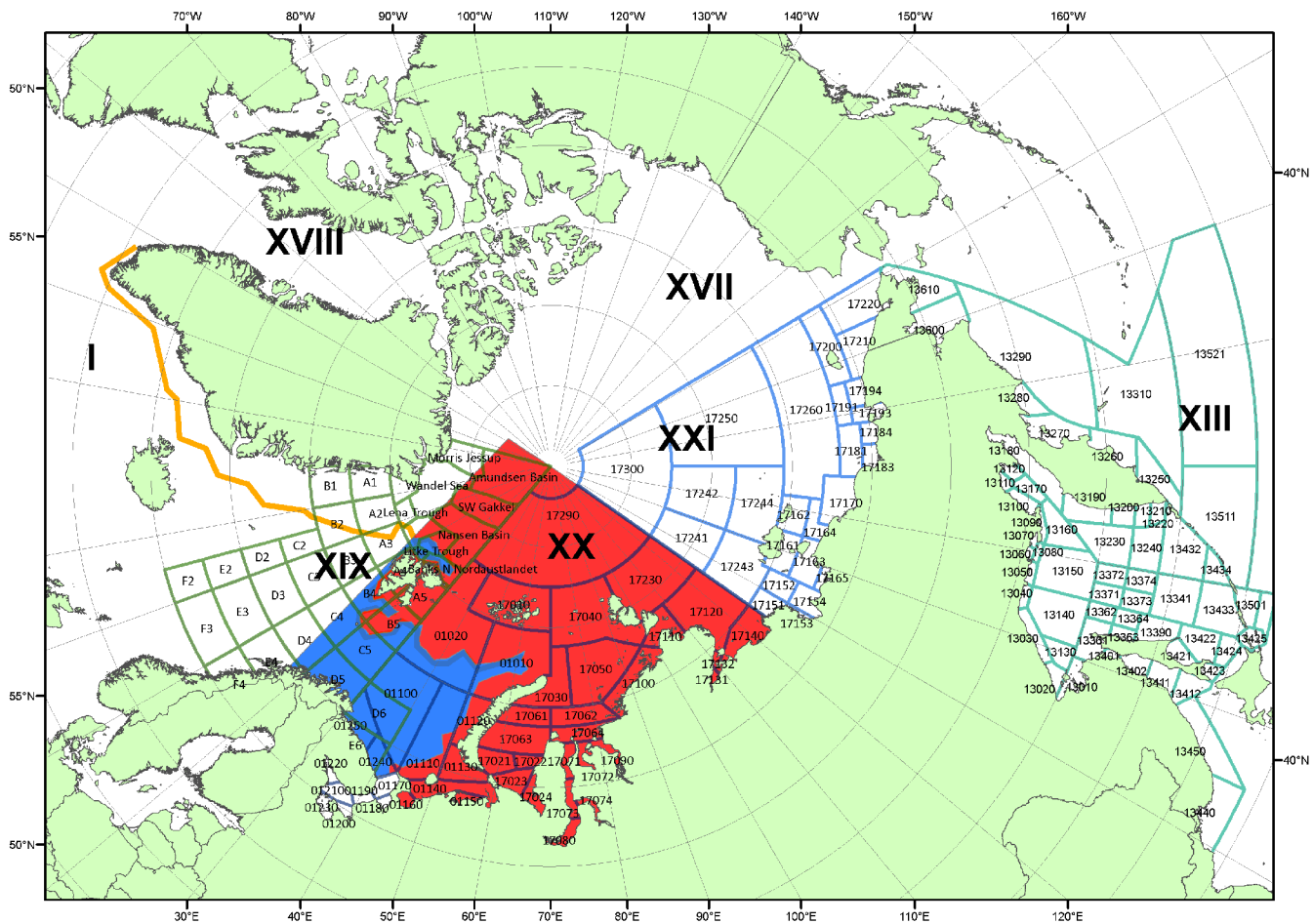
Рисунок 3 – Положение кромки льда (районов безледокольного плавания) в МЕТЗОНах XX-XXI на 18.03.2014 1200UTC и МЕТЗОНах I- XIX на 17.03.2014 2300UTC
