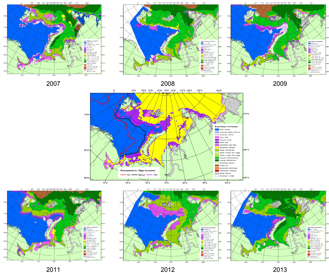
Рисунок 4 – Обзорная ледовая карта акваторий нац. парка «Русская Арктика» и заповедных территорий Таймыра за 18.03.2014 г. и аналогичные периоды 2007-2013 гг. на основе ледового анализа ААНИИ и Национального ледового центра США.
