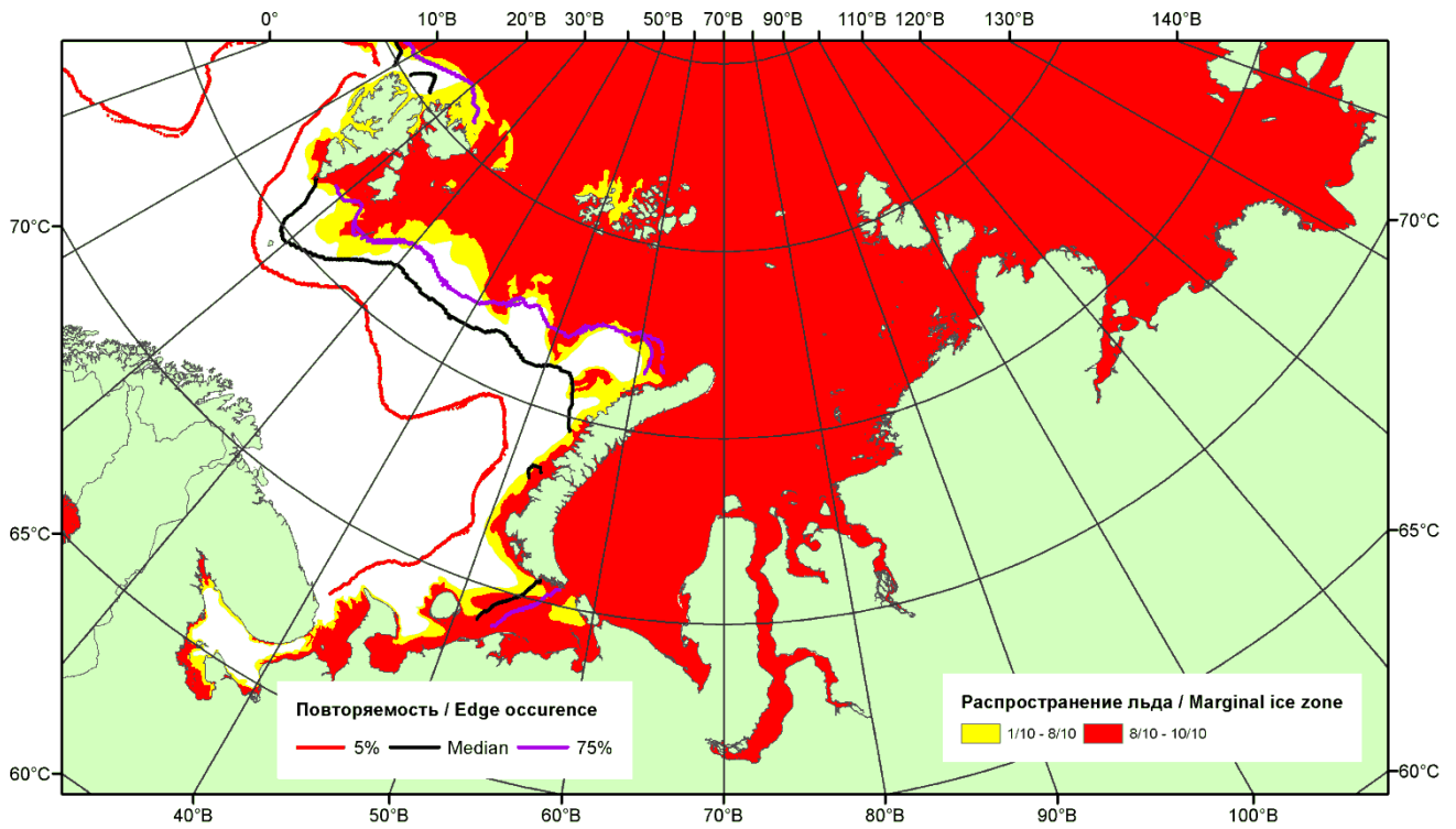
Рисунок 2 – Положение кромки льда (районов безледокольного плавания) и сплошных льдов акваторий нац. парка «Русская Арктика» и заповедных территорий Таймыра за 05.01.2015 г. на основе ледового анализа Национального Ледового Центра США и повторяемость кромки за 01-05.01 за период 1979-2012 гг. по наблюдениям SSMR-SSM/I-SSMIS (алгоритм NASATEAM)
