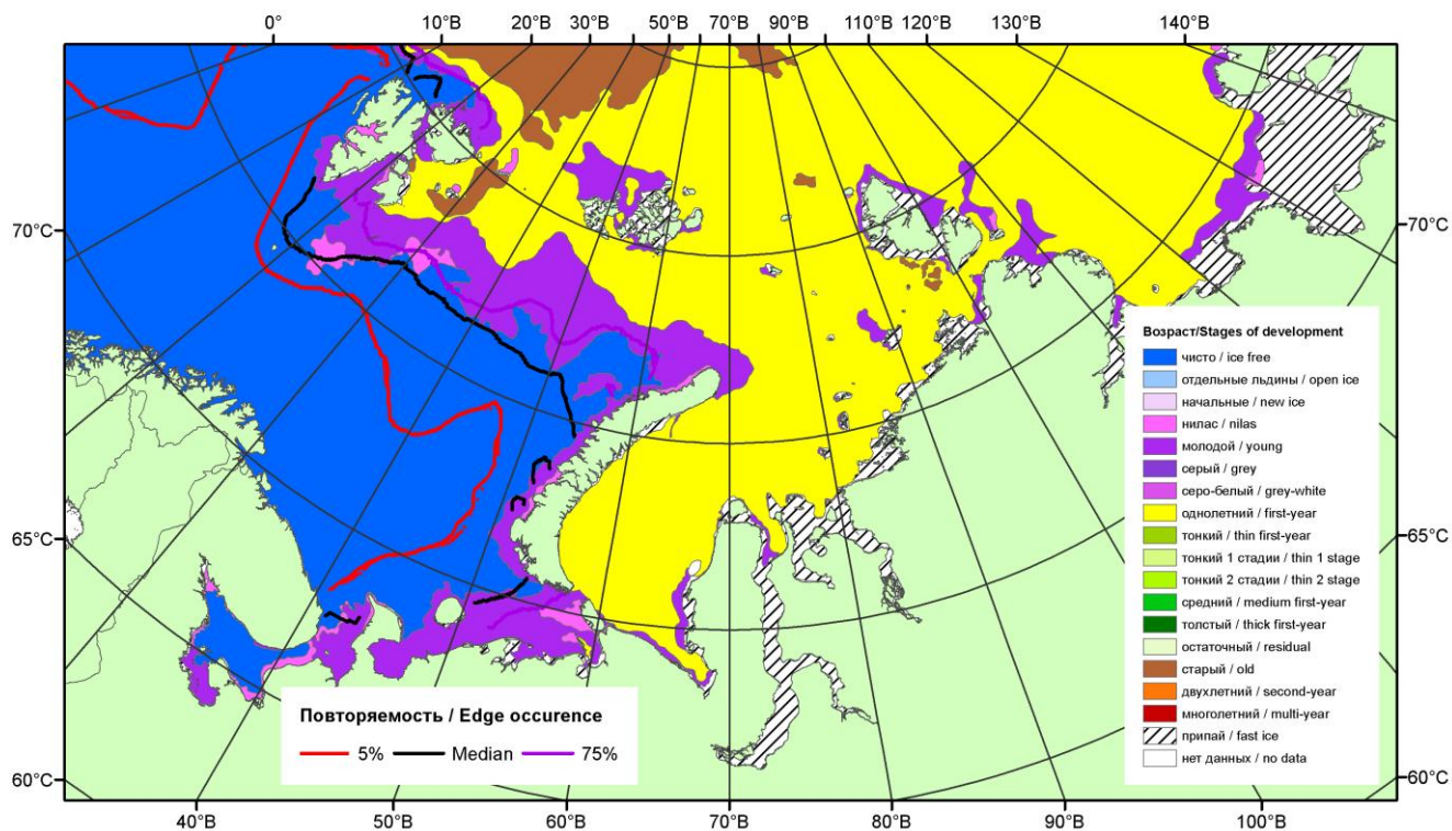
Рисунок 1 – Обзорная ледовая карта акваторий нац. парка «Русская Арктика» и заповедных территорий Таймыра за 06.01.2015 г. на основе ледового анализа ААНИИ (06.01.2015) и повторяемость кромки за 06-10.01 за период 1979-2012 гг. по наблюдениям SSMR-SSM/I-SSMIS (алгоритм NASATEAM).
