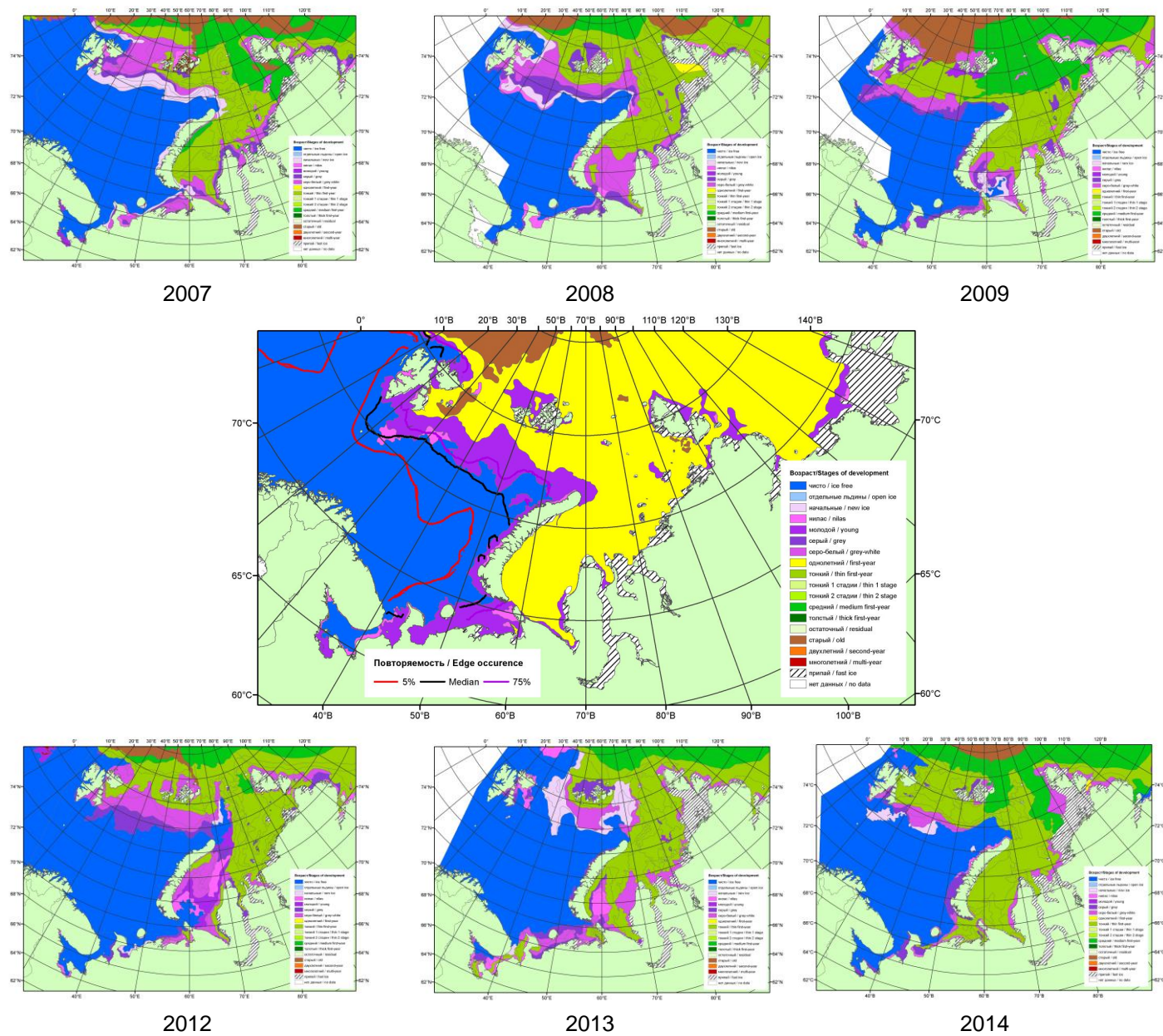
Рисунок 3 – Обзорная ледовая карта акваторий нац. парка «Русская Арктика» и заповедных территорий Таймыра за 05.01.2015 г. и аналогичные периоды 2007-2014 гг. на основе ледового анализа ААНИИ и Национального ледового центра США.
