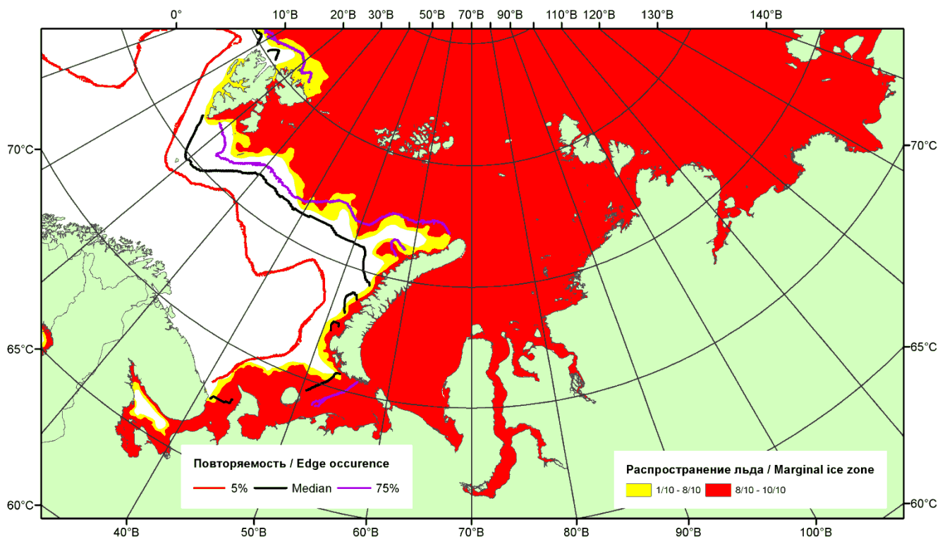
Рисунок 2 – Положение кромки льда (районов безледокольного плавания) и сплоченных льдов акваторий нац. парка «Русская Арктика» и заповедных территорий Таймыра за 12.01.2015 г. на основе ледового анализа Национального Ледового Центра США и повторяемость кромки за 11-15.01 за период 1979-2012 гг. по наблюдениям SSMR-SSM/I-SSMIS (алгоритм NASATEAM)
