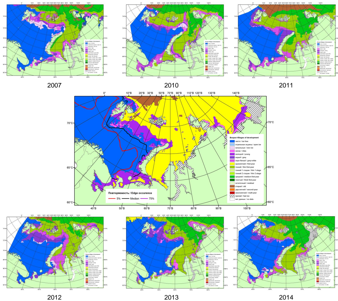
Рисунок 3 – Обзорная ледовая карта акваторий нац. парка «Русская Арктика» и заповедных территорий Таймыра за 13.01.2015 г. и аналогичные периоды 2007-2014 гг. на основе ледового анализа ААНИИ и Национального ледового центра США.
