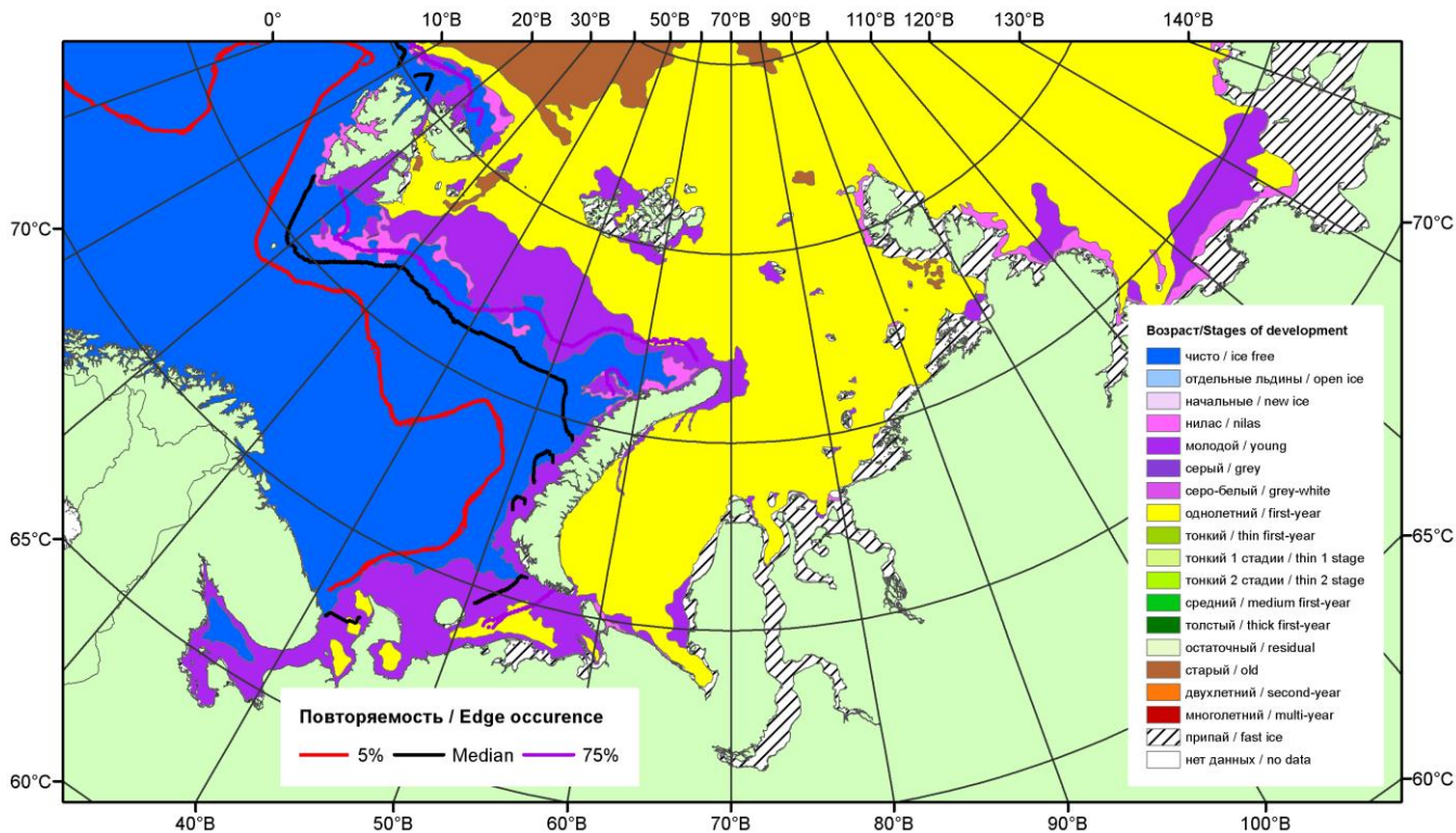
Рисунок 1 – Обзорная ледовая карта акваторий нац. парка «Русская Арктика» и заповедных территорий Таймыра за 13.01.2015 г. на основе ледового анализа ААНИИ (13.01.2015) и повторяемость кромки за 11-15.01 за период 1979-2012 гг. по наблюдениям SSMR-SSM/I-SSMIS (алгоритм NASATEAM).
