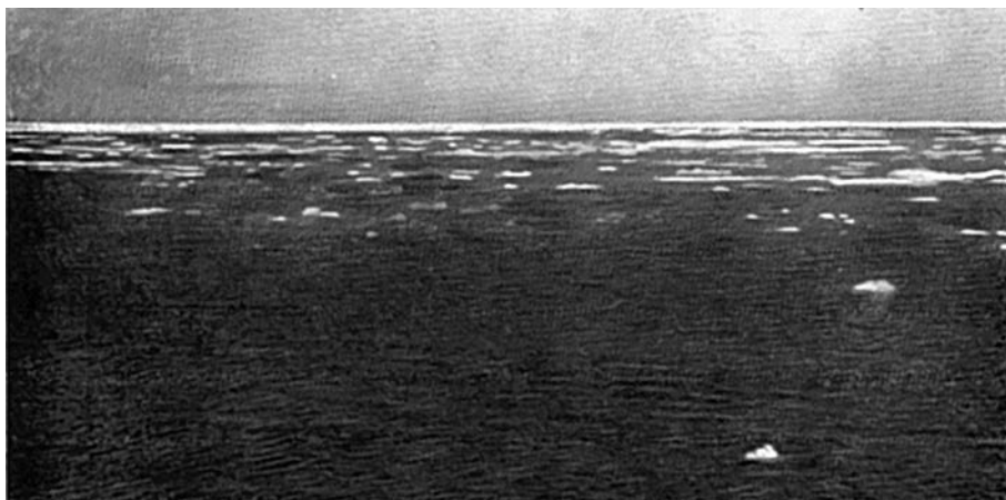
4.4.8.2а. Разреженная кромка льда.
