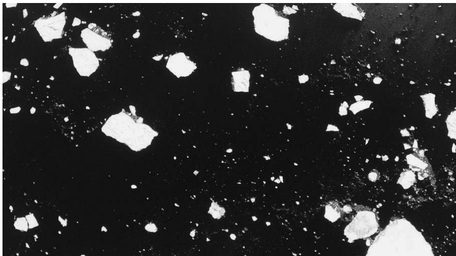
4.2.6б. Отдельные льдины. Апрель. Охотское море.
