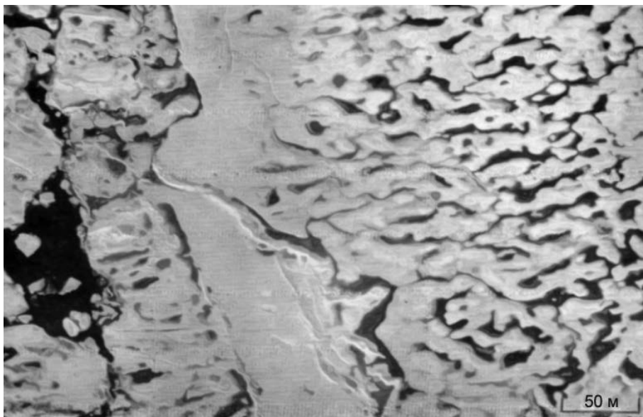
2.5.3в. Толстый однолетний лед летом. Август. Северная часть Восточно-Сибирского моря.
