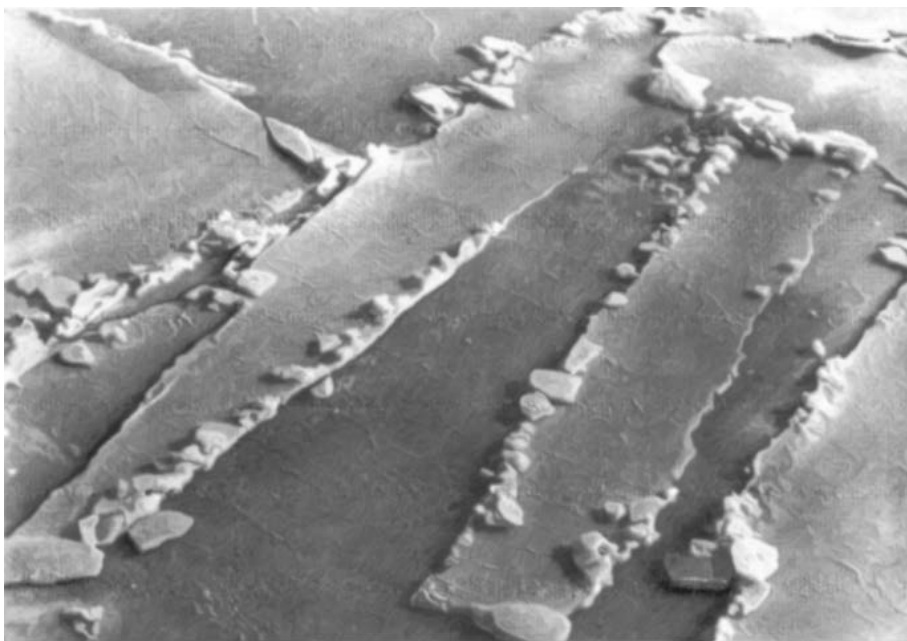
2.2.1б. Темный нилас, образовавший при сжатии зубчатонаслоенного льда. Март, Белое море.
