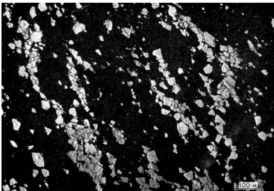
4.2.5а. Редкий лед, крупнобитый и мелкобитый однолетний толстый лед, сбиваемый под воздействием ветра и волнения в полосы. Апрель. Район к западу от Шпицбергена.
