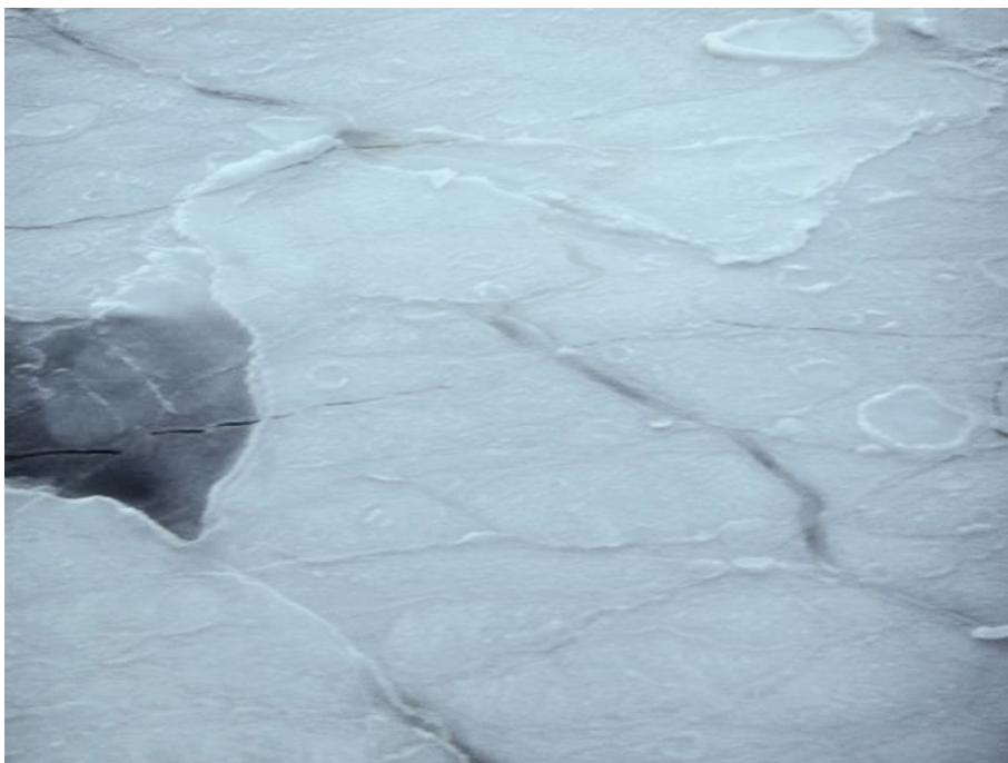
2.2.1д. Темный нилас, образовавшийся из блинчатого льда. Март 2006 г. Район моря Содружества, Антарктика.
