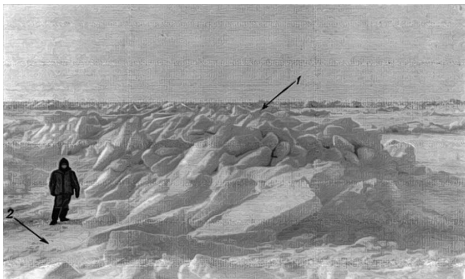
8.2.2.1б. Мощная гряда торосов, образовавшаяся в результате выторашивания белого льда в разводе между многолетними полями. 1 — гребень гряды, 2 — подошва гряды.
