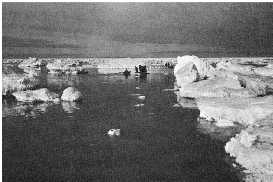
3.4. Лед севший на мель.
