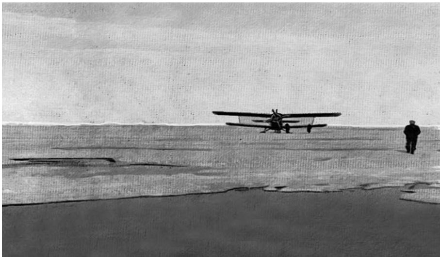
9.36. Обсохший толстый однолетний лед. Сохранившиеся озёрца из-за меньшей отражательной способности воды по сравнению с обнажившимся льдом интенсивно углубляются.
