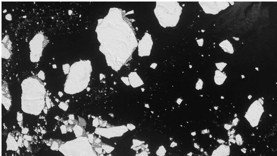
4.2.5б. Редкий лед. Однолетний тонкий. Охотское море.
