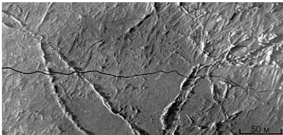
7.1.1а. Трещина, прошедшая по полю однолетнего толстого льда. Апрель. Арктический бассейн.
