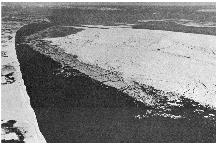
4.4.1б. Скопление дрейфующего льда.
