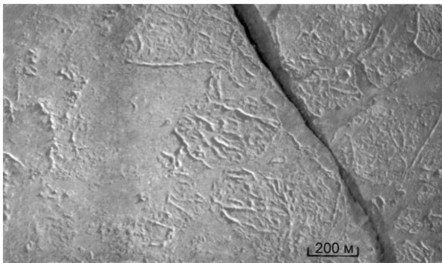
4.3.5a. Сморози обломков полей и крупнобитого многолетнего и остаточного однолетнего льда, в развоях между которыми образовался серо-белый лед.
