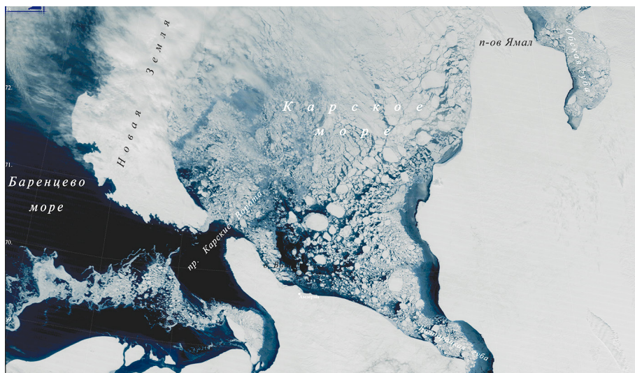
12.7. Относительно легкий район.
