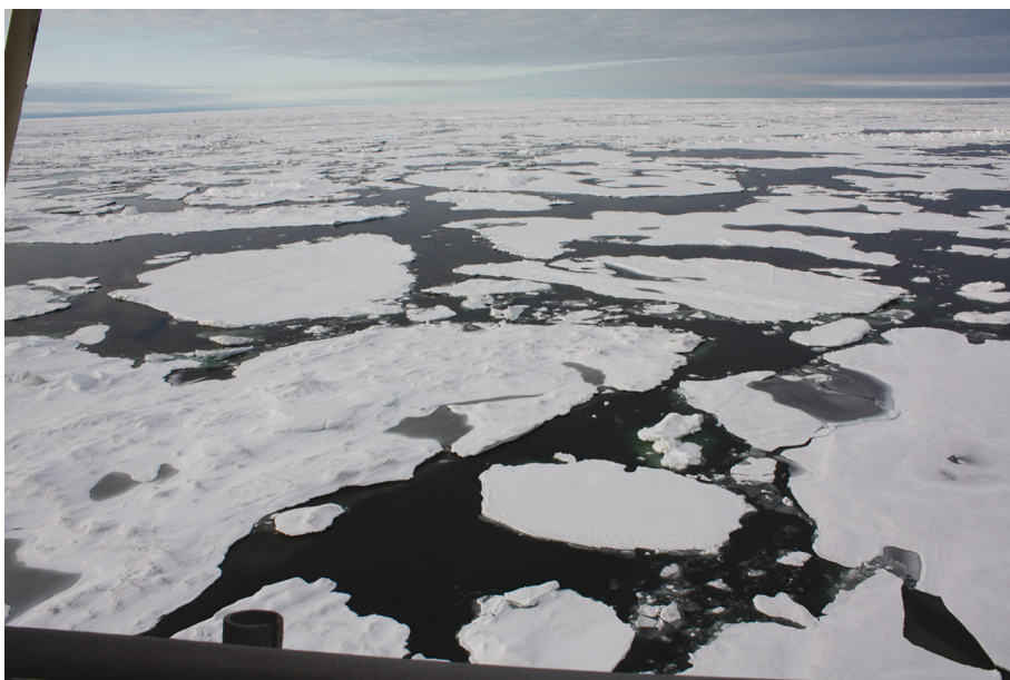
1.1а. Морской лед. Август. Море Лаптевых.
