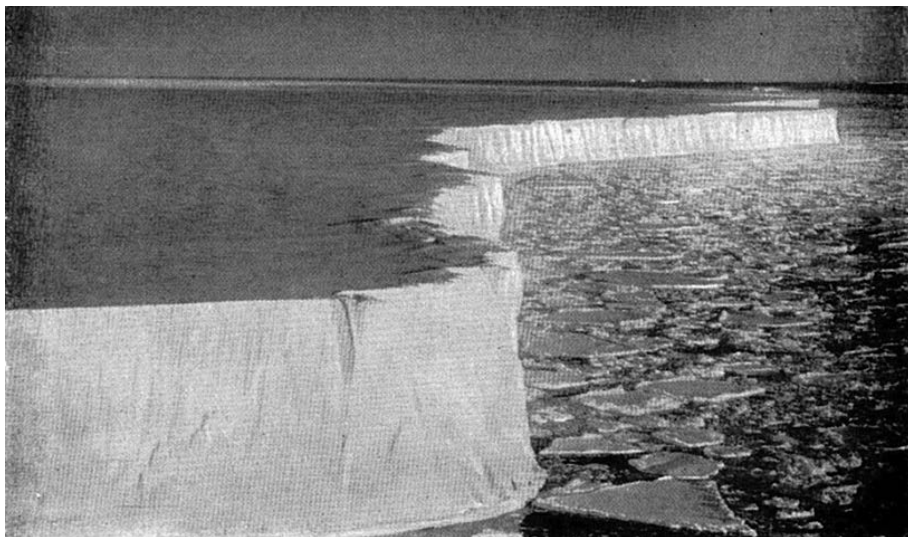
10.3.1а. Ледяной барьер. Февраль. Моря Антарктики.
