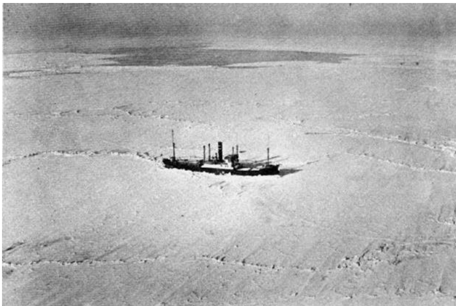
12.1а. Судно, затертое льдами. Март. Ботнический залив.
