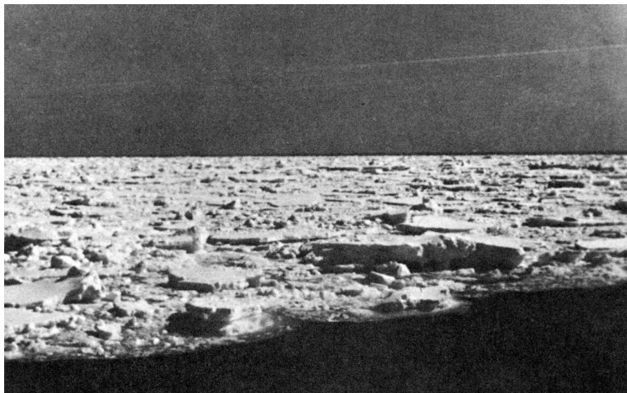
4.4.8.1б. Сплощенная кромка льда.
