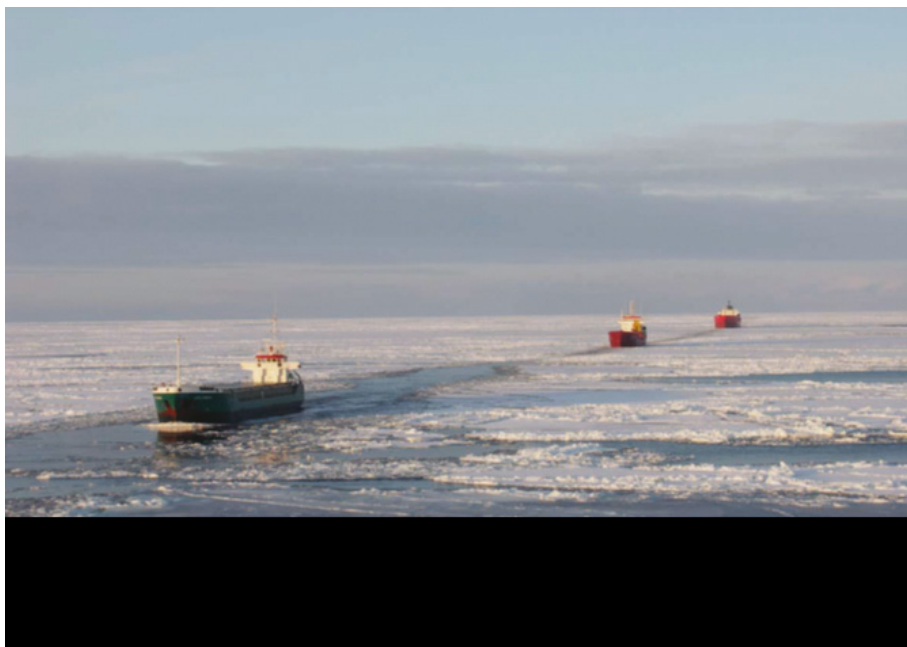
2.4.2г. Канал, проложенный караваном в серо-белом льду. На переднем плане нилас. Март. Белое море.
