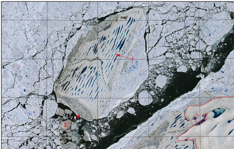
10.4.3д. Ледяной остров.
