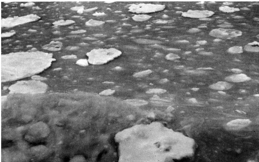
2.1.3в. Снежура. Декабрь. Балтийское море.
