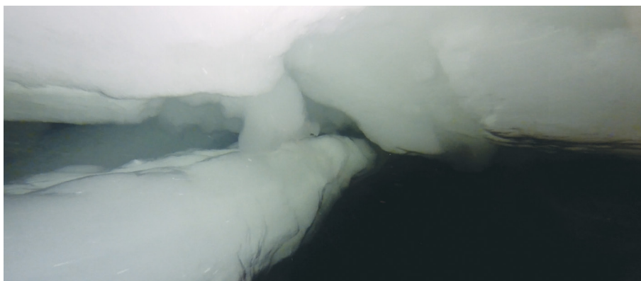
13.4а. Подторос. Карское море.
