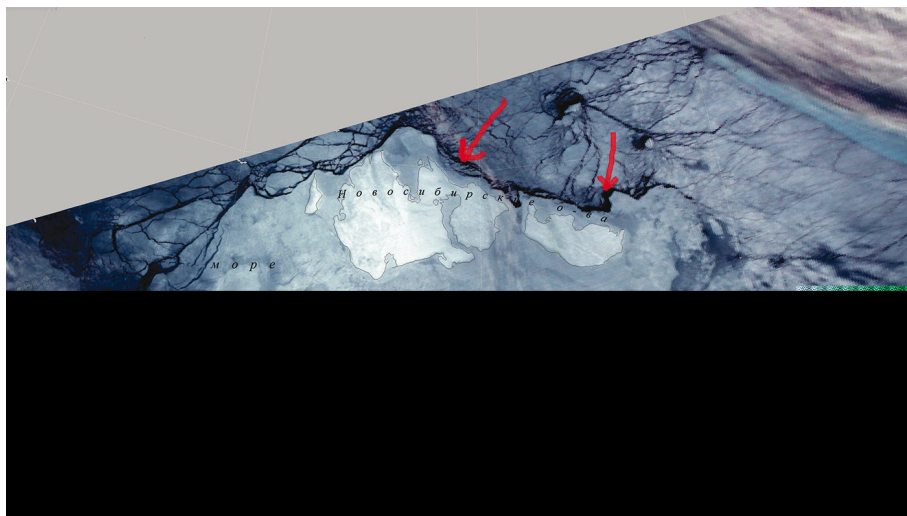
7.4.3а. Стационарная полынья. Февраль. Великая Сибирская полынья.
