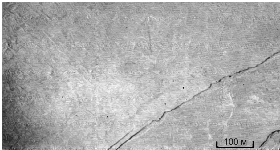
8.1a. Ровный лед, толстый однолетний.
