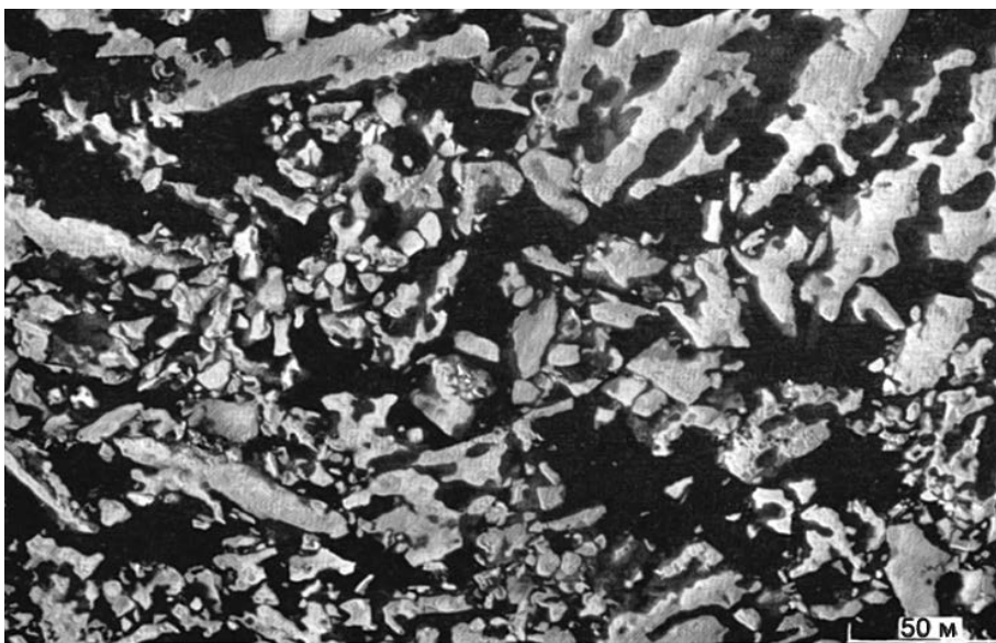
9.4а. Гнилой лед. Август. Восточно-Сибирское море.
