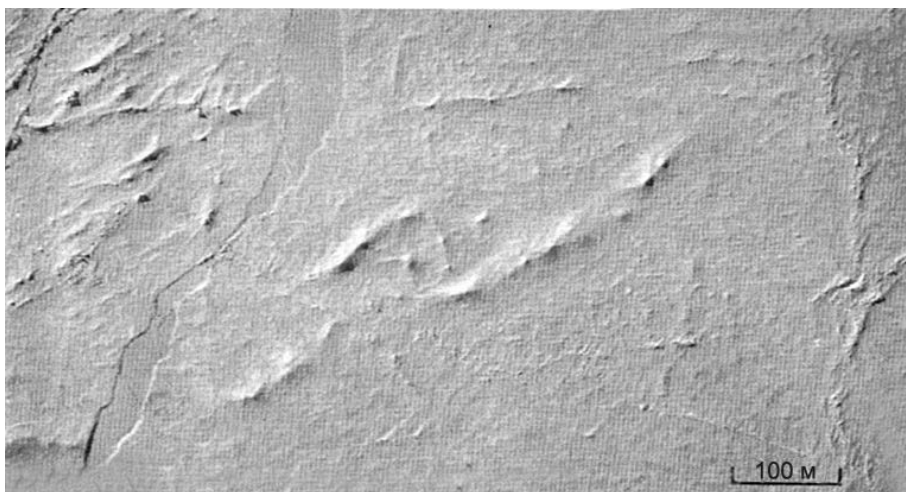
8.2.2.4. Умеренно всхолмленный многолетний лед. В центре снимка ледяной холм (бугор) и старая монолитная гряда. Апрель. Арктический бассейн.
