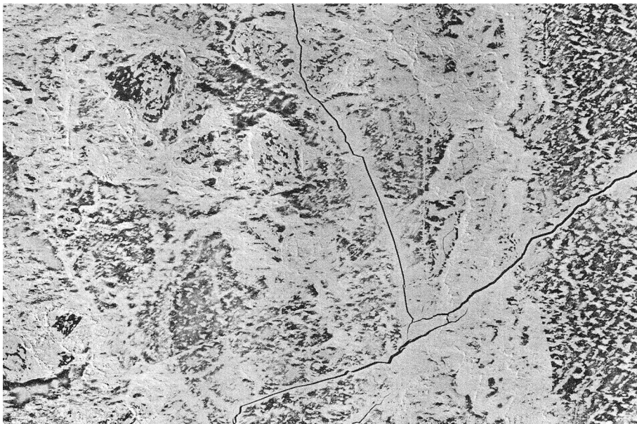
7.1.1д. Трещина. Арктический бассейн.
