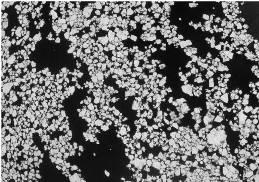
4.3.2.6а. Мелкобитый лед. Апрель. Охотское море.
