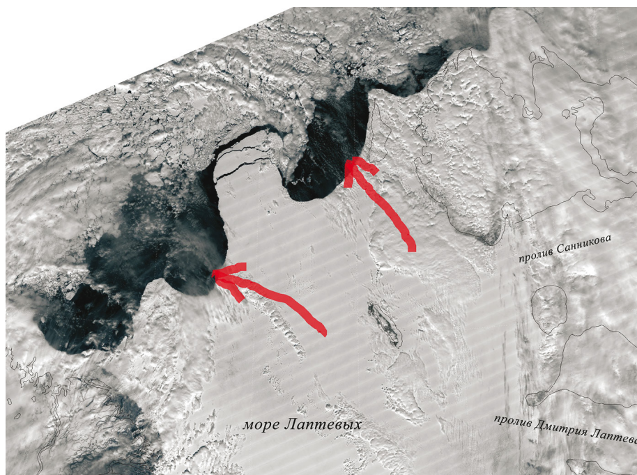
7.4.2а. Заприпайная полынья. Снимок ИСЗ АQUA(MODIS). Май. Море Лаптевых.
