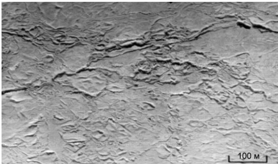
4.2.1.1b. Смерзшийся лед. Однолетний лед средней толщины. Апрель, Карское море.
