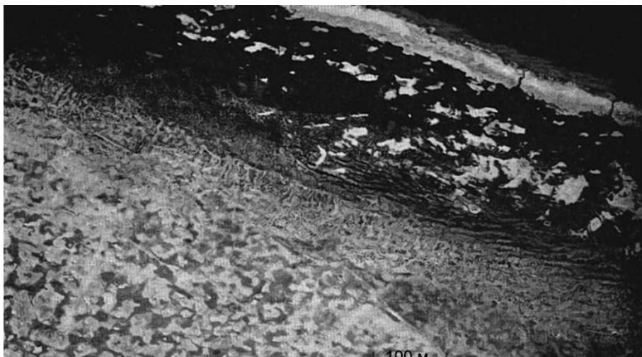
9.6. Закраина. В правом верхнем углу яркой белой полосой выделяется сменяющаяся с грунтом подошва припая. Однолетний лед припая обсох, но сильно пропитан водой и имеет темно-серый цвет. Июль. Восточно-Сибирское море.
