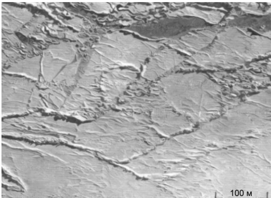
2.5.3а. Толстый однолетний лед толщиной 210—240 см. Апрель. Приполюсный район.
