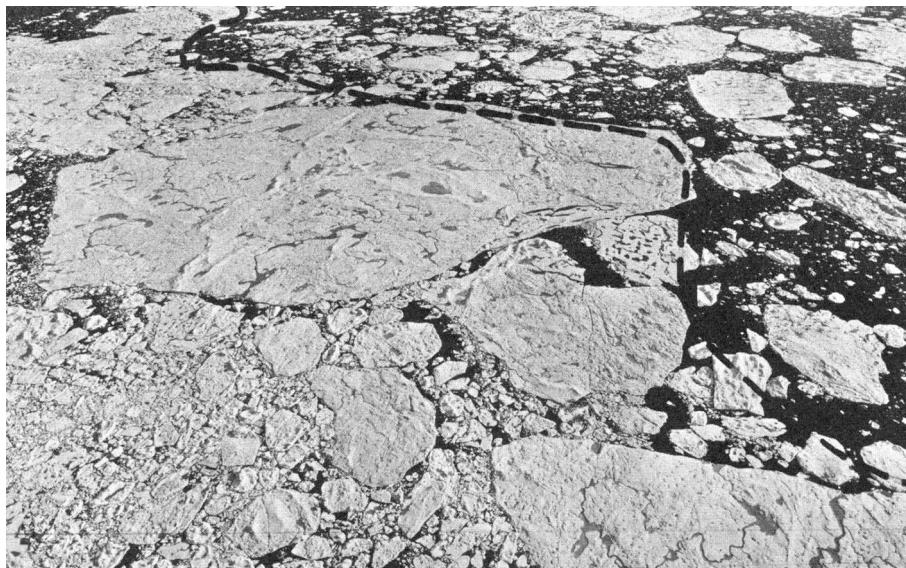
4.4.9.2. Граница между льдами различной сплоченности.
