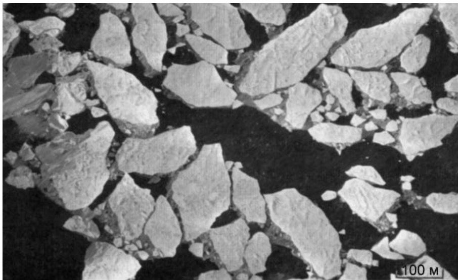
4.2.4а. Разреженный лед, обломки полей, крупнобитый и тертый лед. Апрель. Район западнее Шпицбергена.
