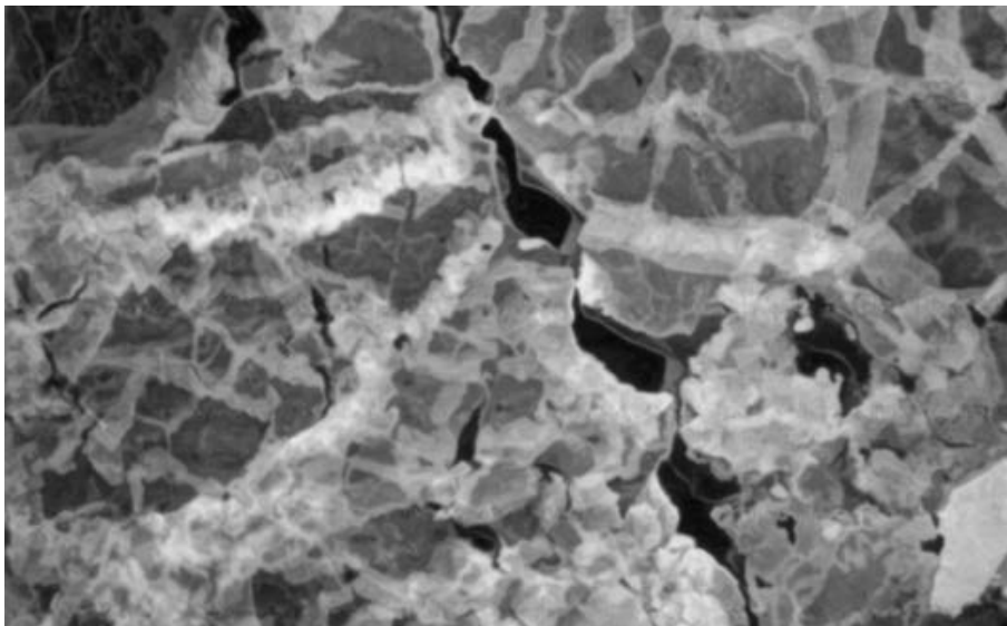
2.2.2б. Светлый нилас в прикромочной зоне. Наслоенность льда 7 баллов.
