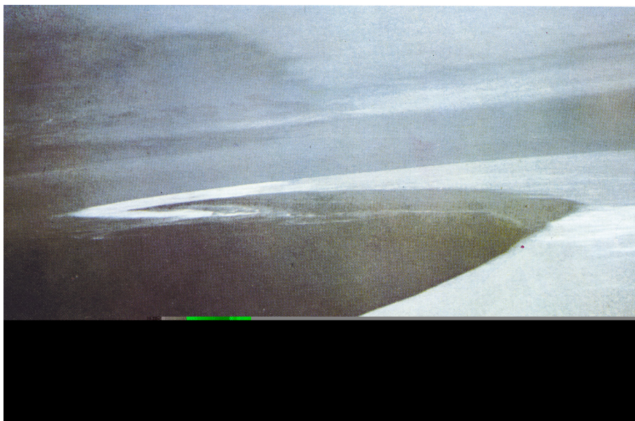
4.4.4б. Язык льда.
