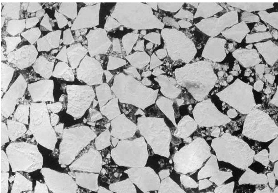
4.3.2.5в. Крупнобитый и мелкобитый тонкий однолетний лед. Апрель. Охотское море.
