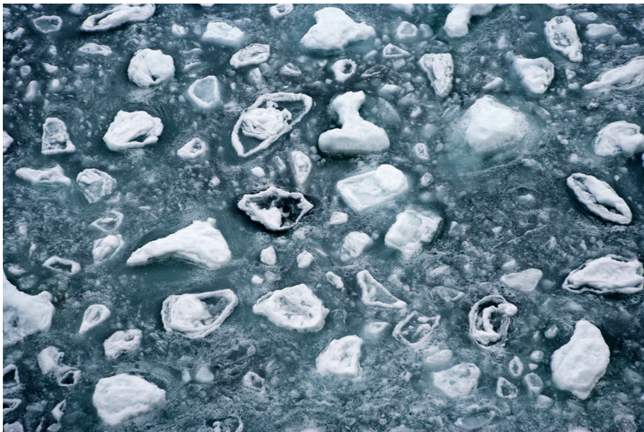
2.1.4б. Шуга и мелкобитый лед. Сентябрь. Восточно-Сибирское море.
