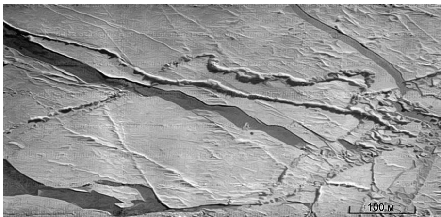
8.2.2.1а. Свежая гряда торосов, образовавшаяся на однолетнем толстом, слабо заснеженном льду. В результате притапливания льда около гряды образовалась наледь.
