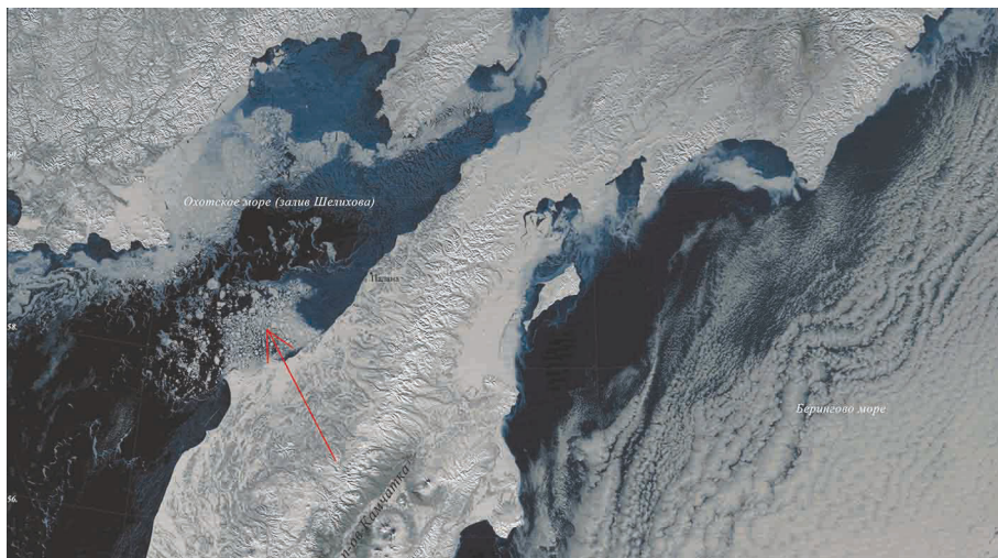
4.4.1а. Скопление дрейфующего льда. Март. Залив Шелихова.
