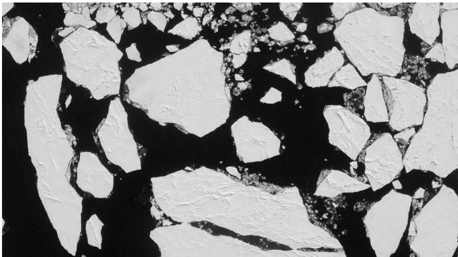
4.2.4б. Разреженный однолетний лед. Апрель. Охотское море.
