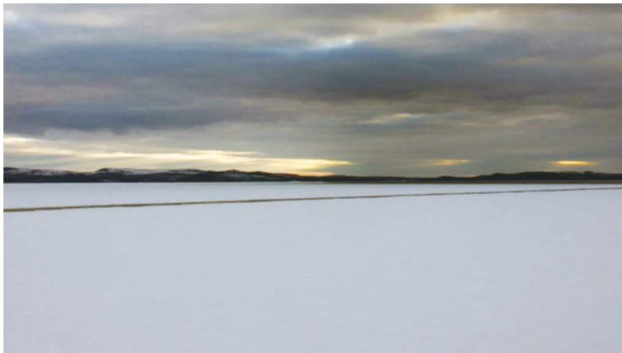
8.1в. Ровный однолетний тонкий лед, припай разрушенностью 1 балл. В середине снимка канал. Апрель. Кандалакшский залив.
