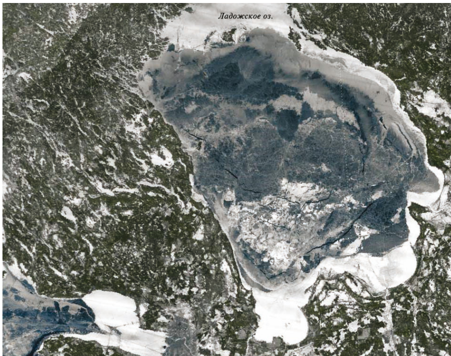
1.3в. Озерный лед. Февраль. Ладожское озеро. Снимок ИСЗ TERRA(MODIS), 26 февраля 2007 г.
