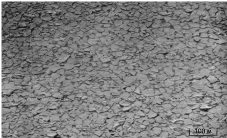
4.2.2а. Очень сплоченный дрейфующий лед (однолетний толстый, крупнобитый, мелкобитый). Апрель. Район западнее Шпицбергена.
