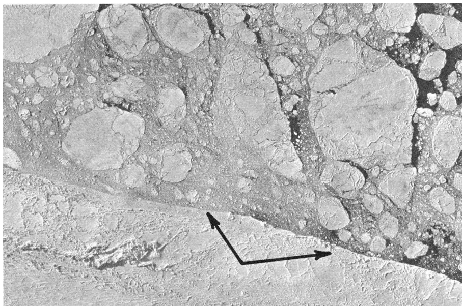
4.4.9.1а. Граница припая.
