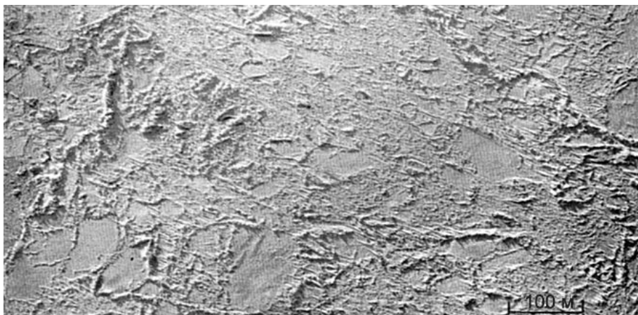
8.2.3а. Торосистый однолетний лед средней толщины.
