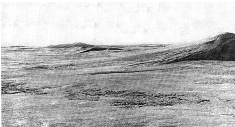
8.2.2.3б. Сильно сглаженная гряда. Август. Северная часть Восточно-Сибирского моря.
