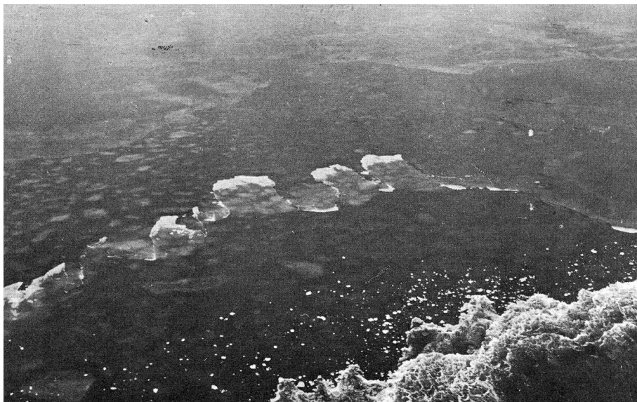
8.2.1.2б. Зубчатонаслоенный лед.
