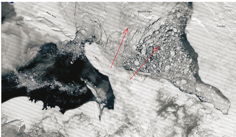
4.4.9. Ледовая граница между сплошным дрейфующим и сплоченным льдом. Май. Юго-запад Карского моря.
