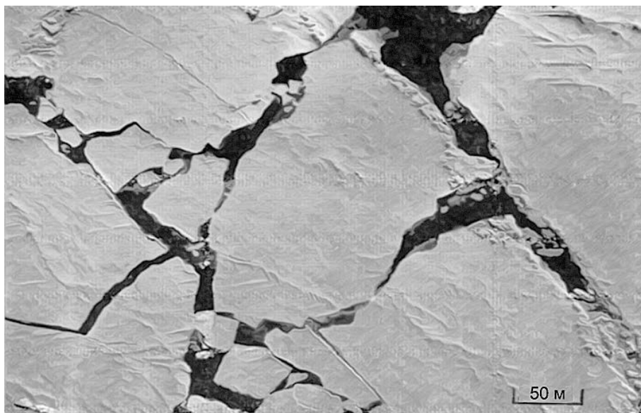
5.1a. Лед после взлома в стадии подвижек. Разлом произошел совсем недавно, о чем можно судить по отсутствию молодого льда в каналах и совпадению контуров соседних льдин.
