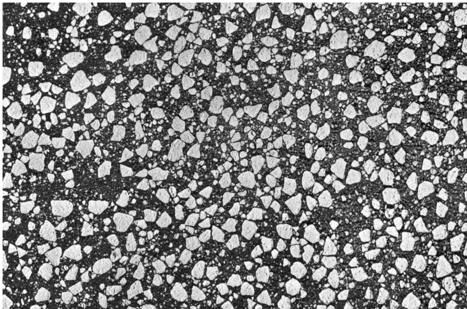
4.3.2.6в. Мелкобитый и тертый лед.
