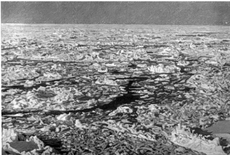
5.1б. Лед на расплыве. Март. Белое море.
