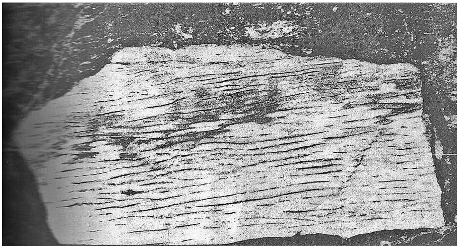
10.4.3в. Ледяной остров. Аэрофотоснимок льдины для СП-18.
