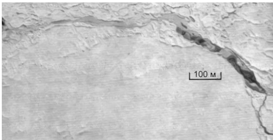
2.6.2а. Двухлетний лед. Апрель, район к востоку от архипелага Шпицберген.
