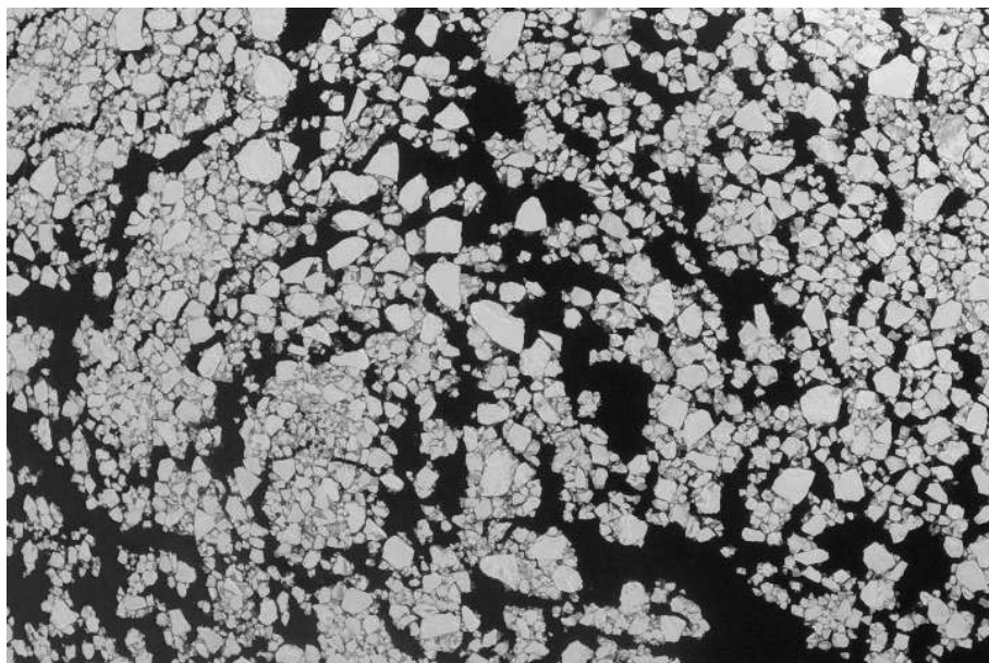
4.2.3б. Сплоченный лед. Апрель. Охотское море.
