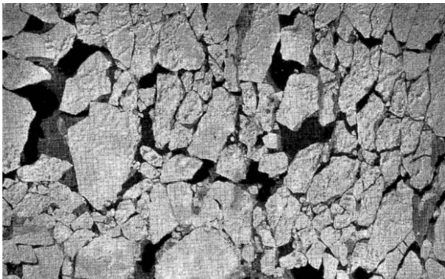
4.2.3а. Сплоченный лед. Обломки полей и крупнобитый лед различного возраста, от серого до однолетнего толстого. На чистой воде между льдинами образуется темный нилас. Апрель. Северная часть Баренцева моря.
