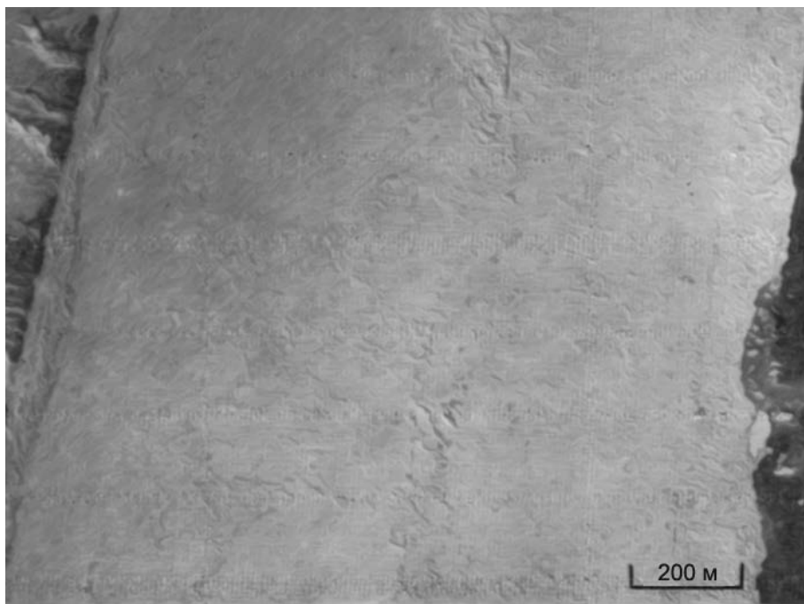
3.1а. Припай однолетнего толстого льда. Вдоль кромки припая полоса смерзшегося тертого льда.
