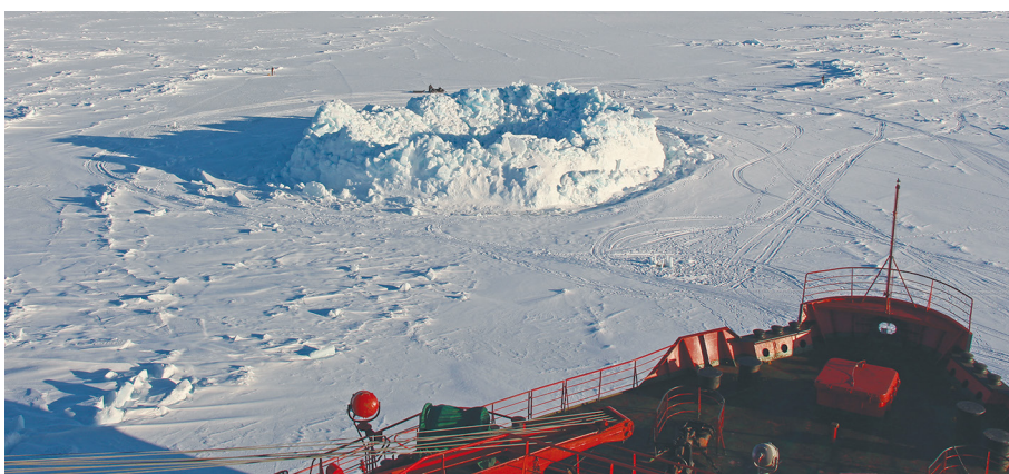
3.4.2ж. Стамуха. Апрель. Каспийском море.
