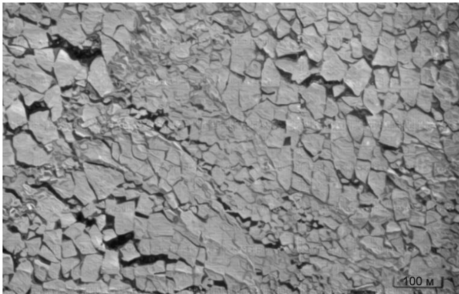
4.2.2б. Очень сплоченный лед (однолетний толстый, слаботоросистый, преимущественно крупнобитый). Апрель. Район западнее Шпицбергена.
