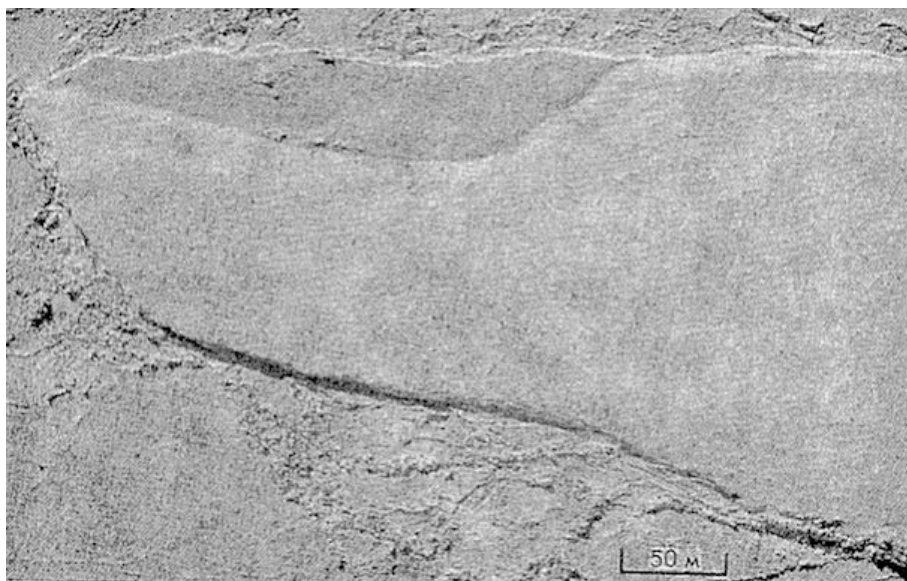
10.4.3а. Часть ледяного дрейфующего острова. Апрель. Арктический бассейн.
