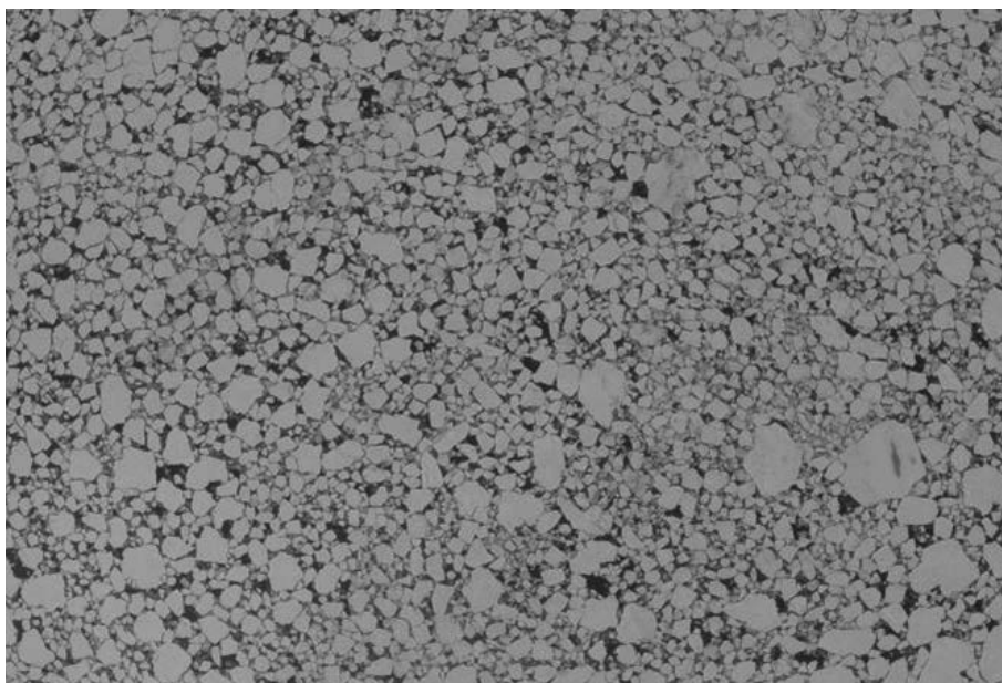
4.2.2в. Очень сплоченный лед. Апрель. Охотское море.
