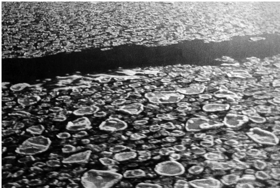
2.3в. Блинчатый лед и кильватерный след. Декабрь. Балтийское море.
