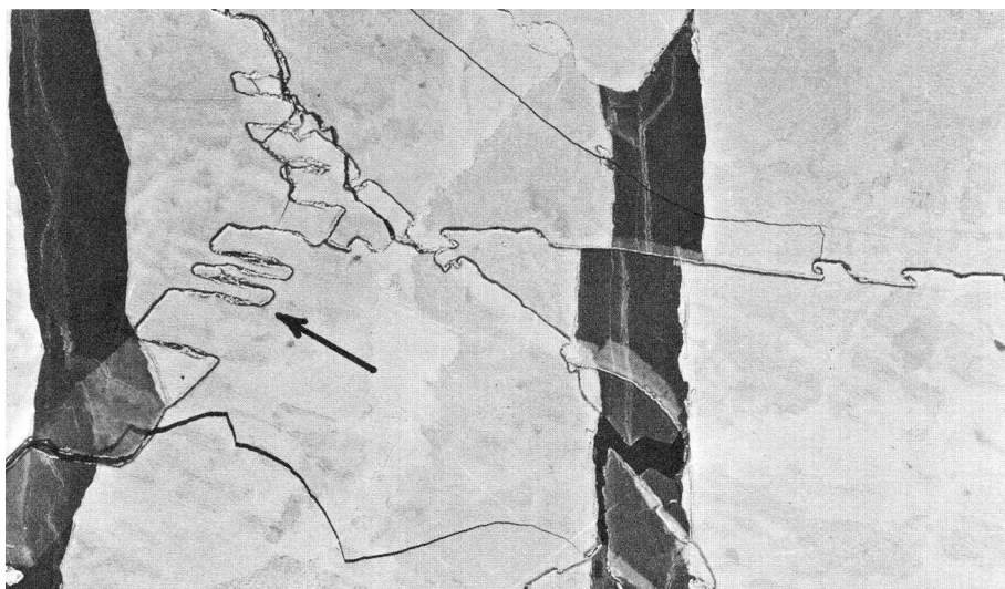
8.2.1.2а. Зубчатонаслоенный лед.
