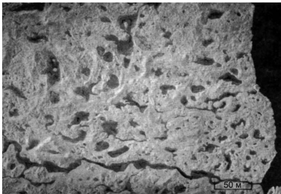
2.6.3д. Часть поля многолетнего льда летом. Август. Северная часть Восточно-Сибирского моря.
