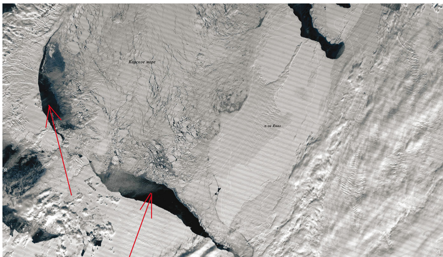
7.4.3б. Стационарная полынья. Апрель. Карское море.
