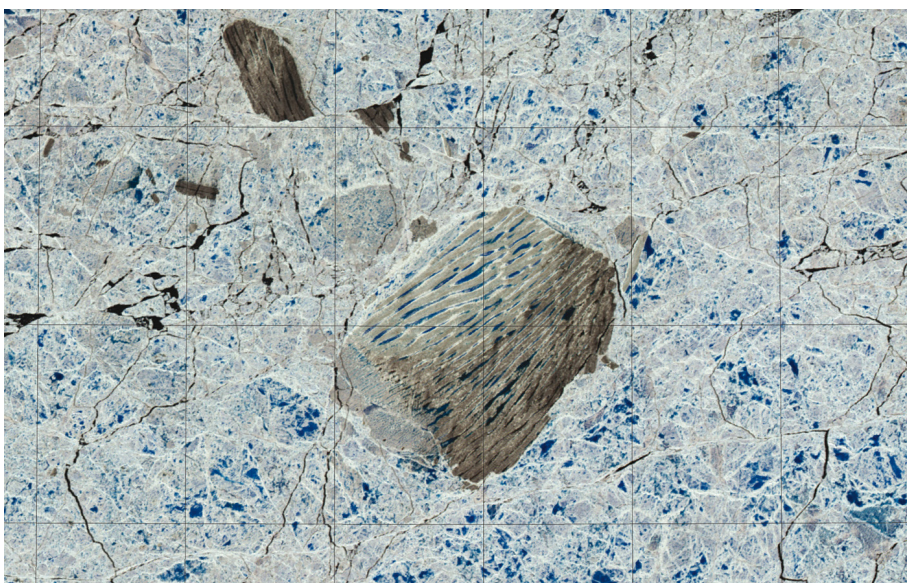
10.4.3г. Ледяной остров. Многоканальное изображение дрейфующего острова Маркхем, полученное 16 июля 2009 г. с помощью прибора ASTER (Advanced Spaceborne Thermal Emission and Reflection Radiometer).
