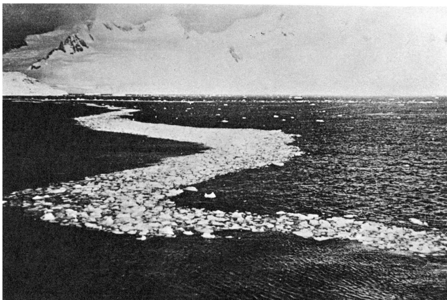
4.4.3г. Пояс льда.
