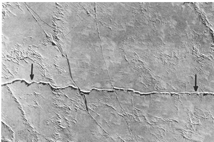
8.2.2д. Гряда торосов в летний период. Апрель. Карское море.
