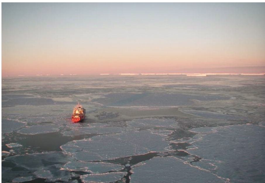
2.4.1д. Обломки полей серого льда. Разрывы заполнены шугой, светлым и темным ниласом. Март 2006 г. Район моря Дейвиса, Антарктика.
