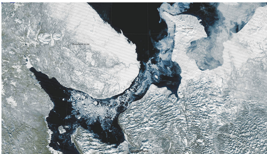
12.6б. Легкий район. Апрель. Белое море.
