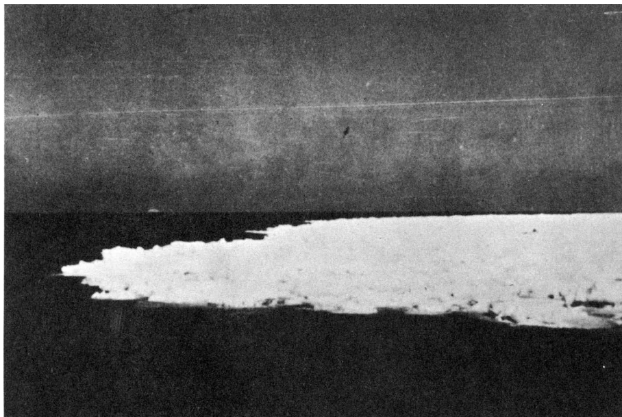
4.4.4а. Язык льда.
