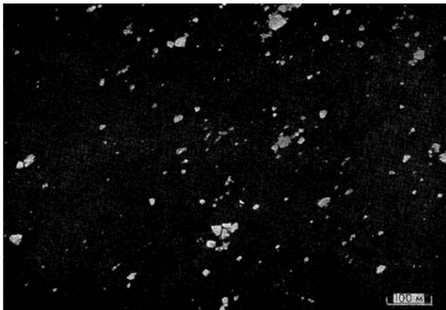
4.2.6а. Отдельные льдины. Крупнобитый и мелкобитый однолетний лед. Апрель. Гренландское море.
