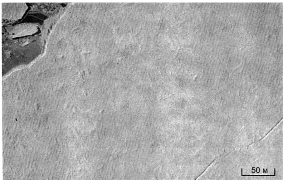
8.2.2.2а. Сглаженный, сильно заснеженный, многолетний лед. Июнь. Приполюсный район.
