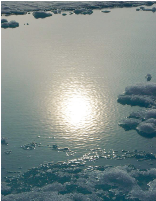
2.2.3а. Склянка на снежнице.
