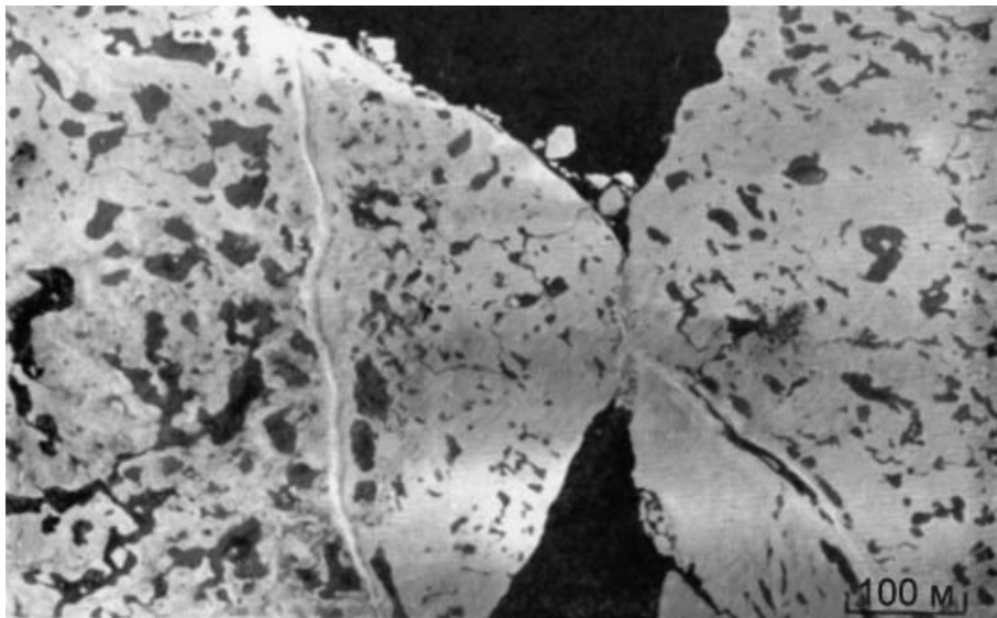
4.4.5.1. Перемычка на стыке многолетних ледяных полей.
