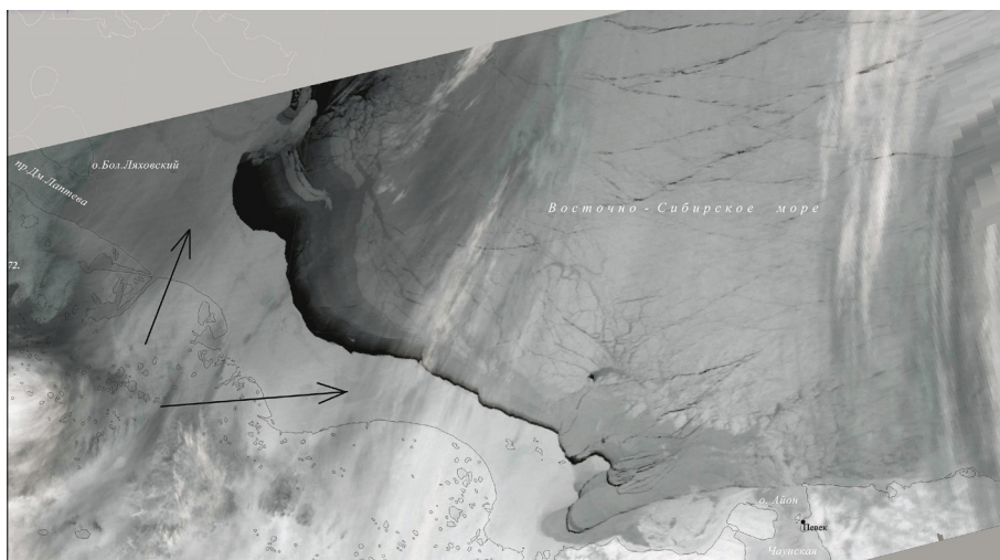
1.1.1б Припай. Радиолокационный снимок. Январь. Восточно-Сибирское море
